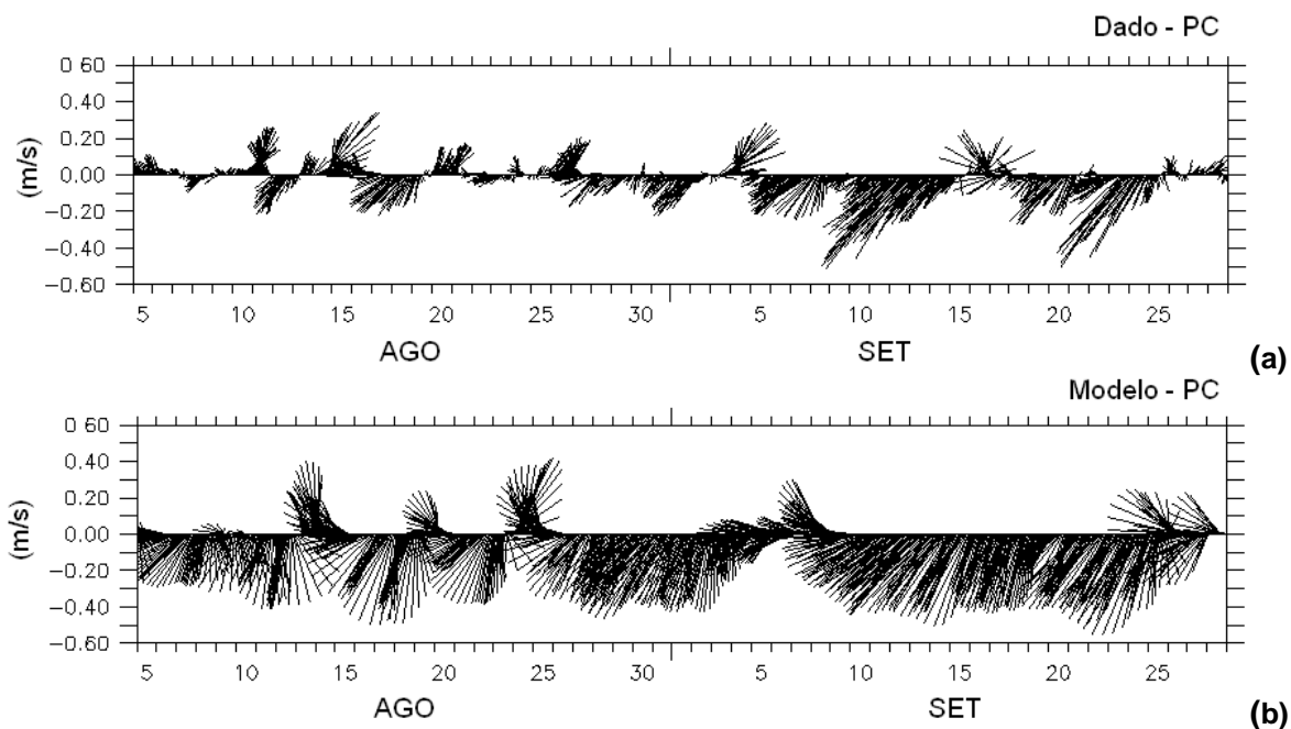
Figura IV.2-4 - Diagrama stick plot dos vetores de corrente medida no Ponto PC (a) e calculada pelo modelo (b) entre os dias 5 de agosto e 28 de setembro de 1992.
