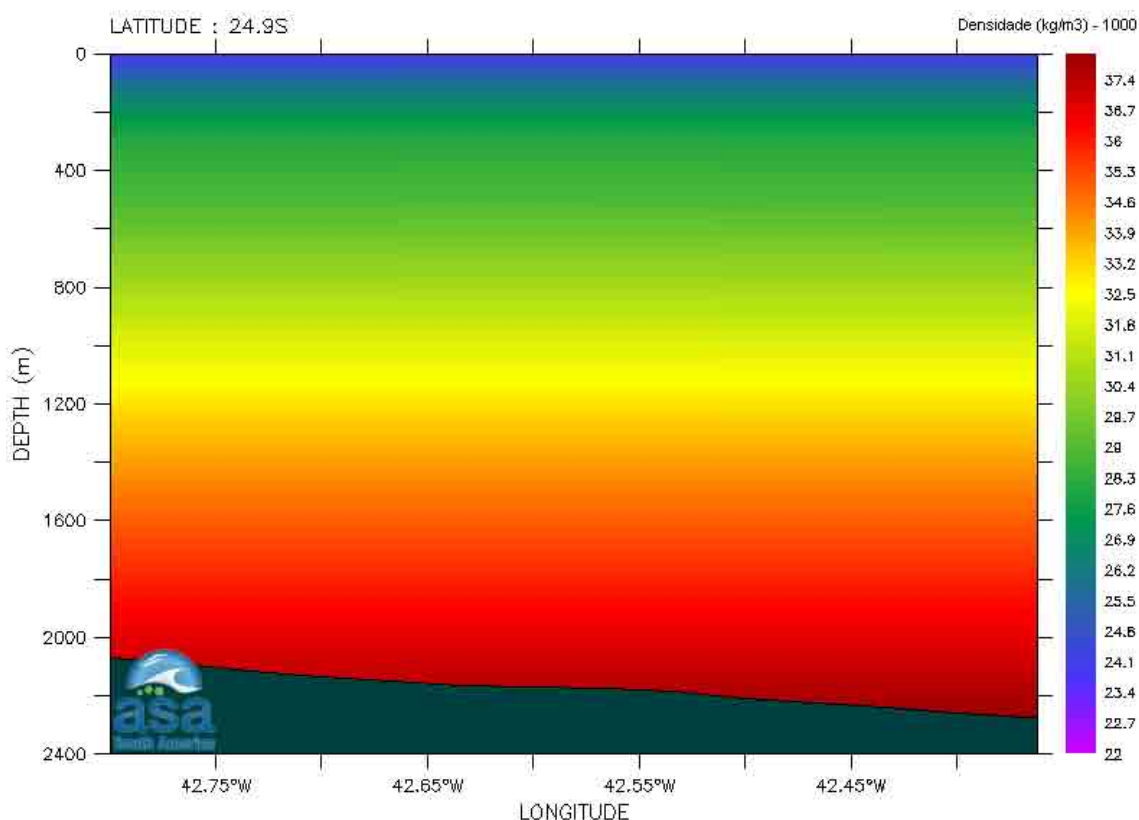
Figura II.4-1 - Seção vertical de densidade ( \text{kg/m}^3 ) ao longo de 24,9°S para o período de janeiro a março (verão), Área do Pré-Sal.
