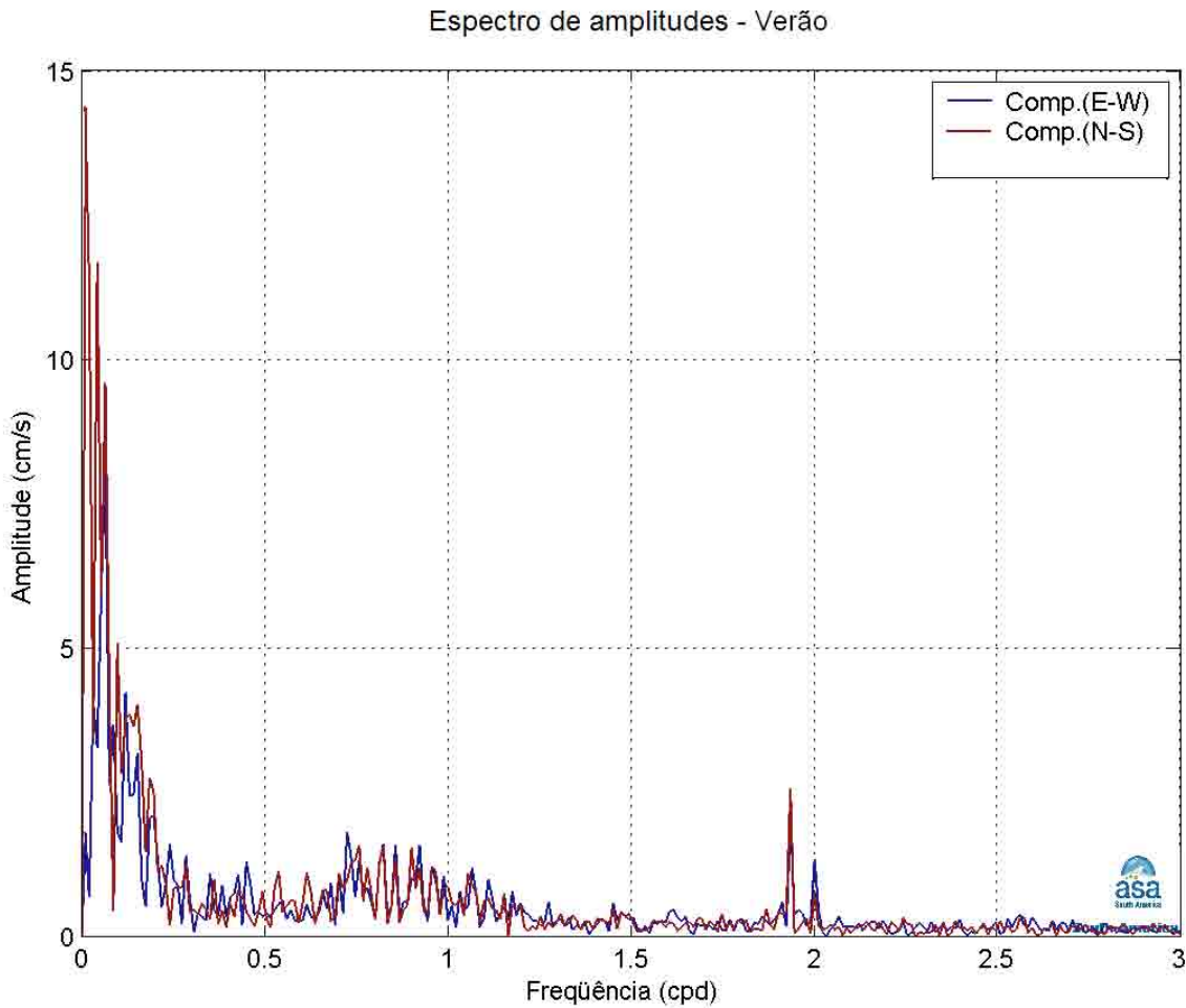
Figura II.2-7 - Espectro de amplitudes (cm/s) da corrente registrada no fundeio BM/333 do experimento ACM12 do WOCE, medida a 230 m de profundidade. Verão de 1992, intervalo de amostragem: 2h.
