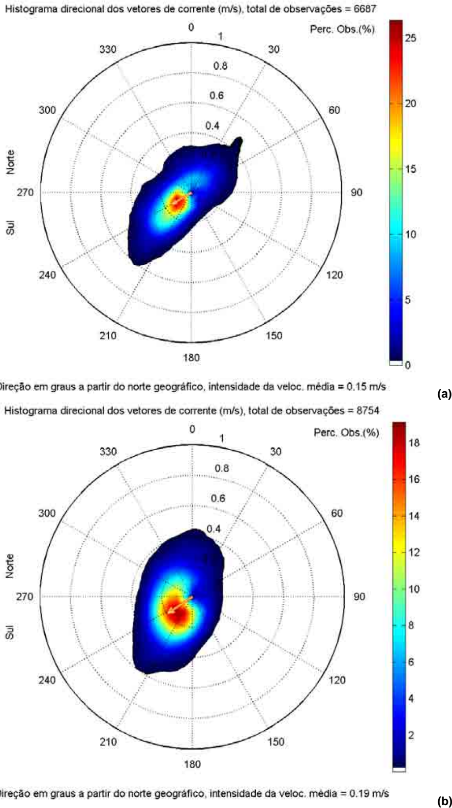
Figura IV.2-9 - Velocidade média e histograma direcional dos vetores de corrente medidos na região do ponto PC (a), e resultantes da simulação numérica (b), para o período de janeiro a dezembro de 1992.
