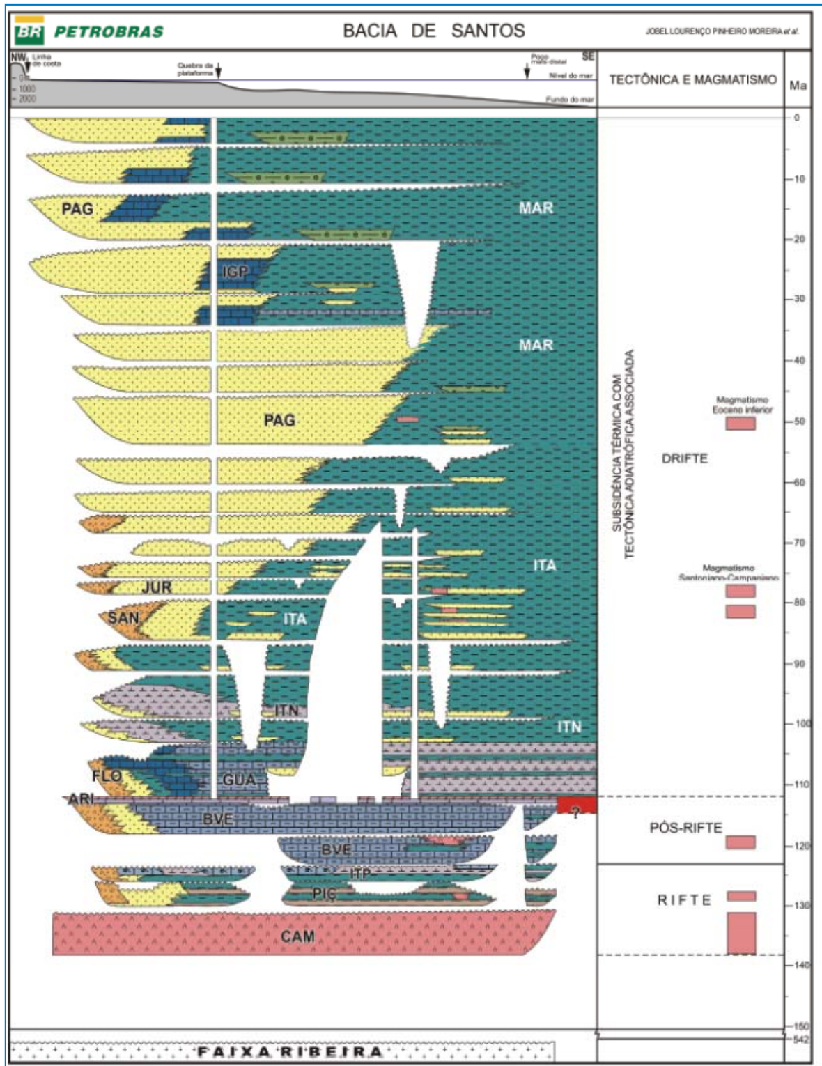
Figura II.5.1.4-8 - Coluna estratigráfica esquemática da Bacia de Santos.
