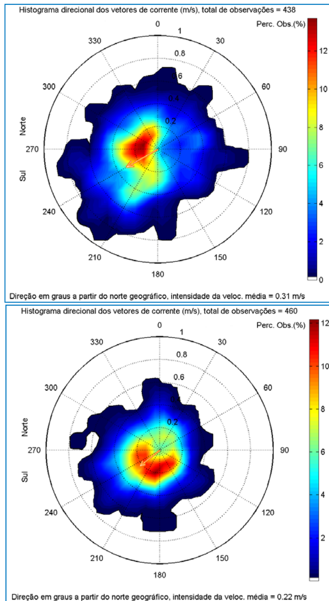
Figura II.5.1.2-34 - Histograma direcional dos vetores de corrente do HYCOM em superfície para janeiro a março (a) e junho a agosto (b) de 2004 a 2008.
