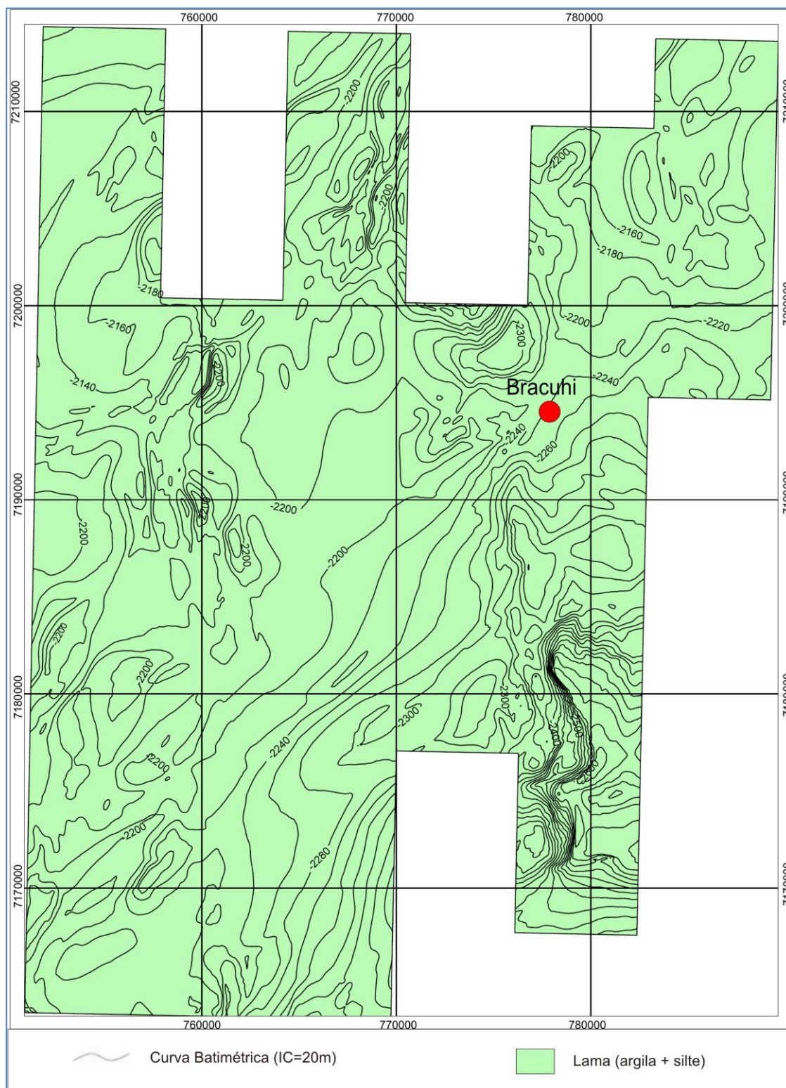
Figura II.5.1.4-21 - Mapa faciológico local - Área de Júpiter e Bracuhi (Bloco BM-S-24).
