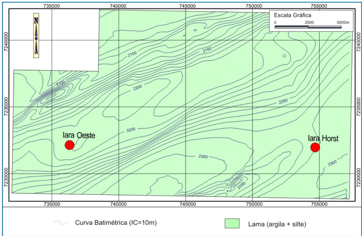
Figura II.5.1.4-16 - Mapa faciológico local - Área de lara (Bloco BM-S-11).
