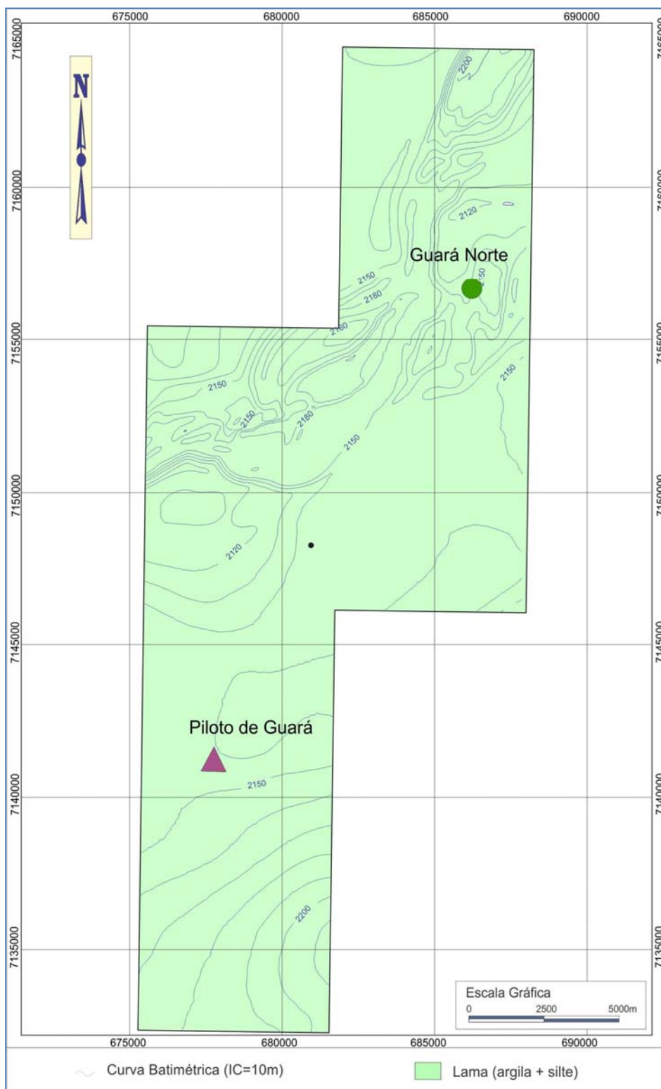
Figura II.5.1.4-19 - Mapa faciológico local - Área de Guarás (Bloco BM-S-9).
