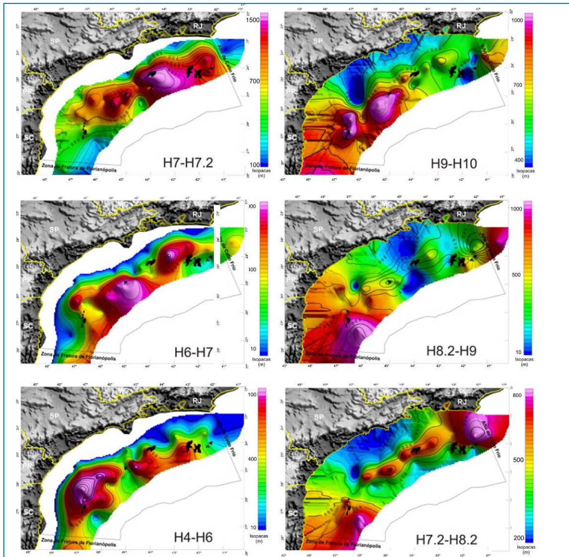
Figura II.5.1.4-4 - Mapas de isópacos de diferentes seqüências da Bacia de Santos, mostrando: a) migração dos depocentros para nordeste no Cretáceo superior (H4 - H7.2); b) definição de um depocentro alongado NE/SW na parte central da bacia, que se torna proeminente na porção norte da bacia, no intervalo Paleoceno /Oligoceno inferior H7.2 - H8.2); c) implantação de importante depocentro terciário na porção sul da bacia (H7.2 - H10).
