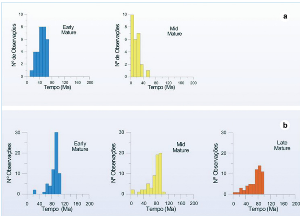
Figura II.5.1.4-10 - Distribuição temporal da maturação. a) gerador Itajaí-Açu. b) gerador Guaratiba. Early Mature corresponde ao estágio inicial de maturação (0.5 < Ro% < 0.7). Mid Mature corresponde ao pico de maturação (0.7 < Ro% < 1.0). Late Mature corresponde à fase final de geração (1.0 < Ro% < 1.3).
