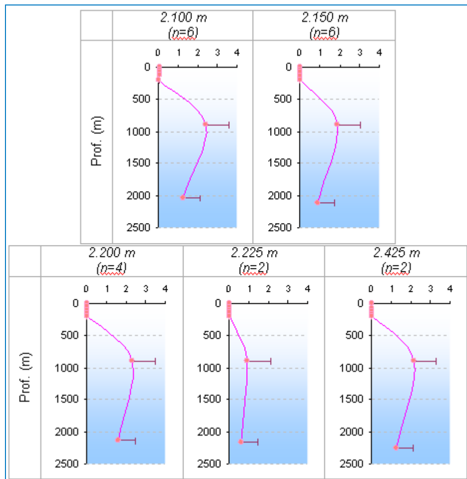
Figura II.5.1.3-16 - Valores médios de nitrito ( \mu\text{mol.L}^{-1} ) encontrados na Bacia de Santos.
