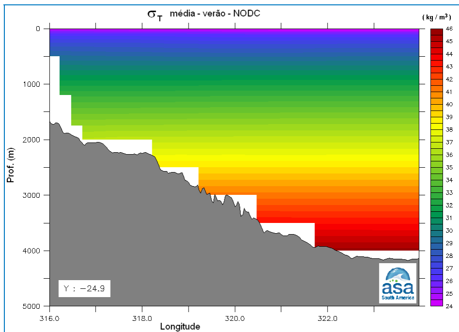
Figura II.5.1.2-8 - Seção vertical de \sigma_T (kg/m³) ao longo de 24,90°S para o período de janeiro a março (verão), de acordo com os dados do NODC.
