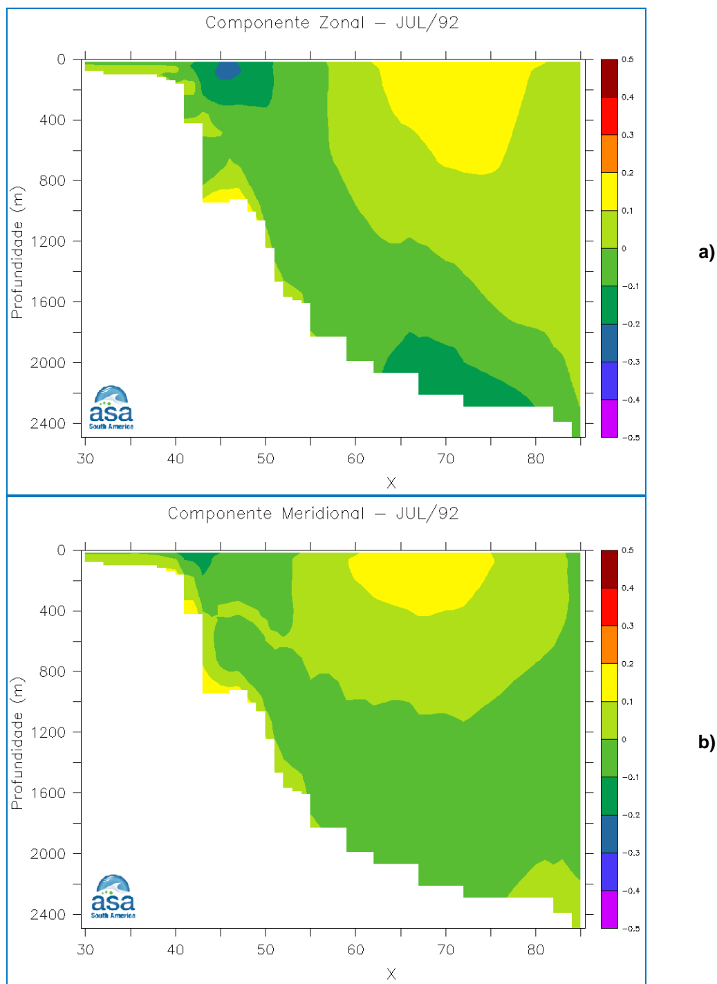
Figura II.5.1.2-40 - Seções de velocidade (m/s) zonal (a) e meridional (b), médias para julho de 1992, extraídas ao longo da linha amarela indicada na Figura II.5.1.2-39 .
