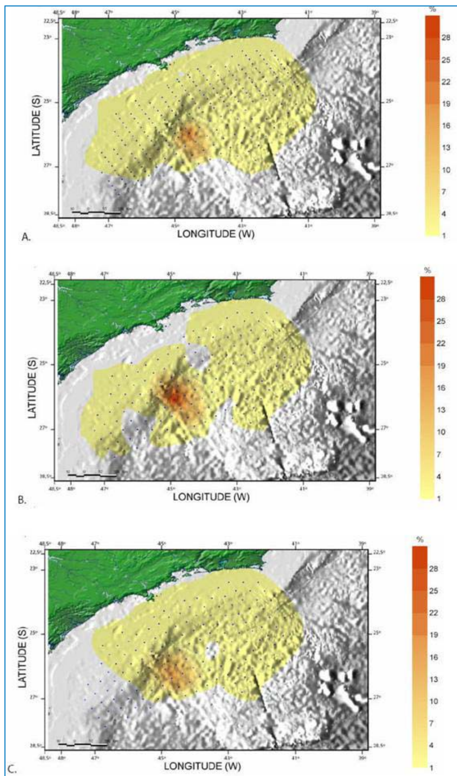
Figura II.5.1.3-2 - Variação Espacial das Concentrações de Carbono Orgânico Total na Bacia de Santos. A) Superfície, B) Termocline e C) Fundo.
