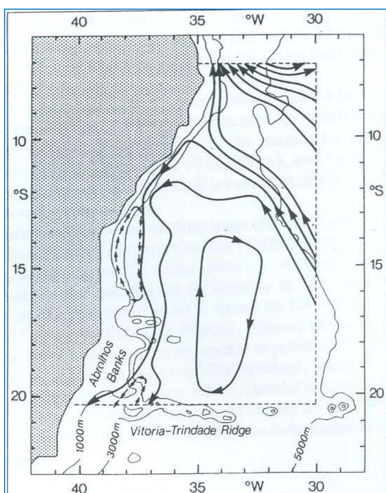
Figura II.5.1.2-18 - Representação esquemática do campo de fluxo geostrófico nos primeiros 500 m, com base em dados hidrográficos históricos, coletados na região demarcada.
