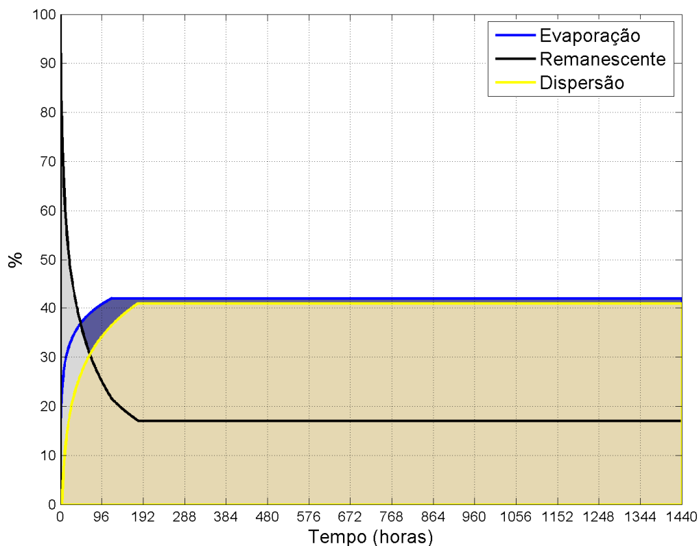
Figura II.6.1.1-50 - Evolução temporal do balanço de massa ao longo da simulação da trajetória do volume de pior caso ( 116.076 \text{ m}^3 ) em condições meteorológicas frequentes, no cenário de inverno.
