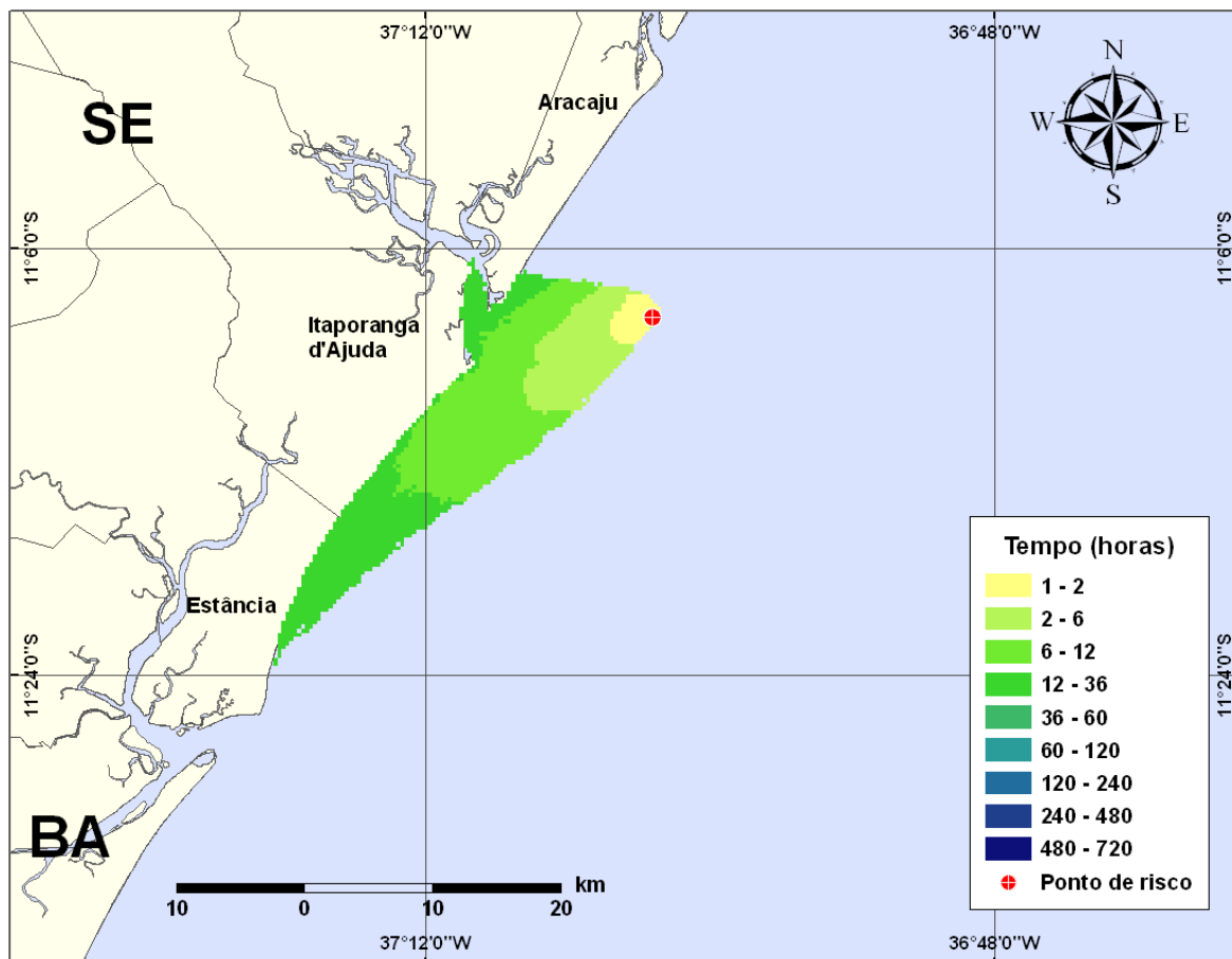
Figura III-10 - Cenário PGA3_DIESEL_VER_500_30D. (Fase: instalação/perfuração). Contornos de deslocamento de óleo na água para um acidente com óleo tipo DIESEL, ocorrendo no Ponto-PGA3, do Campo Guaricema, durante os meses de verão (janeiro a março), com derrame de 500 m 3 (instantâneo), após 30 dias de simulação.
