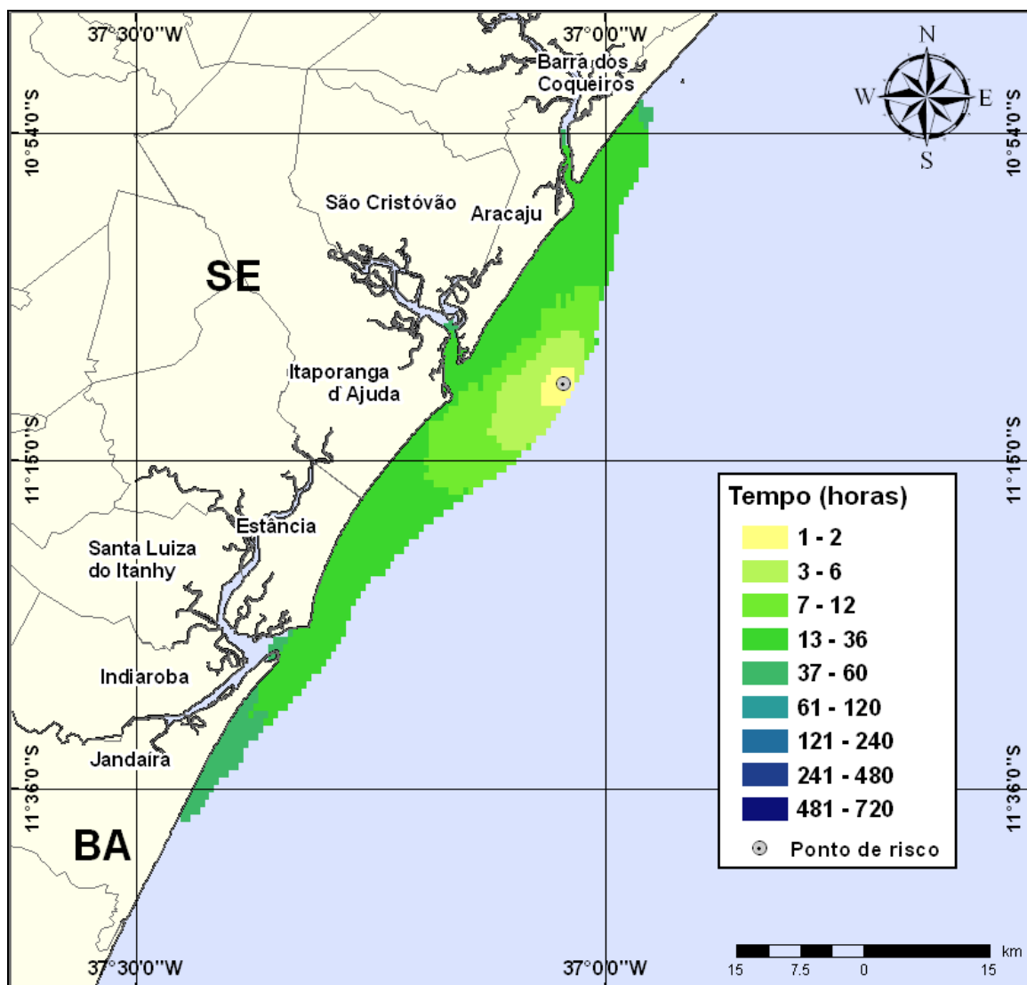
Figura III-86 - Cenário PGA10_INV_8_30D (Fase:instalação/produção/perfuração). Contornos de deslocamento de óleo na água para um acidente com óleo tipo GUARICEMA ocorrendo no Ponto-PGA10, durante os meses de inverno (junho a agosto), com derrame de 8 \text{ m}^3 (instantâneo), após 30 dias de simulação.
