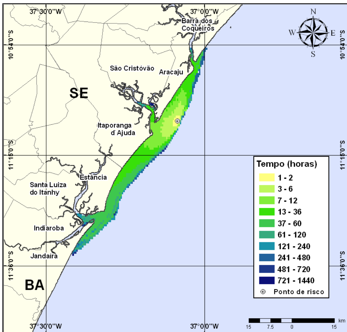
Figura III-106 - Cenário PE5_INV_7500_60D (Fase: perfuração). Contornos de deslocamento de óleo na água para um acidente com óleo tipo GUARICEMA ocorrendo no Ponto-PE5, durante os meses de inverno (junho a agosto), com derrame de 7.500 m 3 (ao longo de 30 dias), após 60 dias de simulação.
