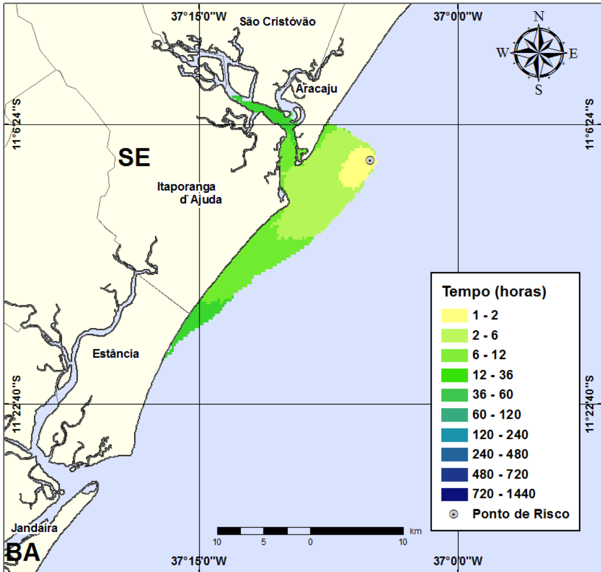
Figura III-38 - Cenário PE5_VER_8_30D (Fase: perfuração). Contornos de deslocamento de óleo na água para um acidente com óleo tipo GUARICEMA ocorrendo no Ponto-PE5, durante os meses de verão (janeiro a março), com derrame de 8 m 3 (instantâneo), após 30 dias de simulação.
