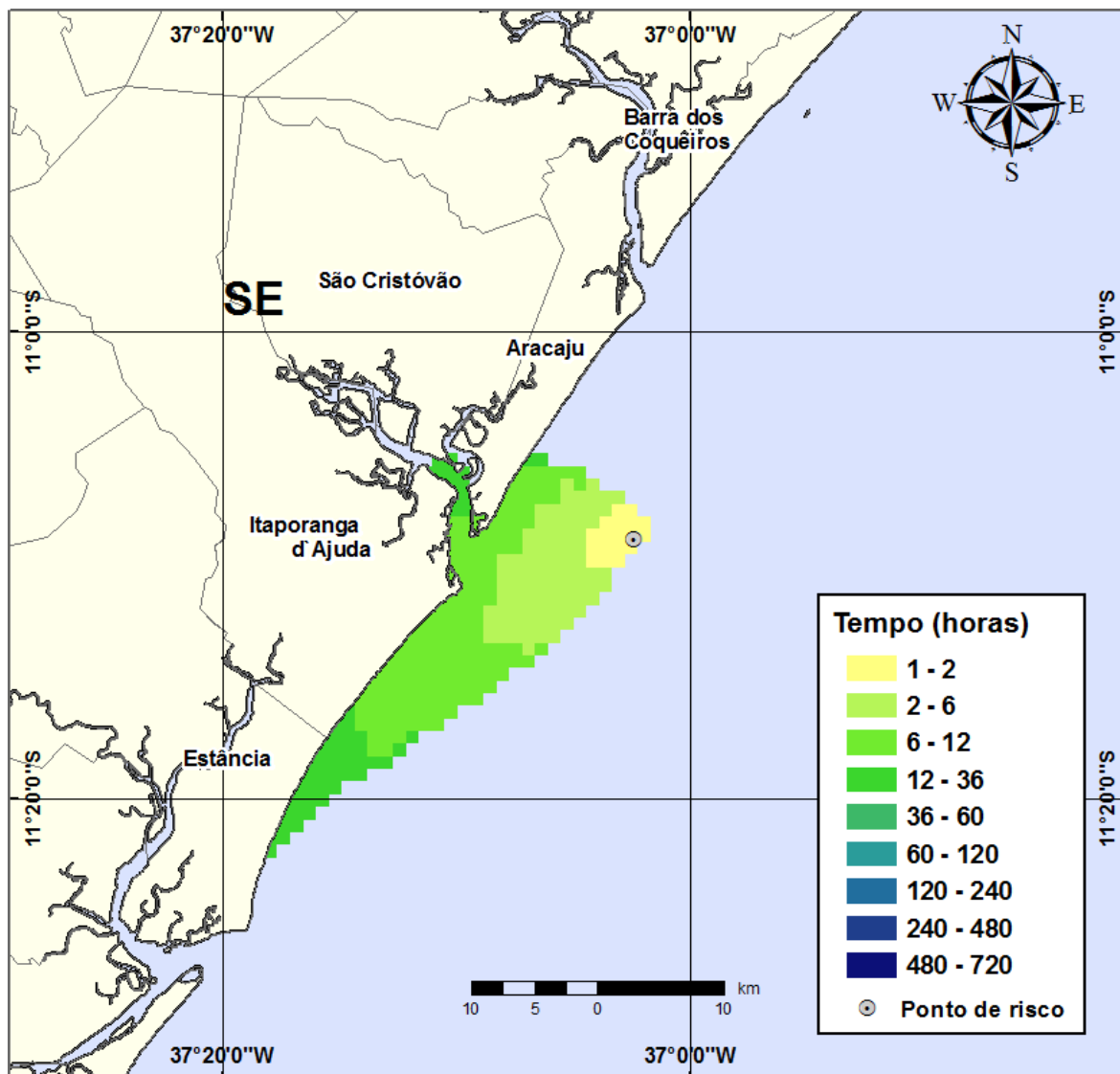
Figura III-22 - Cenário PGA3_VER_264_30D. (Fase: produção). Contornos de deslocamento de óleo na água para um acidente com óleo tipo GUARICEMA, ocorrendo no Ponto-PGA3, do Campo Guaricema, durante os meses de verão (janeiro a março), com derrame de 264 m 3 (instantâneo), após 30 dias de simulação.
