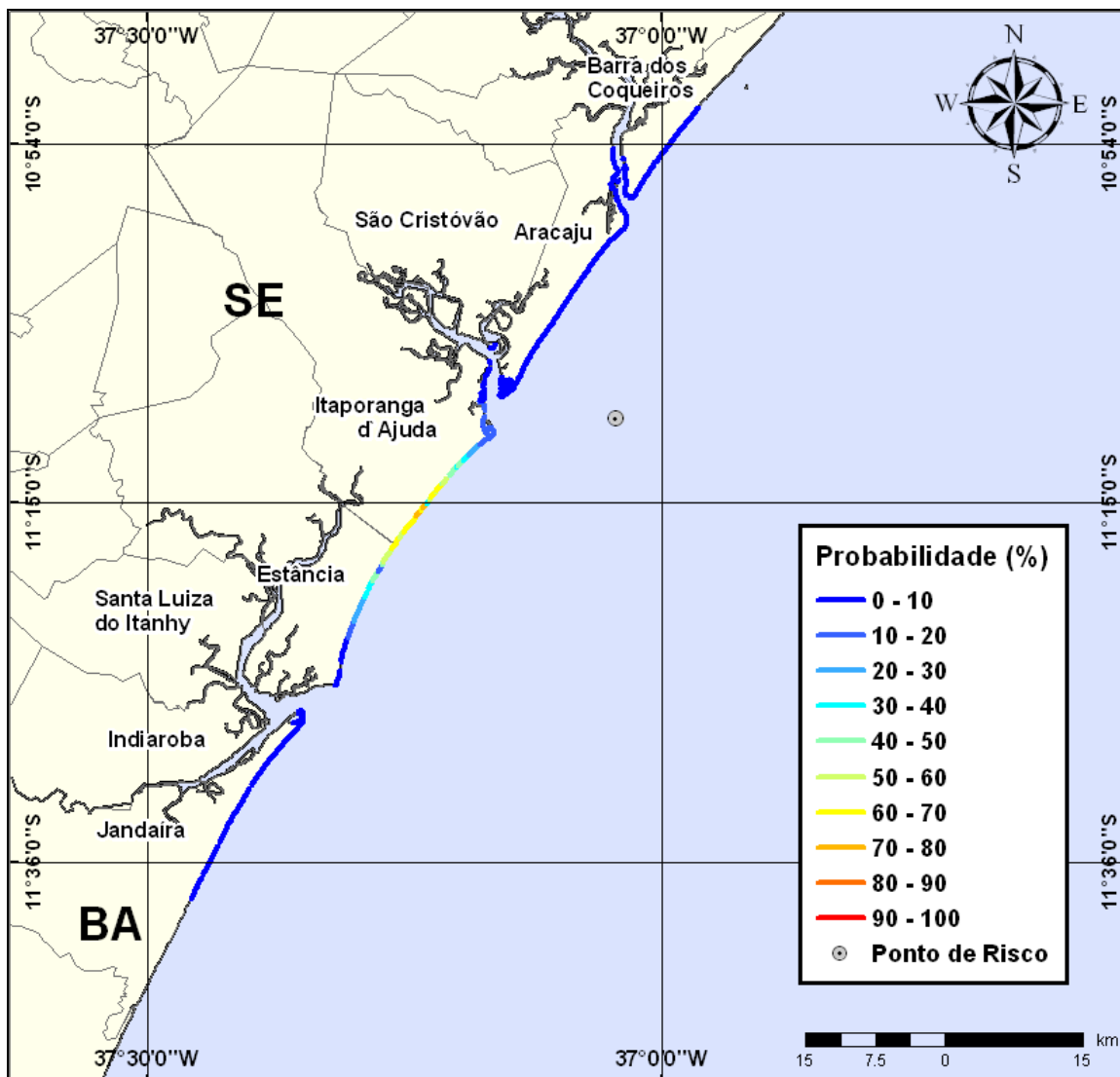
Figura III-87 - Cenário PGA10_INV_8_30D (Fase: Fase:instalação/produção/perfuração). Linhas de probabilidade de óleo na costa para um acidente com óleo tipo GUARICEMA ocorrendo no Ponto-PGA10, durante os meses de inverno (junho a agosto), com derrame de 8 \text{ m}^3 (instantâneo), após 30 dias de simulação.
