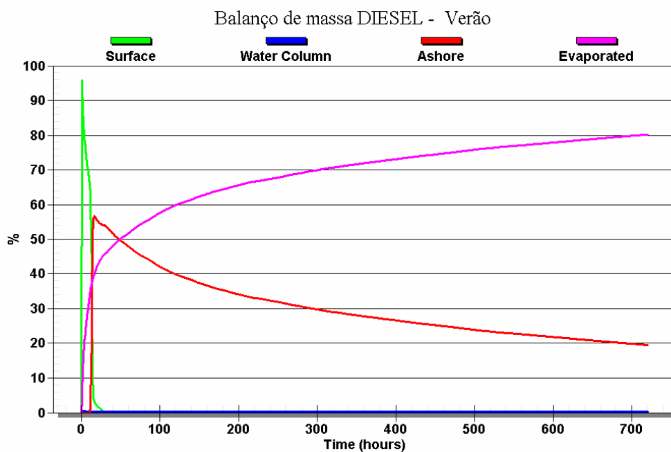
Figura III-122- Balanço de massa do cenário DET_PGA31_DIESEL_VER_500_30D.
