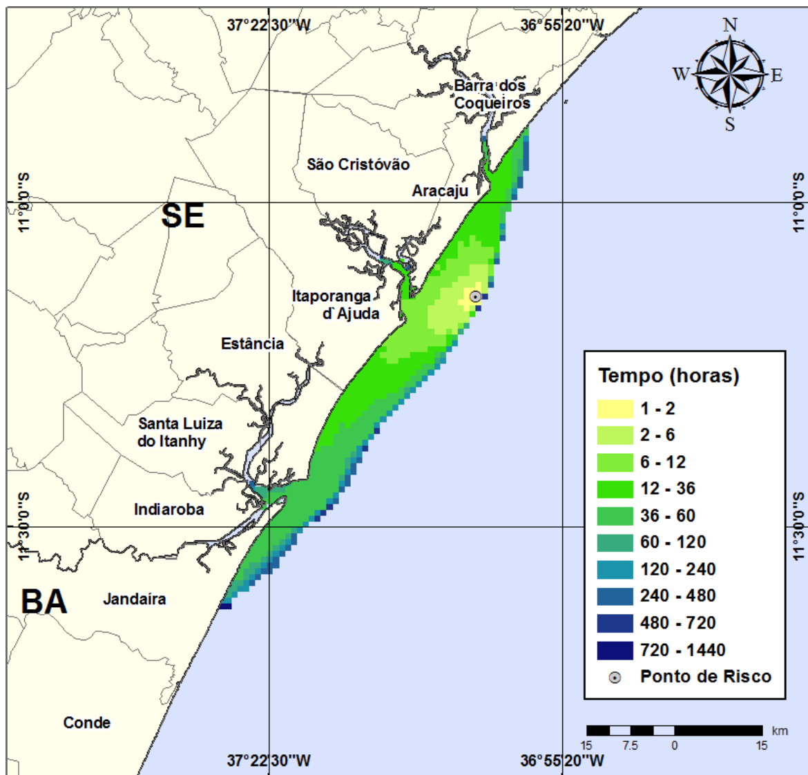
Figura III-110 - Cenário GA07_INV_7500_60D. (v). Contornos de deslocamento de óleo na água para um acidente com óleo tipo GUARICEMA, ocorrendo no Ponto-GA07, do Campo Guaricema, durante os meses de inverno (junho a agosto), com derrame de 7.500 m 3 (ao longo de 30 dias), após 60 dias de simulação.
