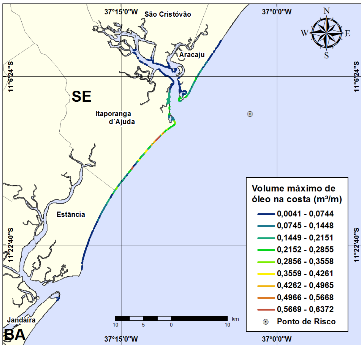
Figura III-36 - Cenário PGA10_VER_PC_60D (Fase: perfuração). Linhas de volume máximo de óleo na costa para um acidente com óleo tipo GUARICEMA ocorrendo no Ponto-PGA10, durante os meses de verão (janeiro a março), com derrame de 7.500 m 3 (ao longo de 30 dias), após 60 dias de simulação.
