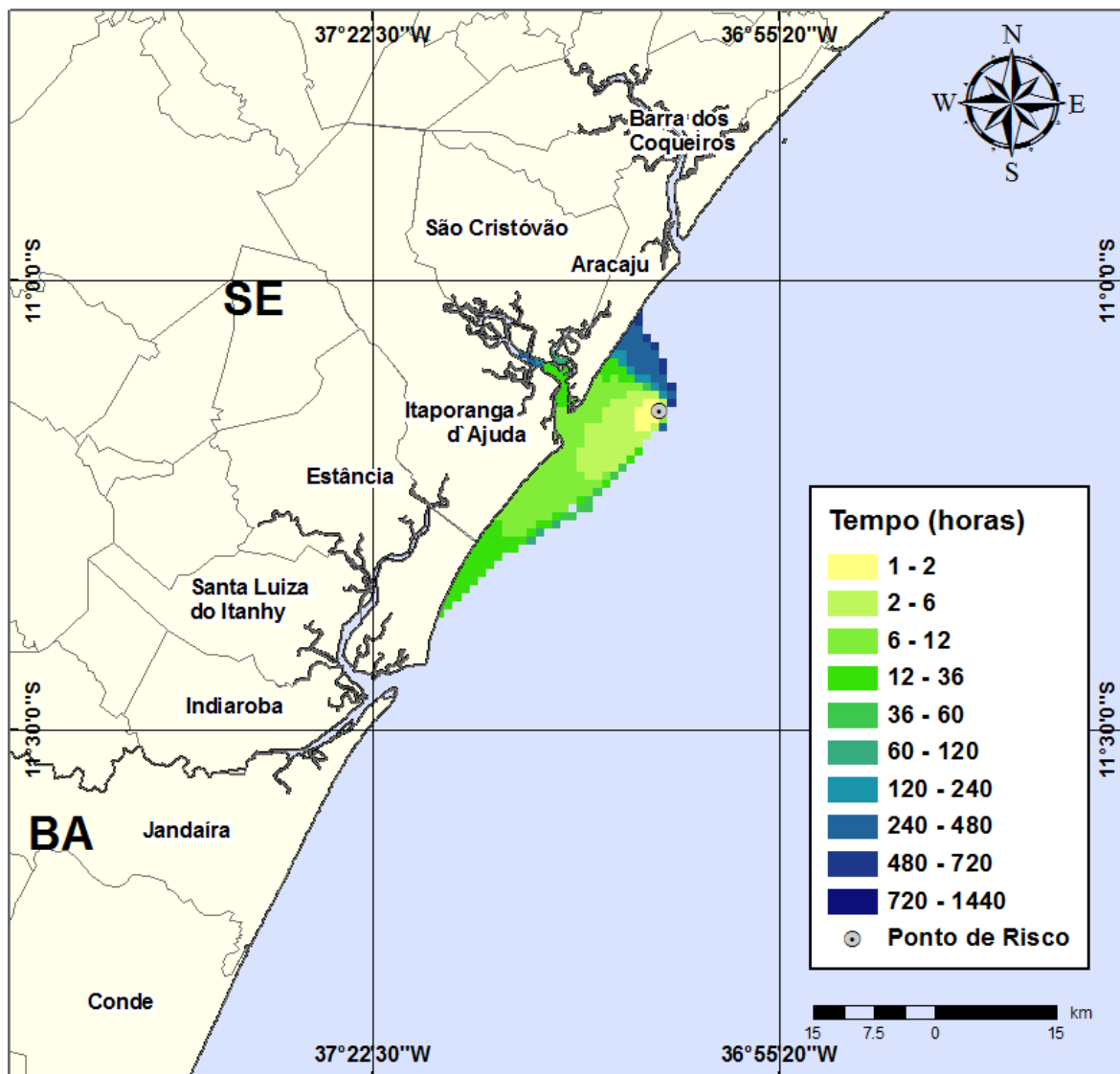
Figura III-50 - Cenário GA07_VER_7500_60D. (Fase: produção). Contornos de deslocamento de óleo na água para um acidente com óleo tipo GUARICEMA, ocorrendo no Ponto-GA07, do Campo Guaricema, durante os meses de verão (janeiro a março), com derrame de 7.500 m 3 (ao longo de 30 dias), após 60 dias de simulação.
