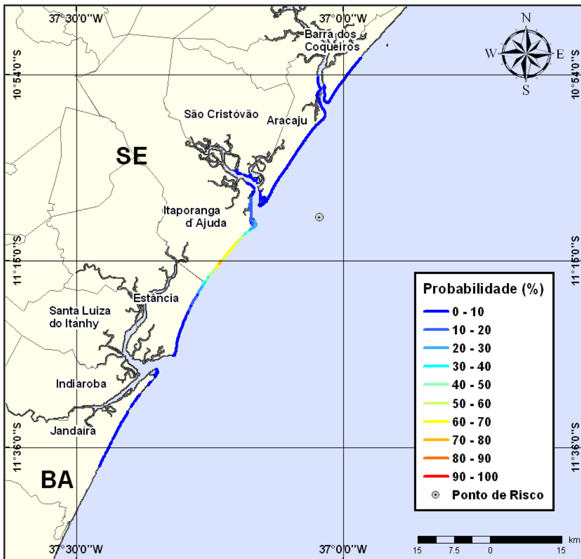
Figura III-91 - Cenário PGA10_INV_200_30D (Fase:instalação/produção/perfuração). Linhas de probabilidade de óleo na costa para um acidente com óleo tipo GUARICEMA ocorrendo no Ponto-PGA10, durante os meses de inverno (junho a agosto), com derrame de 200 m 3 (instantâneo), após 30 dias de simulação.
