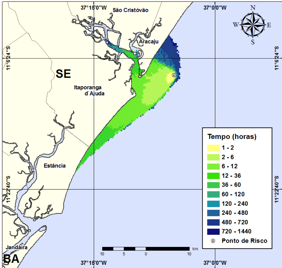
Figura III-46 - Cenário PE5_VER_7500_30D (Fase: perfuração) Contornos de deslocamento de óleo na água para um acidente com óleo tipo GUARICEMA ocorrendo no Ponto-PE5, durante os meses de verão (janeiro a março), com derrame de 7.500 m 3 (ao longo de 30 dias), após 60 dias de simulação.
