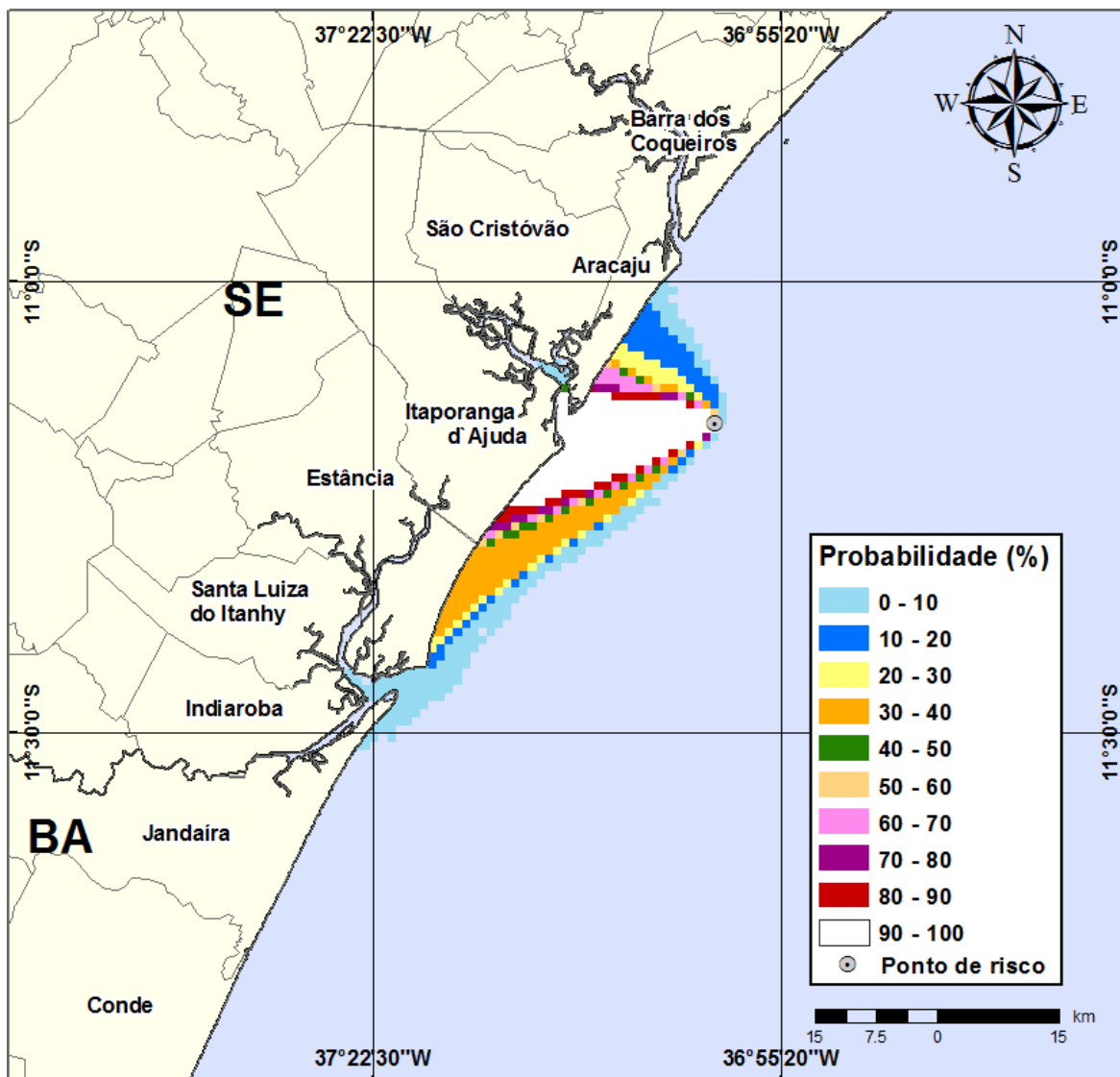
Figura III-57 - Cenário GA64_VER_7500_60D. (Fase: produção). Contornos de probabilidade de óleo na água para um acidente com óleo tipo GUARICEMA, ocorrendo no Ponto-GA64, do Campo Guaricema, durante os meses de verão (janeiro a março), com derrame de 7.500 m 3 (ao longo de 30 dias), após 60 dias de simulação.
