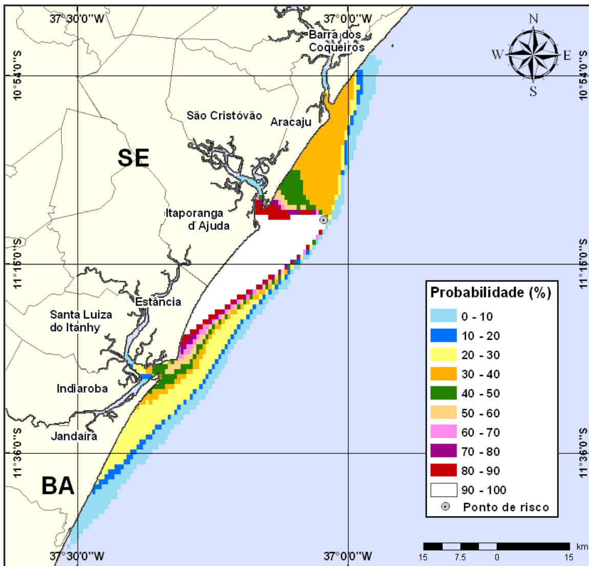
Figura III-93 - Cenário PGA10_INV_7500_60D (Fase: perfuração). Contornos de probabilidade de óleo na água para um acidente com óleo tipo GUARICEMA ocorrendo no Ponto-PGA10, durante os meses de inverno (junho a agosto), com derrame de 7.500 m 3 (ao longo de 30 dias), após 60 dias de simulação.
