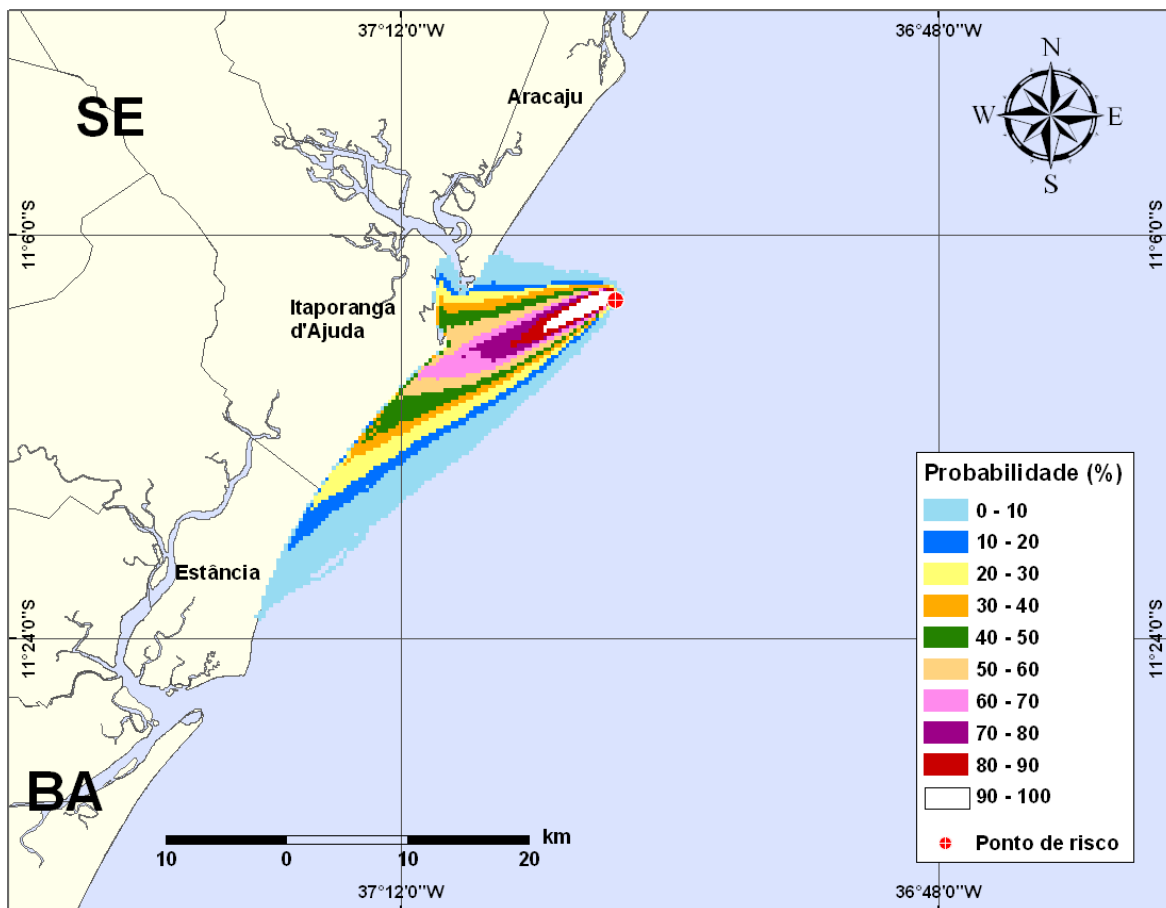
Figura III-1 - Cenário PGA3_DIESEL_VER_8_30D . (Fase: instalação/perfuração). Contornos de probabilidade de óleo na água para um acidente com óleo tipo DIESEL, ocorrendo no Ponto-PGA3, do Campo Guaricema, durante os meses de verão (janeiro a março), com derrame de 8 m 3 (instantâneo), após 30 dias de simulação.
