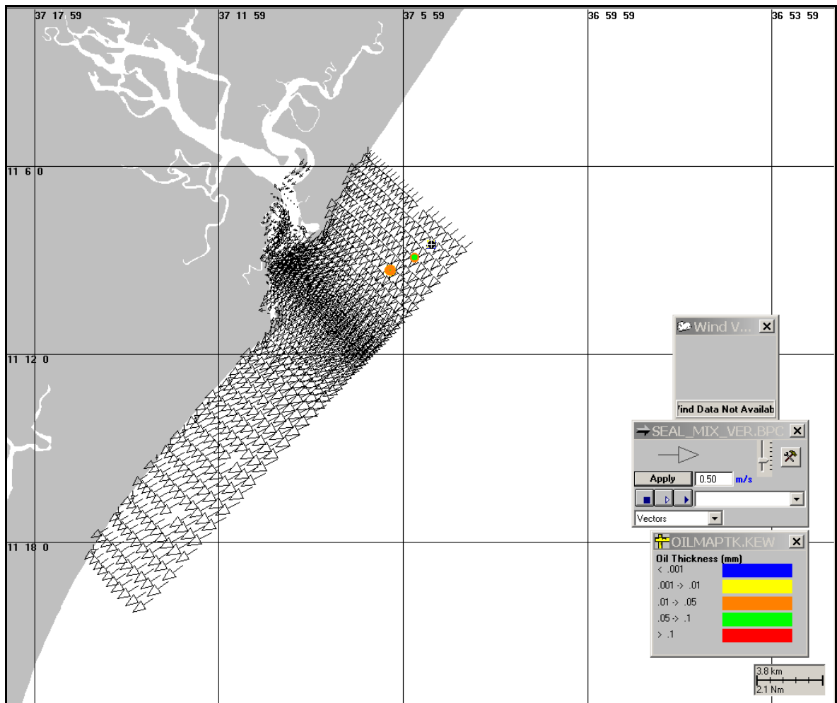
Figura III-132 - Cenário DET_PE5_INV_7500_60D. Condições meteorológicas e oceanográficas e espessuras da mancha de óleo no início da simulação.
