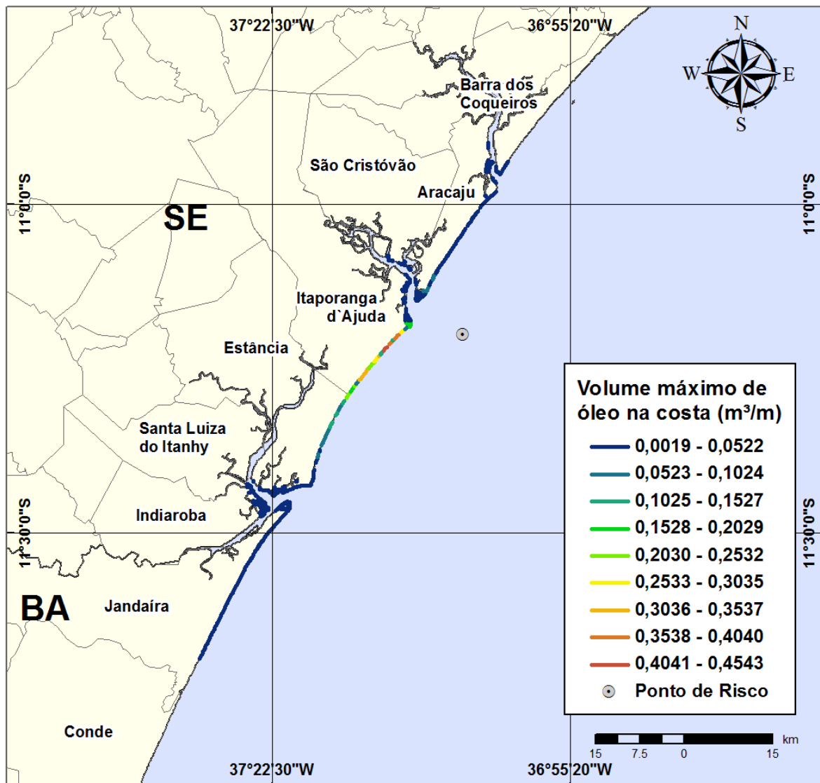
Figura III-116 - Cenário GA58_INV_7500_60D. (Fase: produção). Linhas de volume máximo de óleo na costa para um acidente com óleo tipo GUARICEMA, ocorrendo no Ponto-GA58, do Campo Guaricema, durante os meses de inverno (junho a agosto), com derrame 7.500 m 3 (ao longo de 30 dias), após 60 dias de simulação.
