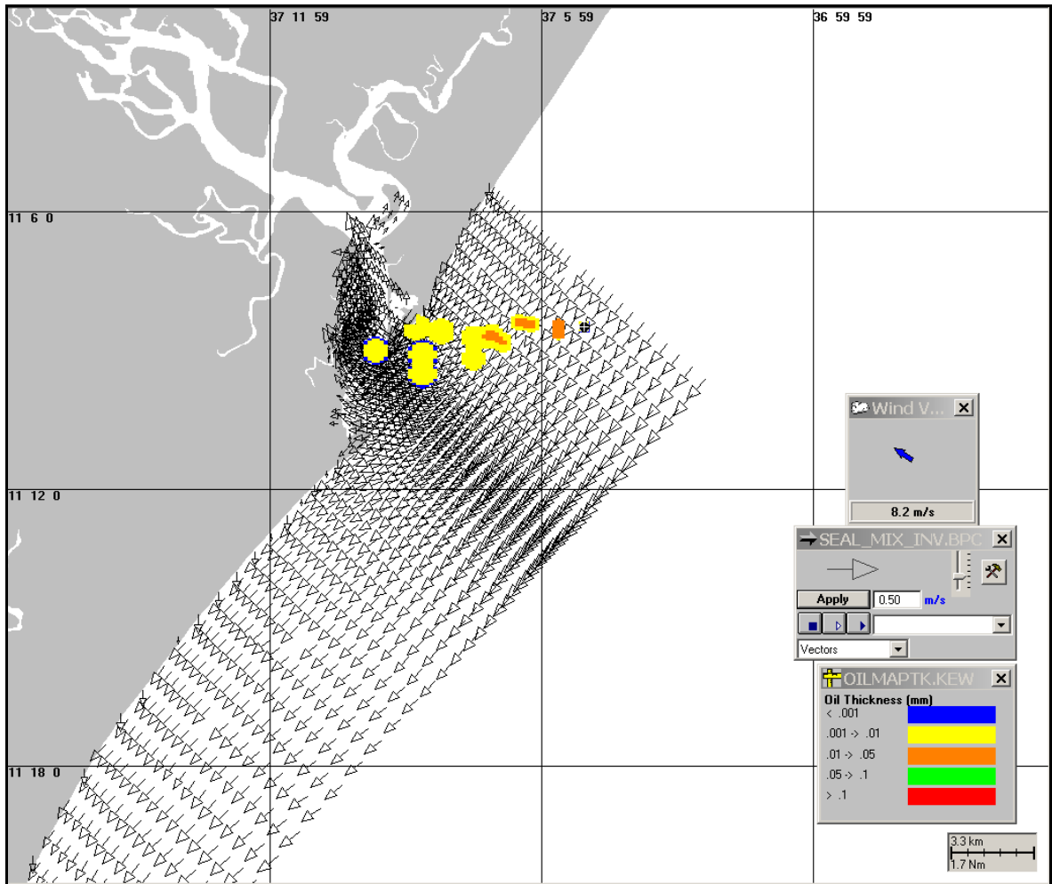
Figura III-134 - Cenário DET_PE5_INV_7500_60D. Condições meteorológicas e oceanográficas e espessuras da mancha de óleo no instante de primeiro toque na costa da simulação.
