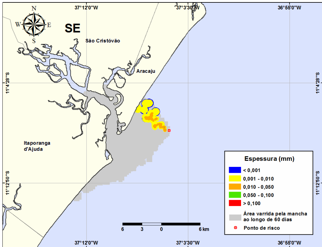
Figura III-137 - DET_FREQ_PE5_INV_7500_60D. Cenário determinístico para a condição mais frequente, para um derrame ocorrido durante o inverno com óleo cru, a partir do Ponto-PE5 no Campo Guaricema.
