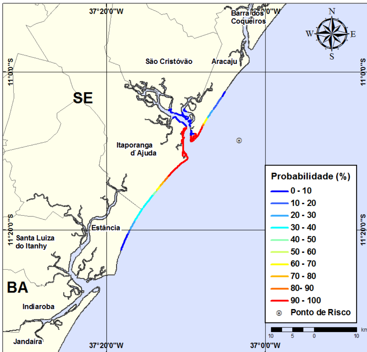
Figura III-51 - Cenário GA07_VER_7500_60D. (Fase: produção). Linhas de probabilidade de óleo na costa para um acidente com óleo tipo GUARICEMA, ocorrendo no Ponto-GA07, do Campo Guaricema, durante os meses de verão (janeiro a março), com derrame de 7.500 m 3 (ao longo de 30 dias), após 60 dias de simulação.
