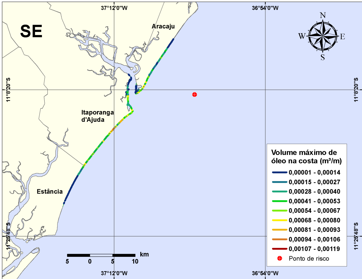
Figura III-64 - Cenário PGA3_DIESEL_INV_8_30D. (Fase: instalação/perfuração). Linhas de volume máximo de óleo na costa para um acidente com óleo tipo DIESEL, ocorrendo no Ponto-PGA3, do Campo Guaricema, durante os meses de inverno (junho a agosto), com derrame de 8 m³ (instantâneo), após 30 dias de simulação.
