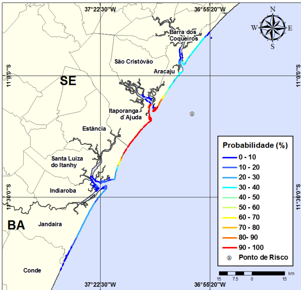
Figura III-119 - Cenário GA64_INV_7500_60D. (Fase: produção). Linhas de probabilidade de óleo na costa para um acidente com óleo tipo GUARICEMA, ocorrendo no Ponto-GA64, do Campo Guaricema, durante os meses de inverno (junho a agosto), com derrame de 7.500 m 3 (ao longo de 30 dias), após 60 dias de simulação.
