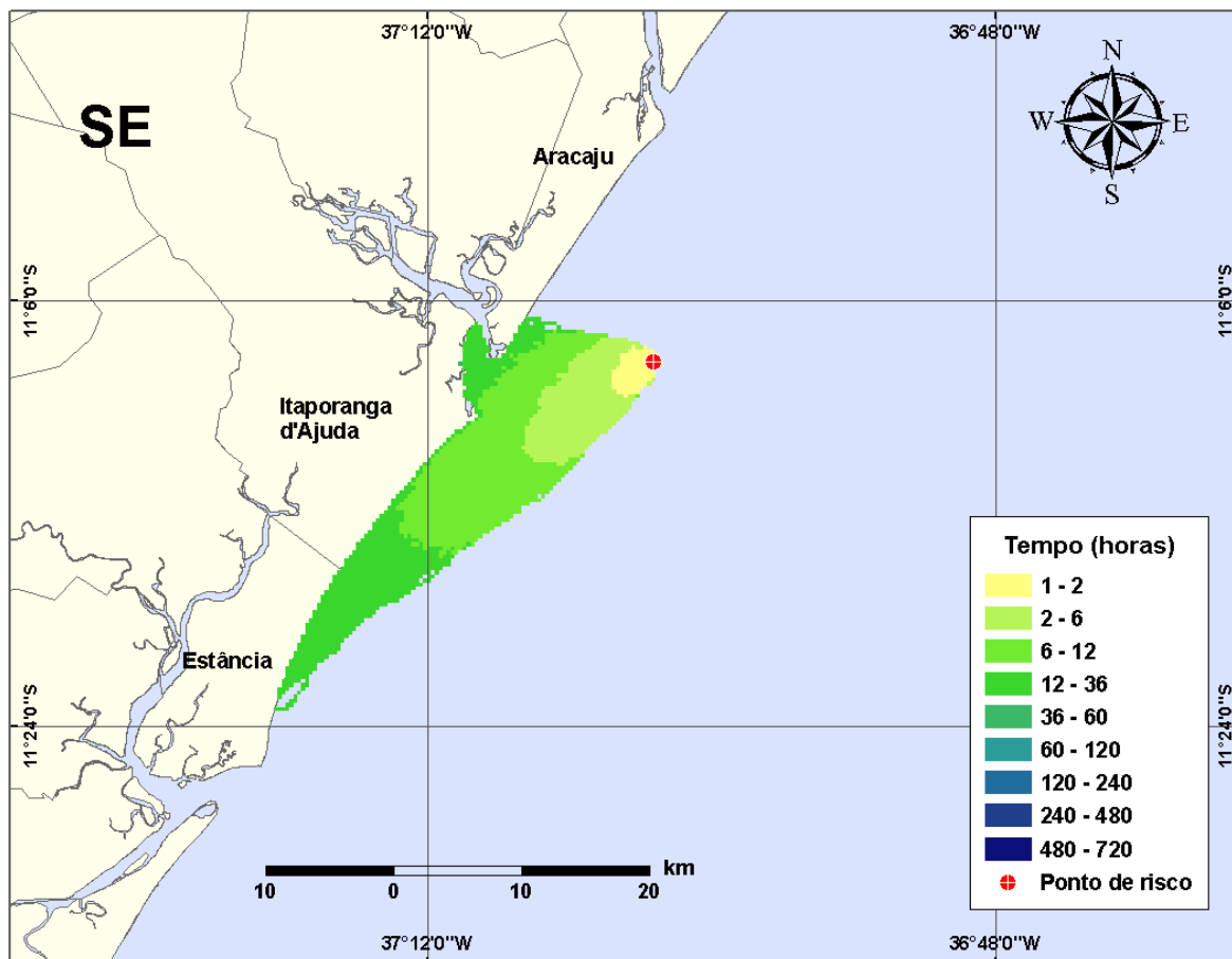
Figura III-18 - Cenário PGA3_VER_200_30D. (Fase: instalação/produção). Contornos de deslocamento de óleo na água para um acidente com óleo tipo GUARICEMA, ocorrendo no Ponto-PGA3, do Campo Guaricema, durante os meses de verão (janeiro a março), com derrame de 200 m 3 (instantâneo), após 30 dias de simulação.
