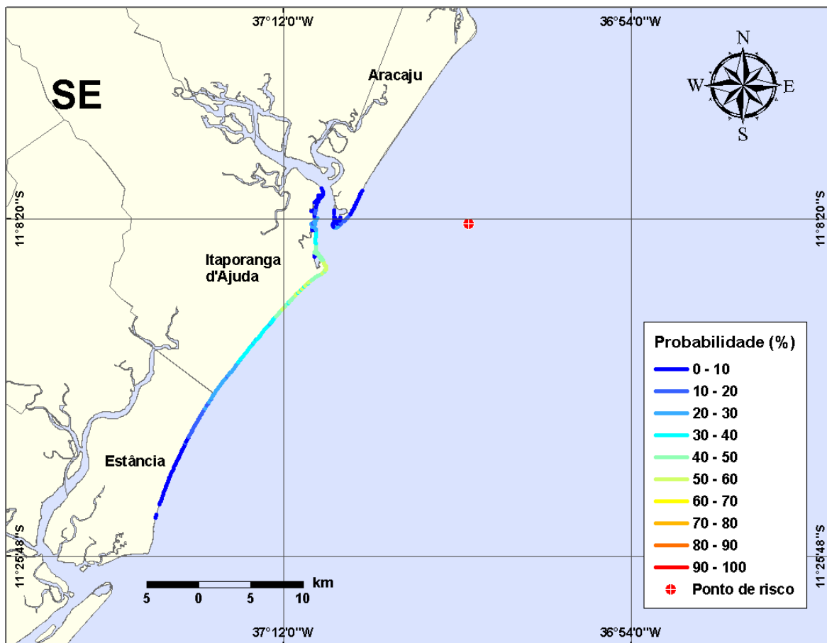
Figura III-15 - Cenário PGA3_VER_8_30D. (Fase: instalação/produção). Linhas de probabilidade de óleo na costa para um acidente com óleo tipo GUARICEMA, ocorrendo no Ponto-PGA3, do Campo Guaricema, durante os meses de verão (janeiro a março), com derrame de 8 m 3 (instantâneo), após 30 dias de simulação.
