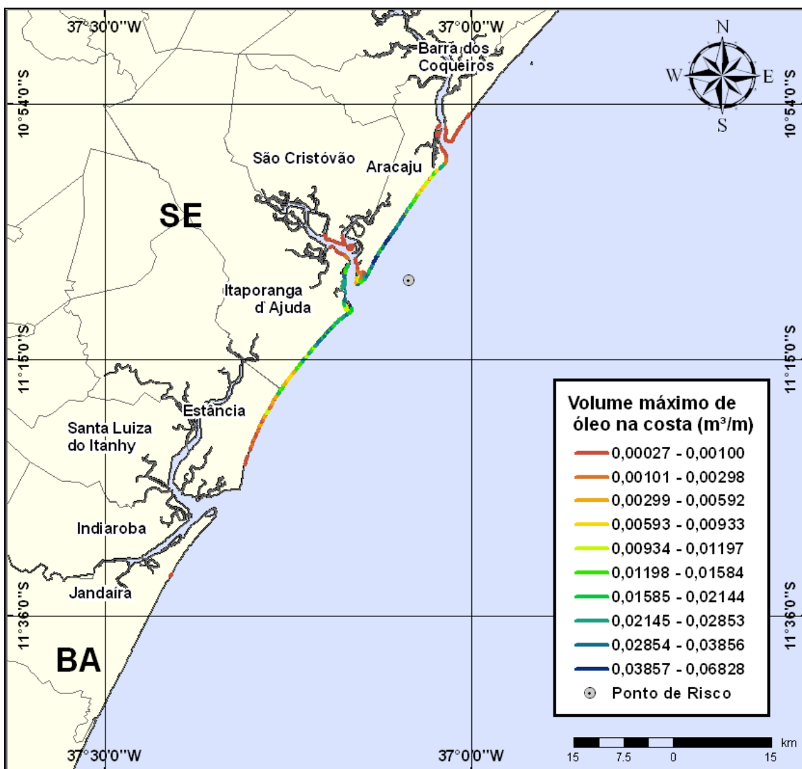
Figura III-104 - Cenário PE5_INV_200_30D (Fase: perfuração). Linhas de volume máximo de óleo na costa para um acidente com óleo tipo GUARICEMA ocorrendo no Ponto-PE5, durante os meses de inverno (junho a agosto), com derrame de 200 m 3 (instantâneo), após 30 dias de simulação.
