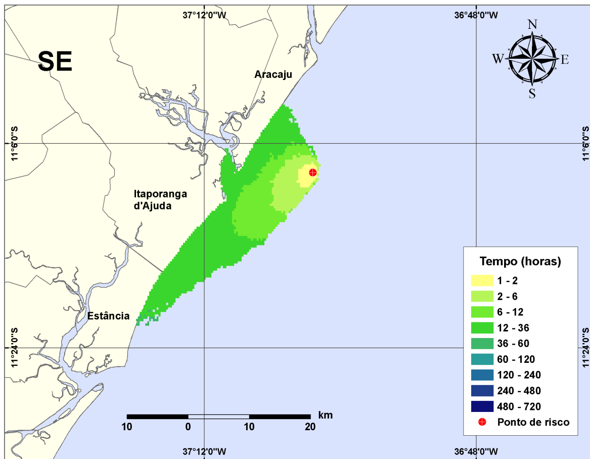
Figura III-74 - Cenário PGA3_INV_8_30D. (Fase: instalação/produção). Contornos de deslocamento de óleo na água para um acidente com óleo tipo GUARICEMA, ocorrendo no Ponto-PGA3, do Campo Guaricema, durante os meses de inverno (junho a agosto), com derrame de 8 m 3 (instantâneo), após 30 dias de simulação.
