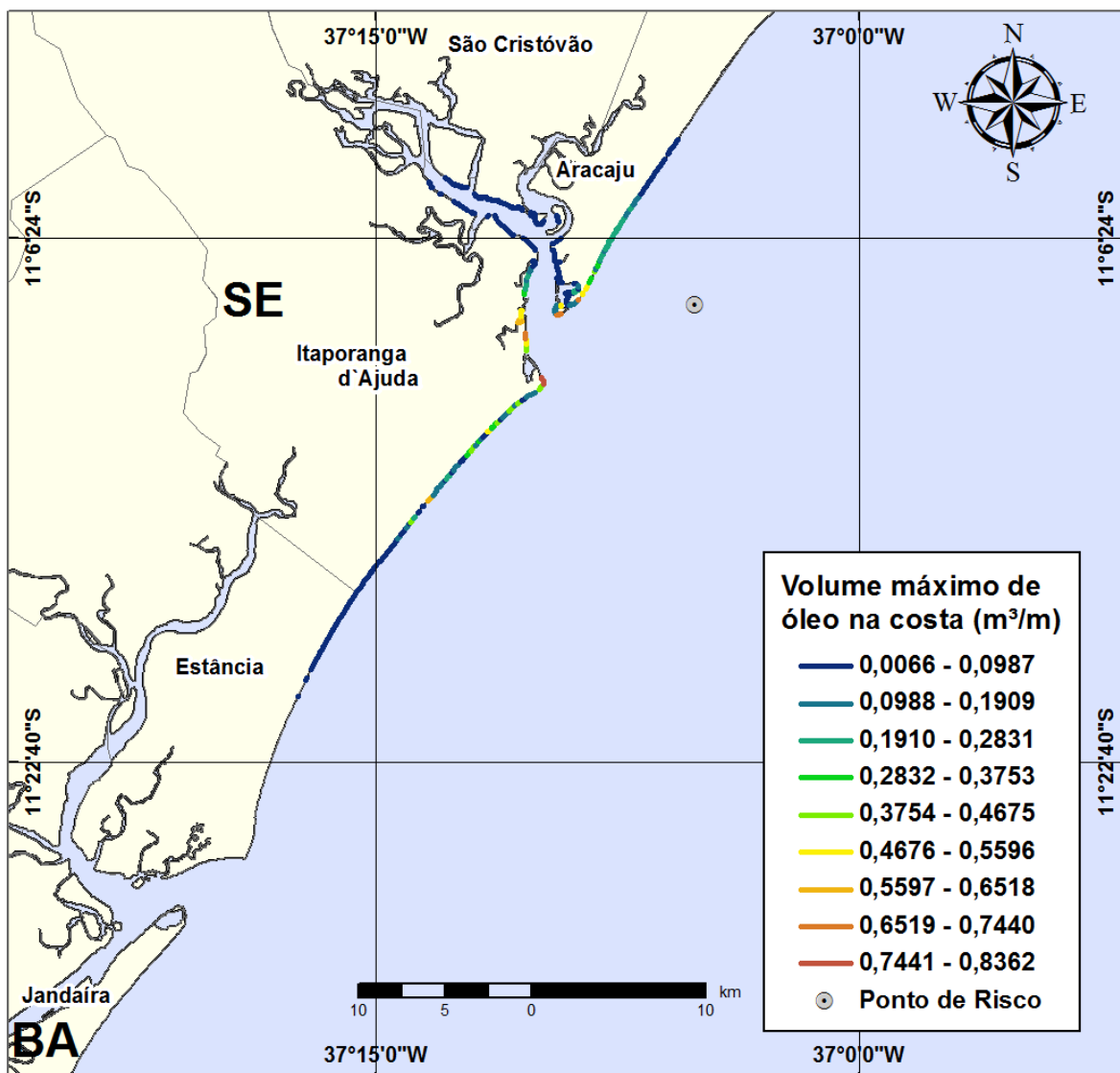
Figura III-48 - Cenário PE5_VER_7500_30D (Fase: perfuração). Linhas de volume máximo de óleo na costa para um acidente com óleo tipo GUARICEMA ocorrendo no Ponto-PE5, durante os meses de verão (janeiro a março), com derrame de 7.500 m 3 (ao longo de 30 dias), após 60 dias de simulação.
