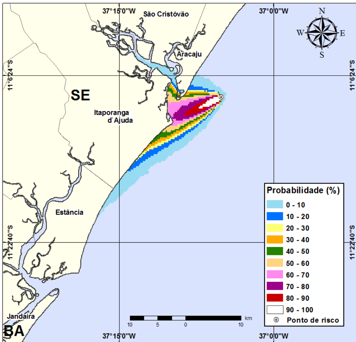
Figura III-41 - Cenário PE5_VER_200_30D (Fase: perfuração). Contornos de probabilidade de óleo na água para um acidente com óleo tipo GUARICEMA ocorrendo no Ponto-PE5, durante os meses de verão (janeiro a março), com derrame de 200 m 3 (instantâneo), após 30 dias de simulação.
