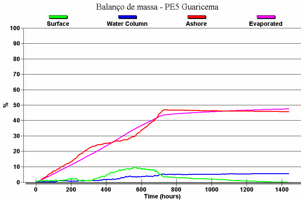
Figura III-124 - Balanço de massa do cenário DET_PE5_PC_VER_7500_60D.
