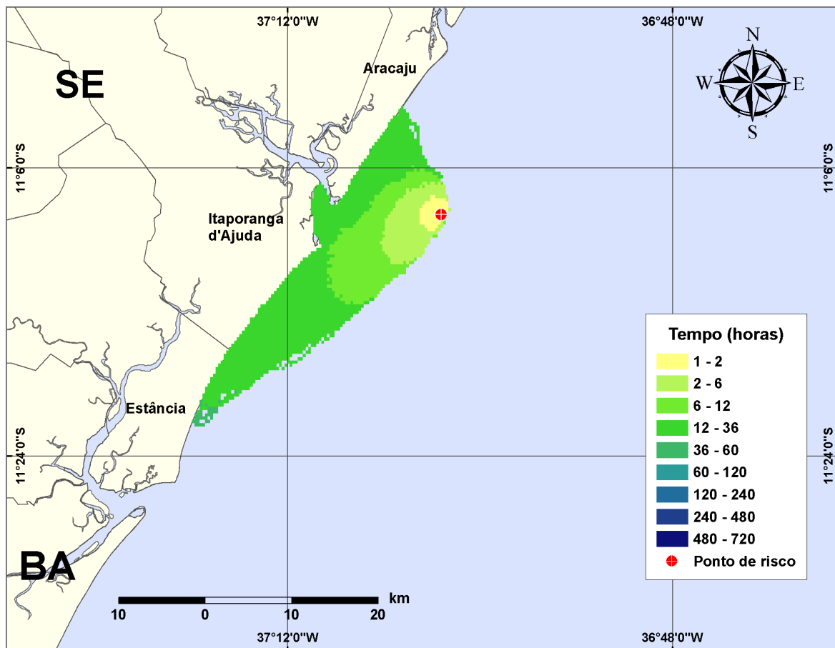
Figura III-66 - Cenário PGA3_DIESEL_INV_200_30D. (Fase: instalação/perfuração). Contornos de deslocamento de óleo na água para um acidente com óleo tipo DIESEL, ocorrendo no Ponto-PGA3, do Campo Guaricema, durante os meses de inverno (junho a agosto), com derrame de 200 m 3 (instantâneo), após 30 dias de simulação.
