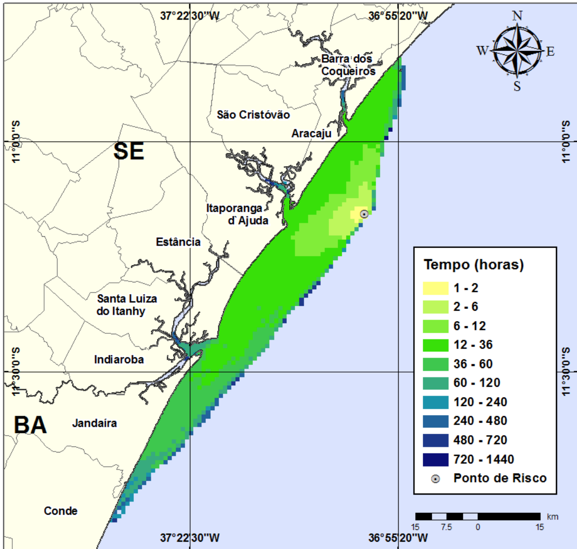
Figura III-118 - Cenário GA64_INV_7500_60D. (Fase: produção). Contornos de deslocamento de óleo na água para um acidente com óleo tipo GUARICEMA, ocorrendo no Ponto-GA64, do Campo Guaricema, durante os meses de inverno (junho a agosto), com derrame de 7.500 m 3 (ao longo de 30 dias), após 60 dias de simulação.
