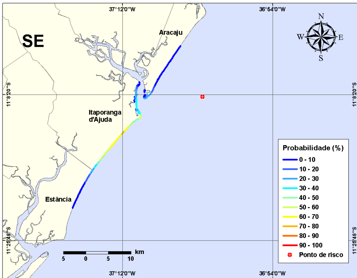
Figura III-79 - Cenário PGA3_INV_200_30D. (Fase: instalação/produção). Linhas de probabilidade de óleo na costa para um acidente com óleo tipo GUARICEMA, ocorrendo no Ponto-PGA3, do Campo Guaricema, durante os meses de inverno (junho a agosto), com derrame de 200 m 3 (instantâneo), após 30 dias de simulação.
