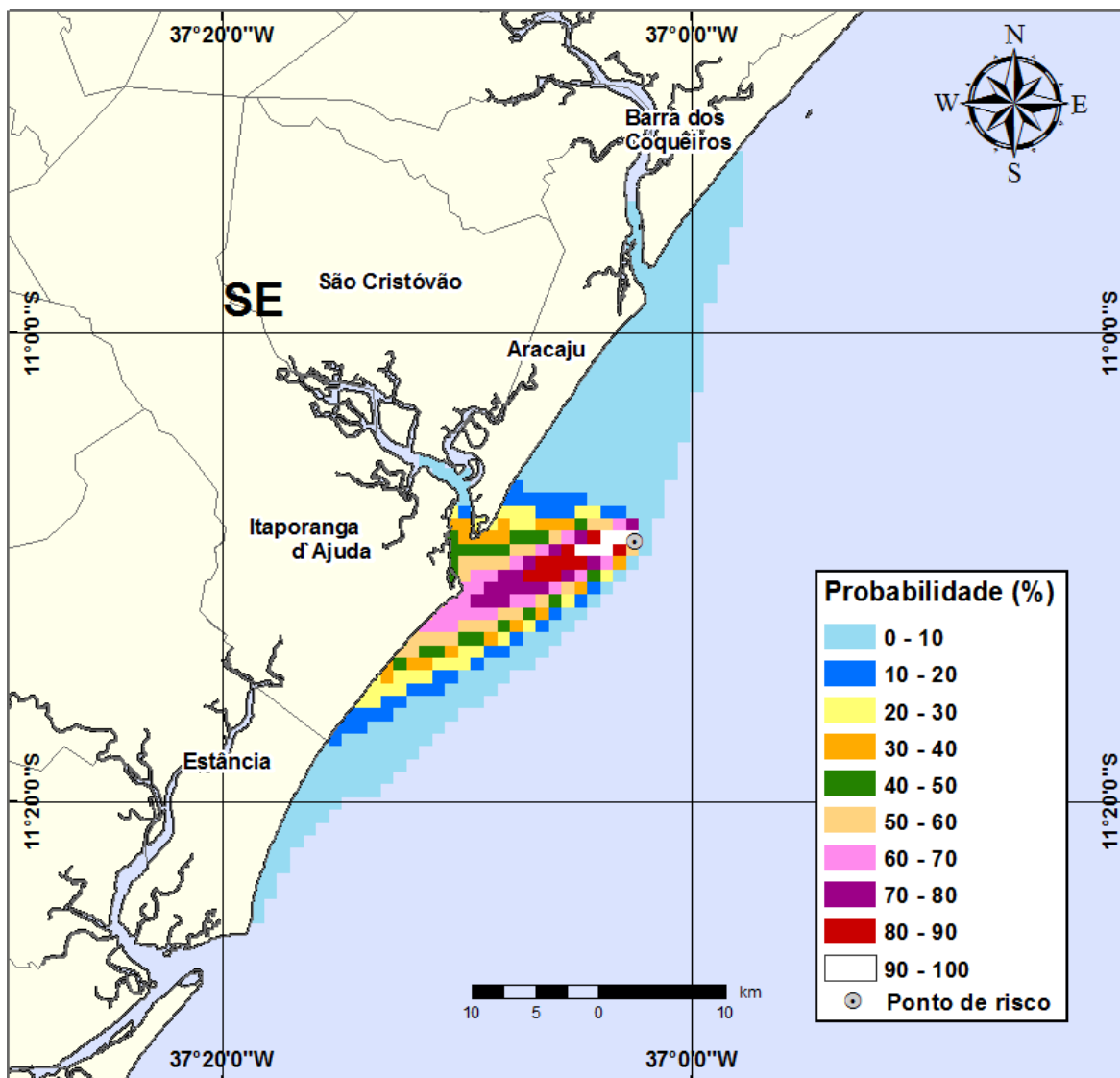
Figura III-81 - Cenário PGA3_INV_264_30D. (Fase: produção). Contornos de probabilidade de óleo na água para um acidente com óleo tipo GUARICEMA, ocorrendo no Ponto-PGA3, do Campo Guaricema, durante os meses de inverno (junho a agosto), com derrame de 264 m 3 (instantâneo), após 30 dias de simulação.
