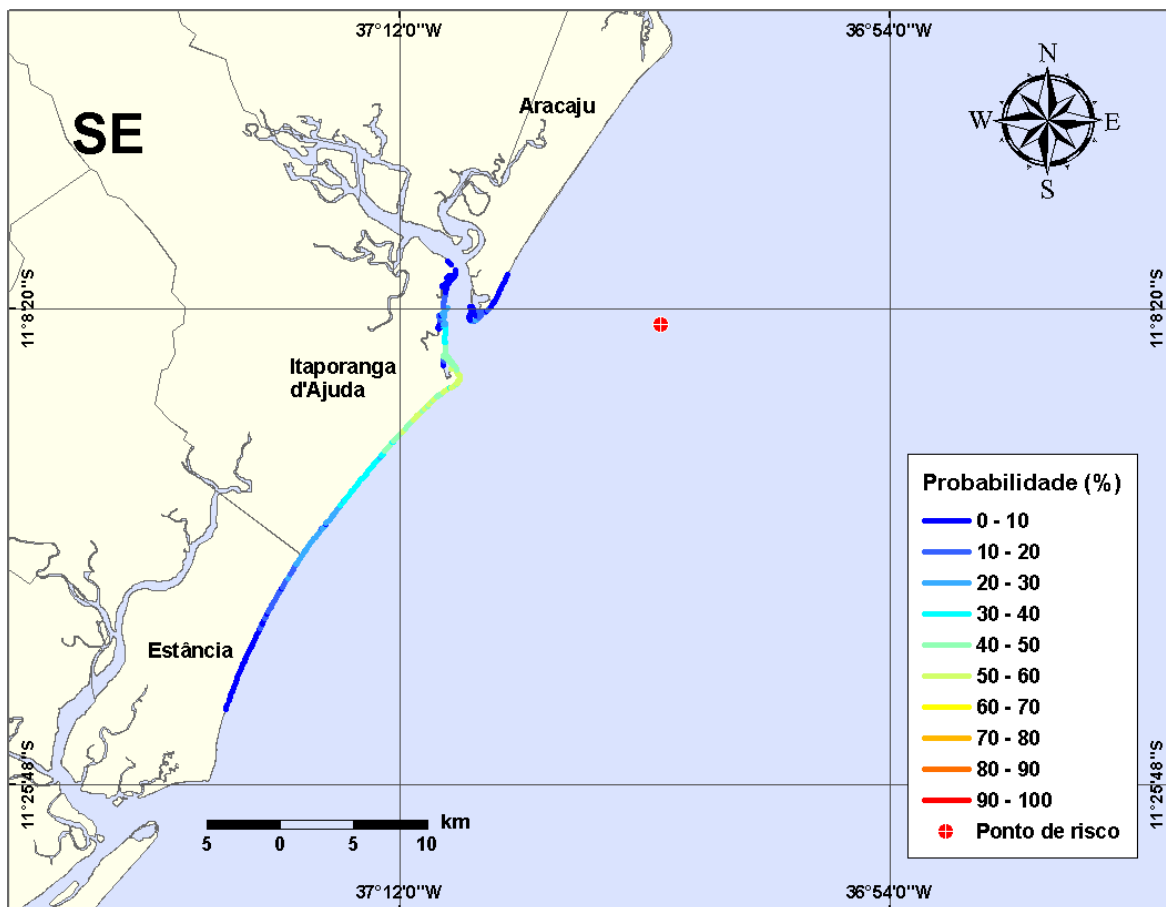
Figura III-7 - Cenário PGA3_DIESEL_VER_200_30D. (Fase: instalação/perfuração). Linhas de probabilidade de óleo na costa para um acidente com óleo tipo DIESEL, ocorrendo no Ponto-PGA3, do Campo Guaricema, durante os meses de verão (janeiro a março), com derrame de 200 m 3 (instantâneo), após 30 dias de simulação.
