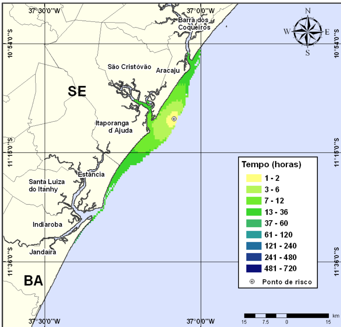
Figura III-102 - Cenário PE5_INV_200_30D (Fase: perfuração). Contornos de deslocamento de óleo na água para um acidente com óleo tipo GUARICEMA ocorrendo no Ponto-PE5, durante os meses de inverno (junho a agosto), com derrame de 200 m 3 (instantâneo), após 30 dias de simulação.
