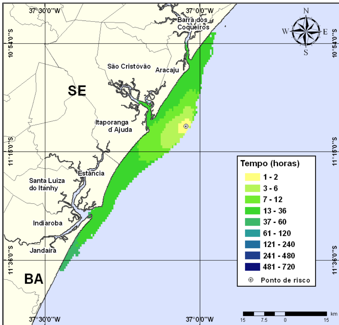
Figura III-90 - Cenário PGA10_INV_200_30D (Fase: Fase:instalação/produção/perfuração). Contornos de deslocamento de óleo na água para um acidente com óleo tipo GUARICEMA ocorrendo no Ponto-PGA10, durante os meses de inverno (junho a agosto), com derrame de 200 m 3 (instantâneo), após 30 dias de simulação.
