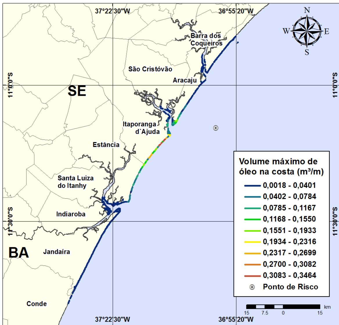
Figura III-120 - Cenário GA64_INV_7500_60D. (Fase: produção). Linhas de volume máximo de óleo na costa para um acidente com óleo tipo GUARICEMA, ocorrendo no Ponto-GA64, do Campo Guaricema, durante os meses de inverno (junho a agosto), com derrame 7.500 m 3 (ao longo de 30 dias), após 60 dias de simulação.
