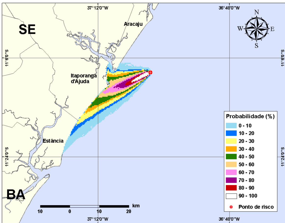
Figura III-13 - Cenário PGA3_VER_8_30D. (Fase: instalação/produção). Contornos de probabilidade de óleo na água para um acidente com óleo tipo GUARICEMA, ocorrendo no Ponto-PGA3, do Campo Guaricema, durante os meses de verão (janeiro a março), com derrame de 8 m 3 (instantâneo), após 30 dias de simulação.
