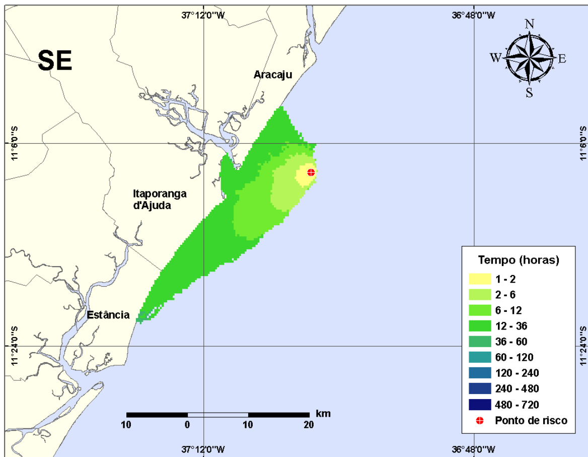
Figura III-78 - Cenário PGA3_INV_200_30D. (Fase: instalação/produção). Contornos de deslocamento de óleo na água para um acidente com óleo tipo GUARICEMA, ocorrendo no Ponto-PGA3, do Campo Guaricema, durante os meses de inverno (junho a agosto), com derrame de 200 m 3 (instantâneo), após 30 dias de simulação.
