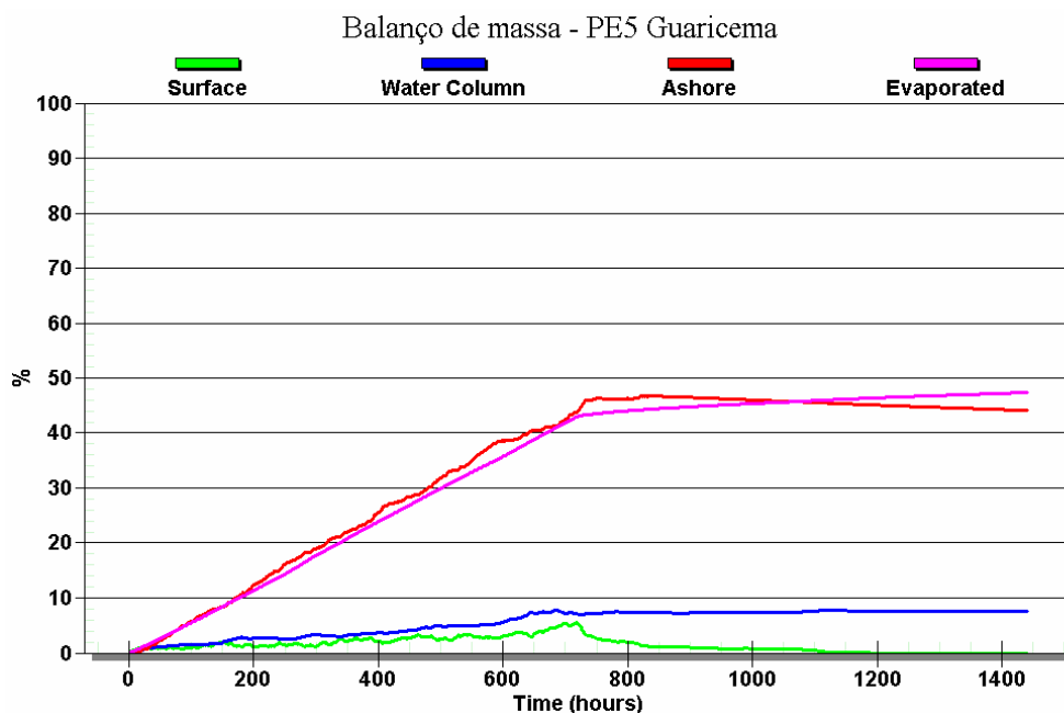
Figura III-131 - Balanço de massa do cenário DET_PE5_INV_7500_60D.
