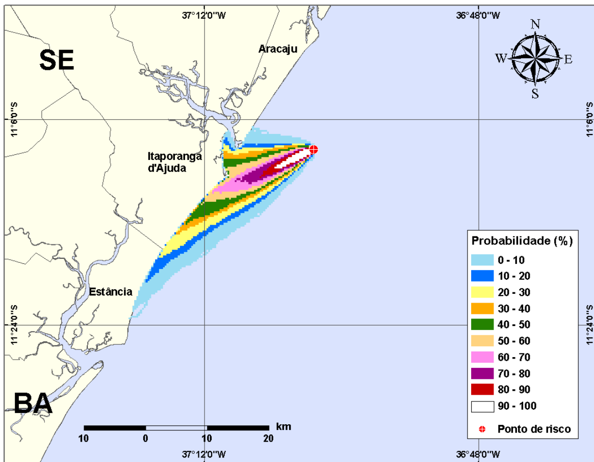
Figura III-17 - Cenário PGA3_VER_200_30D. (Fase: instalação/produção). Contornos de probabilidade de óleo na água para um acidente com óleo tipo GUARICEMA, ocorrendo no Ponto-PGA3, do Campo Guaricema, durante os meses de verão (janeiro a março), com derrame de 200 m 3 (instantâneo), após 30 dias de simulação.
