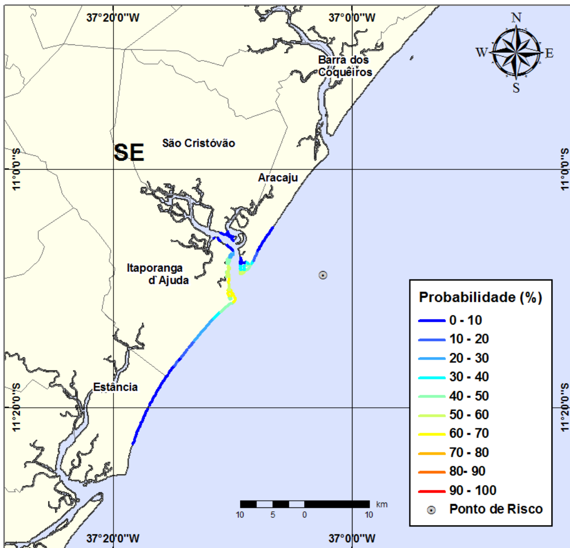
Figura III-23 - Cenário PGA3_VER_264_30D. (Fase: produção). Linhas de probabilidade de óleo na costa para um acidente com óleo tipo GUARICEMA, ocorrendo no Ponto-PGA3, do Campo Guaricema, durante os meses de verão (janeiro a março), com derrame de 264 m 3 (instantâneo), após 30 dias de simulação.
