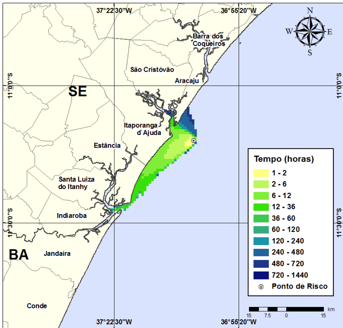
Figura III-54 - Cenário GA58_VER_7500_60D. (Fase: produção). Contornos de deslocamento de óleo na água para um acidente com óleo tipo GUARICEMA, ocorrendo no Ponto-GA58, do Campo Guaricema, durante os meses de verão (janeiro a março), com derrame de 7.500 m 3 (ao longo de 30 dias), após 60 dias de simulação.
