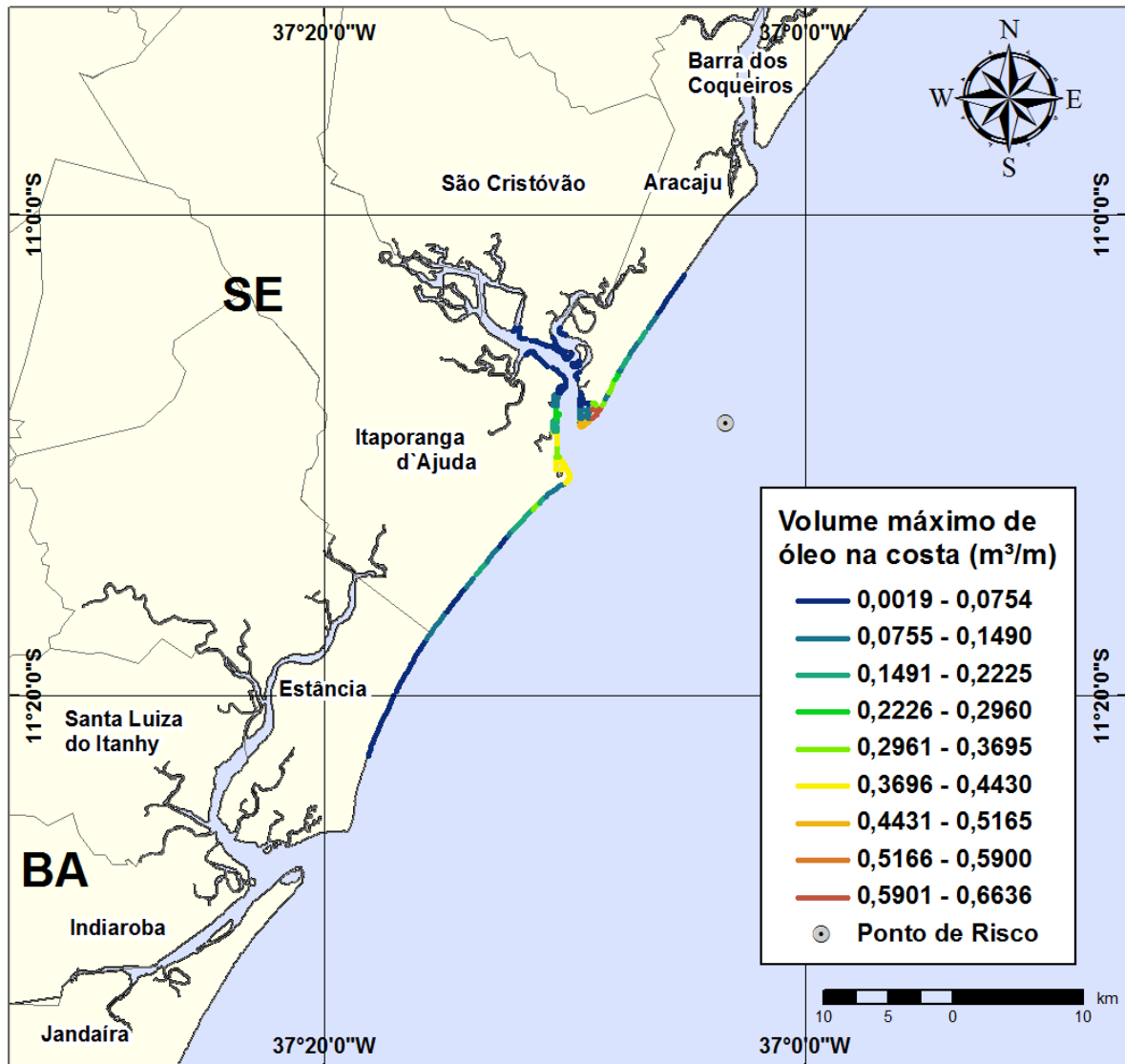
Figura III-52 - Cenário GA07_VER_7500_60D. (Fase: produção). Linhas de volume máximo de óleo na costa para um acidente com óleo tipo GUARICEMA, ocorrendo no Ponto-GA07, do Campo Guaricema, durante os meses de verão (janeiro a março), com derrame de 7.500 m 3 (ao longo de 30 dias), após 60 dias de simulação.
