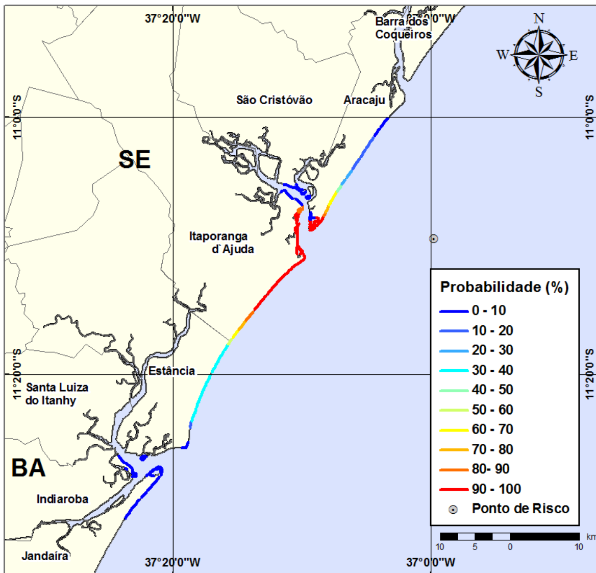
Figura III-59 - Cenário GA64_VER_7500_60D. (Fase: produção). Linhas de probabilidade de óleo na costa para um acidente com óleo tipo GUARICEMA, ocorrendo no Ponto-GA64, do Campo Guaricema, durante os meses de verão (janeiro a março), com derrame de 7.500 m 3 (ao longo de 30 dias), após 60 dias de simulação.
