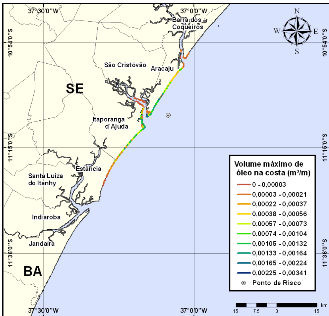
Figura III-100 - Cenário PE5_INV_8_30D (Fase: perfuração). Linhas de volume máximo de óleo na costa para um acidente com óleo tipo GUARICEMA ocorrendo no Ponto-PE5, durante os meses de inverno (junho a agosto), com derrame de 8 m 3 (instantâneo), após 30 dias de simulação.
