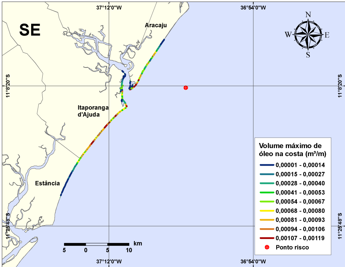
Figura III-76 - Cenário PGA3_INV_8_30D. (Fase: instalação/produção). Linhas de volume máximo de óleo na costa para um acidente com óleo tipo GUARICEMA, ocorrendo no Ponto-PGA3, do Campo Guaricema, durante os meses de inverno (junho a agosto), com derrame de 8 m 3 (instantâneo), após 30 dias de simulação.
