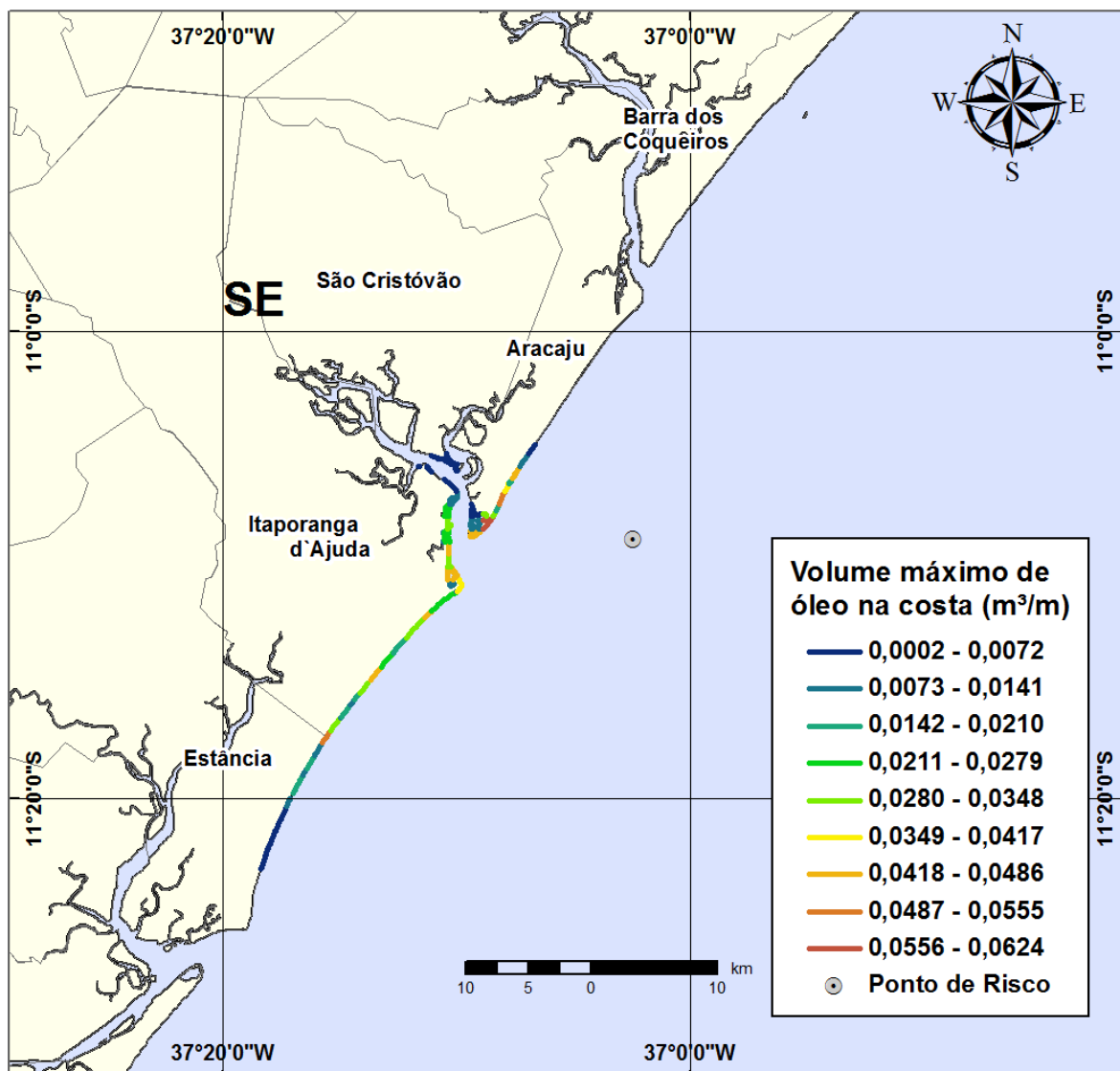
Figura III-24 - Cenário PGA3_VER_264_30D. (Fase: produção). Linhas de volume máximo de óleo na costa para um acidente com óleo tipo GUARICEMA, ocorrendo no Ponto-PGA3, do Campo Guaricema, durante os meses de verão (janeiro a março), com derrame de 264 m 3 (instantâneo), após 30 dias de simulação.
