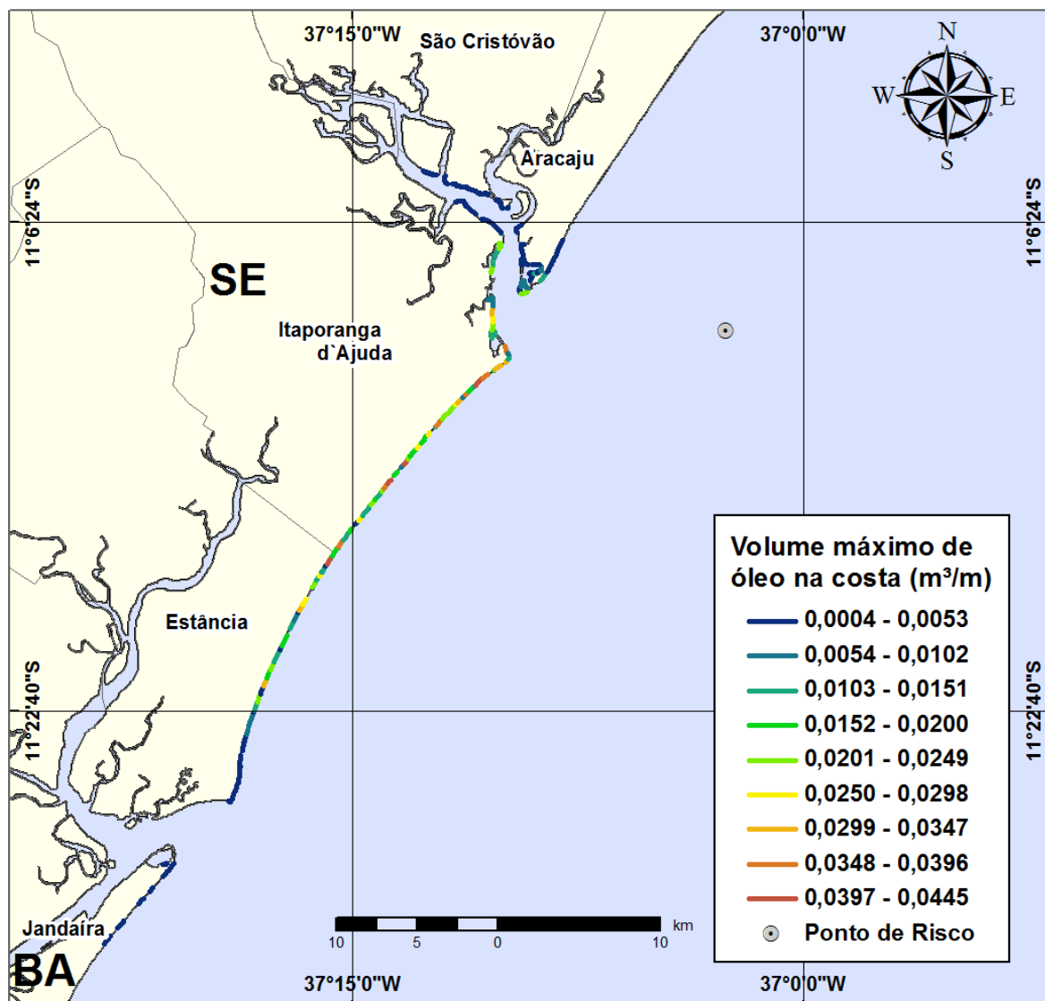
Figura III-32 - Cenário PGA10_VER_200_30D. (Fase:instalação/produção/ perfuração). Linhas de volume máximo de óleo na costa para um acidente com óleo tipo GUARICEMA ocorrendo no Ponto-PGA10, durante os meses de verão (janeiro a março), com derrame de 200 m 3 (instantâneo), após 30 dias de simulação.
