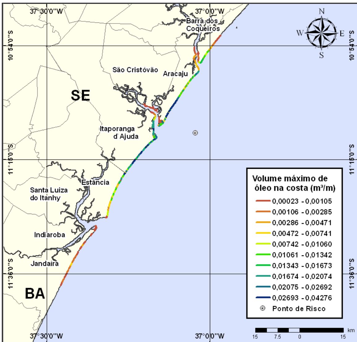
Figura III-92 - Cenário PGA10_INV_200_30D (Fase:instalação/produção/perfuração). Linhas de volume máximo de óleo na costa para um acidente com óleo tipo GUARICEMA ocorrendo no Ponto-PGA10, durante os meses de inverno (junho a agosto), com derrame de 200 m 3 (instantâneo), após 30 dias de simulação.
