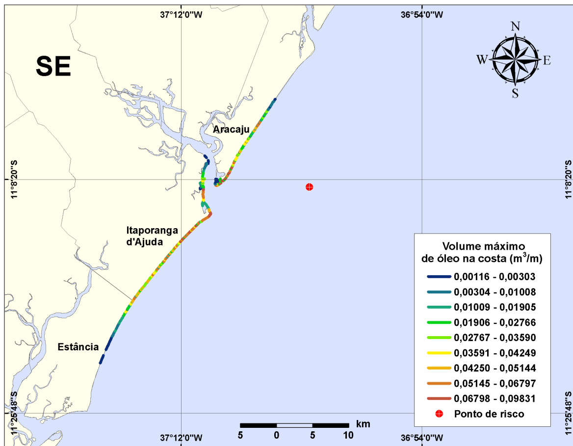
Figura III-72 - Cenário PGA3_DIESEL_INV_PC_30D. (Fase: instalação/produção). Linhas de volume máximo de óleo na costa para um acidente com óleo tipo DIESEL, ocorrendo no Ponto-PGA3, do Campo Guaricema, durante os meses de inverno (junho a agosto), com derrame de 500 m^3 (instantâneo), após 30 dias de simulação.
