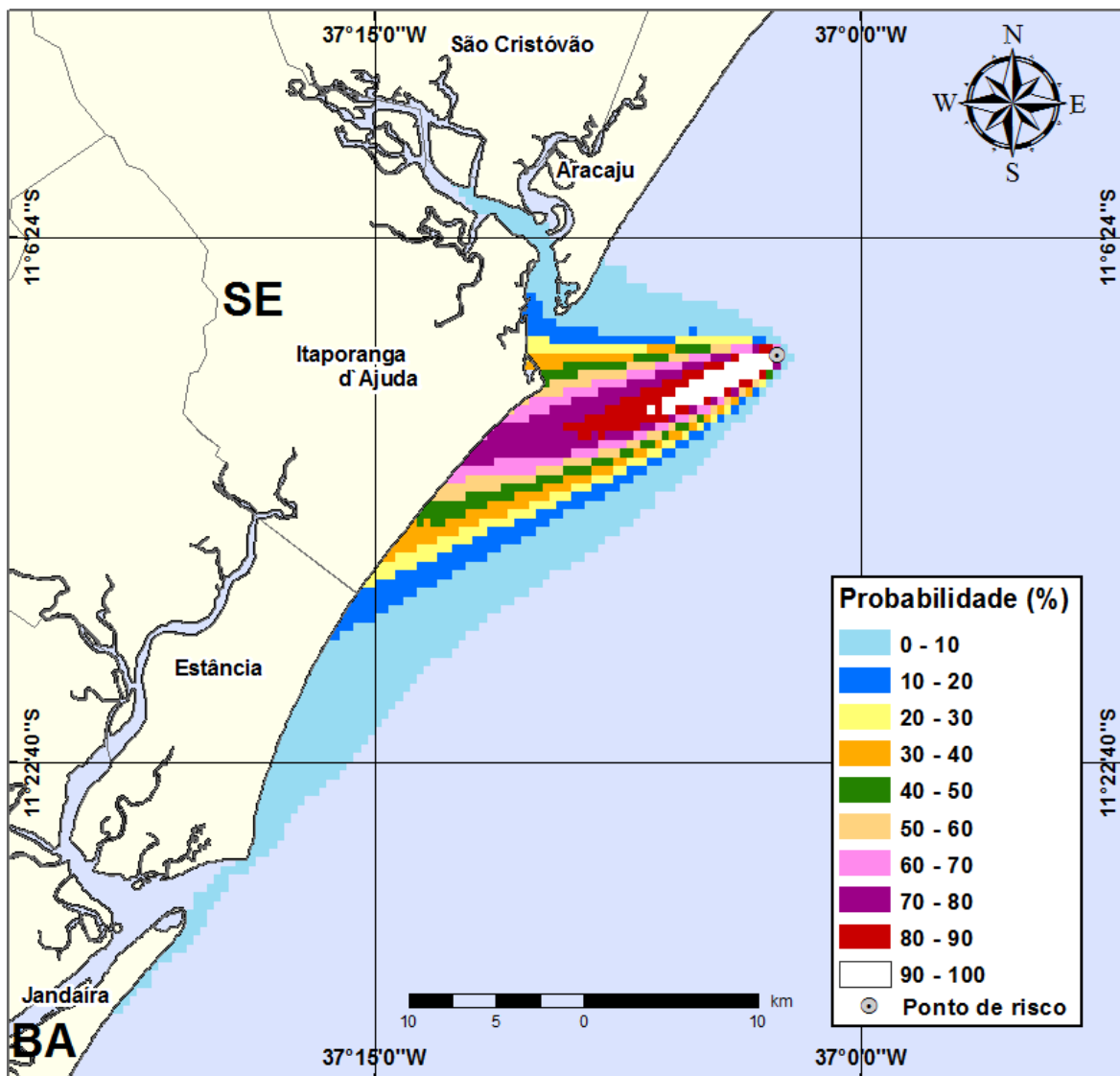
Figura III-29 - Cenário PGA10_VER_200_30D. (Fase:instalação/produção/ perfuração). Contornos de probabilidade de óleo na água para um acidente com óleo tipo GUARICEMA ocorrendo no Ponto-PGA10, durante os meses de verão (janeiro a março), com derrame de 200 m 3 (instantâneo), após 30 dias de simulação.
