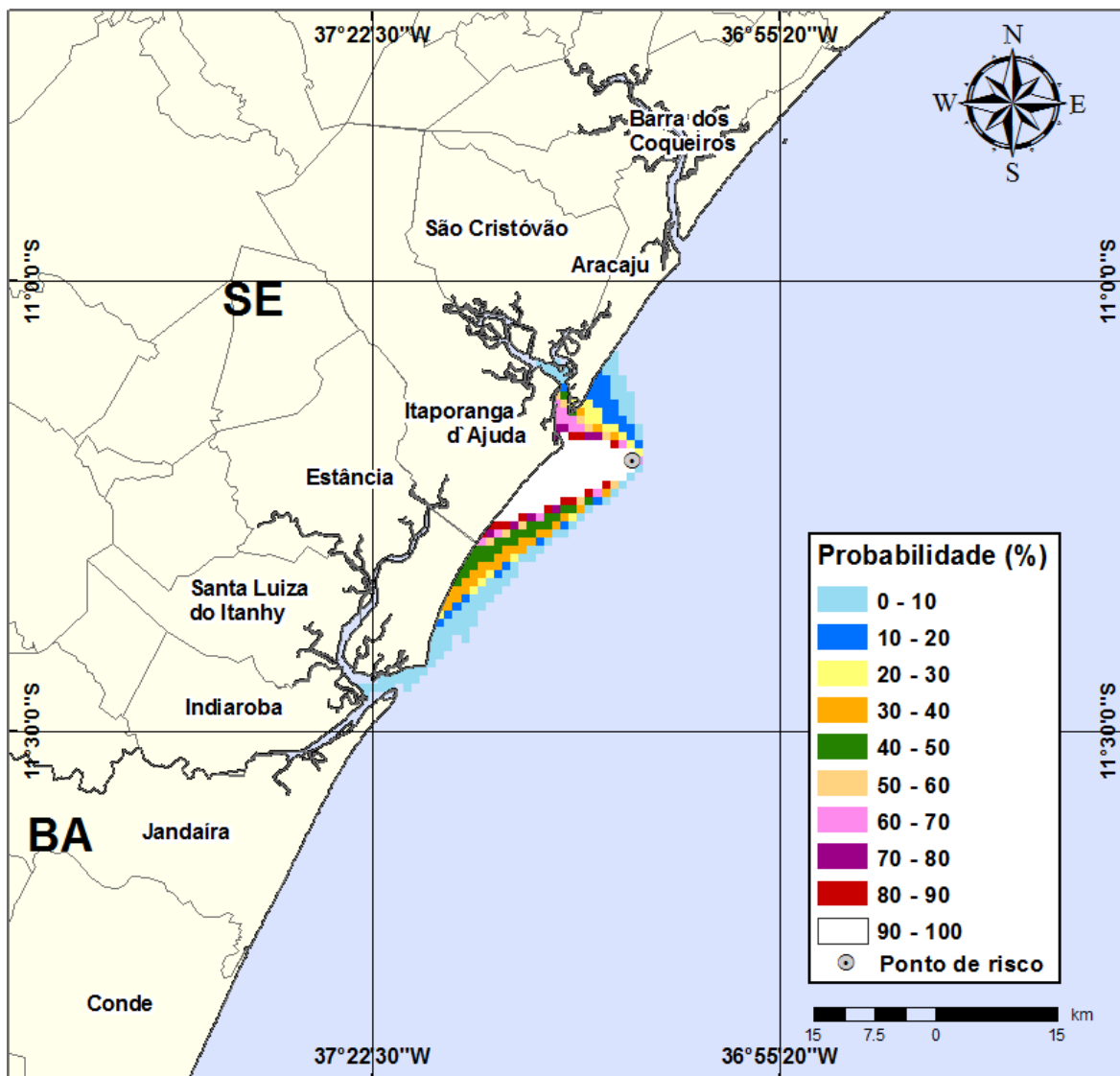
Figura III-53 - Cenário GA58_VER_7500_60D. (Fase: produção). Contornos de probabilidade de óleo na água para um acidente com óleo tipo GUARICEMA, ocorrendo no Ponto-GA58, do Campo Guaricema, durante os meses de verão (janeiro a março), com derrame de 7.500 m 3 (ao longo de 30 dias), após 60 dias de simulação.
