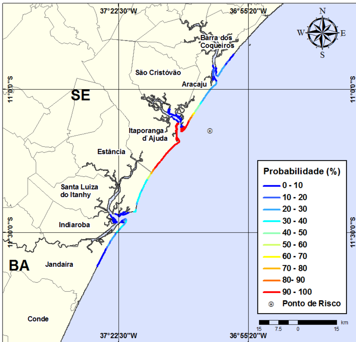
Figura III-111 - Cenário GA07_INV_7500_60D. (Fase: produção). Linhas de probabilidade de óleo na costa para um acidente com óleo tipo GUARICEMA, ocorrendo no Ponto-GA07, do Campo Guaricema, durante os meses de inverno (junho a agosto), com derrame de 7.500 m 3 (ao longo de 30 dias), após 60 dias de simulação.
