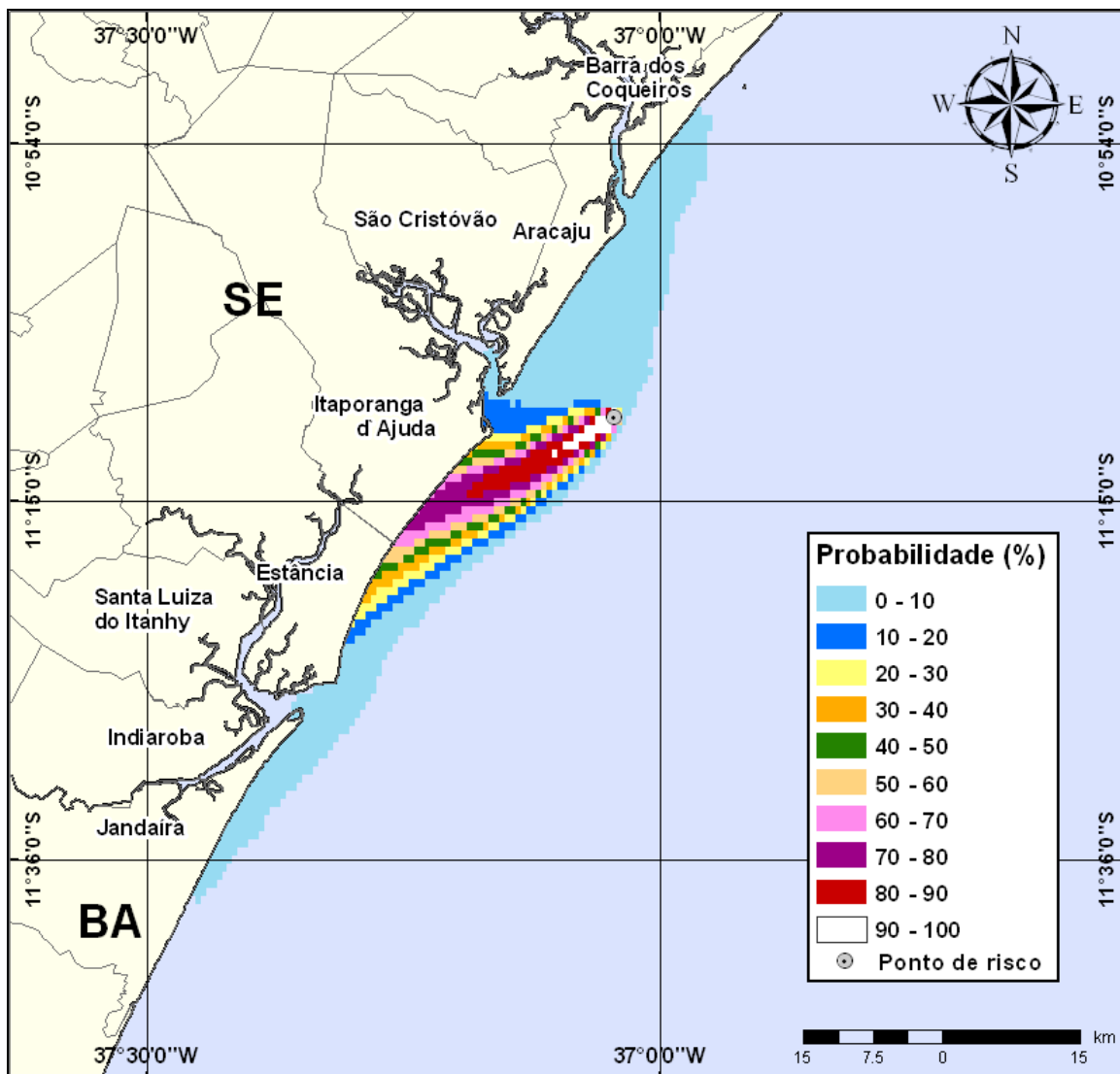
Figura III-85 - Cenário PGA10_INV_8_30D (Fase:instalação/produção/perfuração). Contornos de probabilidade de óleo na água para um acidente com óleo tipo GUARICEMA ocorrendo no Ponto-PGA10, durante os meses de inverno (junho a agosto), com derrame de 8 m 3 (instantâneo), após 30 dias de simulação.
