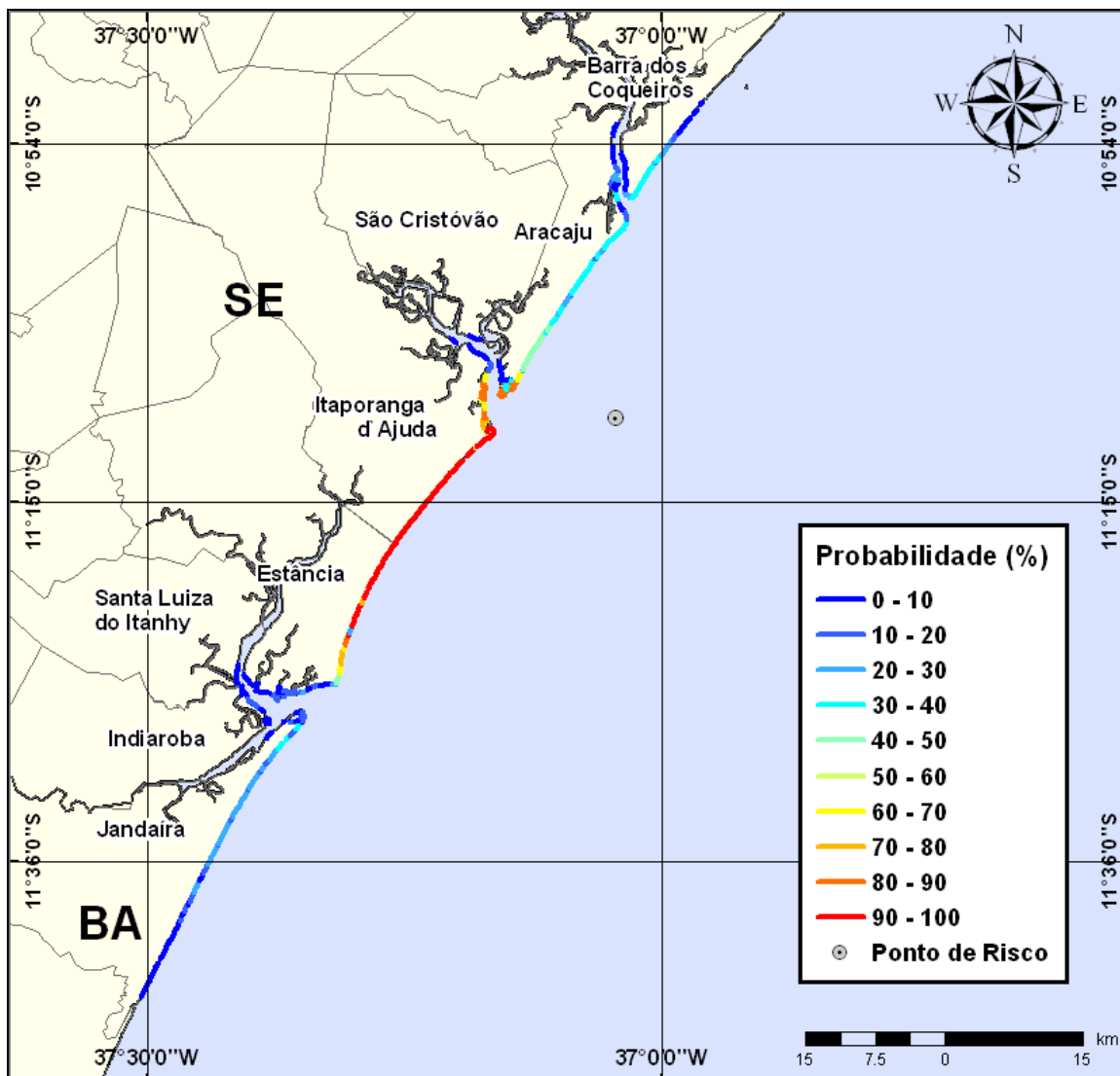
Figura III-95 - Cenário PGA10_INV_7500_60D (Fase: perfuração). Linhas de probabilidade de óleo na costa para um acidente com óleo tipo GUARICEMA ocorrendo no Ponto-PGA10, durante os meses de inverno (junho a agosto), com derrame de 7.500 m 3 (ao longo de 30 dias), após 60 dias de simulação.
