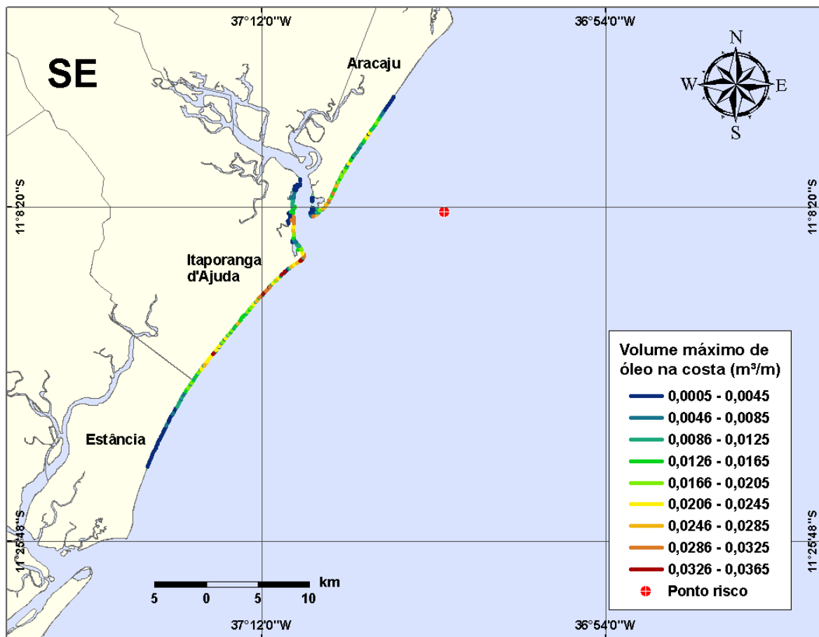
Figura III-80 - Cenário PGA3_INV_200_30D. (Fase: instalação/produção). Linhas de volume máximo de óleo na costa para um acidente com óleo tipo GUARICEMA, ocorrendo no Ponto-PGA3, do Campo Guaricema, durante os meses de inverno (junho a agosto), com derrame de 200 m 3 (instantâneo), após 30 dias de simulação.
