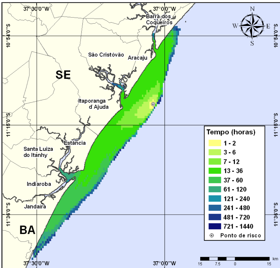
Figura III-94 - Cenário PGA10_INV_7500_60D (Fase: perfuração). Contornos de deslocamento de óleo na água para um acidente com óleo tipo GUARICEMA ocorrendo no Ponto-PGA10, durante os meses de inverno (junho a agosto), com derrame de 7.500 m 3 (ao longo de 30 dias), após 60 dias de simulação.
