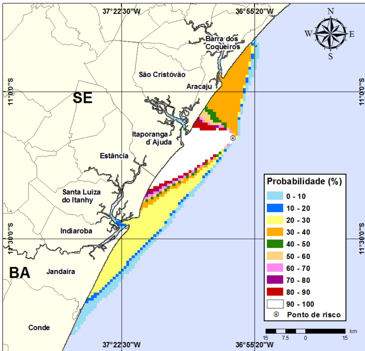
Figura III-117 - Cenário GA64_INV_7500_60D. (Fase: produção). Contornos de probabilidade de óleo na água para um acidente com óleo tipo GUARICEMA, ocorrendo no Ponto-GA64, do Campo Guaricema, durante os meses de inverno (junho a agosto), com derrame de 7.500 m 3 (ao longo de 30 dias), após 60 dias de simulação.
