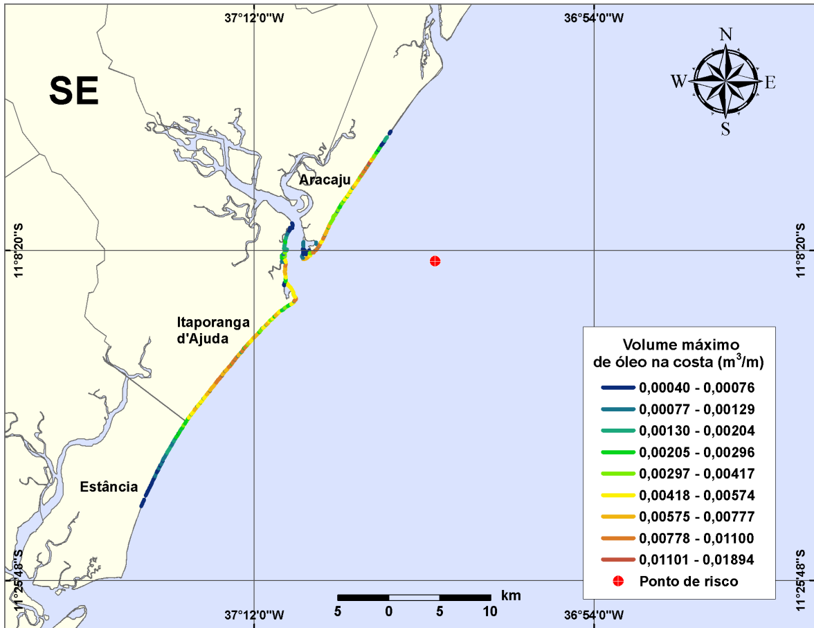
Figura III-68- Cenário PGA3_DIESEL_INV_200_30D. (Fase: instalação/perfuração). Linhas de volume máximo de óleo na costa para um acidente com óleo tipo DIESEL, ocorrendo no Ponto-PGA3, do Campo Guaricema, durante os meses de inverno (junho a agosto), com derrame de 200 m 3 (instantâneo), após 30 dias de simulação.
