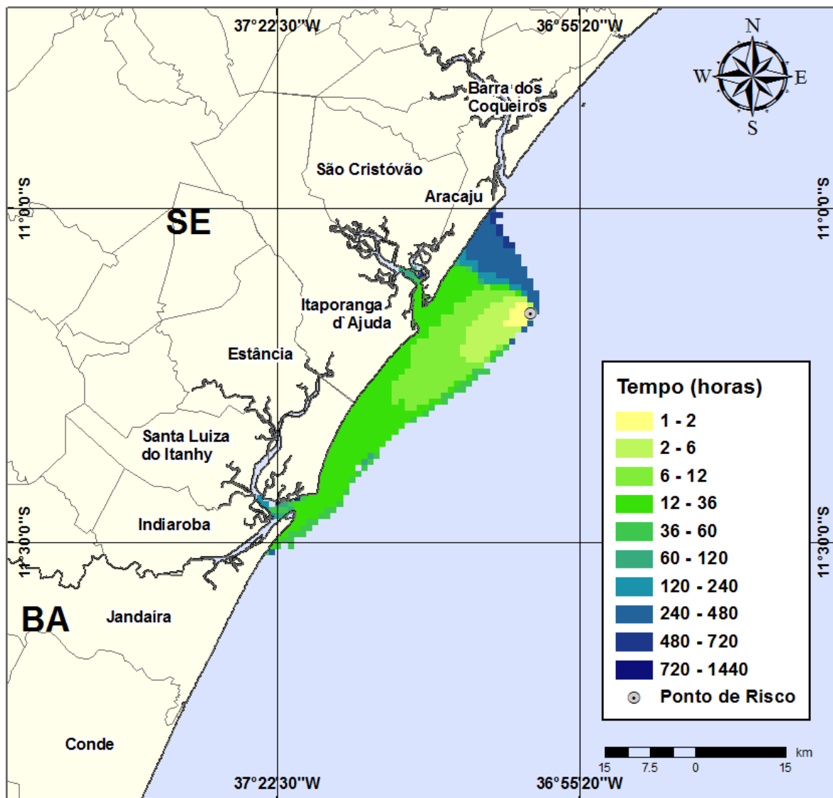
Figura III-58 - Cenário GA64_VER_7500_60D. (Fase: produção). Contornos de deslocamento de óleo na água para um acidente com óleo tipo GUARICEMA, ocorrendo no Ponto-GA64, do Campo Guaricema, durante os meses de verão (janeiro a março), com derrame de 7.500 m 3 (ao longo de 30 dias), após 60 dias de simulação.
