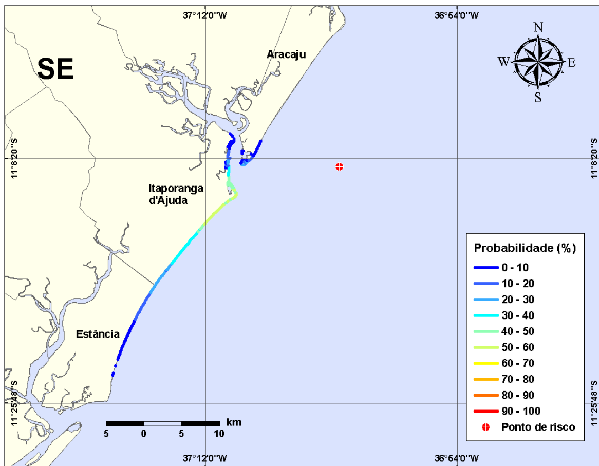
Figura III-11 - Cenário PGA3_DIESEL_VER_500_30D. (Fase: instalação/perfuração). Linhas de probabilidade de óleo na costa para um acidente com óleo tipo DIESEL, ocorrendo no Ponto-PGA3, do Campo Guaricema, durante os meses de verão (janeiro a março), com derrame de 500 m 3 (instantâneo), após 30 dias de simulação.
