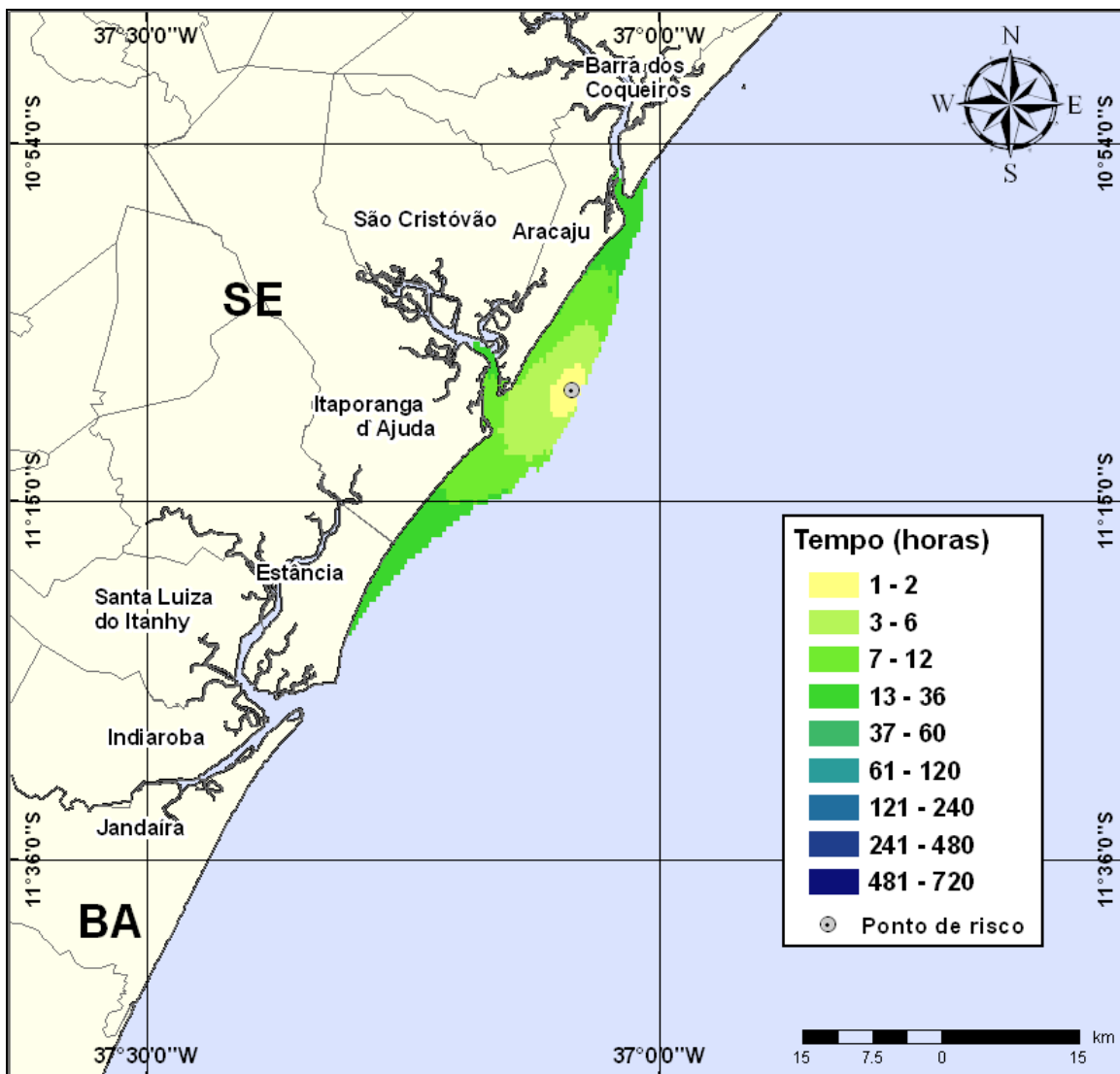
Figura III-98 - Cenário PE5_INV_8_30D (Fase: perfuração). Contornos de deslocamento de óleo na água para um acidente com óleo tipo GUARICEMA ocorrendo no Ponto-PE5, durante os meses de inverno (junho a agosto), com derrame de 8 m 3 (instantâneo), após 30 dias de simulação.
