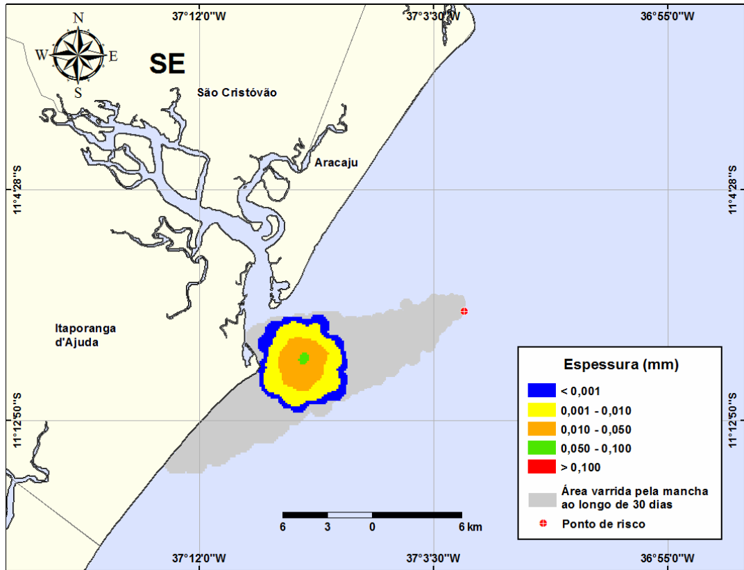
Figura III-128 - DET_PGA3_DIESEL_INV_500_30D. Cenário determinístico crítico para um derrame ocorrido durante o inverno com óleo DIESEL, a partir do Ponto-PGA3 no Campo Guaricema.
