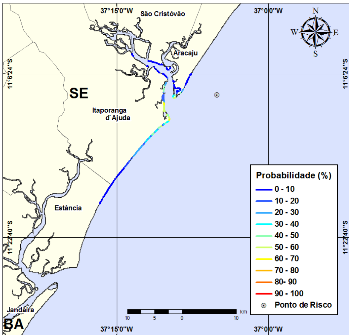
Figura III-43 - Cenário PE5_VER_200_30D (Fase: perfuração). Linhas de probabilidade de óleo na costa para um acidente com óleo tipo GUARICEMA ocorrendo no Ponto-PE5, durante os meses de verão (janeiro a março), com derrame de 200 m 3 (instantâneo), após 30 dias de simulação.
