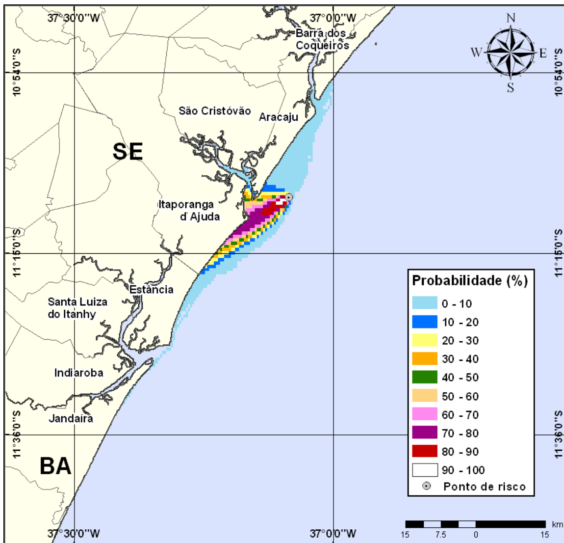
Figura III-101 - Cenário PE5_INV_200_30D (Fase: perfuração). Contornos de probabilidade de óleo na água para um acidente com óleo tipo GUARICEMA ocorrendo no Ponto-PE5, durante os meses de inverno (junho a agosto), com derrame de 200 m 3 (instantâneo), após 30 dias de simulação.
