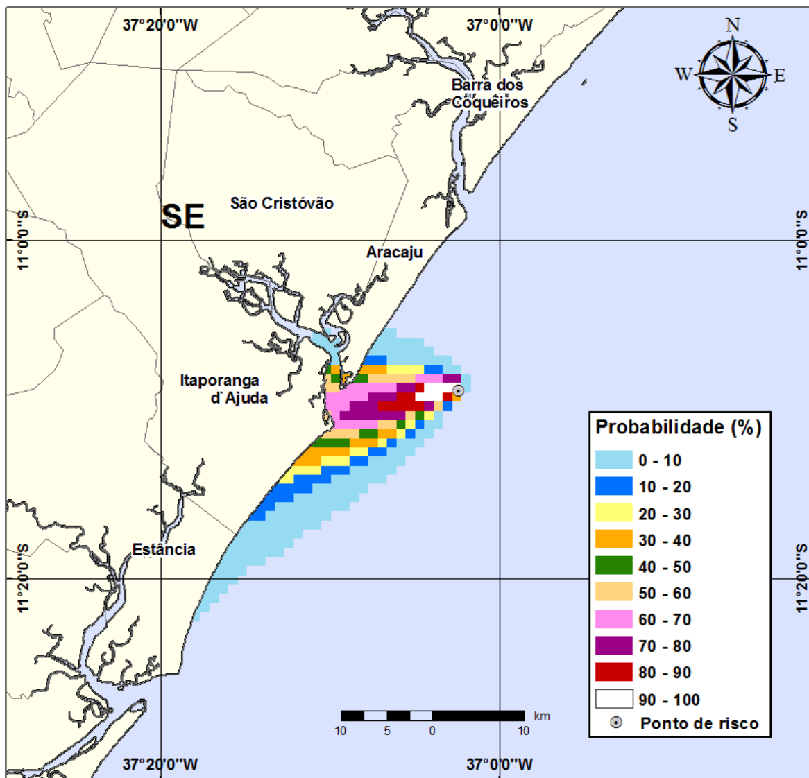
Figura III-21 - Cenário PGA3_VER_264_30D. (Fase: produção). Contornos de probabilidade de óleo na água para um acidente com óleo tipo GUARICEMA, ocorrendo no Ponto-PGA3, do Campo Guaricema, durante os meses de verão (janeiro a março), com derrame de 264 m 3 (instantâneo), após 30 dias de simulação.
