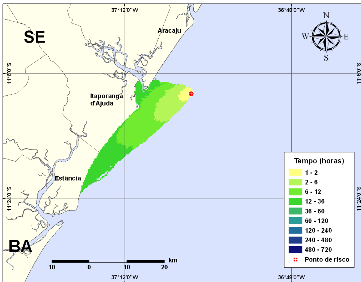
Figura III-2 - Cenário PGA3_DIESEL_VER_8_30D. (Fase: instalação/perfuração). Contornos de deslocamento de óleo na água para um acidente com óleo tipo DIESEL, ocorrendo no Ponto-PGA3, do Campo Guaricema, durante os meses de verão (janeiro a março), com derrame de 8 m 3 (instantâneo), após 30 dias de simulação.
