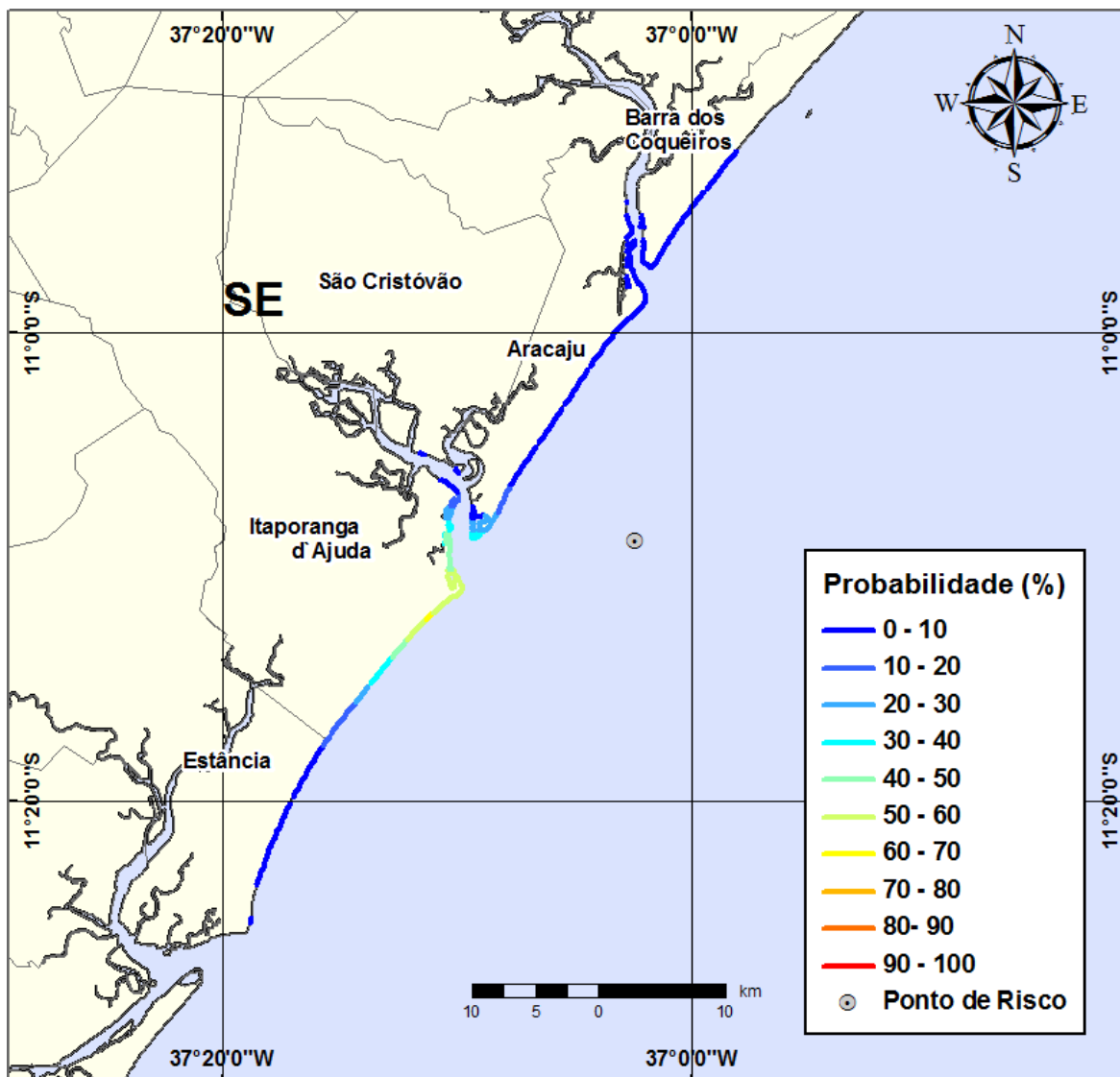
Figura III-83 - Cenário PGA3_INV_264_30D. (Fase: produção). Linhas de probabilidade de óleo na costa para um acidente com óleo tipo GUARICEMA, ocorrendo no Ponto-PGA3, do Campo Guaricema, durante os meses de inverno (junho a agosto), com derrame de 264 m 3 (instantâneo), após 30 dias de simulação.
