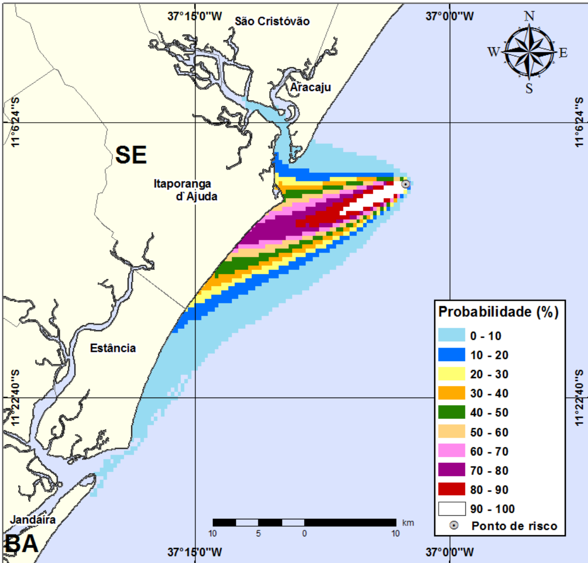
Figura III-25 - Cenário PGA10_VER_8_30D. (Fase: instalação/produção/perfuração) Contornos de probabilidade de óleo na água para um acidente ocorrendo no Ponto-PGA10, durante os meses de verão (janeiro a março), com derrame de 8 m 3 (instantâneo), após 30 dias de simulação.
