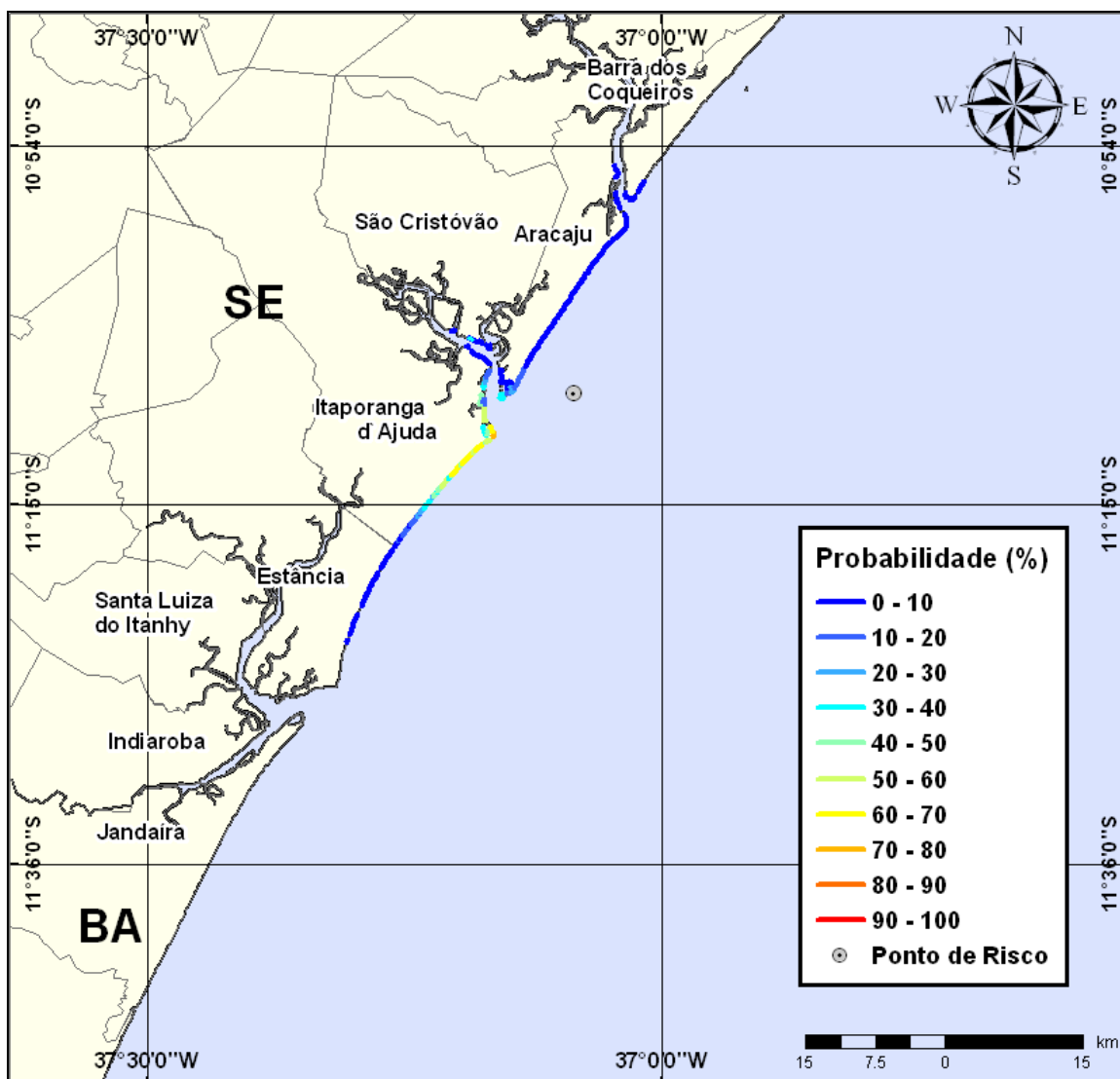
Figura III-99 - Cenário PE5_INV_8_30D (Fase: perfuração). Linhas de probabilidade de óleo na costa para um acidente com óleo tipo GUARICEMA ocorrendo no Ponto-PE5, durante os meses de inverno (junho a agosto), com derrame de 8 m 3 (instantâneo), após 30 dias de simulação.
