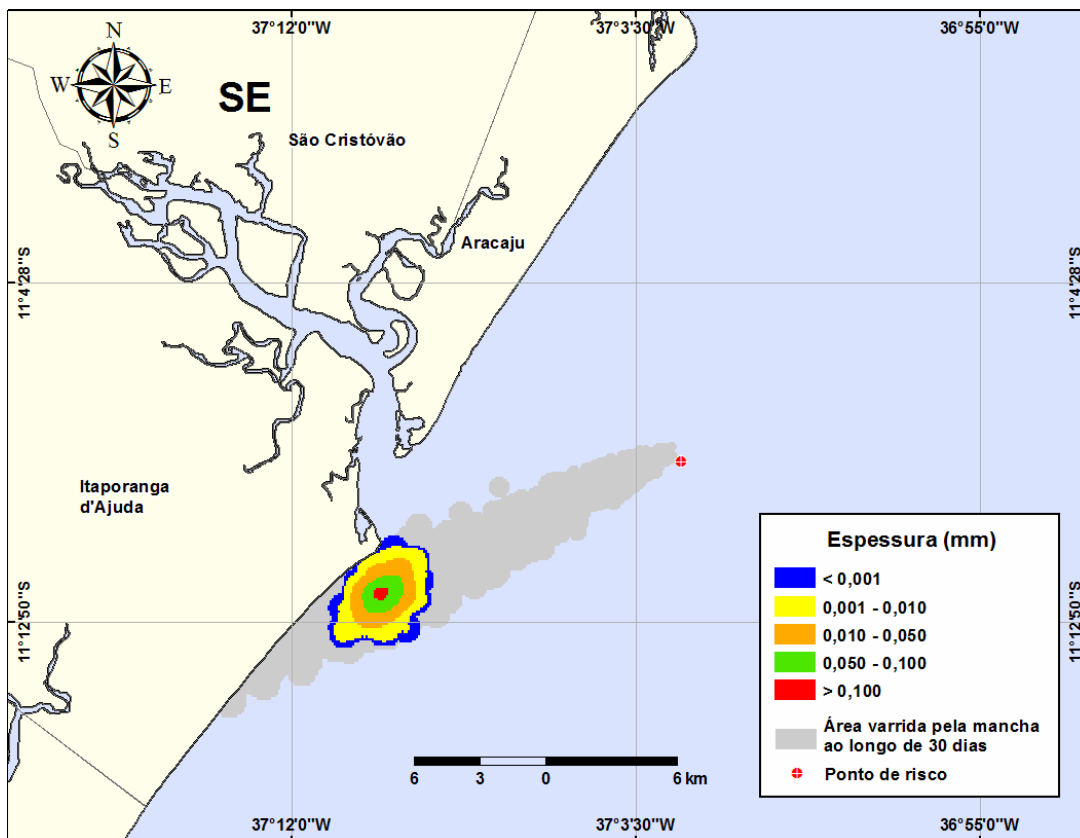
Figura III-121 - DET_PGA3_DIESEL_VER_500_30D. Cenário determinístico crítico para um derrame ocorrido durante o verão com óleo DIESEL, a partir do Ponto PGA3 no Campo Guaricema.
