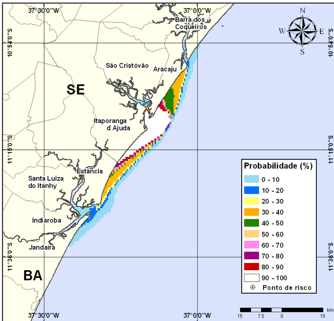
Figura III-105 - Cenário PE5_INV_7500_60D (Fase: perfuração). Contornos de probabilidade de óleo na água para um acidente com óleo tipo GUARICEMA ocorrendo no Ponto-PE5, durante os meses de inverno (junho a agosto), com derrame de 7.500 m 3 (ao longo de 30 dias), após 60 dias de simulação.
