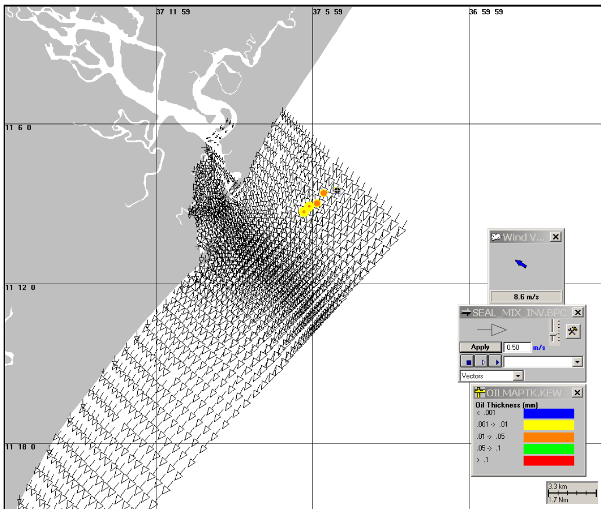
Figura III-133 - Cenário DET_PE5_INV_7500_60D . Condições meteorológicas e oceanográficas e espessuras da mancha de óleo 2 horas após o início da simulação.
