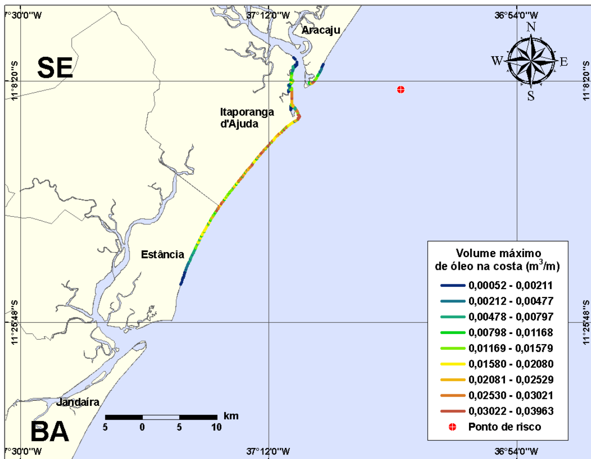
Figura III-8 - Cenário PGA3_DIESEL_VER_200_30D. (Fase: instalação/perfuração). Linhas de volume máximo de óleo na costa para um acidente com óleo tipo DIESEL, ocorrendo no Ponto-PGA3, do Campo Guaricema, durante os meses de verão (janeiro a março), com derrame de 200 m 3 (instantâneo), após 30 dias de simulação.
