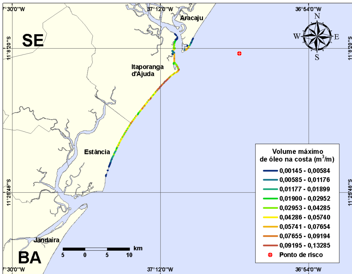
Figura III-12 - Cenário PGA3_DIESEL_VER_500_30D. (Fase: instalação/perfuração). Linhas de volume máximo de óleo na costa para um acidente com óleo tipo DIESEL, ocorrendo no Ponto-PGA3, do Campo Guaricema, durante os meses de verão (janeiro a março), com derrame de 500 m 3 (instantâneo), após 30 dias de simulação.
