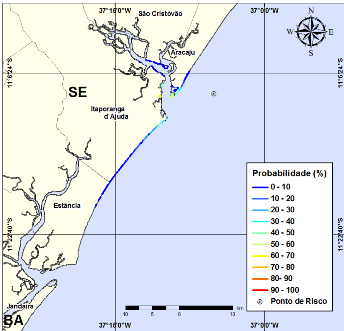
Figura III-39 - Cenário PE5_VER_8_30D (Fase: perfuração) Linhas de probabilidade de óleo na costa para um acidente com óleo tipo GUARICEMA ocorrendo no Ponto-PE5, durante os meses de verão (janeiro a março), com derrame de 8 m 3 (instantâneo), após 30 dias de simulação.
