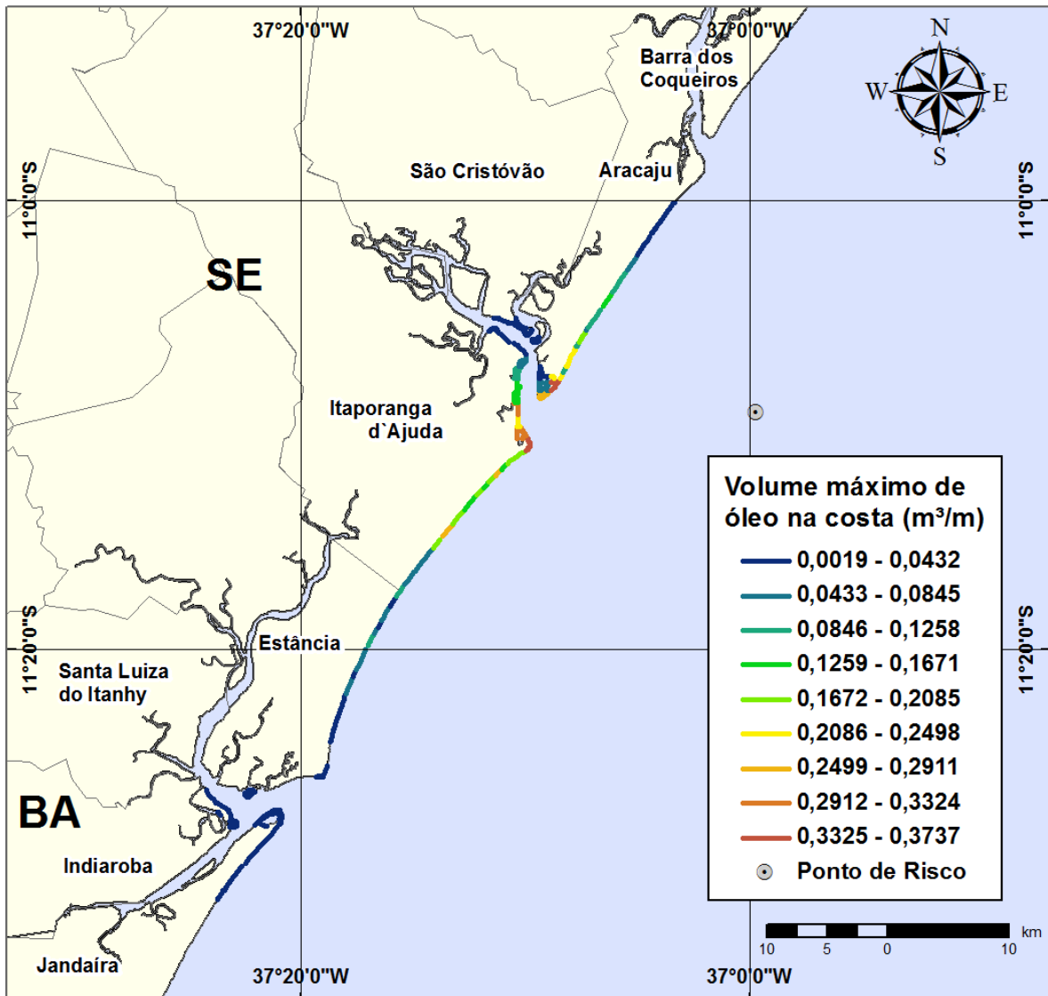
Figura III-60 - Cenário GA64_VER_7500_60D. (Fase: produção). Linhas de volume máximo de óleo na costa para um acidente com óleo tipo GUARICEMA, ocorrendo no Ponto-GA64, do Campo Guaricema, durante os meses de verão (janeiro a março), com derrame de 7.500 m 3 (ao longo de 30 dias), após 60 dias de simulação.
