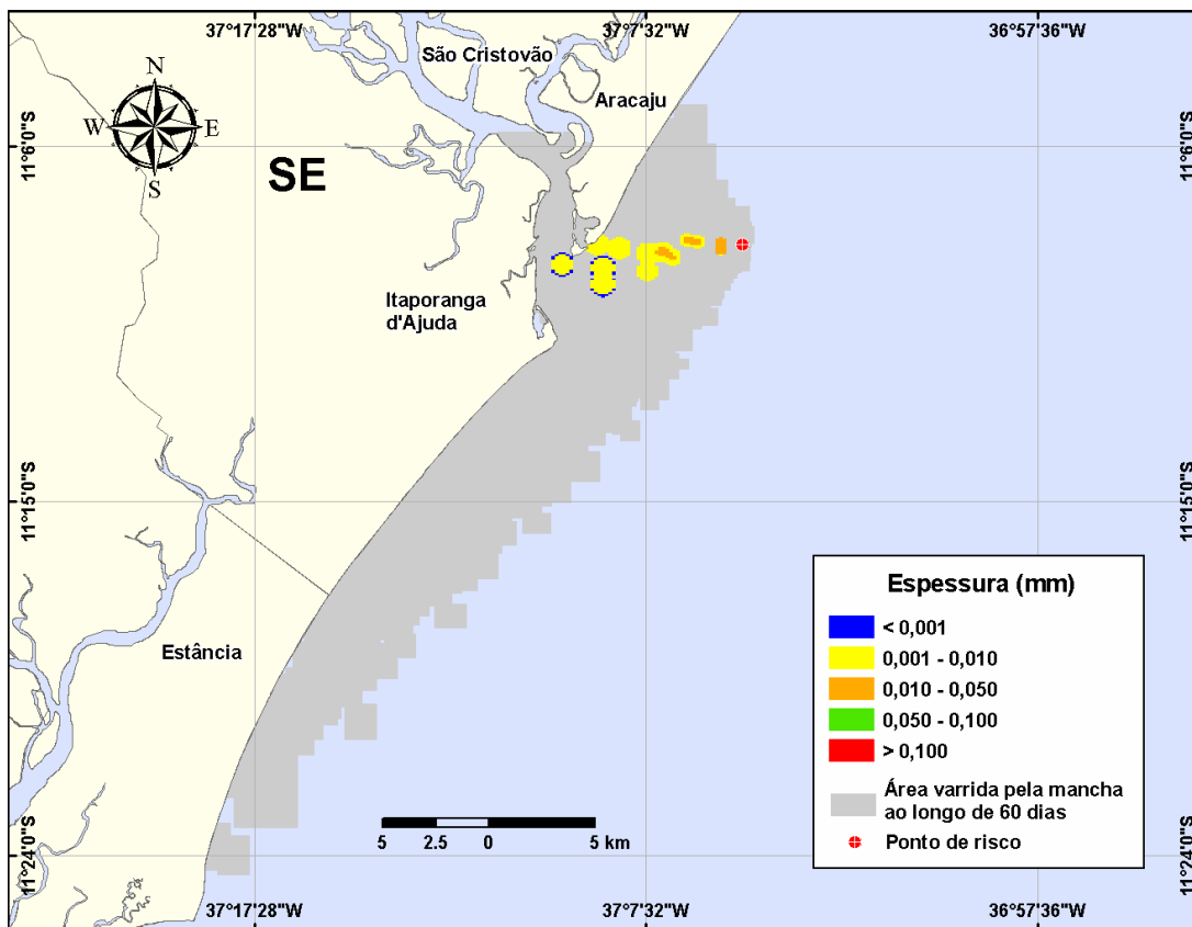
Figura III-130 - DET_PE5_INV_7500_60D. Cenário determinístico crítico para um derrame ocorrido durante o inverno com óleo cru, a partir do Ponto-PE5 no Campo Guaricema.
