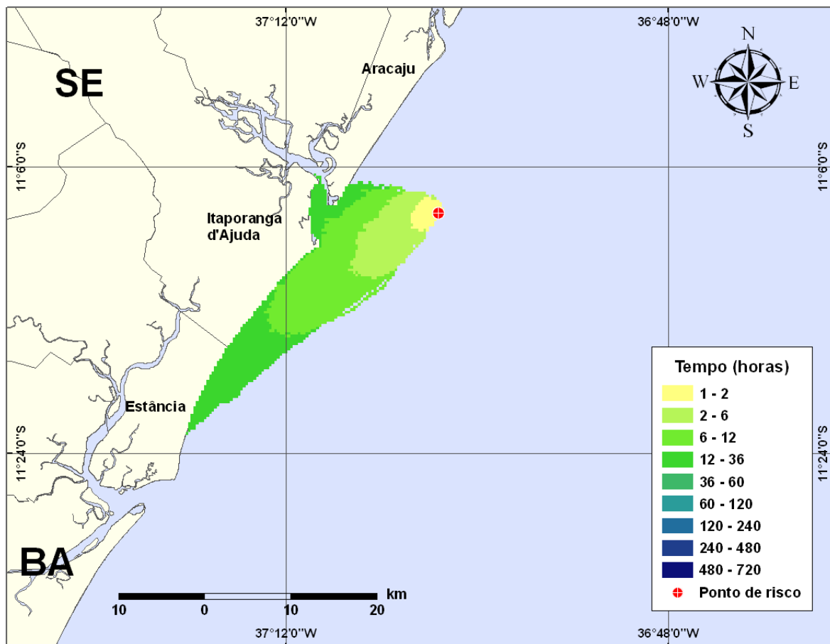
Figura III-6 - Cenário PGA3_DIESEL_VER_200_30D. (Fase: instalação/perfuração). Contornos de deslocamento de óleo na água para um acidente com óleo tipo DIESEL, ocorrendo no Ponto-PGA3, do Campo Guaricema, durante os meses de verão (janeiro a março), com derrame de 200 m 3 (instantâneo), após 30 dias de simulação.
