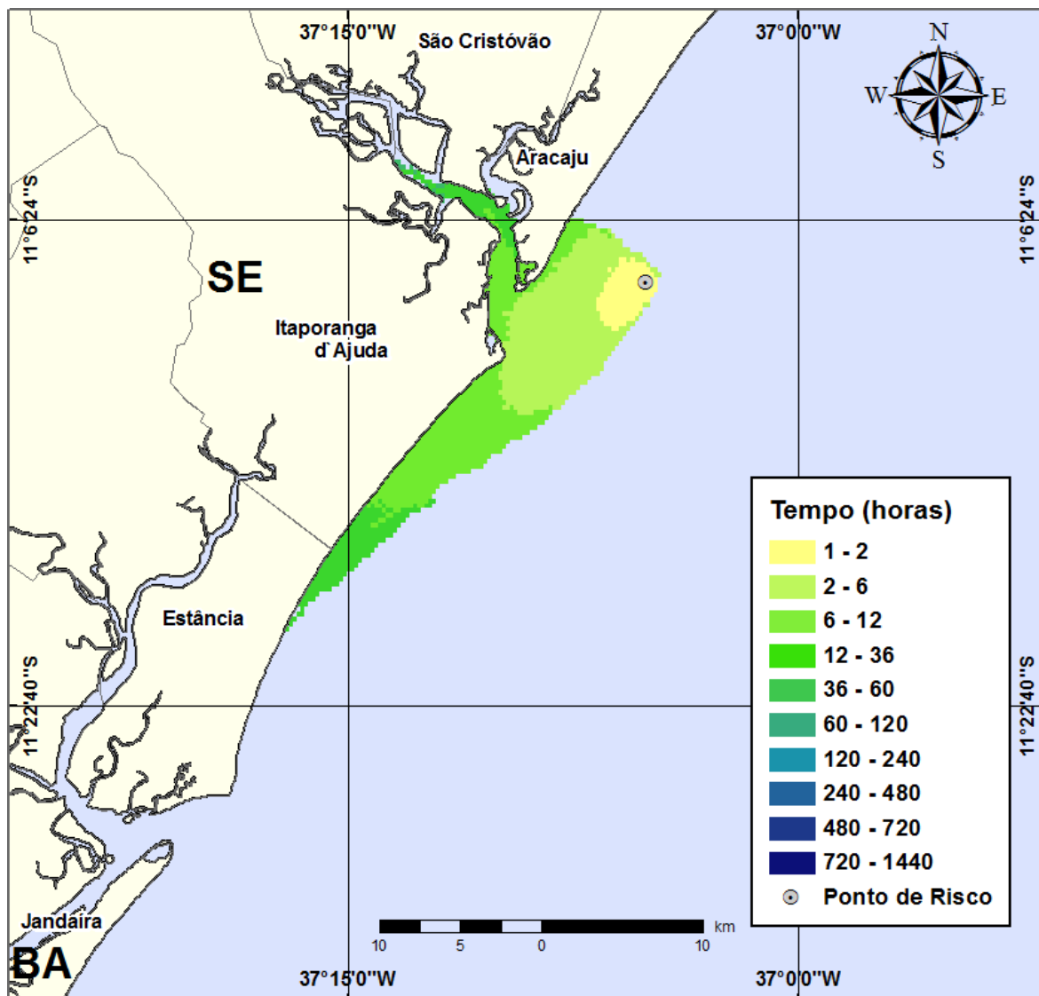
Figura III-42 - Cenário PE5_VER_200_30D (Fase: perfuração). Contornos de deslocamento de óleo na água para um acidente com óleo tipo GUARICEMA ocorrendo no Ponto-PE5, durante os meses de verão (janeiro a março), com derrame de 200 m 3 (instantâneo), após 30 dias de simulação.
