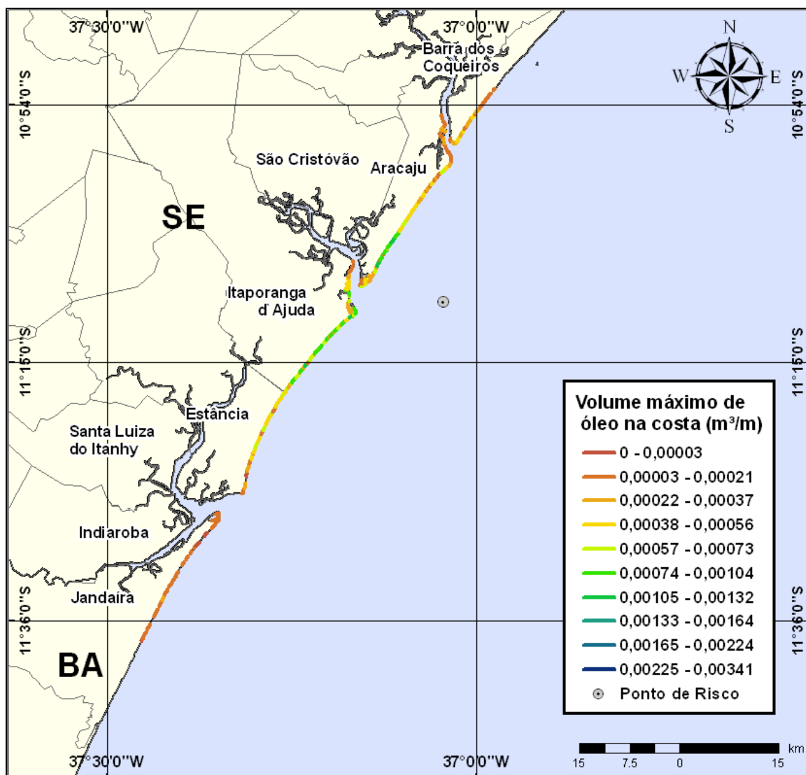
Figura III-88 - Cenário PGA10_INV_8_30D (Fase: Fase:instalação/produção /perfuração). Linhas de volume máximo de óleo na costa para um acidente com óleo tipo GUARICEMA ocorrendo no Ponto-PGA10, durante os meses de inverno (junho a agosto), com derrame de 8 m 3 (instantâneo), após 30 dias de simulação.
