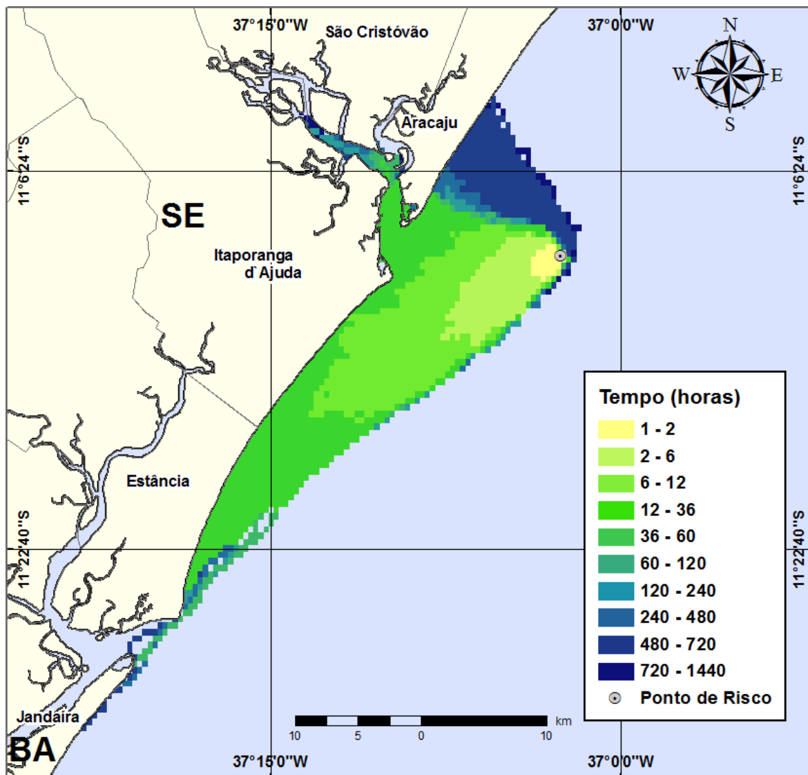
Figura III-34 - Cenário PGA10_VER_7500_60D (Fase: perfuração). Contornos de deslocamento de óleo na água para um acidente com óleo tipo GUARICEMA ocorrendo no Ponto-PGA10, durante os meses de verão (janeiro a março), com derrame de 7.500 m 3 (ao longo de 30 dias), após 60 dias de simulação.
