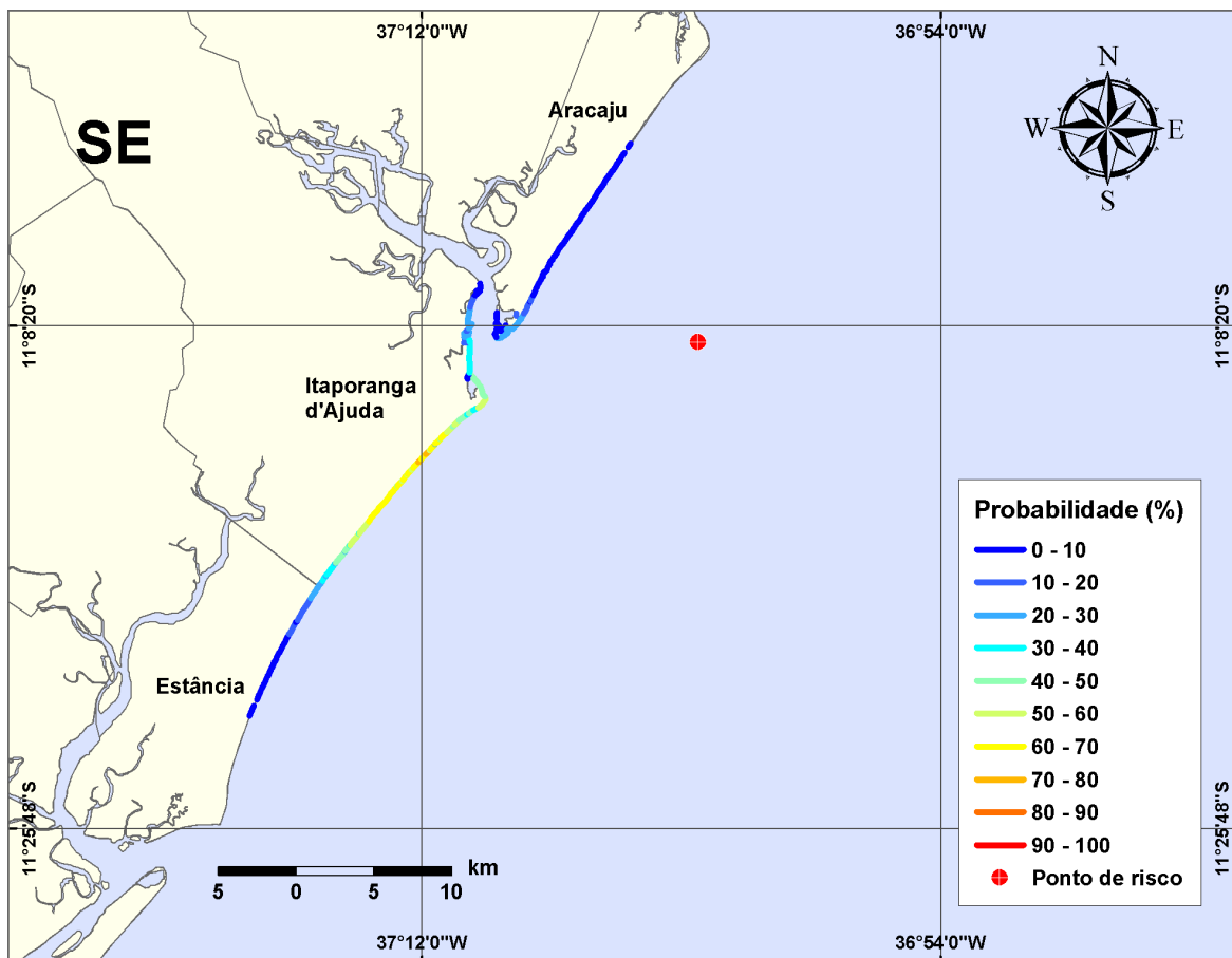
Figura III-67 - Cenário PGA3_DIESEL_INV_200_30D. (Fase: instalação/perfuração). Linhas de probabilidade de óleo na costa para um acidente com óleo tipo DIESEL, ocorrendo no Ponto-PGA3, do Campo Guaricema, durante os meses de inverno (junho a agosto), com derrame de 200 m 3 (instantâneo), após 30 dias de simulação.
