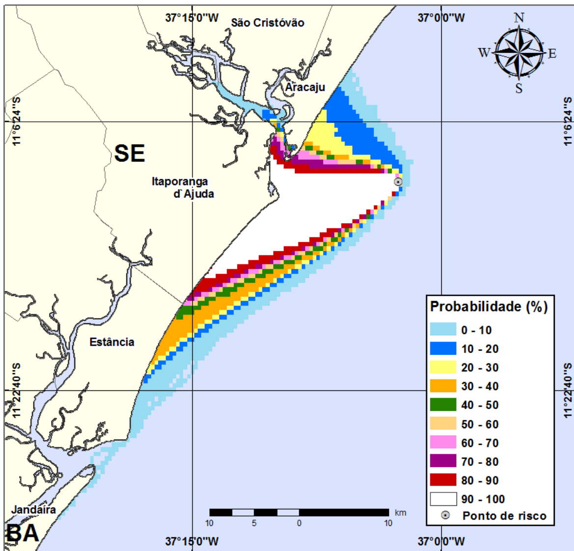
Figura III-33 - Cenário PGA10_VER_7500_60D (Fase: perfuração). Contornos de probabilidade de óleo na água para um acidente com óleo tipo GUARICEMA ocorrendo no Ponto-PGA10, durante os meses de verão (janeiro a março), com derrame de 7.500 m 3 (ao longo de 30 dias), após 60 dias de simulação.
