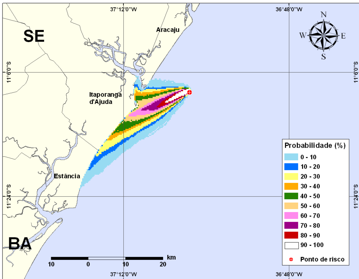
Figura III-5 - Cenário PGA3_DIESEL_VER_200_30D. (Fase: instalação/perfuração). Contornos de probabilidade de óleo na água para um acidente com óleo tipo DIESEL, ocorrendo no Ponto-PGA3, do Campo Guaricema, durante os meses de verão (janeiro a março), com derrame de 200 m 3 (instantâneo), após 30 dias de simulação.
