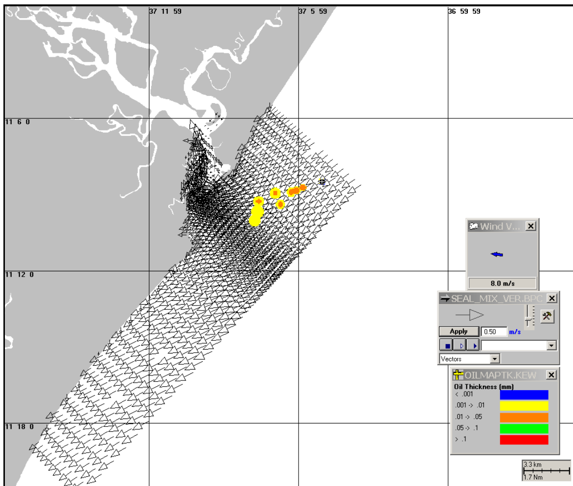
Figura III-126 - Cenário DET_PE5_VER_7500_60D. Condições meteorológicas e oceanográficas e espessuras da mancha de óleo 4 horas após o início da simulação.
