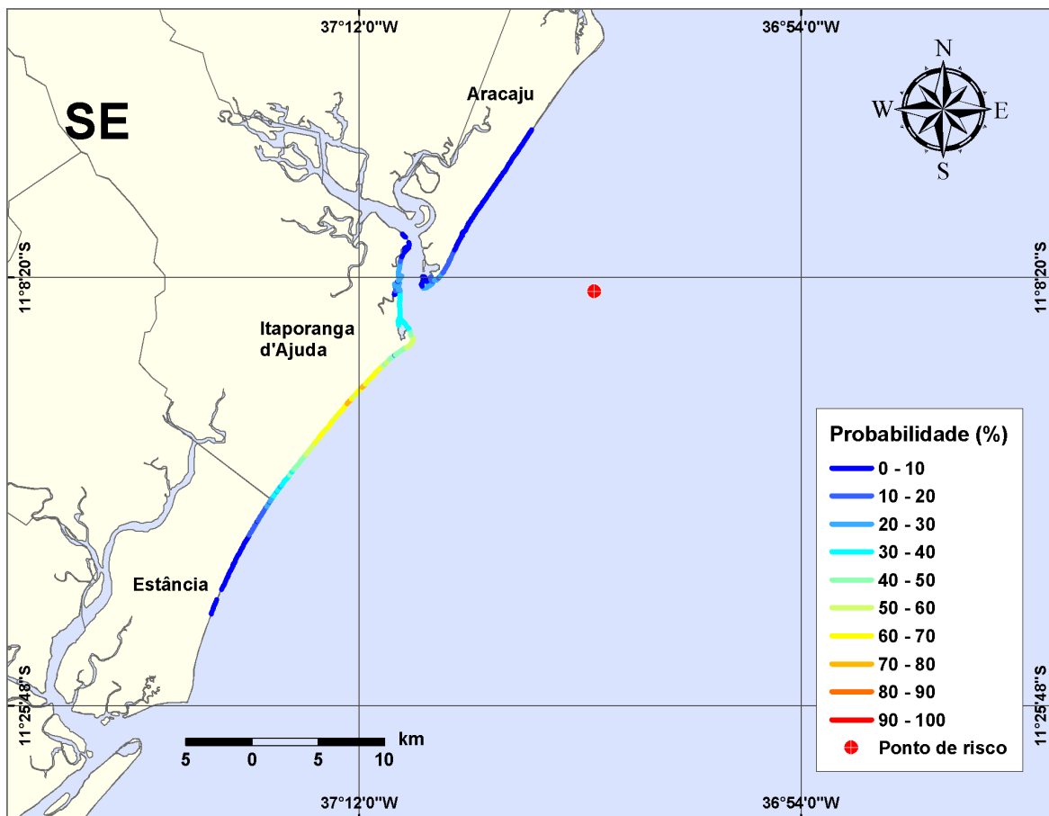
Figura III-71 - Cenário PGA3_DIESEL_INV_PC_30D. (Fase: instalação/produção). Linhas de probabilidade de óleo na costa para um acidente com óleo tipo DIESEL, ocorrendo no Ponto-PGA3, do Campo Guaricema, durante os meses de inverno (junho a agosto), com derrame de 500 m 3 (instantâneo), após 30 dias de simulação.
