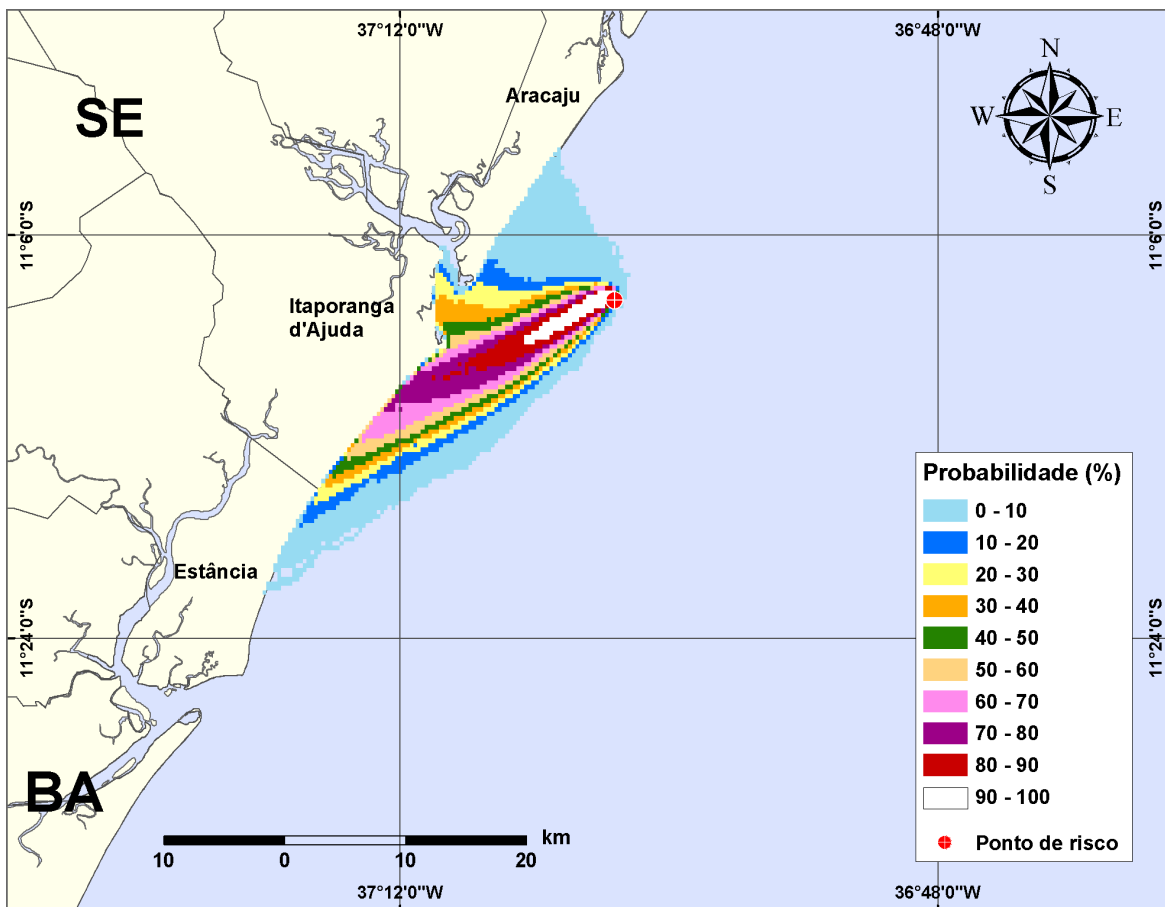
Figura III-69 - Cenário PGA3_DIESEL_INV_PC_30D. (Fase: instalação/perfuração). Contornos de probabilidade de óleo na água para um acidente com óleo tipo DIESEL, ocorrendo no Ponto-PGA3, do Campo Guaricema, durante os meses de inverno (junho a agosto), com derrame de 500 m 3 (instantâneo), após 30 dias de simulação.
