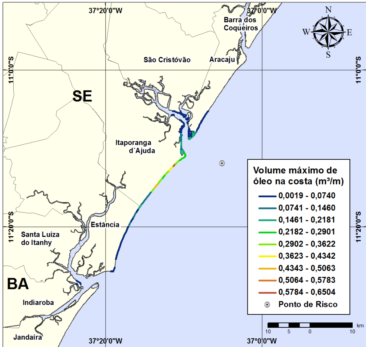
Figura III-56 - Cenário GA58_VER_7500_60D. (Fase: produção). Linhas de volume máximo de óleo na costa para um acidente com óleo tipo GUARICEMA, ocorrendo no Ponto-GA58, do Campo Guaricema, durante os meses de verão (janeiro a março), com derrame de 7.500 m 3 (ao longo de 30 dias), após 60 dias de simulação.
