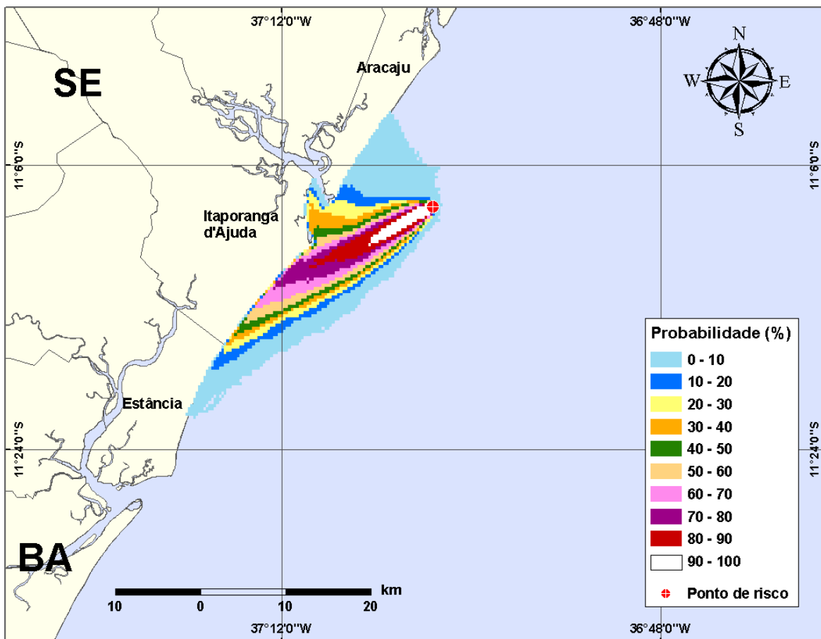
Figura III-77 - Cenário PGA3_INV_200_30D. (Fase: instalação/produção). Contornos de probabilidade de óleo na água para um acidente com óleo tipo GUARICEMA, ocorrendo no Ponto-PGA3, do Campo Guaricema, durante os meses de inverno (junho a agosto), com derrame de 200 m 3 (instantâneo), após 30 dias de simulação.
