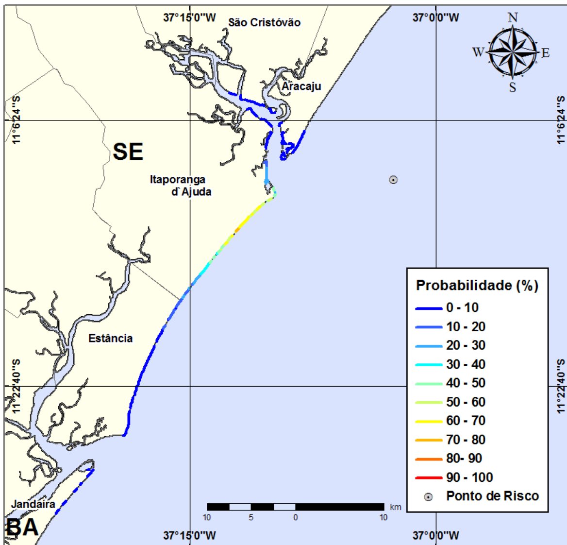
Figura III-31 - Cenário PGA10_VER_200_30D. (Fase:instalação/produção/ perfuração). Linhas de probabilidade de óleo na costa para um acidente com óleo tipo GUARICEMA ocorrendo no Ponto-PGA10, durante os meses de verão (janeiro a março), com derrame de 200 m 3 (instantâneo), após 30 dias de simulação.
