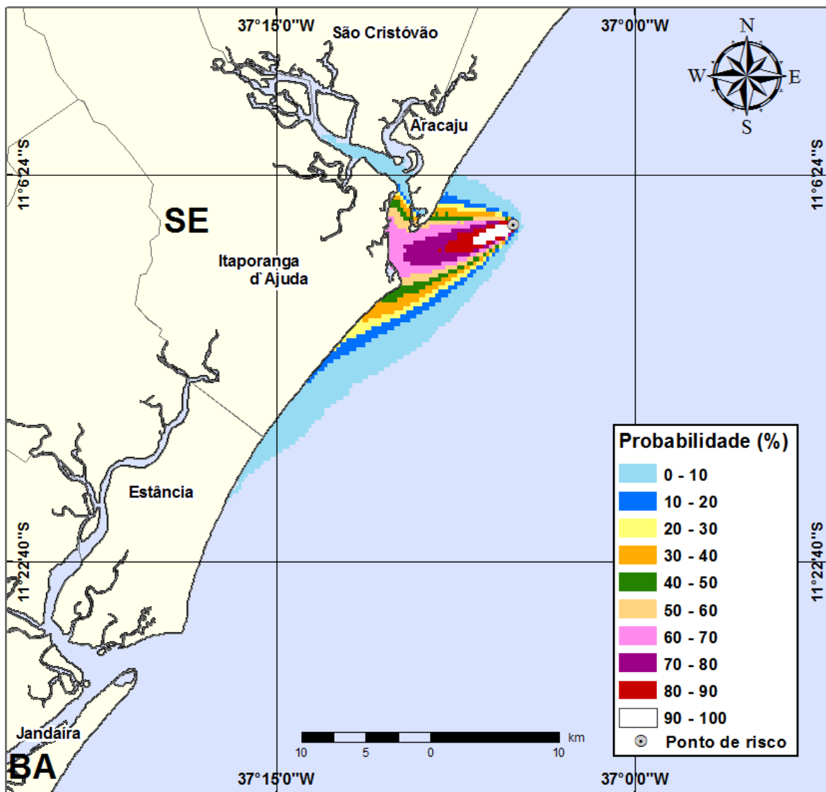
Figura III-37 - Cenário PE5_VER_8_30D (Fase: perfuração). Contornos de probabilidade de óleo na água para um acidente com óleo tipo GUARICEMA ocorrendo no Ponto-PE5, durante os meses de verão (janeiro a março), com derrame de 8 m 3 (instantâneo), após 30 dias de simulação.
