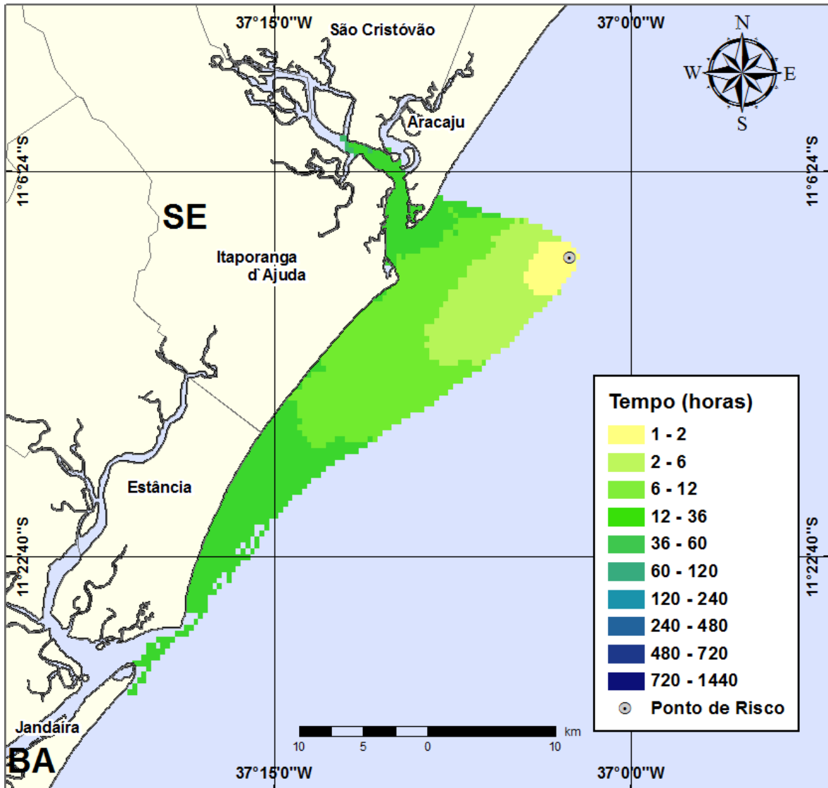
Figura III-26 - Cenário PGA10_VER_8_30D. (Fase:instalação/produção/perfuração) Contornos de deslocamento de óleo na água para um acidente ocorrendo no Ponto-PGA10, durante os meses de verão (janeiro a março), com derrame de 8 m 3 (instantâneo), após 30 dias de simulação.
