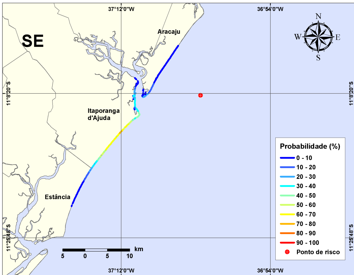
Figura III-75 - Cenário PGA3_INV_8_30D. (Fase: instalação/produção). Linhas de probabilidade de óleo na costa para um acidente com óleo tipo GUARICEMA, ocorrendo no Ponto-PGA3, do Campo Guaricema, durante os meses de inverno (junho a agosto), com derrame de 8 m 3 (instantâneo), após 30 dias de simulação.
