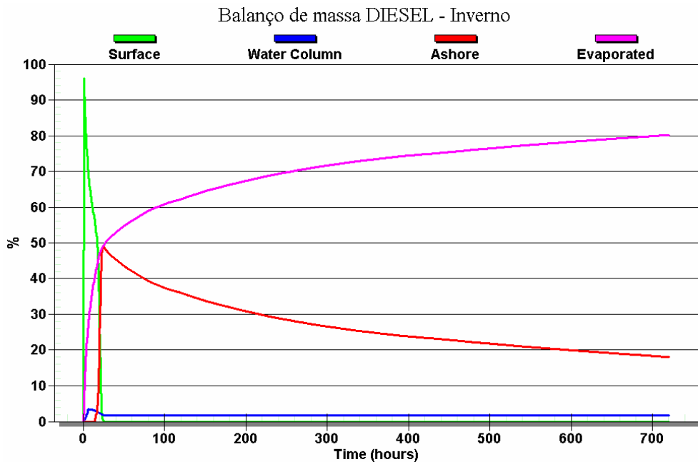
Figura III-129- Balanço de massa do cenário DET_PGA3_DIESEL_INV_500_30D.
