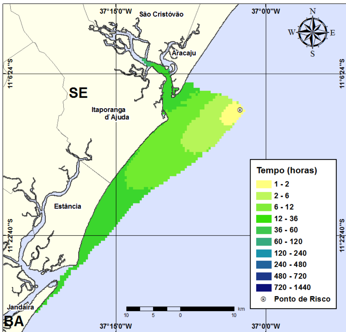
Figura III-30 - Cenário PGA10_VER_200_30D (Fase:instalação/produção/perfuração). Contornos de deslocamento de óleo na água para um acidente com óleo tipo GUARICEMA ocorrendo no Ponto-PGA10, durante os meses de verão (janeiro a março), com derrame de 200 m 3 (instantâneo), após 30 dias de simulação.
