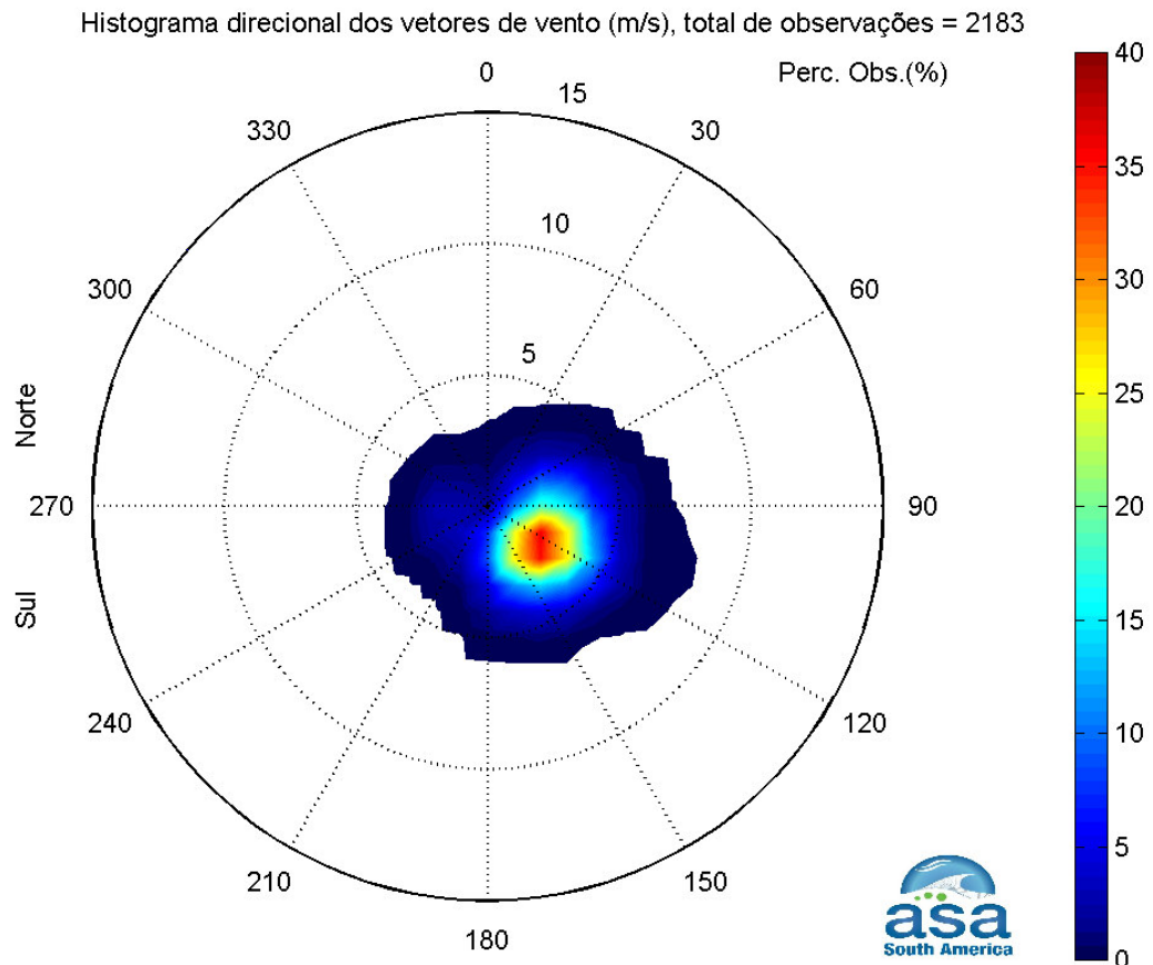
Figura II-7 - Histograma direcional dos vetores de vento INFRATERO Aracaju para o inverno (junho a agosto de 2002), na posição 10^{\circ}59'S e 37^{\circ}04'W . Os círculos concêntricos indicam a intensidade do vetor de vento (m/s), enquanto que a barra de cores (lateral) indica a porcentagem de incidência. A direção apresentada refere-se ao norte geográfico e segue a convenção meteorológica.
