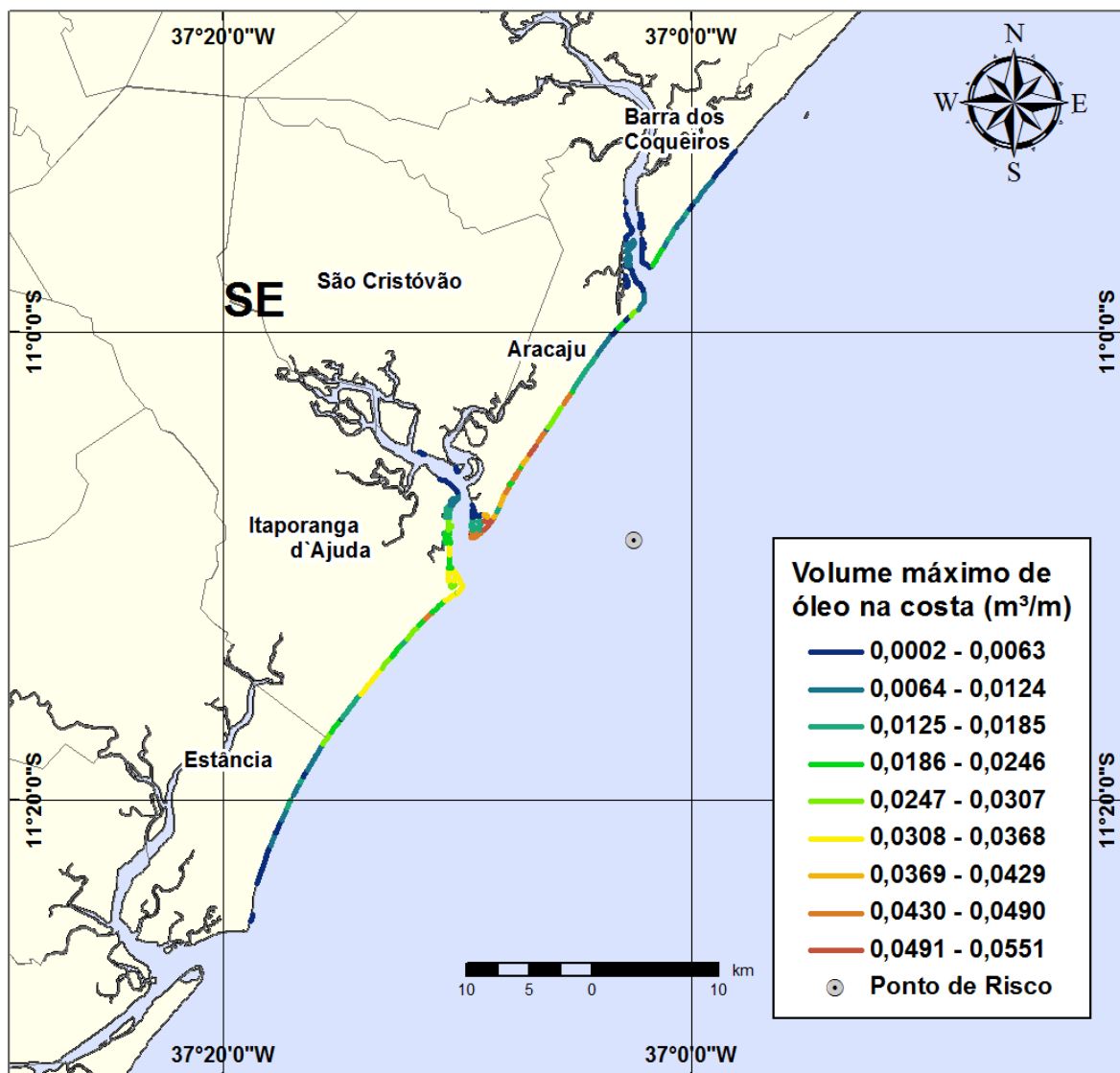
Figura III-84 - Cenário PGA3_INV_264_30D. (Fase: produção). Linhas de volume máximo de óleo na costa para um acidente com óleo tipo GUARICEMA, ocorrendo no Ponto-PGA3, do Campo Guaricema, durante os meses de inverno (junho a agosto), com derrame de 264 m 3 (instantâneo), após 30 dias de simulação.
