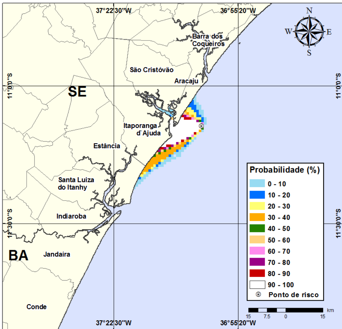
Figura III-49 - Cenário GA07_VER_7500_60D. (Fase: produção). Contornos de probabilidade de óleo na água para um acidente com óleo tipo GUARICEMA, ocorrendo no Ponto-GA07, do Campo Guaricema, durante os meses de verão (janeiro a março), com derrame de 7.500 m 3 (ao longo de 30 dias), após 60 dias de simulação.
