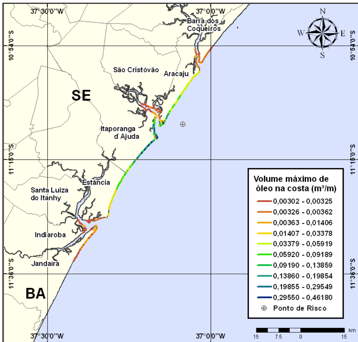
Figura III-108 - Cenário PE5_INV_7500_60D (Fase: perfuração). Linhas de volume máximo de óleo na costa para um acidente com óleo tipo GUARICEMA ocorrendo no Ponto-PE5, durante os meses de inverno (junho a agosto), com derrame de 7.500 m 3 (ao longo de 30 dias), após 60 dias de simulação.
