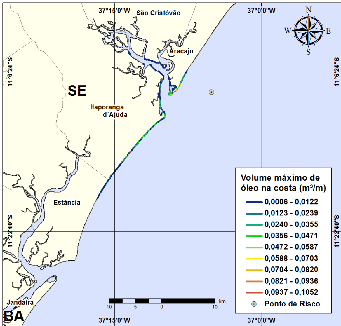
Figura III-44 - Cenário PE5_VER_200_30D (Fase: perfuração). Linhas de volume máximo de óleo na costa para um acidente com óleo tipo GUARICEMA ocorrendo no Ponto-PE5, durante os meses de verão (janeiro a março), com derrame de 200 m 3 (instantâneo), após 30 dias de simulação.
