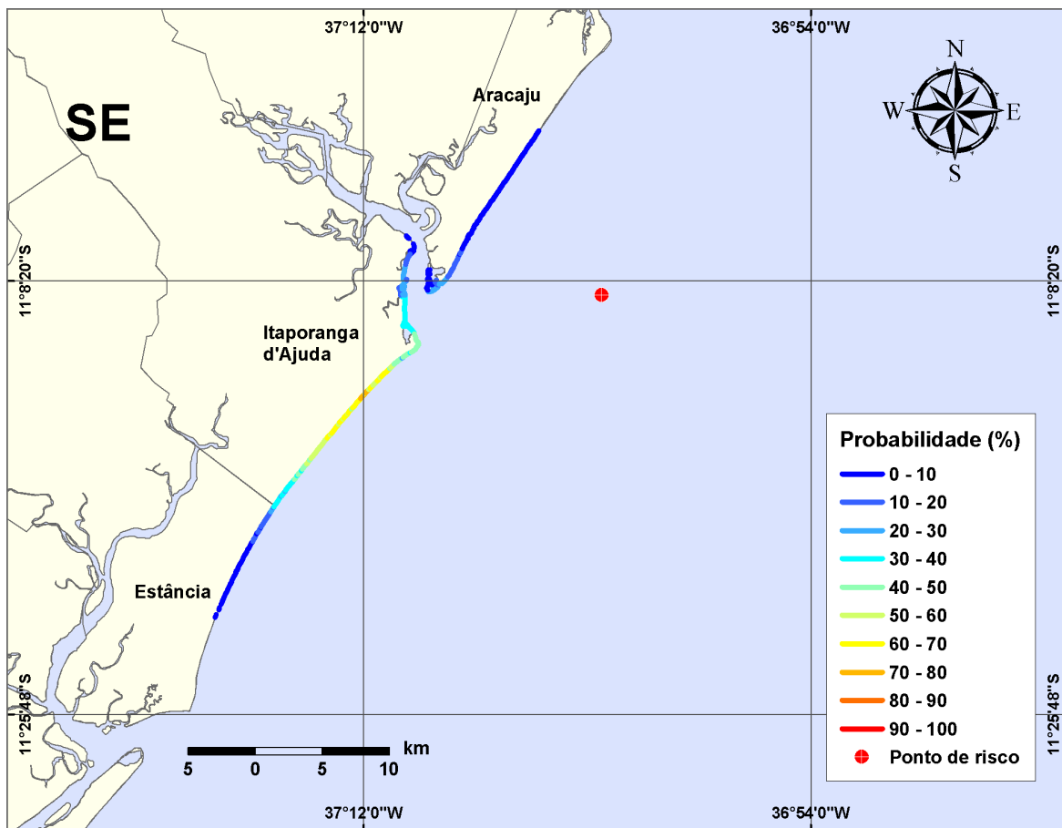
Figura III-63 - Cenário PGA3_DIESEL_INV_8_30D. (Fase: instalação/perfuração). Linhas de probabilidade de óleo na costa para um acidente com óleo tipo DIESEL, ocorrendo no Ponto-PGA3, do Campo Guaricema, durante os meses de inverno (junho a agosto), com derrame de 8 m 3 (instantâneo), após 30 dias de simulação.
