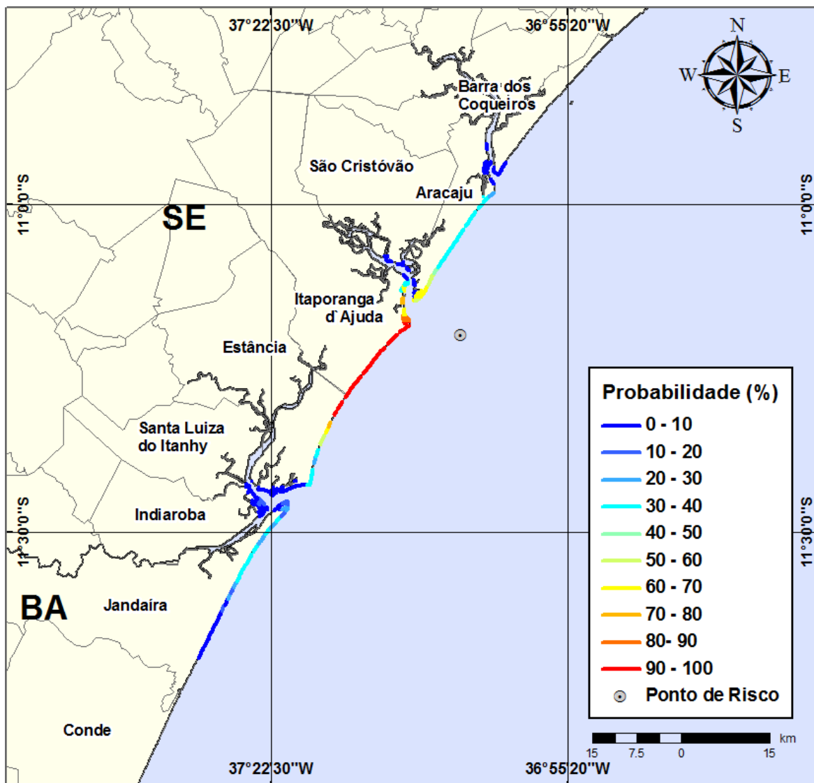
Figura III-115 - Cenário GA58_INV_7500_60D. (Fase: produção). Linhas de probabilidade de óleo na costa para um acidente com óleo tipo GUARICEMA, ocorrendo no Ponto-GA58, do Campo Guaricema, durante os meses de inverno (junho a agosto), com derrame de 7.500 m 3 (ao longo de 30 dias), após 60 dias de simulação.
