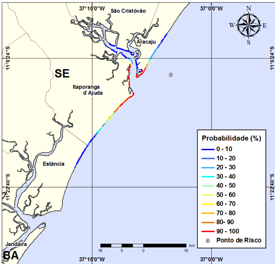
Figura III-47 - Cenário PE5_VER_7500_30D (Fase: perfuração). Linhas de probabilidade de óleo na costa para um acidente com óleo tipo GUARICEMA ocorrendo no Ponto-GPE5A70, durante os meses de verão (janeiro a março), com derrame de 7.500 m 3 (ao longo de 30 dias), após 60 dias de simulação.
