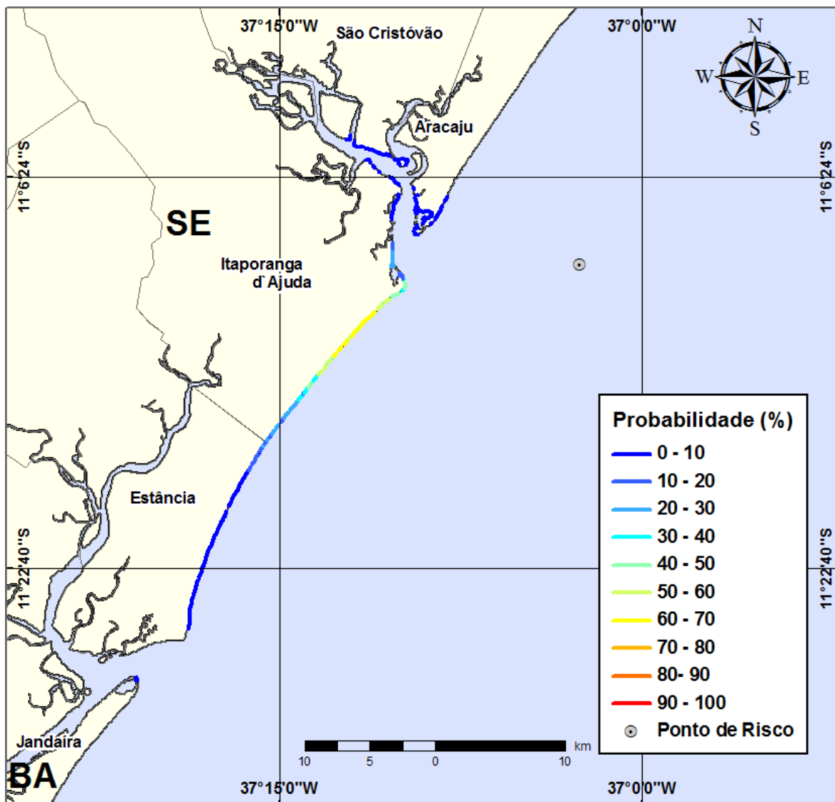
Figura III-27 - Cenário PGA10_VER_8_30D. (Fase: instalação/produção/perfuração). Linhas de probabilidade de óleo na costa para um acidente ocorrendo no Ponto-PGA10, durante os meses de verão (janeiro a março), com derrame de 8 m 3 (instantâneo), após 30 dias de simulação.
