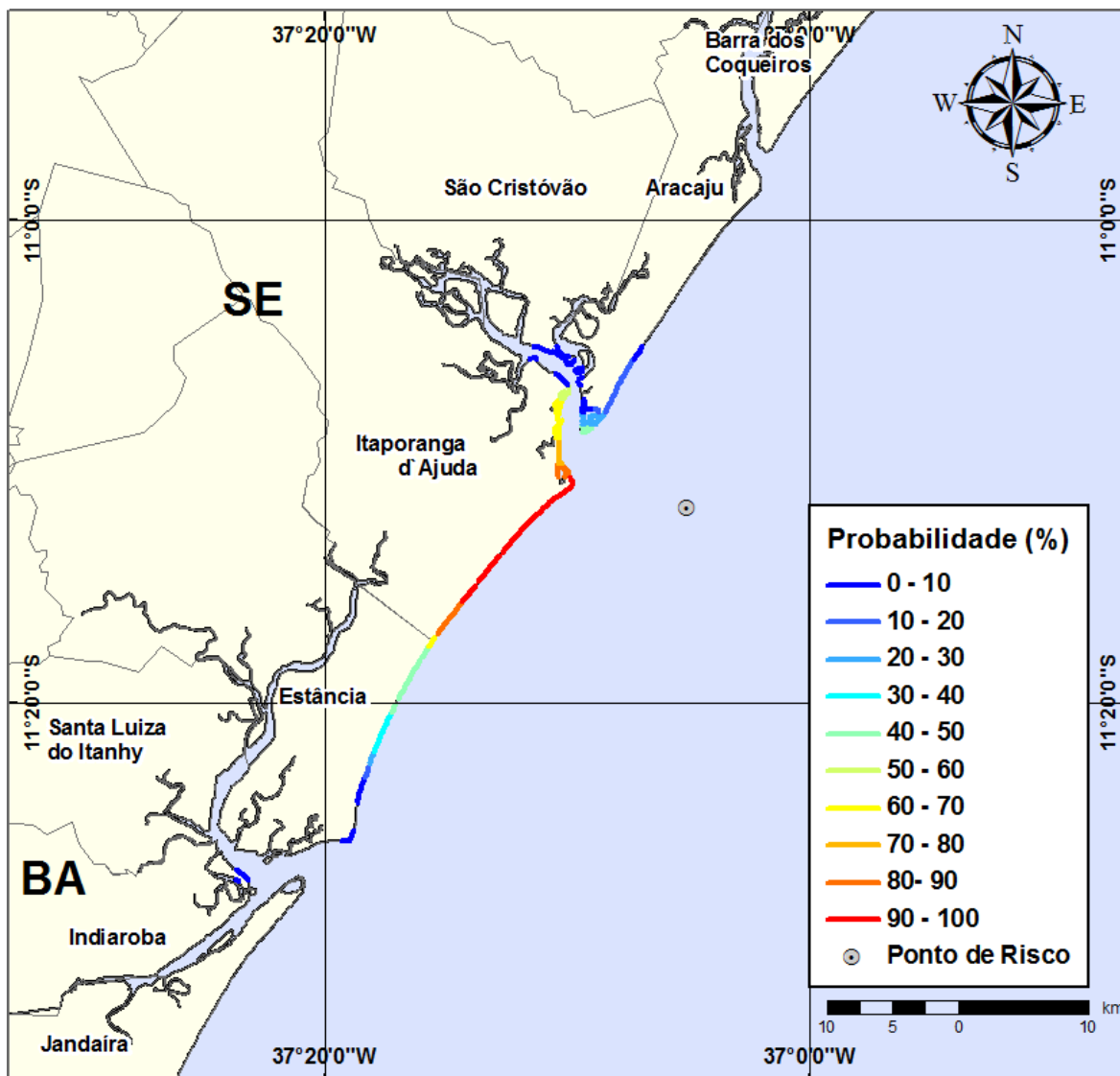
Figura III-55 - Cenário GA58_VER_7500_60D. (Fase: produção). Linhas de probabilidade de óleo na costa para um acidente com óleo tipo GUARICEMA, ocorrendo no Ponto-GA58, do Campo Guaricema, durante os meses de verão (janeiro a março), com derrame de 7.500 m 3 (ao longo de 30 dias), após 60 dias de simulação.
