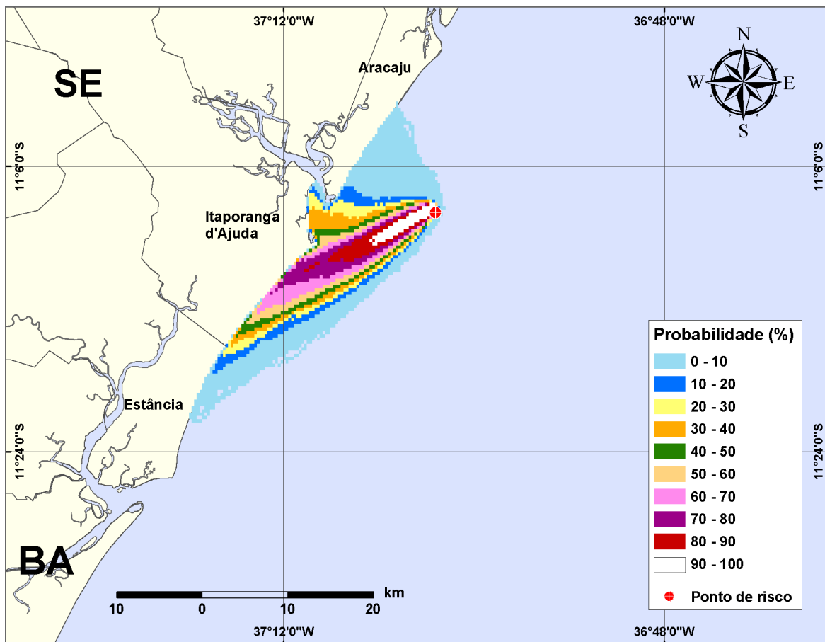
Figura III-65 - Cenário PGA3_DIESEL_INV_200_30D. (Fase: instalação/perfuração). Contornos de probabilidade de óleo na água para um acidente com óleo tipo DIESEL, ocorrendo no Ponto-PGA3, do Campo Guaricema, durante os meses de inverno (junho a agosto), com derrame de 200 m 3 (instantâneo), após 30 dias de simulação.
