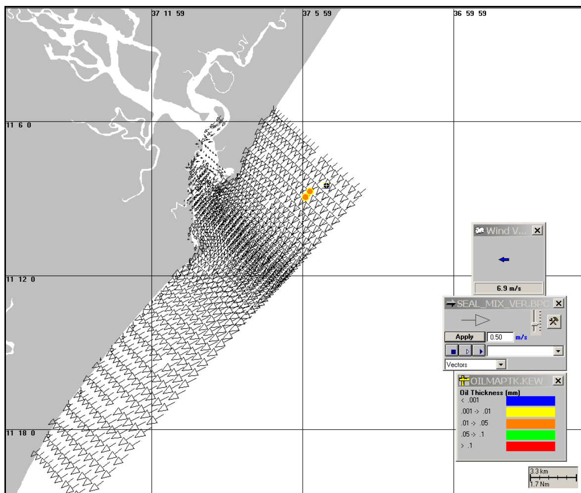
Figura III-125 - Cenário DET_PE5_VER_7500_60D. Condições meteorológicas e oceanográficas e espessuras da mancha de óleo no início da simulação.
