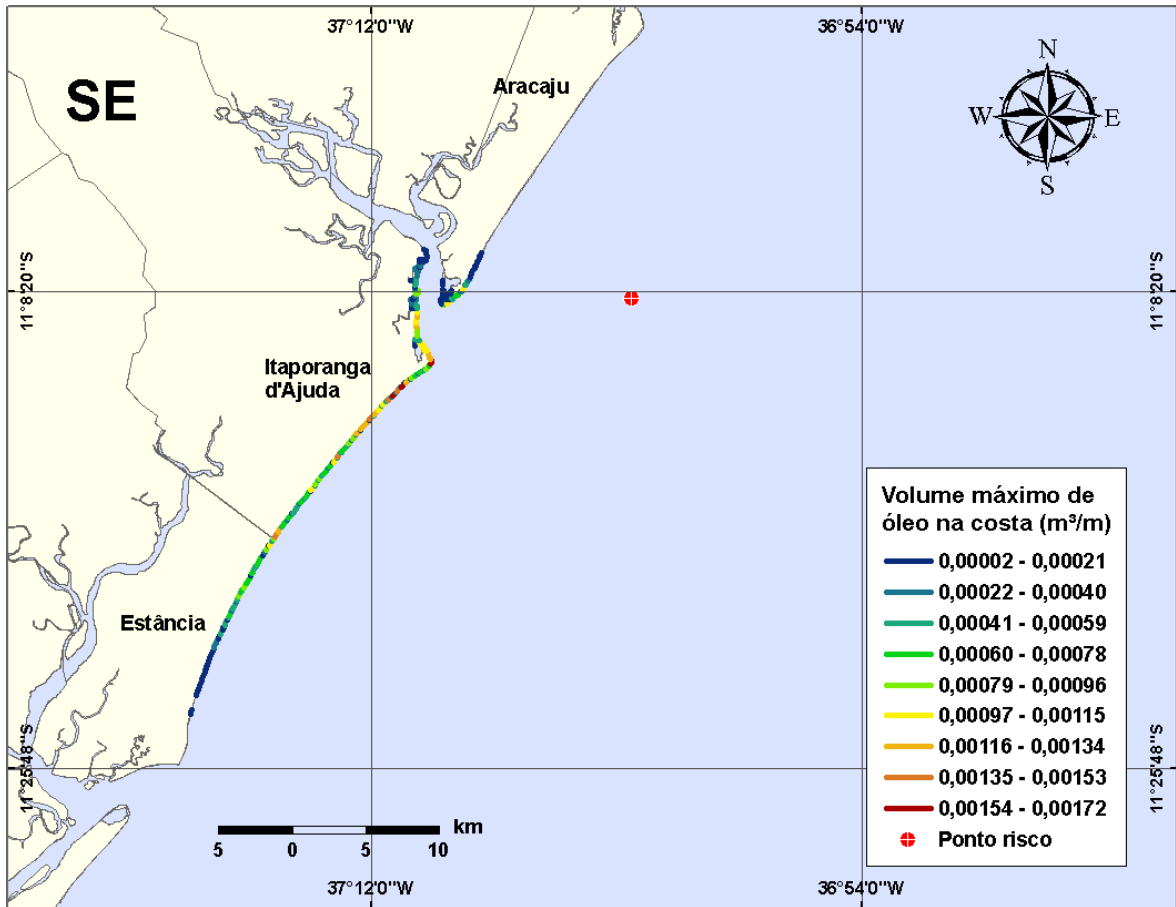
Figura III-16 - Cenário PGA3_VER_8_30D. (Fase: instalação/produção). Linhas de volume máximo de óleo na costa para um acidente com óleo tipo GUARICEMA, ocorrendo no Ponto-PGA3, do Campo Guaricema, durante os meses de verão (janeiro a março), com derrame de 8 m³ (instantâneo), após 30 dias de simulação.
