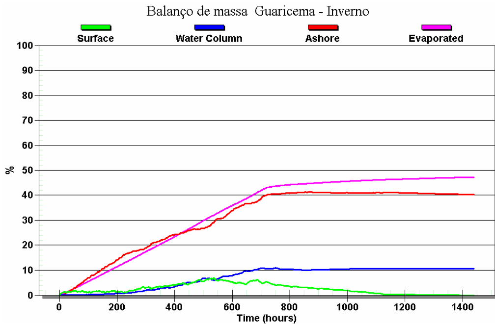
Figura III-138 - Balanço de massa do cenário DET_FREQ_PE5_7500_PC_60D.
