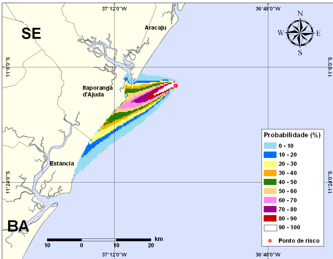
Figura III-9 - Cenário PGA3_DIESEL_VER_500_30D. (Fase: instalação/perfuração). Contornos de probabilidade de óleo na água para um acidente com óleo tipo DIESEL, ocorrendo no Ponto-PGA3, do Campo Guaricema, durante os meses de verão (janeiro a março), com derrame de 500 m 3 (instantâneo), após 30 dias de simulação.
