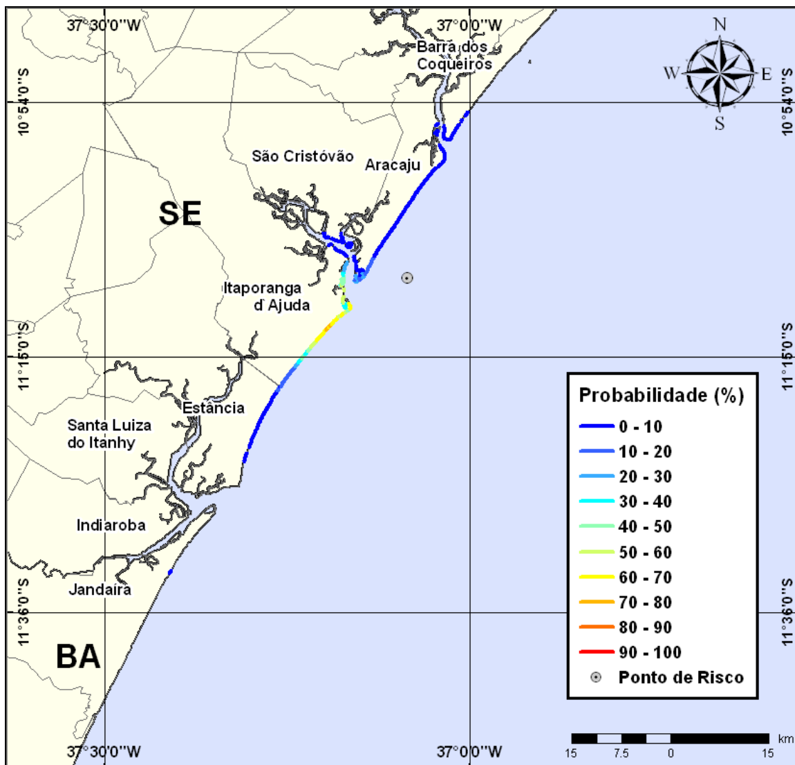
Figura III-103 - Cenário PE5_INV_200_30D (Fase: perfuração). Linhas de probabilidade de óleo na costa para um acidente com óleo tipo GUARICEMA ocorrendo no Ponto-PE5, durante os meses de inverno (junho a agosto), com derrame de 200 m 3 (instantâneo), após 30 dias de simulação.
