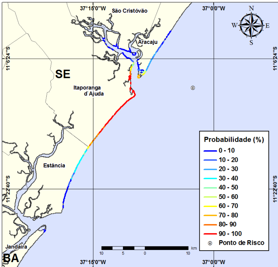
Figura III-35 - Cenário PGA10_VER_7500_60D (Fase: perfuração). Linhas de probabilidade de óleo na costa para um acidente com óleo tipo GUARICEMA ocorrendo no Ponto-PGA10, durante os meses de verão (janeiro a março), com derrame de 7.500 m 3 (ao longo de 30 dias), após 60 dias de simulação.
