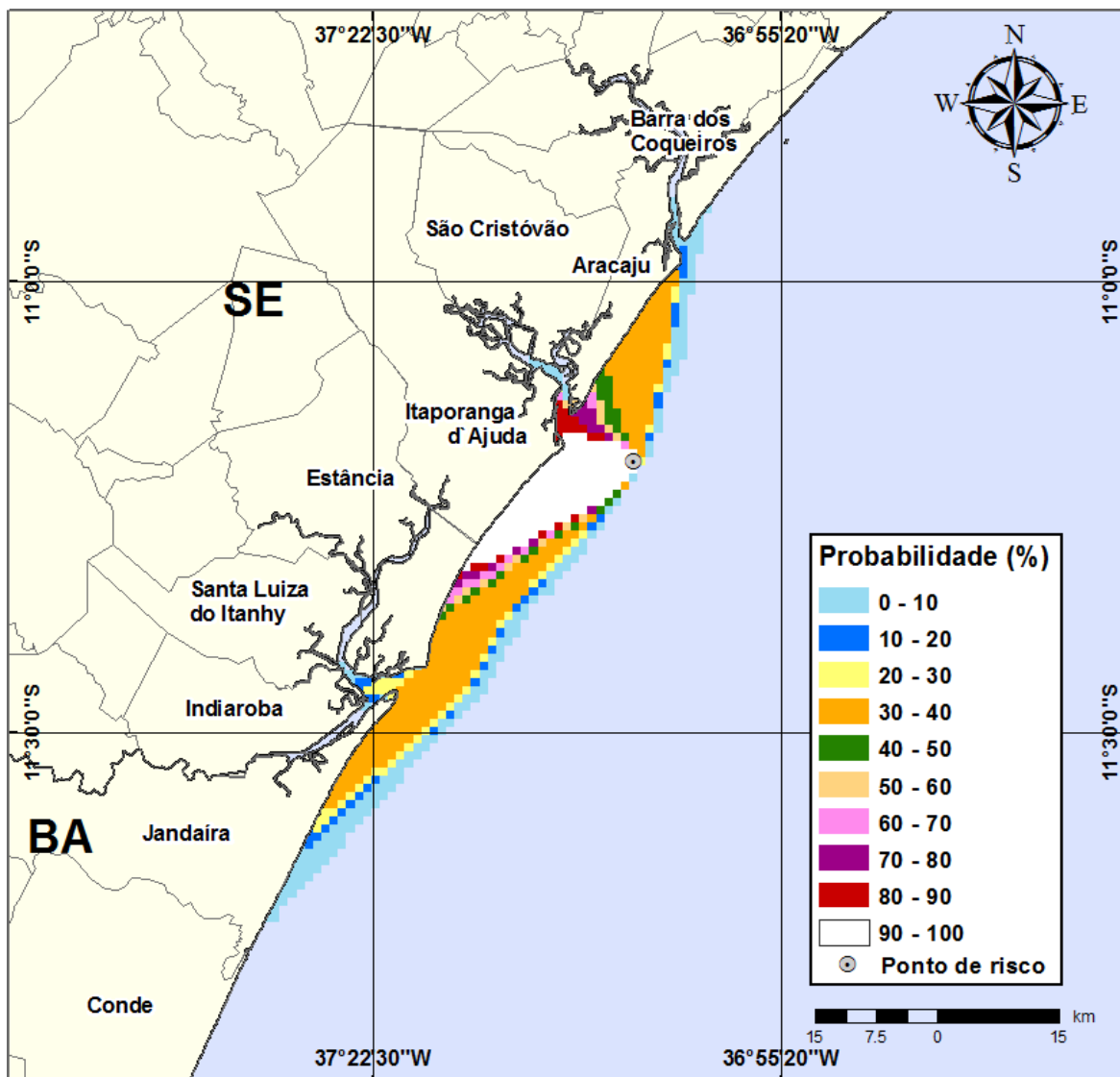
Figura III-113 - Cenário GA58_INV_7500_60D. (Fase: produção). Contornos de probabilidade de óleo na água para um acidente com óleo tipo GUARICEMA, ocorrendo no Ponto-GA58, do Campo Guaricema, durante os meses de inverno (junho a agosto), com derrame de 7.500 m 3 (ao longo de 30 dias), após 60 dias de simulação.
