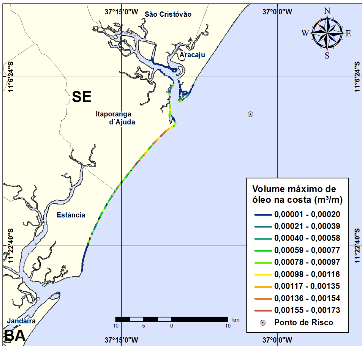
Figura III-28 - Cenário PGA10_VER_8_30D . (Fase: instalação/produção/perfuração). Linhas de volume máximo de óleo na costa para um acidente ocorrendo no Ponto-PGA10, durante os meses de verão (janeiro a março), com derrame de 8 m 3 (instantâneo), após 30 dias de simulação.
