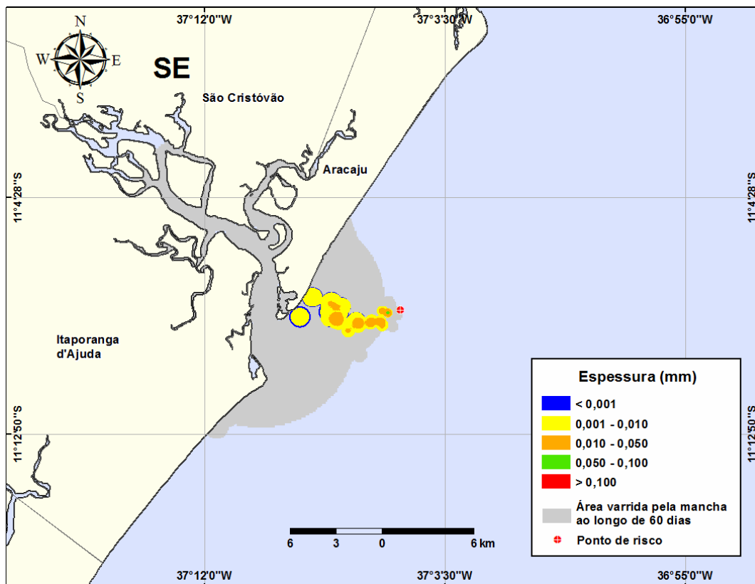
Figura III-135 - DET_FREQ_PE5_VER_7500_60D. Cenário determinístico para a condição mais frequente, para um derrame ocorrido durante o verão com óleo cru a partir do Ponto-PE5 no Campo Guaricema.
