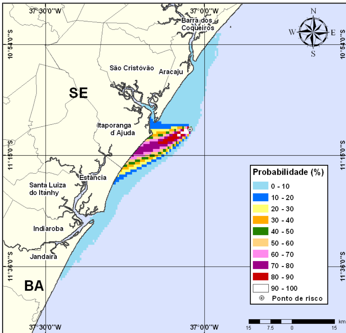
Figura III-89 - Cenário PGA10_INV_200_30D (Fase: Fase:instalação/produção/perfuração). Contornos de probabilidade de óleo na água para um acidente com óleo tipo GUARICEMA ocorrendo no Ponto-PGA10, durante os meses de inverno (junho a agosto), com derrame de 200 m 3 (instantâneo), após 30 dias de simulação.
