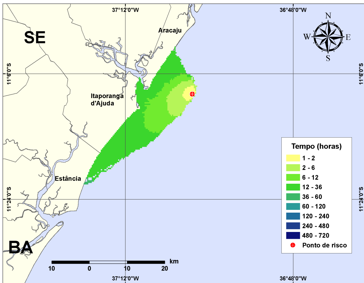
Figura III-70 - Cenário PGA3_DIESEL_INV_PC_30D. (Fase: instalação/perfuração). Contornos de deslocamento de óleo na água para um acidente com óleo tipo DIESEL, ocorrendo no Ponto-PGA3, do Campo Guaricema, durante os meses de inverno (junho a agosto), com derrame de 500 m 3 (instantâneo), após 30 dias de simulação.
