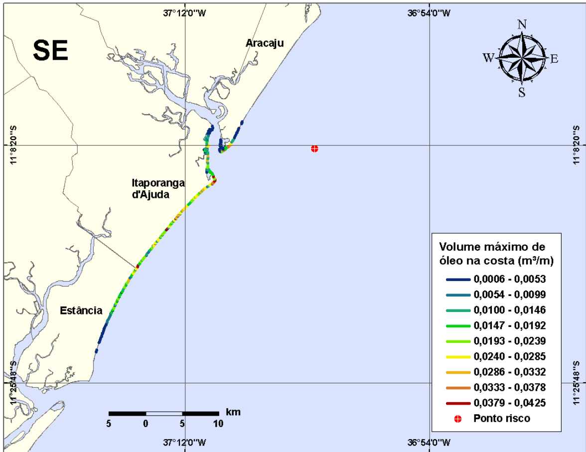
Figura III-20 - Cenário PGA3_VER_200_30D. (Fase: instalação/produção). Linhas de volume máximo de óleo na costa para um acidente com óleo tipo GUARICEMA, ocorrendo no Ponto-PGA3, do Campo Guaricema, durante os meses de verão (janeiro a março), com derrame de 200 m³ (instantâneo), após 30 dias de simulação.
