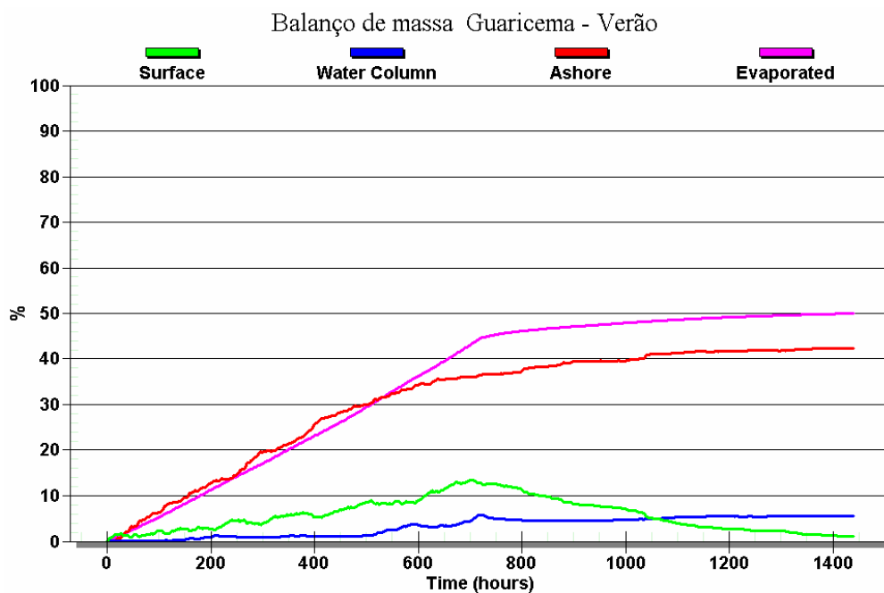
Figura III-136 - Balanço de massa do cenário DET_FREQ_PE5_VER_7500_60D.
