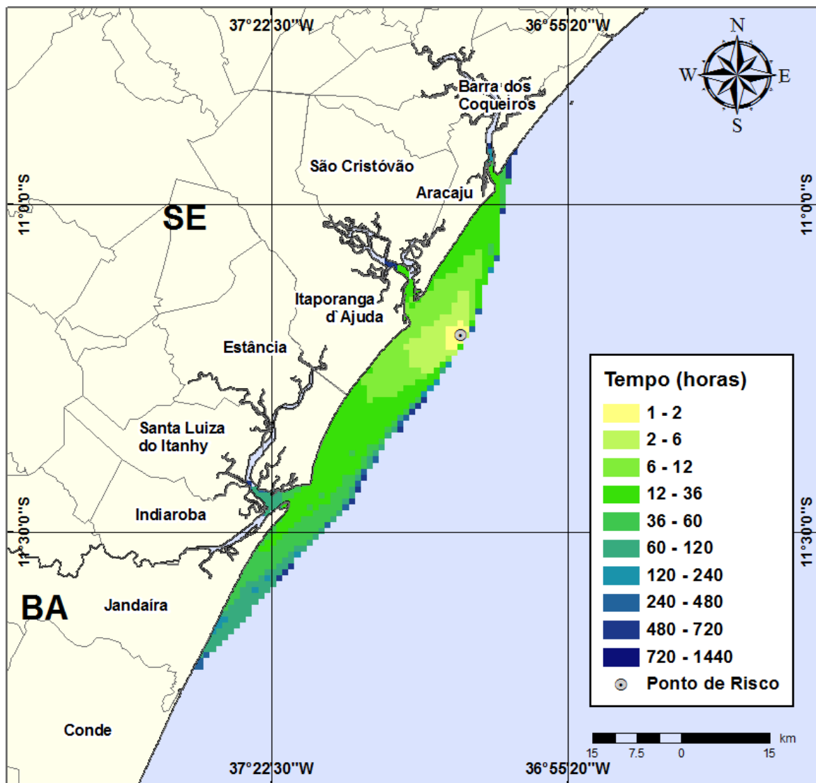
Figura III-114 - Cenário GA58_INV_7500_60D. (Fase: produção). Contornos de deslocamento de óleo na água para um acidente com óleo tipo GUARICEMA, ocorrendo no Ponto-GA58, do Campo Guaricema, durante os meses de inverno (junho a agosto), com derrame de 7.500 m 3 (ao longo de 30 dias), após 60 dias de simulação.
