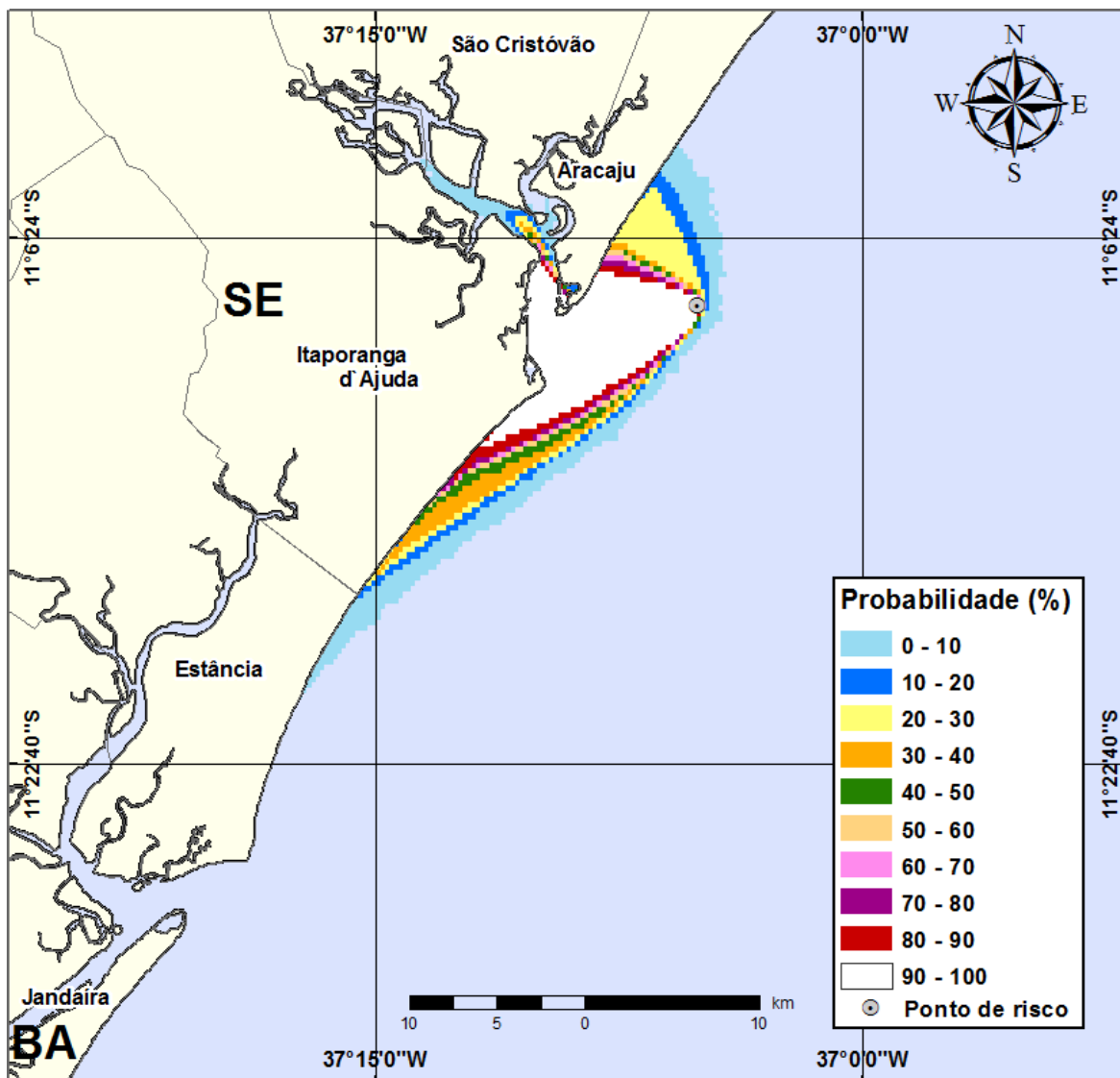
Figura III-45 - Cenário PE5_VER_7500_30D (Fase: perfuração). Contornos de probabilidade de óleo na água para um acidente com óleo tipo GUARICEMA ocorrendo no Ponto-PE5, durante os meses de verão (janeiro a março), com derrame de 7.500 m 3 (ao longo de 30 dias), após 60 dias de simulação.
