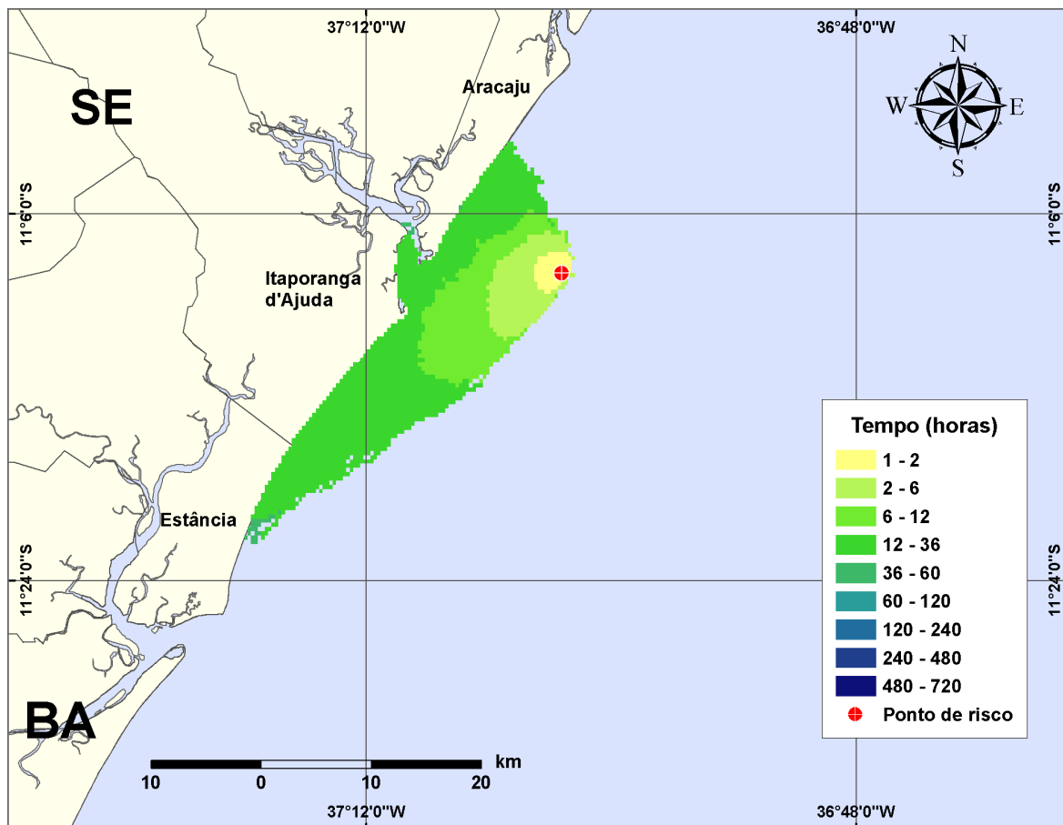
Figura III-62 - Cenário PGA3_DIESEL_INV_8_30D . (Fase: instalação/perfuração). Contornos de deslocamento de óleo na água para um acidente com óleo tipo DIESEL, ocorrendo no Ponto-PGA3, do Campo Guaricema, durante os meses de inverno (junho a agosto), com derrame de 8 \text{ m}^3 (instantâneo), após 30 dias de simulação.
