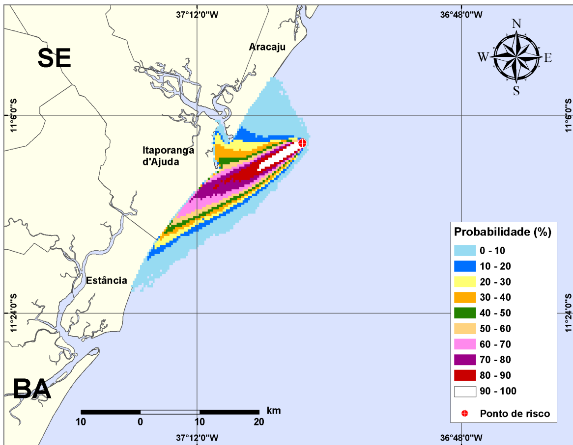
Figura III-73 - Cenário PGA3_INV_8_30D. (Fase: instalação/produção). Contornos de probabilidade de óleo na água para um acidente com óleo tipo GUARICEMA, ocorrendo no Ponto-PGA3, do Campo Guaricema, durante os meses de inverno (junho a agosto), com derrame de 8 m 3 (instantâneo), após 30 dias de simulação.
