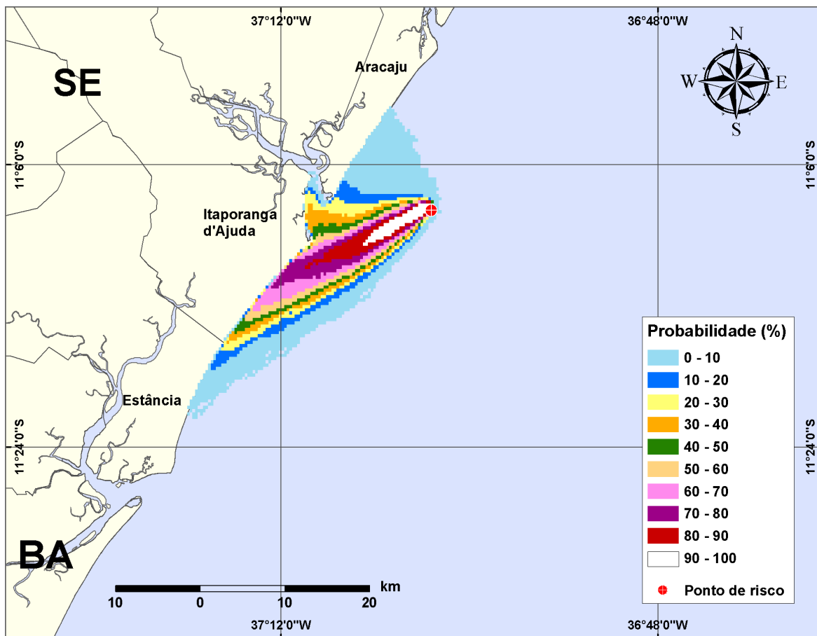
Figura III-61 - Cenário PGA3_DIESEL_INV_8_30D . (Fase: instalação/perfuração). Contornos de probabilidade de óleo na água para um acidente com óleo tipo DIESEL, ocorrendo no Ponto-PGA3, do Campo Guaricema, durante os meses de inverno (junho a agosto), com derrame de 8 m 3 (instantâneo), após 30 dias de simulação.
