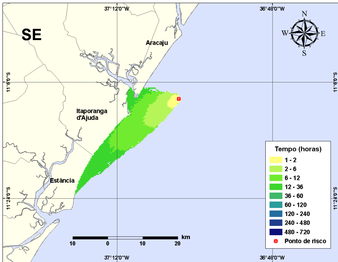
Figura III-14 - Cenário PGA3_VER_8_30D. (Fase: instalação/produção). Contornos de deslocamento de óleo na água para um acidente com óleo tipo GUARICEMA, ocorrendo no Ponto-PGA3, do Campo Guaricema, durante os meses de verão (janeiro a março), com derrame de 8 \text{ m}^3 (instantâneo), após 30 dias de simulação.
