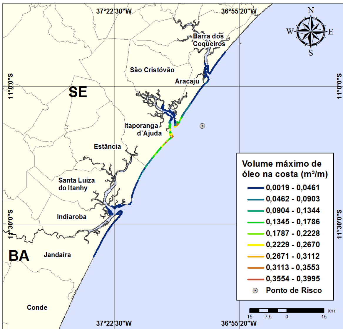
Figura III-112 - Cenário GA07_INV_7500_60D. (Fase: produção). Linhas de volume máximo de óleo na costa para um acidente com óleo tipo GUARICEMA, ocorrendo no Ponto-GA07, do Campo Guaricema, durante os meses de inverno (junho a agosto), com derrame 7.500 m 3 (ao longo de 30 dias), após 60 dias de simulação.
