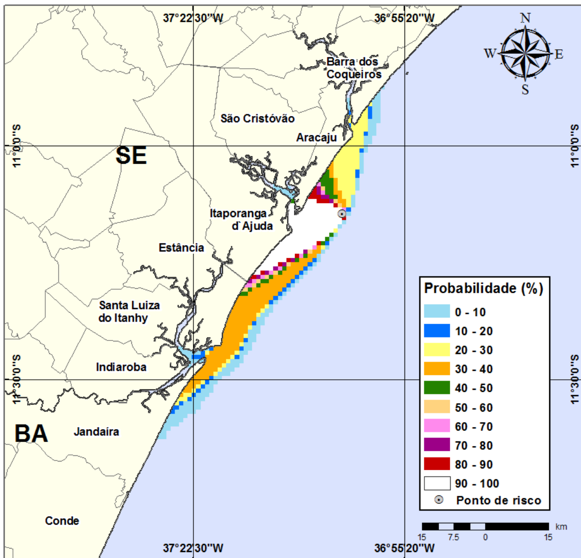
Figura III-109 - Cenário GA07_INV_7500_60D. (Fase: produção). Contornos de probabilidade de óleo na água para um acidente com óleo tipo GUARICEMA, ocorrendo no Ponto-GA07, do Campo Guaricema, durante os meses de inverno (junho a agosto), com derrame de 7.500 m 3 (ao longo de 30 dias), após 60 dias de simulação.
