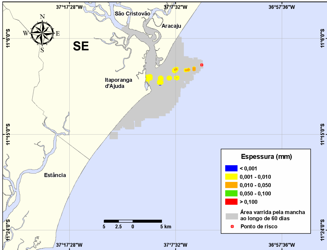
Figura III-123 - DET_PE5_VER_7500_60D. Cenário determinístico crítico para um derrame ocorrido durante o verão com óleo cru, a partir do Ponto PE5 no Campo Guaricema.
