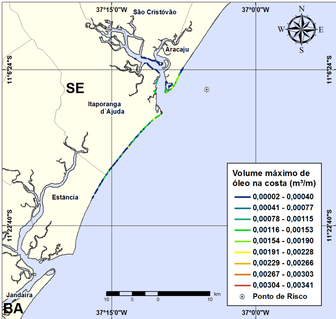
Figura III-40 - Cenário PE5_VER_8_30D (Fase: perfuração). Linhas de volume máximo de óleo na costa para um acidente com óleo tipo GUARICEMA ocorrendo no Ponto-PE5, durante os meses de verão (janeiro a março), com derrame de 8 m 3 (instantâneo), após 30 dias de simulação.
