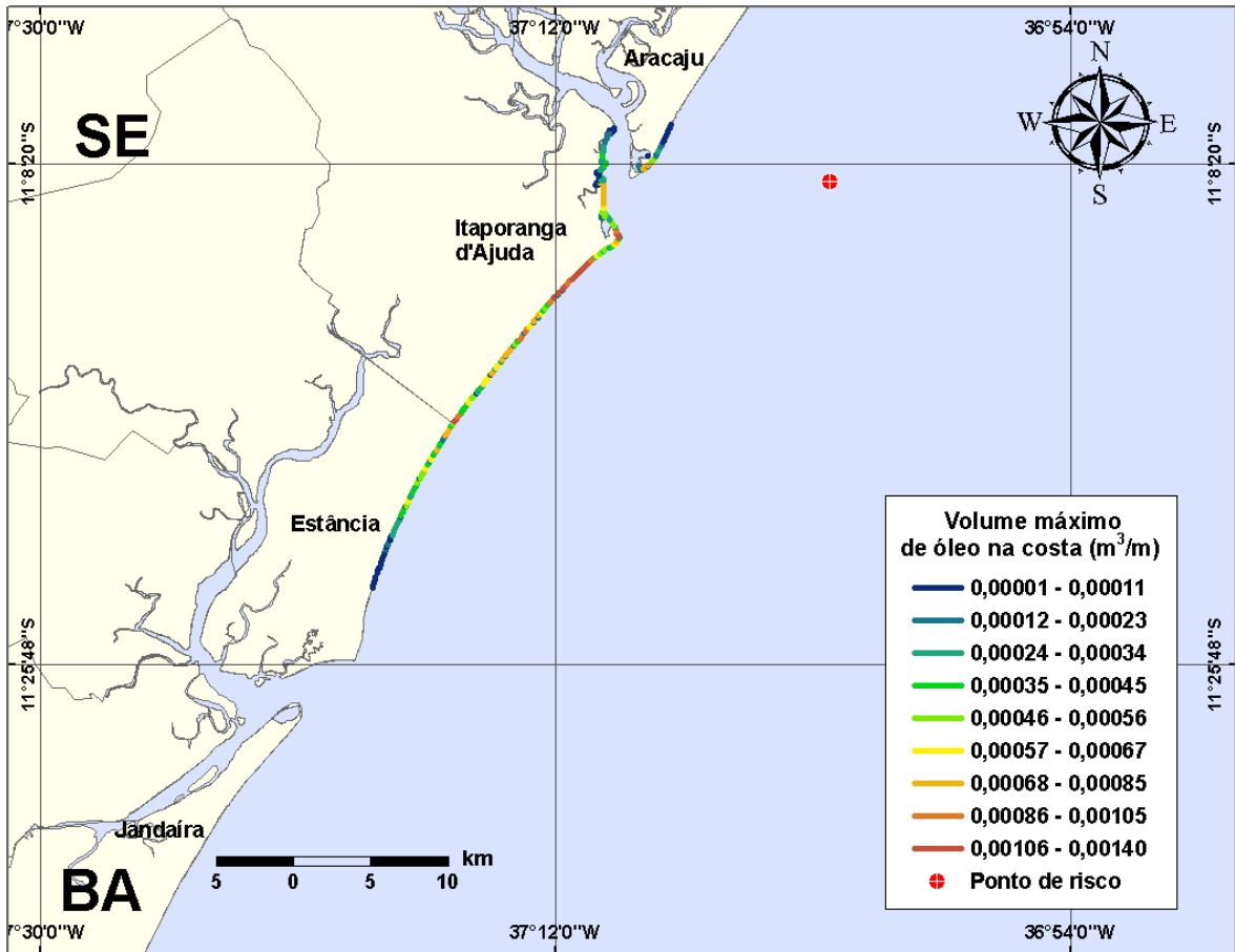
Figura III-4 - Cenário PGA3_DIESEL_VER_8_30D. (Fase: instalação/perfuração). Linhas de volume máximo de óleo na costa para um acidente com óleo tipo DIESEL, ocorrendo no Ponto-PGA3, do Campo Guaricema, durante os meses de verão (janeiro a março), com derrame de 8 m³ (instantâneo), após 30 dias de simulação.
