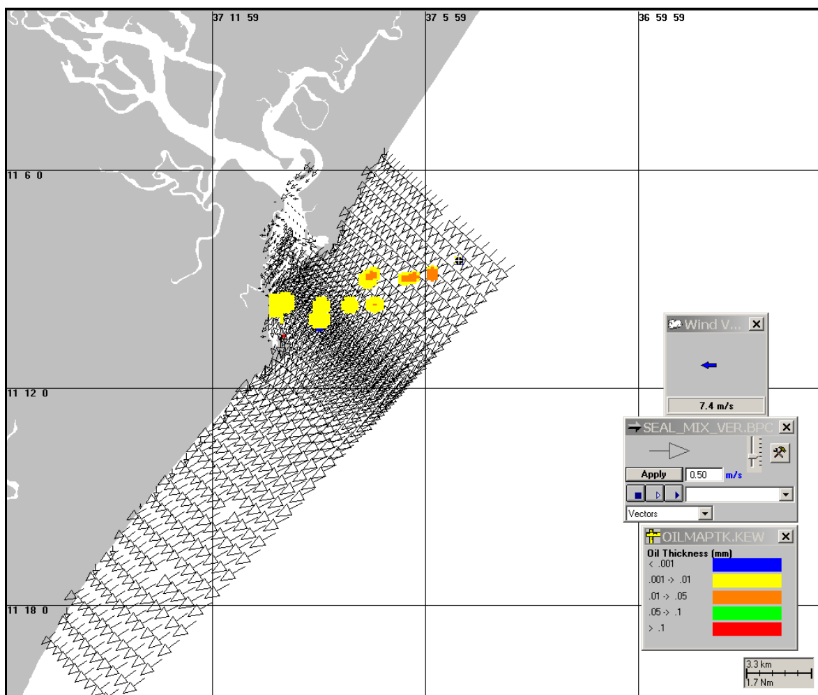
Figura III-127 - Cenário DET_PE5_VER_7500_60D. Condições meteorológicas e oceanográficas e espessuras da mancha de óleo no instante de primeiro toque na costa da simulação.
