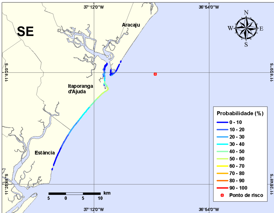
Figura III-19 - Cenário PGA3_VER_200_30D. (Fase: instalação/produção). Linhas de probabilidade de óleo na costa para um acidente com óleo tipo GUARICEMA, ocorrendo no Ponto-PGA3, do Campo Guaricema, durante os meses de verão (janeiro a março), com derrame de 200 m 3 (instantâneo), após 30 dias de simulação.
