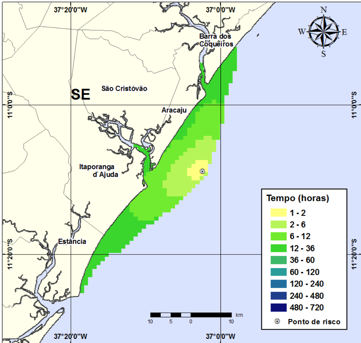
Figura III-82 - Cenário PGA3_INV_264_30D. (Fase: produção). Contornos de deslocamento de óleo na água para um acidente com óleo tipo GUARICEMA, ocorrendo no Ponto-PGA3, do Campo Guaricema, durante os meses de inverno (junho a agosto), com derrame de 264 m 3 (instantâneo), após 30 dias de simulação.
