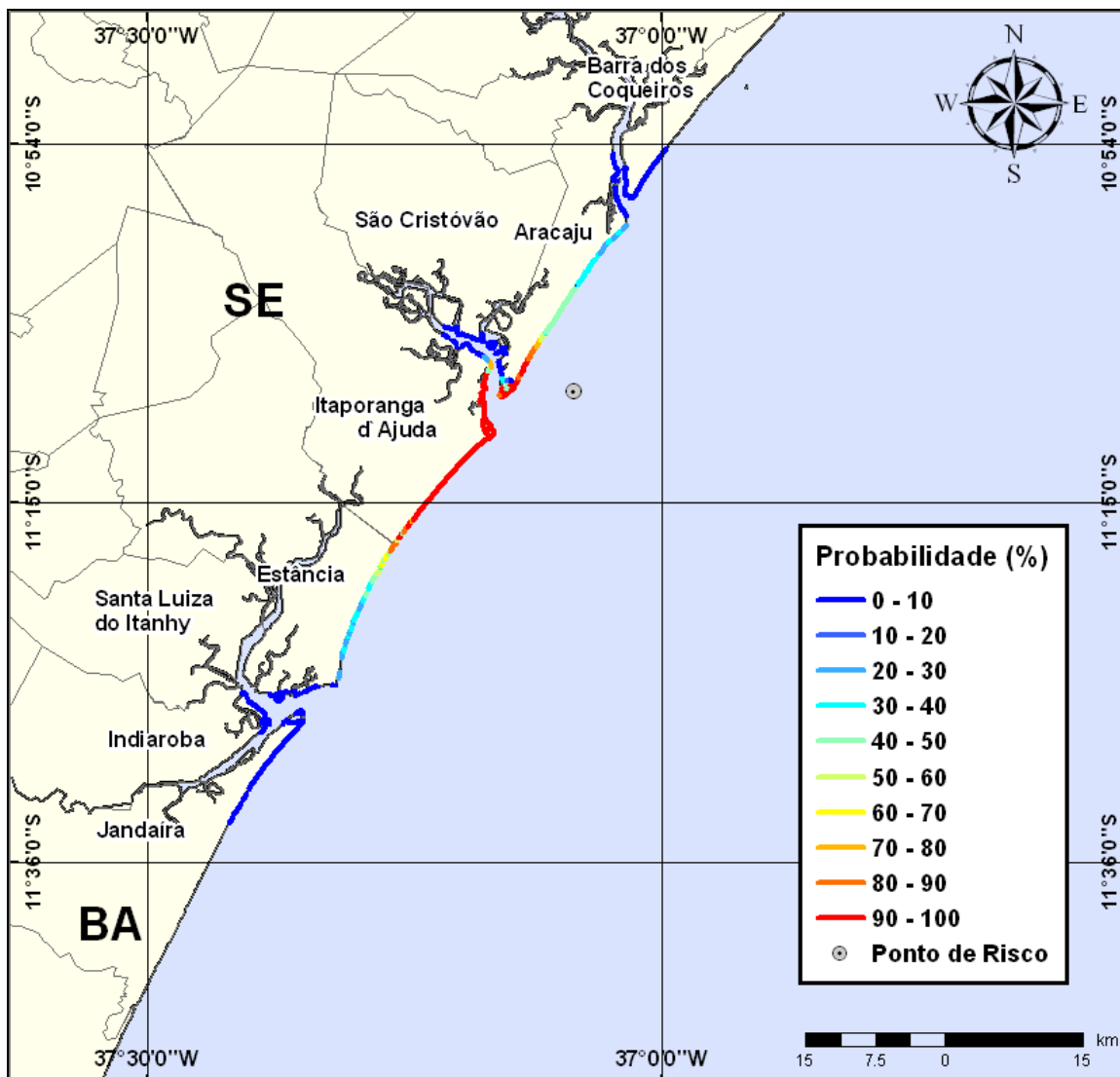
Figura III-107 - Cenário PE5_INV_7500_60D (Fase: perfuração). Linhas de probabilidade de óleo na costa para um acidente ocorrendo com óleo tipo GUARICEMA no Ponto-PE5, durante os meses de inverno (junho a agosto), com derrame de 7.500 m 3 (ao longo de 30 dias), após 60 dias de simulação.
