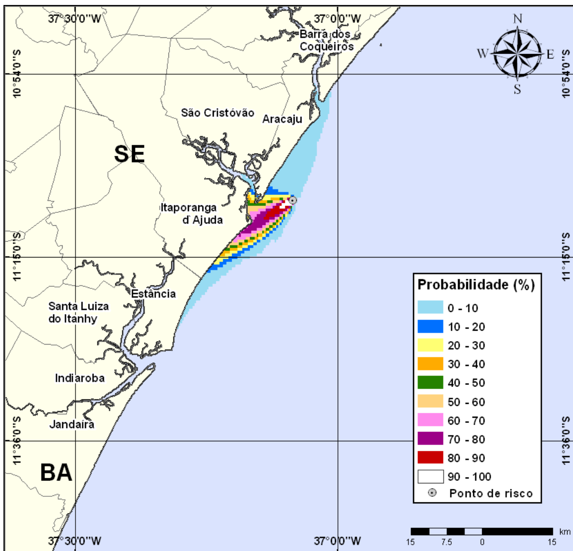
Figura III-97 - Cenário PE5_INV_8_30D (Fase: perfuração). Contornos de probabilidade de óleo na água para um acidente com óleo tipo GUARICEMA ocorrendo no Ponto-PE5, durante os meses de inverno (junho a agosto), com derrame de 8 m 3 (instantâneo), após 30 dias de simulação.
