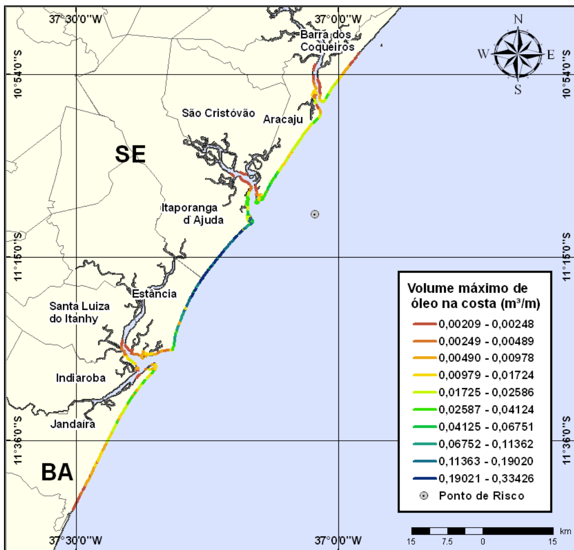
Figura III-96 - Cenário PGA10_INV_7500_60D (Fase: perfuração). Linhas de volume máximo de óleo na costa para um acidente com óleo tipo GUARICEMA ocorrendo no Ponto-PGA10, durante os meses de inverno (junho a agosto), com derrame de 7.500 m 3 (ao longo de 30 dias), após 60 dias de simulação.
