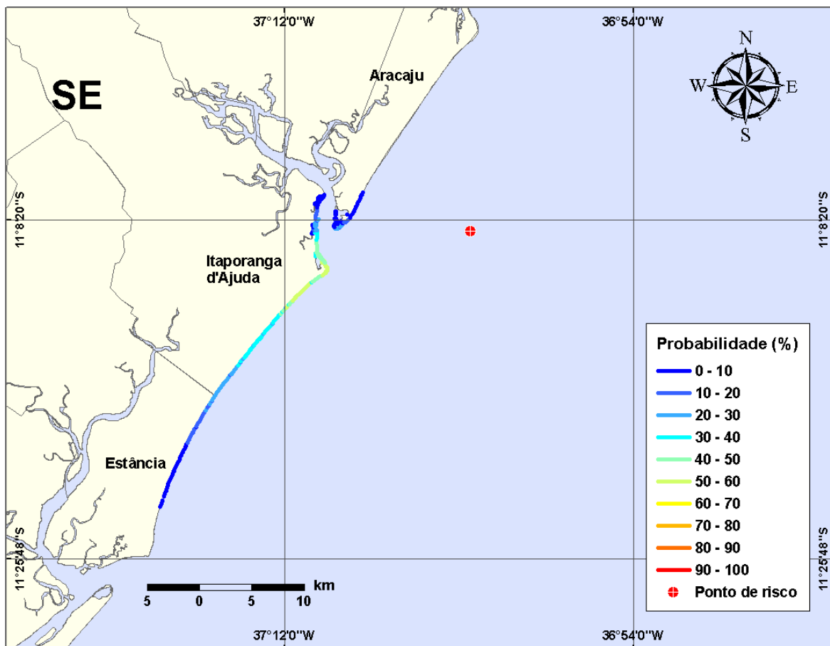
Figura III-3 - Cenário PGA3_DIESEL_VER_8_30D. (Fase: instalação/perfuração). Linhas de probabilidade de óleo na costa para um acidente com óleo tipo DIESEL, ocorrendo no Ponto-PGA3, do Campo Guaricema, durante os meses de verão (janeiro a março), com derrame de 8 m 3 (instantâneo), após 30 dias de simulação.
