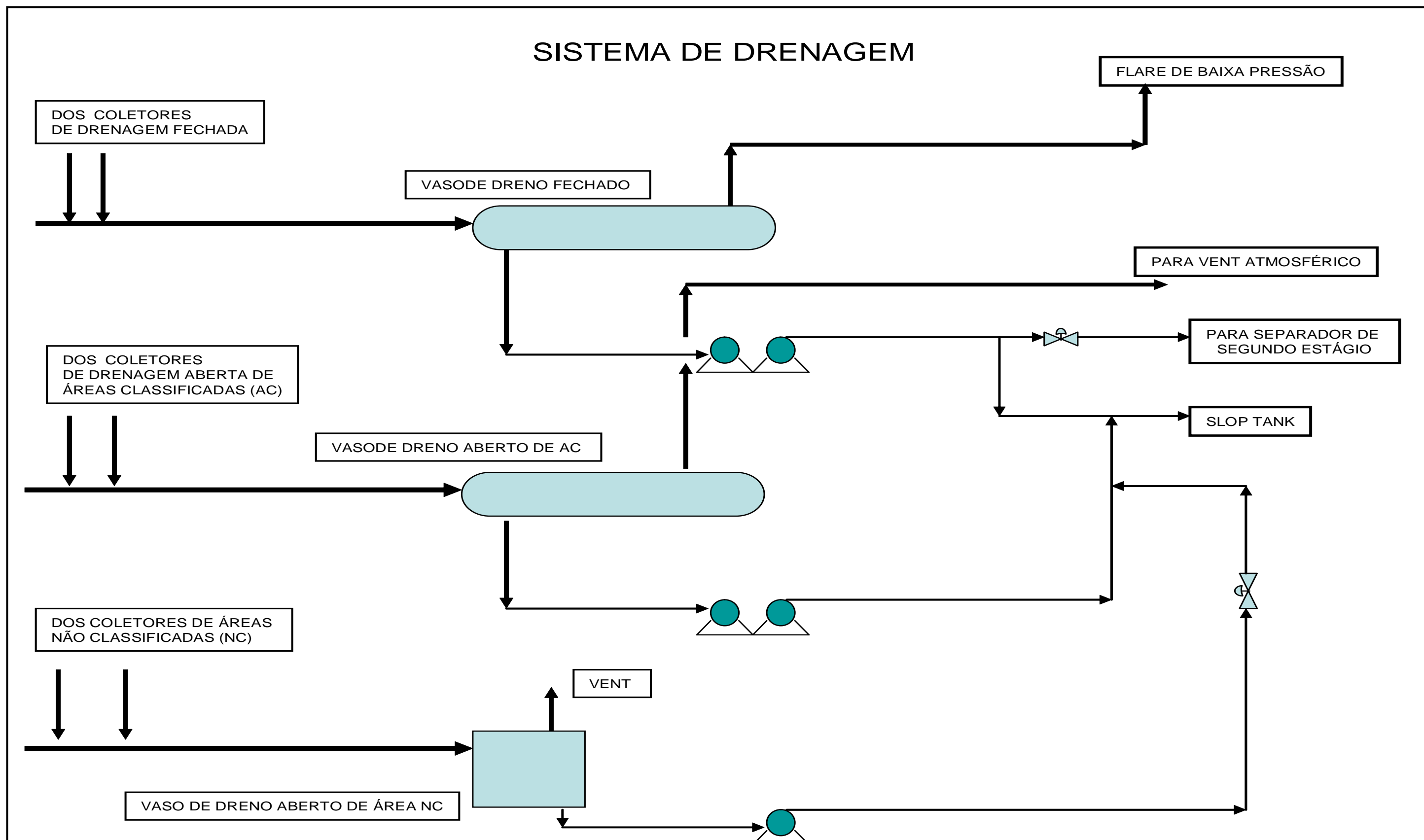
Figura 2.4-19. Diagrama esquemático do sistema de drenagem. Fonte: OGX
