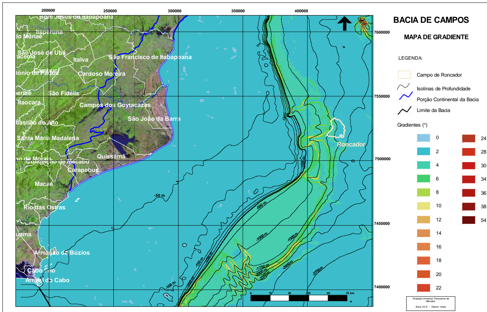
Figura 5.1.5.3-3. Mapa de Gradiente da Bacia de Campos
