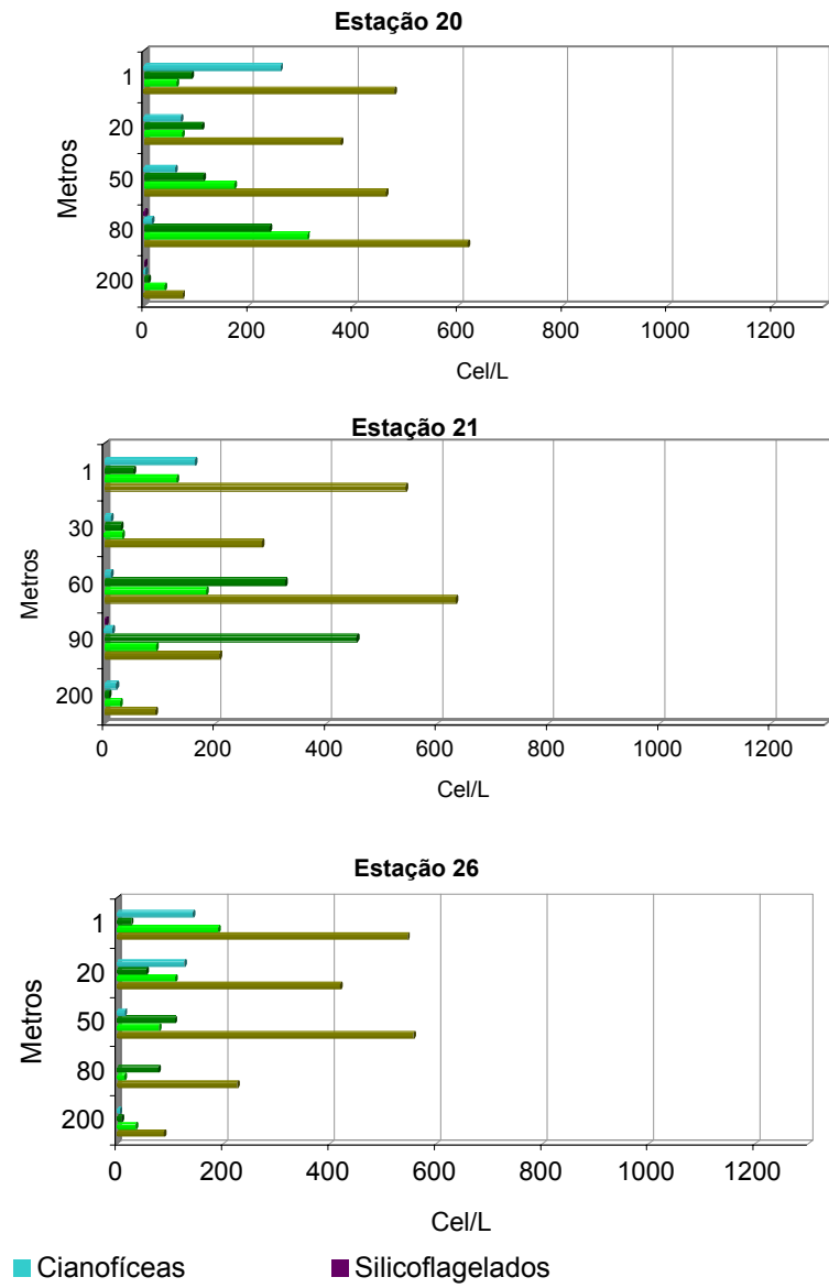
Figura 5.2-15. Densidade dos grupos do microfitoplâncton por profundidade em cada estação de coleta da caracterização de Albacora Leste.
