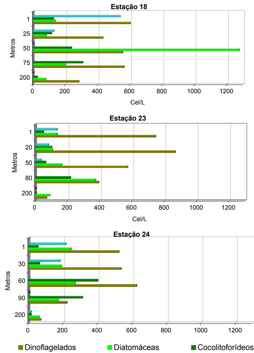
Figura 5.2-15. Densidade dos grupos do microfitoplâncton por profundidade em cada estação de coleta da caracterização de Albacora Leste.
