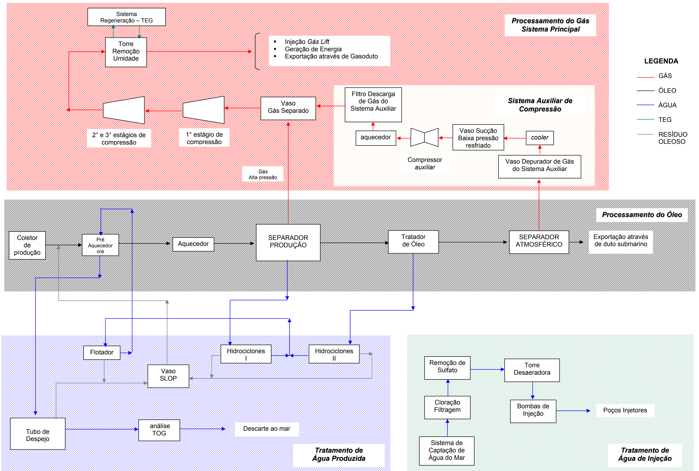
Figura 2.4-6 Fluxograma Simplificado de Processo UEP P-52
