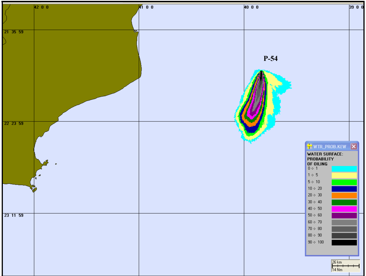
Figura 15 – Cenário P54 VER PIORCASO 36HORAS. Contorno de probabilidades para um acidente ocorrendo no FPSO P-54 durante os meses de verão (Janeiro a março) com derrame de 335.208m 3 após 36 horas.
