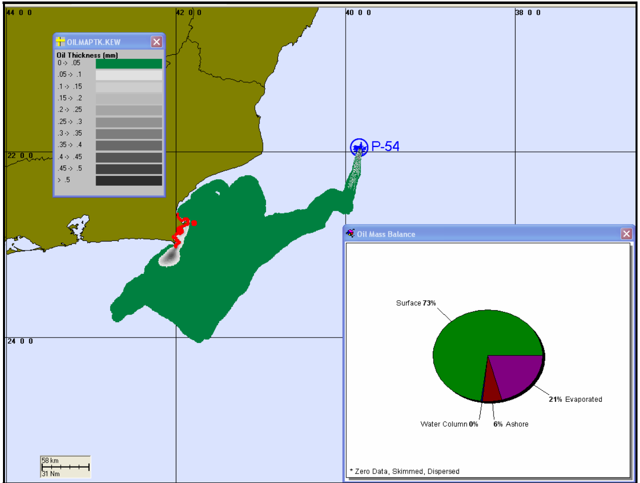
Figura 24 – Cenário de pior caso de vazamento no inverno para o FPSO P-54
