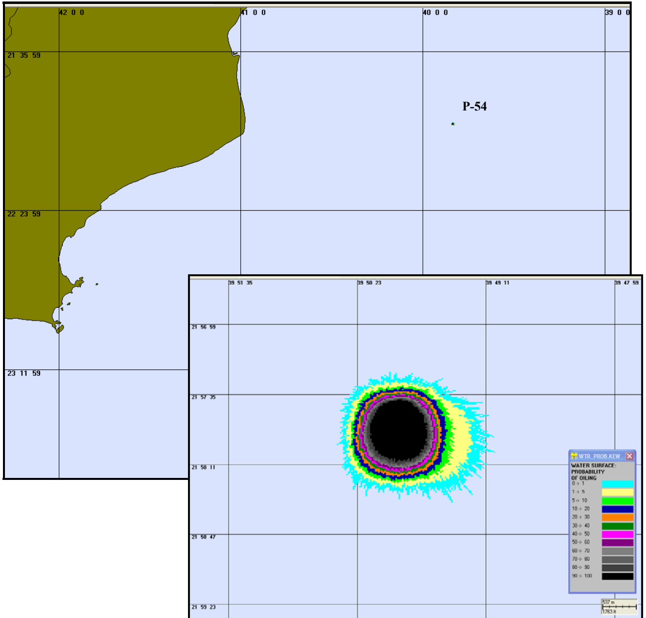
Figura 3 – Cenário P54 VER 8 20PPM . Contorno de probabilidades para um acidente ocorrendo no FPSO P-54 durante os meses de verão (Janeiro a Março) com derrame de 8\text{m}^3 após 1 hora atingindo 20ppm.
