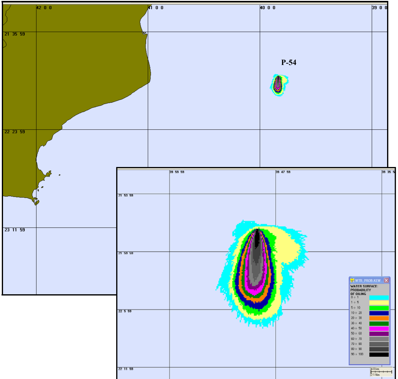
Figura 7 – Cenário P54 VER 200 9HORAS. Contorno de probabilidades para um acidente ocorrendo no FPSO P-54 durante os meses de verão (Janeiro a março) com derrame de 200m 3 após 9 horas.
