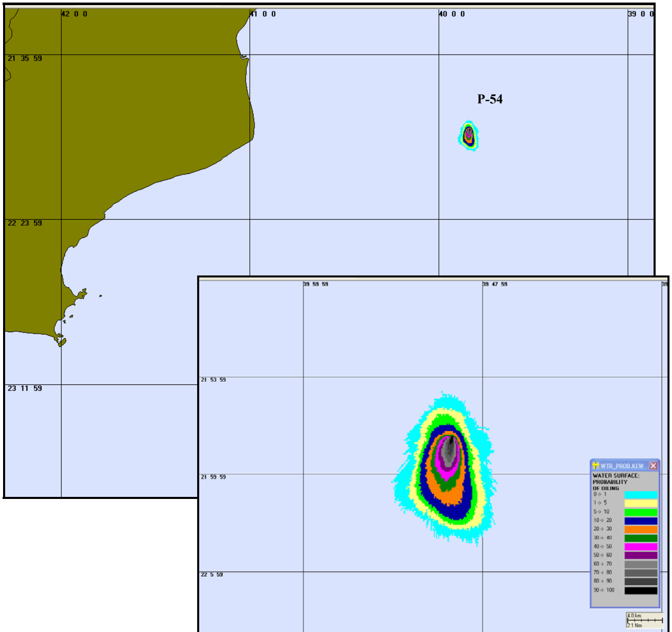
Figura 6 – Cenário P54 INV 200 6HORAS. Contorno de probabilidades para um acidente ocorrendo no FPSO P-54 durante os meses de inverno (Junho a Agosto) com derrame de 200m 3 após 6 horas.
