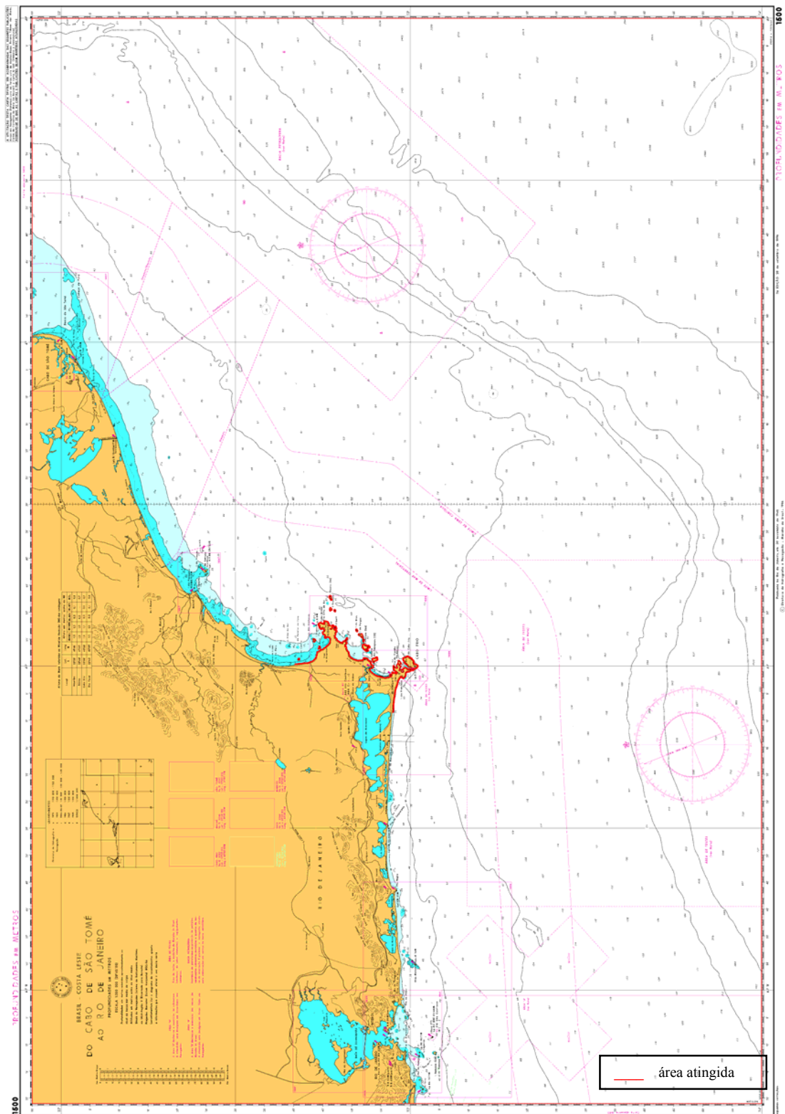
Figura 22 – Cenário P54 INV_PIORCASO_30DIAS. Área total (b) de toque na linha de costa para um acidente ocorrendo durante os meses de inverno (Junho a Agosto).
