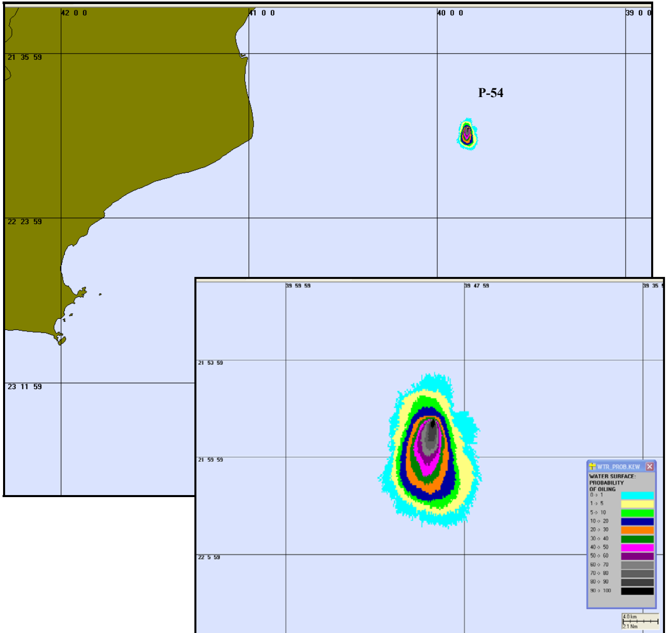
Figura 10 – Cenário P54_INV_PIORCASO_6HORAS. Contorno de probabilidades para um acidente ocorrendo no FPSO P-54 durante os meses de inverno (Junho a Agosto) com derrame de 335.208m 3 após 6 horas.
