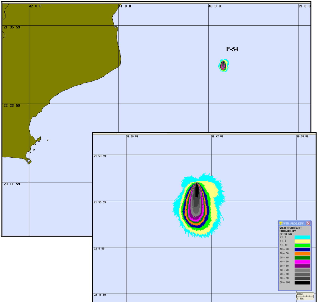
Figura 9 – Cenário P54 VER PIORCASO 6HORAS. Contorno de probabilidades para um acidente ocorrendo no FPSO P-54 durante os meses de verão (Janeiro a março) com derrame de 335.208m 3 após 6 horas.
