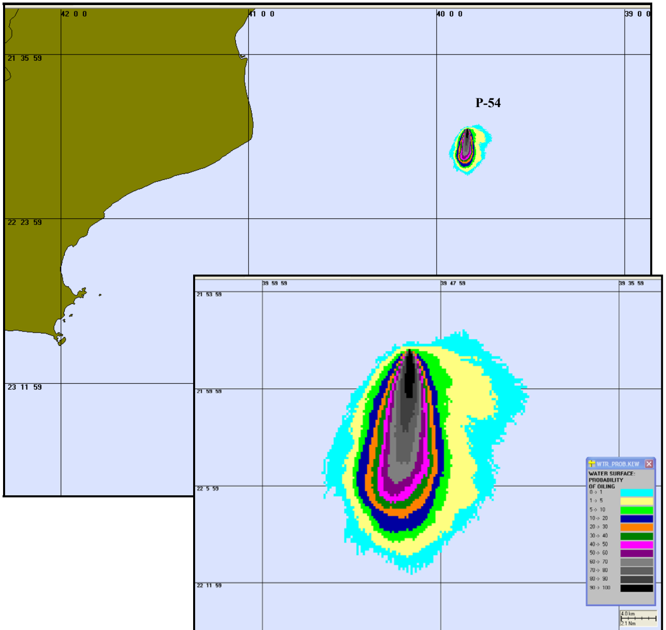
Figura 13 – Cenário P54 VER PIORCASO 12HORAS. Contorno de probabilidades para um acidente ocorrendo no FPSO P-54 durante os meses de verão (Janeiro a março) com derrame de 335.208m 3 após 12 horas.
