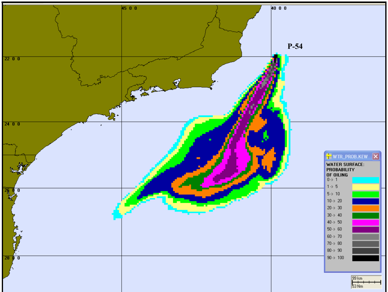
Figura 19 – Cenário P54 VER PIORCASO 30DIAS. Contorno de probabilidades para um acidente ocorrendo no FPSO P-54 durante os meses de verão (Janeiro a março) com derrame de 335.208\text{m}^3 após 30 dias.
