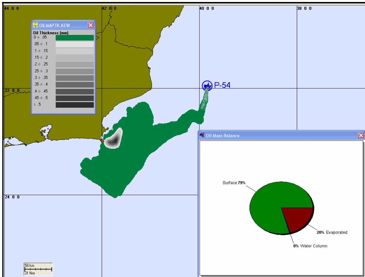
Figura 25 – Instante do primeiro toque na costa para o cenário de pior caso de vazamento no inverno para o FPSO P-54.
