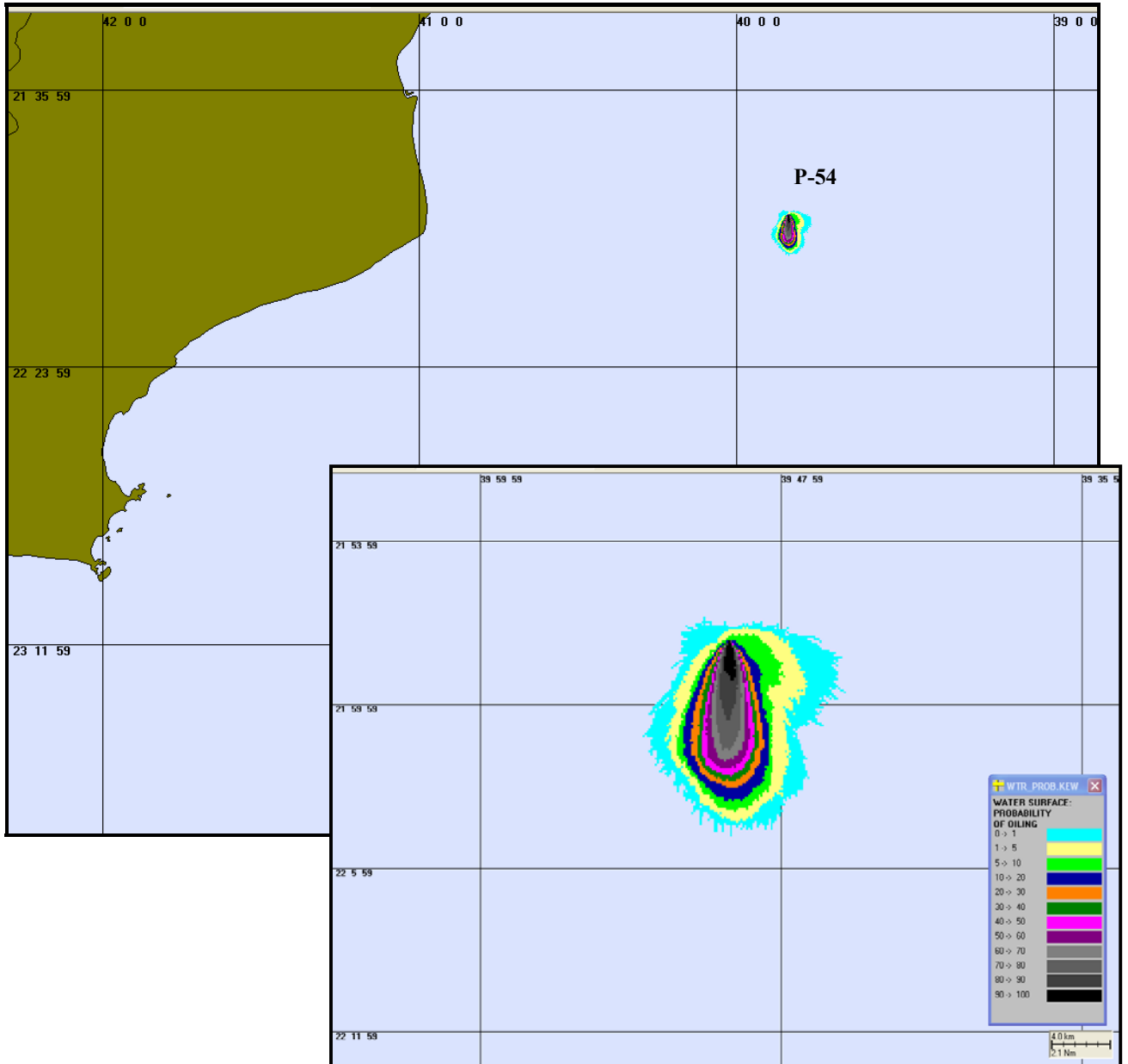
Figura 5 – Cenário P54 VER 200 6HORAS. Contorno de probabilidades para um acidente ocorrendo no FPSO P-54 durante os meses de verão (Janeiro a Março) com derrame de 200m 3 após 6 horas.
