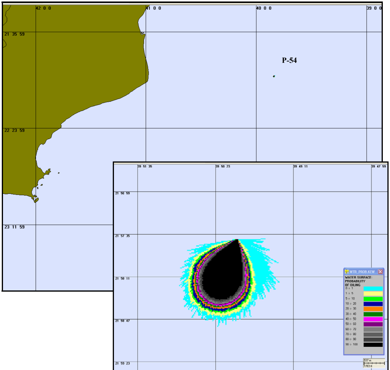
Figura 4 – Cenário P54 INV 8 20PPM. Contorno de probabilidades para um acidente ocorrendo no FPSO P-54 durante os meses de inverno (Junho a Agosto) com derrame de 8m 3 após 1 hora atingindo 20ppm.
