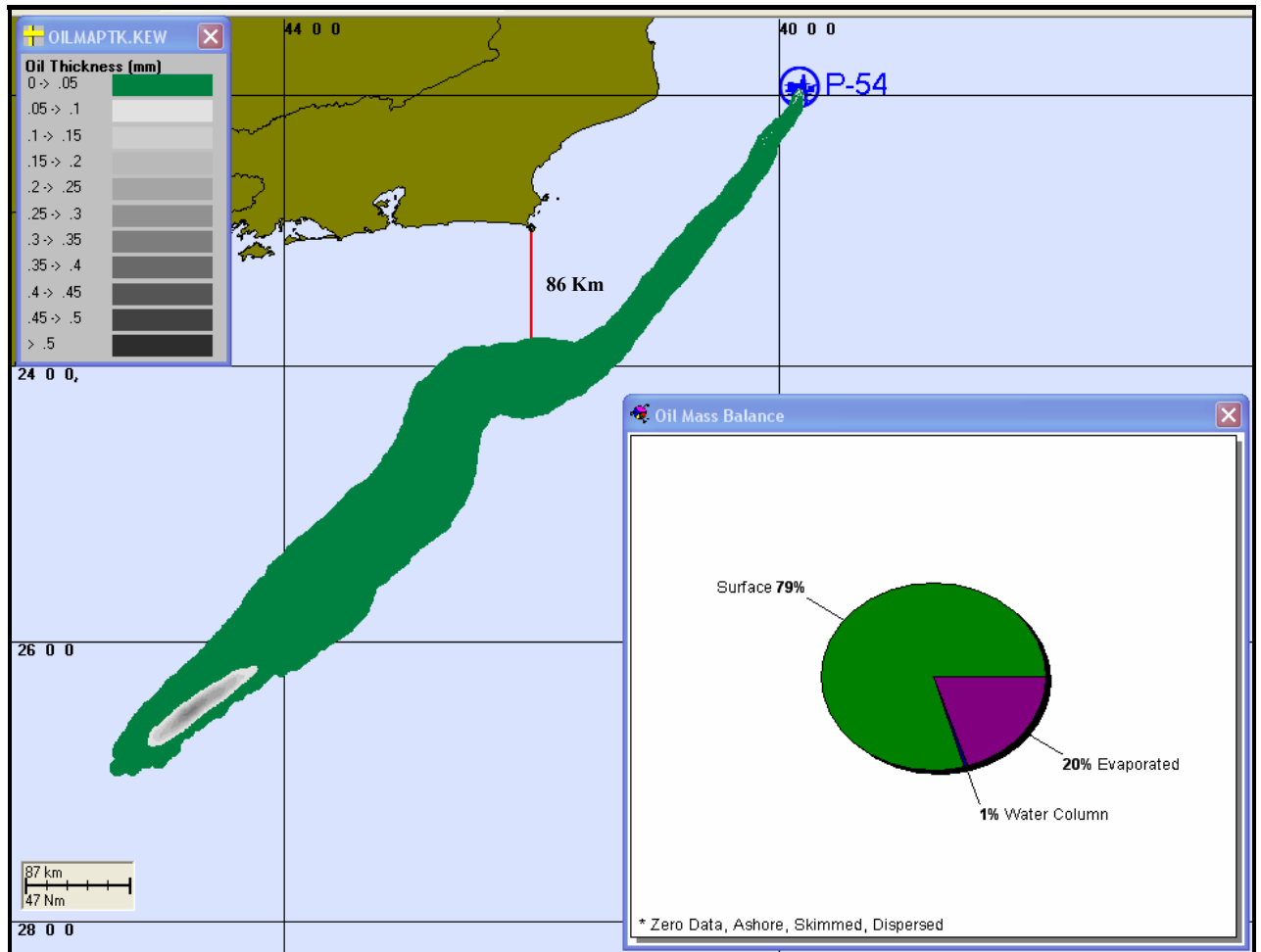
Figura 26 – Cenário de pior caso de vazamento no verão para o FPSO P-54
