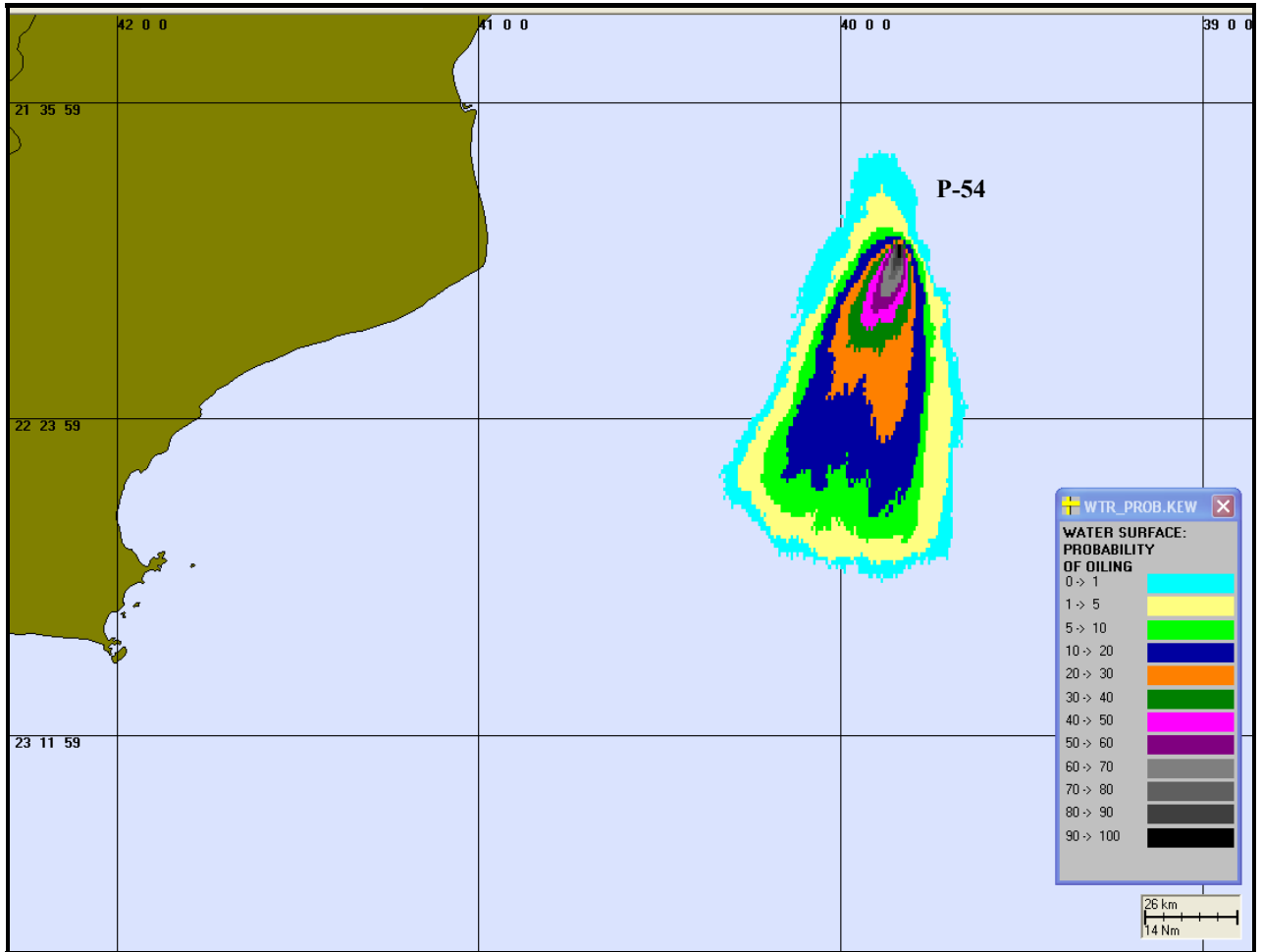
Figura 18 – Cenário P54 INV PIORCASO 60HORAS . Contorno de probabilidades para um acidente ocorrendo no FPSO P-54 durante os meses de inverno (Junho a Agosto) com derrame de 335.208m 3 após 60 horas.
