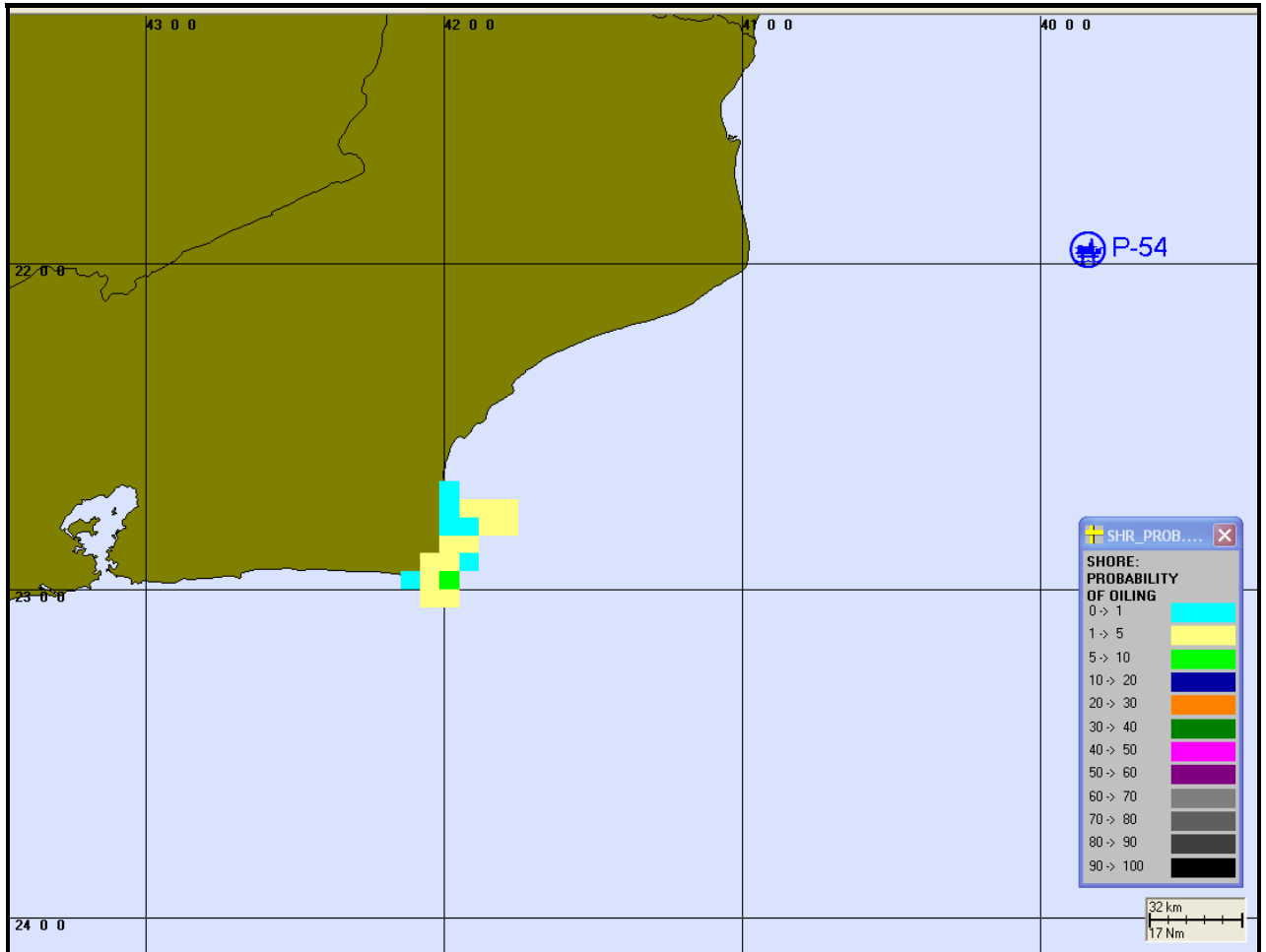
Figura 21 – Cenário P54 INV PIORCASO 30DIAS. Contornos de probabilidade de toque na linha de costa para um acidente ocorrendo durante os meses de inverno (Junho a Agosto).
