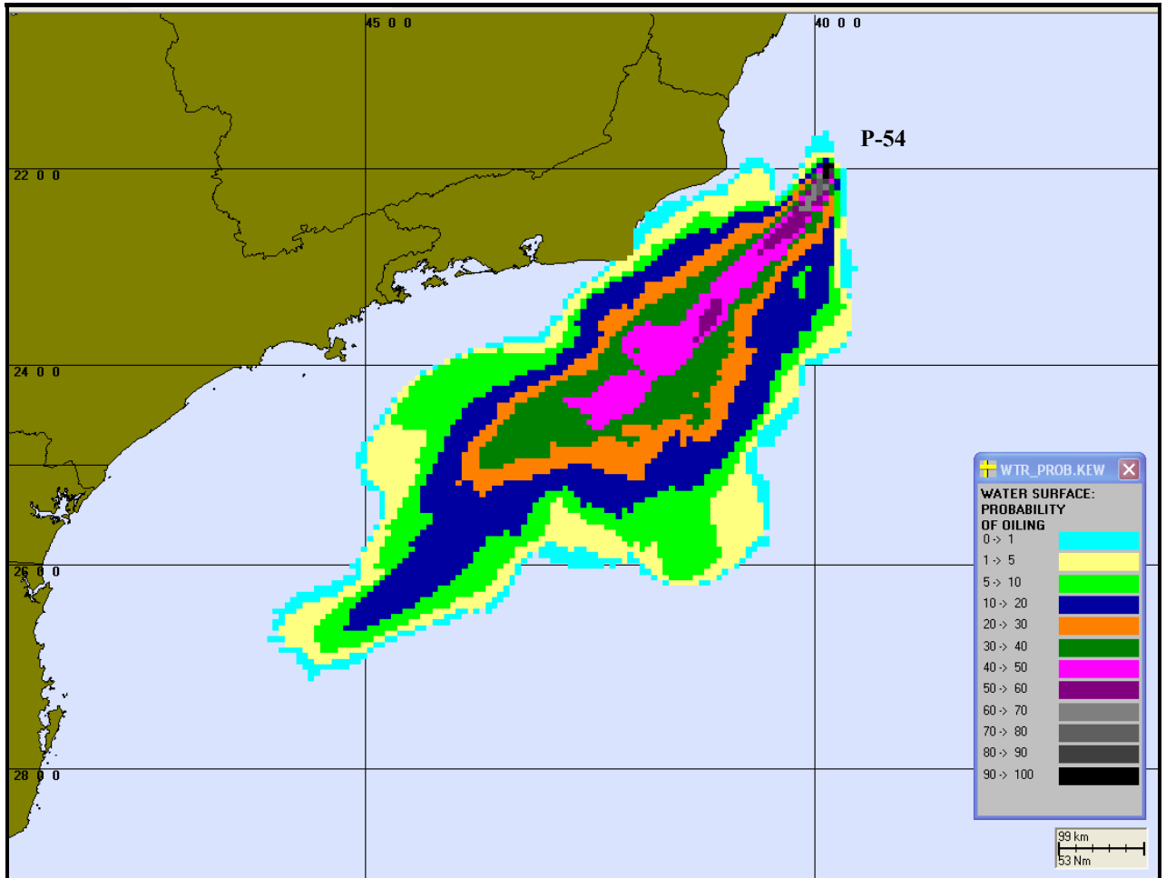
Figura 20 – Cenário P54 INV PIORCASO 30DIAS. Contorno de probabilidades para um acidente ocorrendo no FPSO P-54 durante os meses de inverno (Junho a Agosto) com derrame de 335.208\text{m}^3 após 30 dias.
