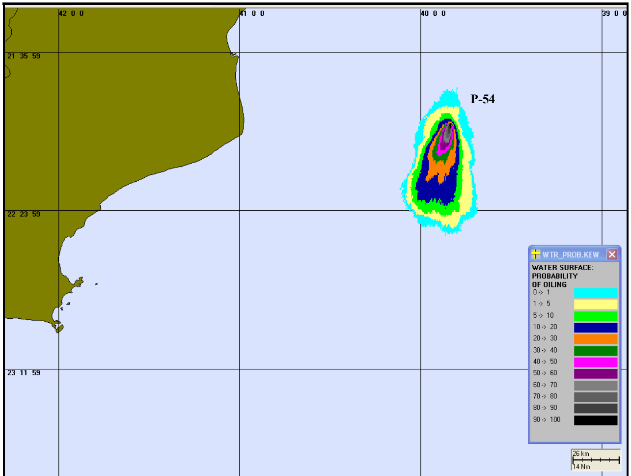
Figura 16 – Cenário P54 INV PIORCASO 36HORAS . Contorno de probabilidades para um acidente ocorrendo no FPSO P-54 durante os meses de inverno (Junho a Agosto) com derrame de 335.208m 3 após 36 horas.
