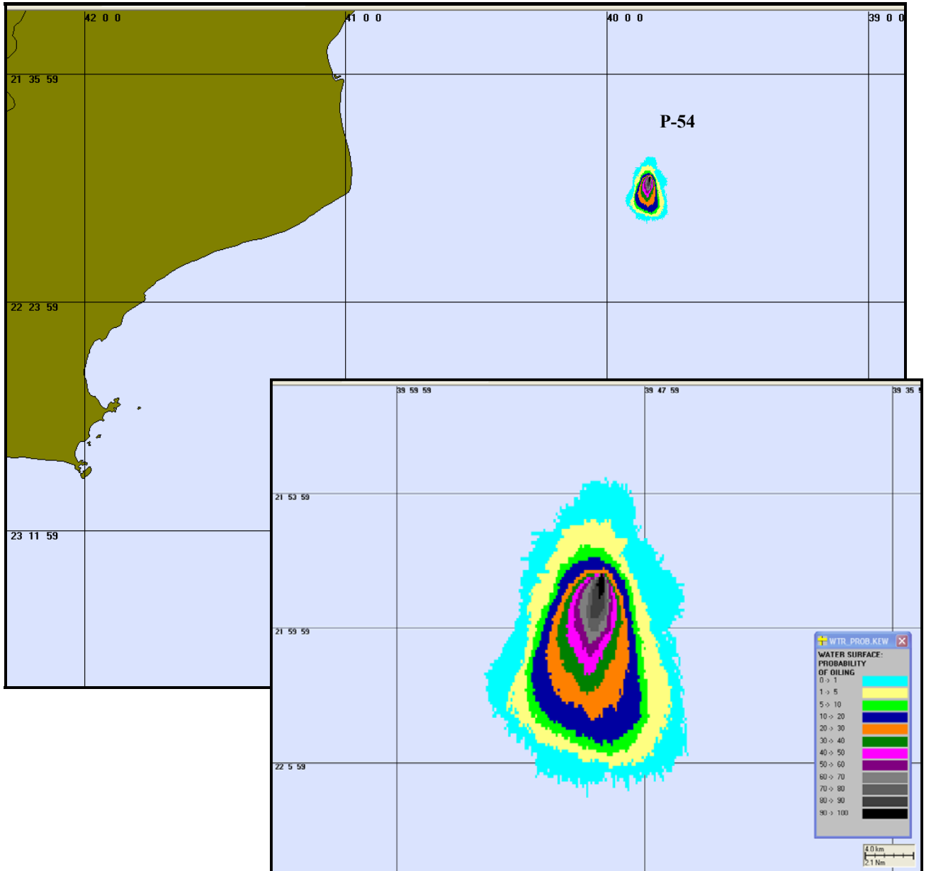
Figura 12 – Cenário P54 INV PIORCASO 9HORAS. Contorno de probabilidades para um acidente ocorrendo no FPSO P-54 durante os meses de inverno (Junho a Agosto) com derrame de 335.208m 3 após 9 horas.
