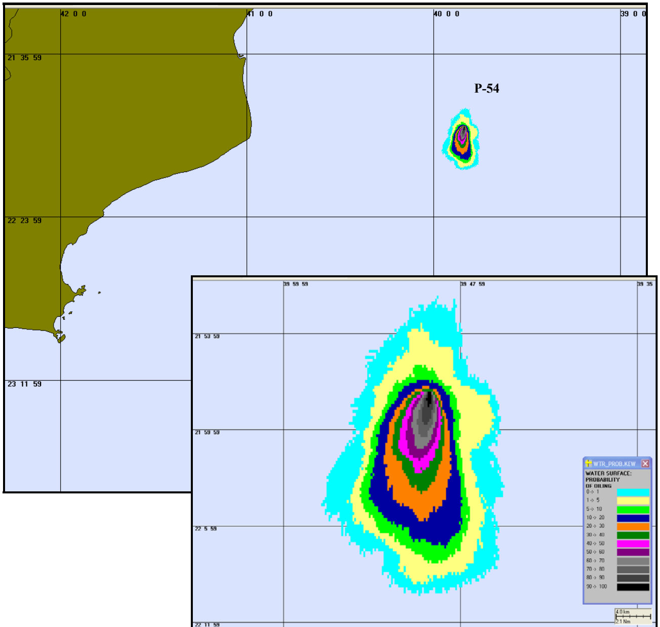
Figura 14 – Cenário P54 INV PIORCASO 12HORAS. Contorno de probabilidades para um acidente ocorrendo no FPSO P-54 durante os meses de inverno (Junho a Agosto) com derrame de 335.208m 3 após 12 horas.
