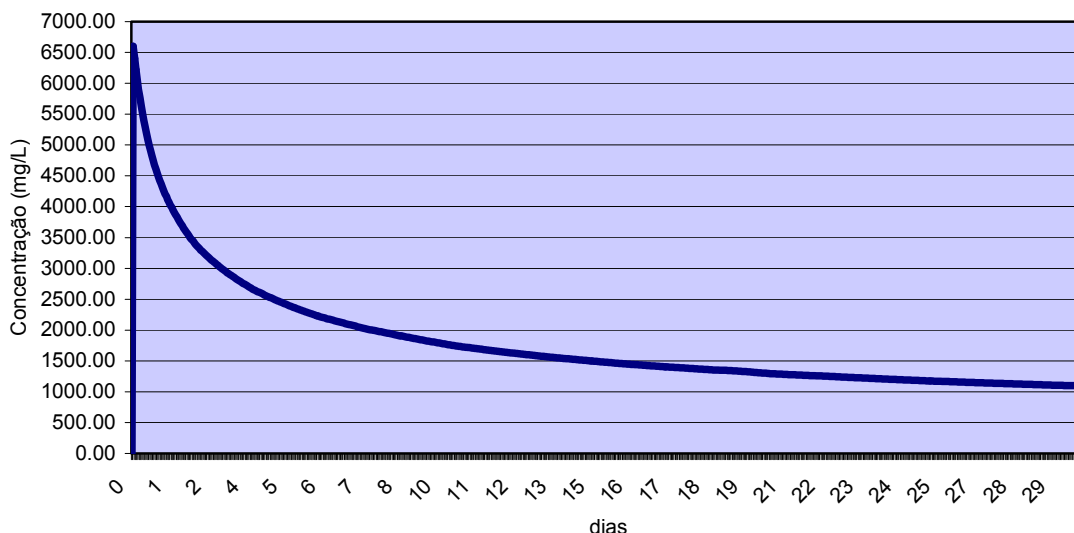
Figura 23 – Evolução temporal da pseudo-concentração da mancha para o cenário P54 INV PIORCASO 30DIAS .
