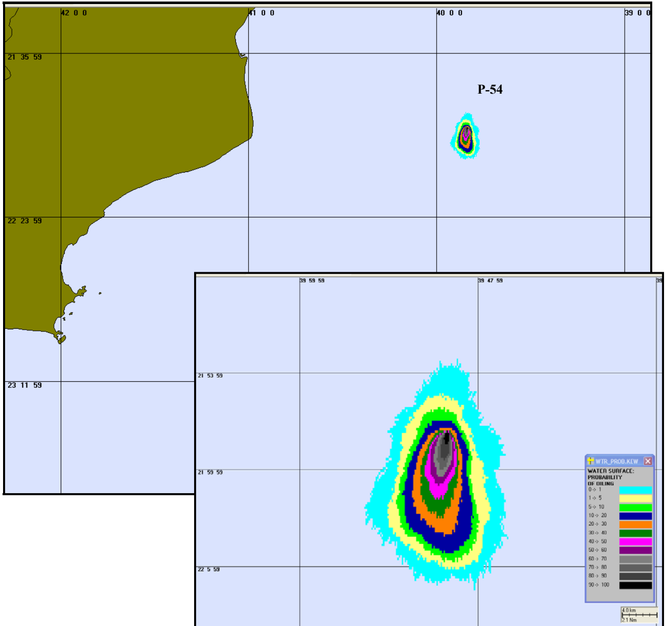
Figura 8 – Cenário P54 INV 200 9HORAS. Contorno de probabilidades para um acidente ocorrendo no FPSO P-54 durante os meses de inverno (Junho a Agosto) com derrame de 200m 3 após 9 horas.
