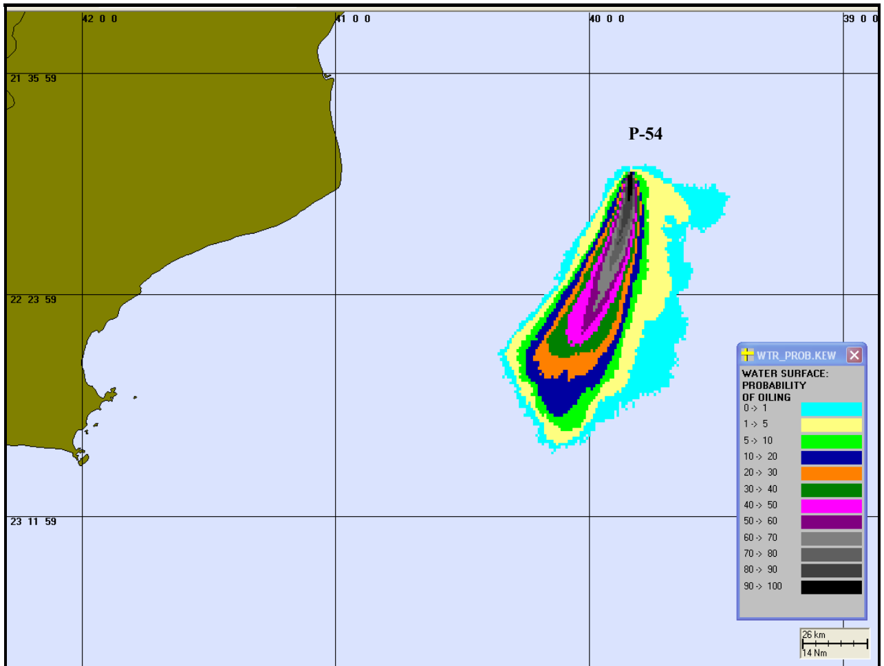
Figura 17 – Cenário P54 VER PIORCASO 60HORAS. Contorno de probabilidades para um acidente ocorrendo no FPSO P-54 durante os meses de verão (Janeiro a março) com derrame de 335.208m 3 após 60 horas.
