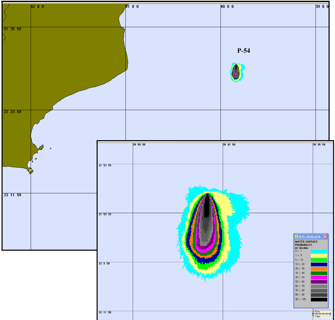
Figura 11 – Cenário P54 VER PIORCASO 9HORAS. Contorno de probabilidades para um acidente ocorrendo no FPSO P-54 durante os meses de verão (Janeiro a março) com derrame de 335.208m 3 após 9 horas.
