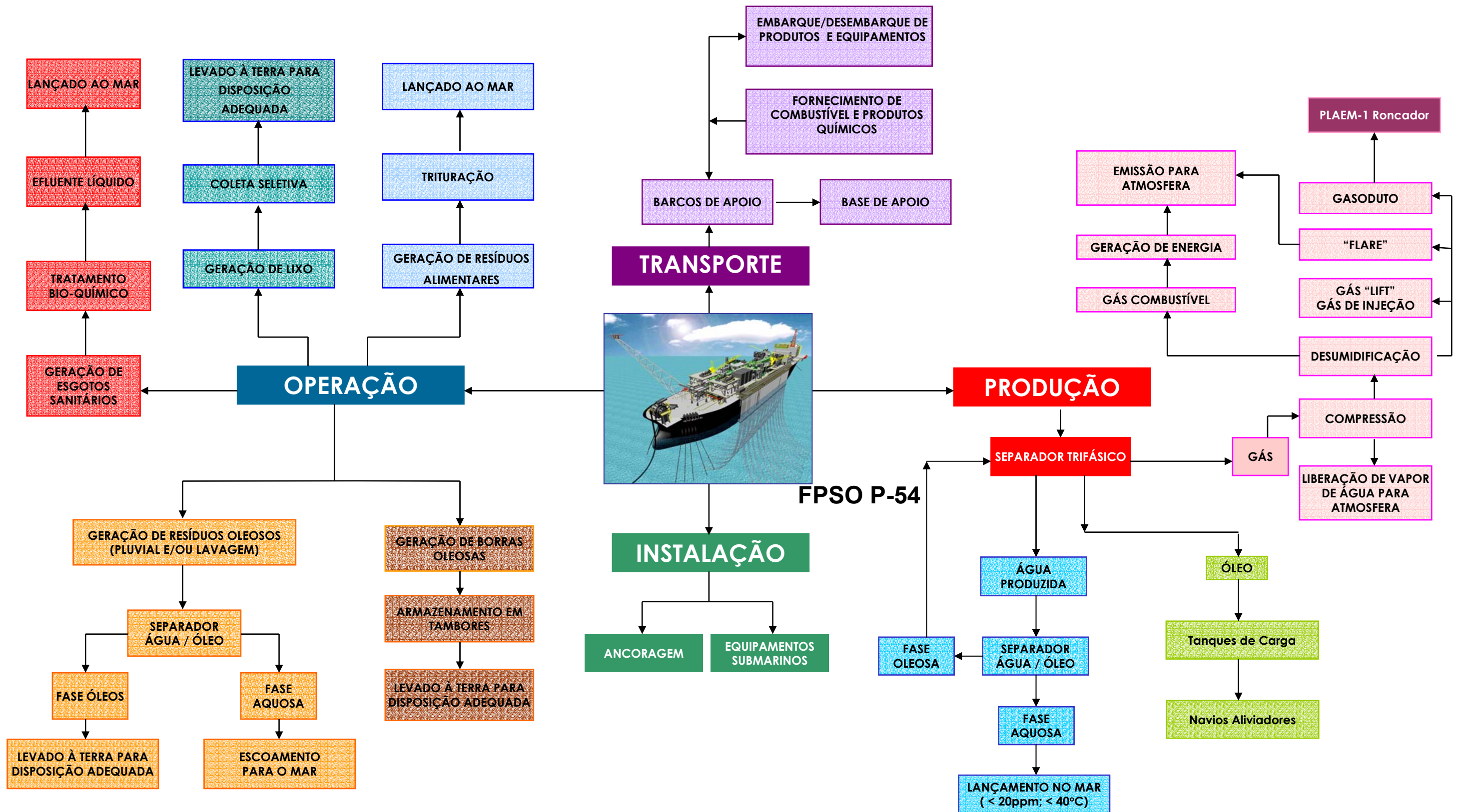
Figura 6.1.2-1. Fluxograma do processo de interesse ambiental
