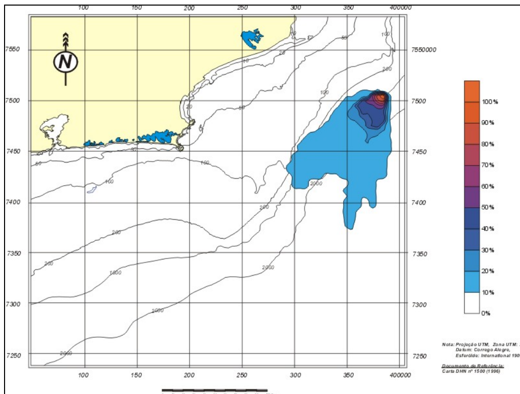
Figura 4-2: Probabilidade de toque de um volume derramado de óleo de 46.000 m 3 na coordenada X=384.591 e Y=7.504.979 com condições de vento forte e maré de enchente.
