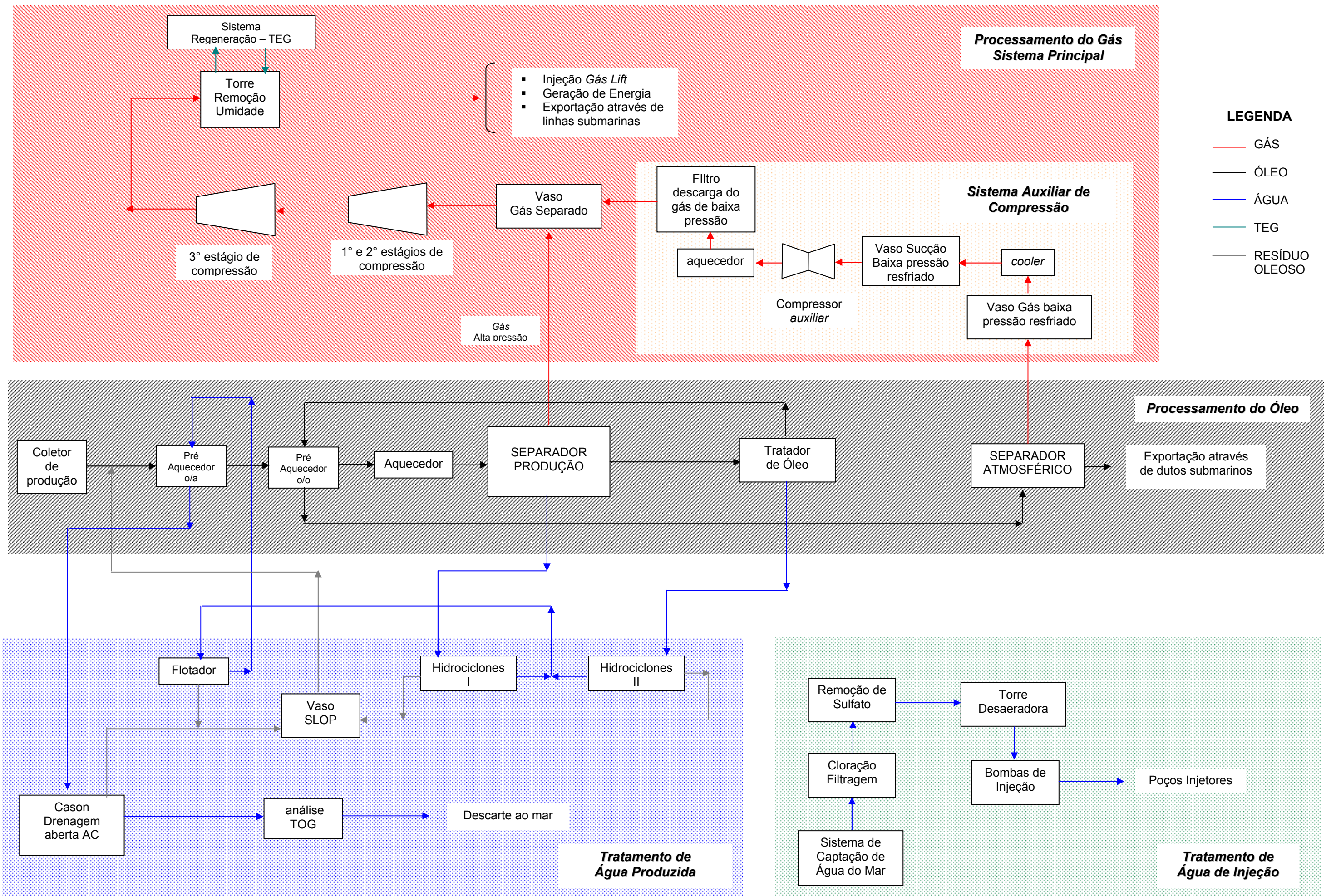
Figura 2.4-2 Fluxograma Simplificado dos Processos de Produção da UEP P-51
