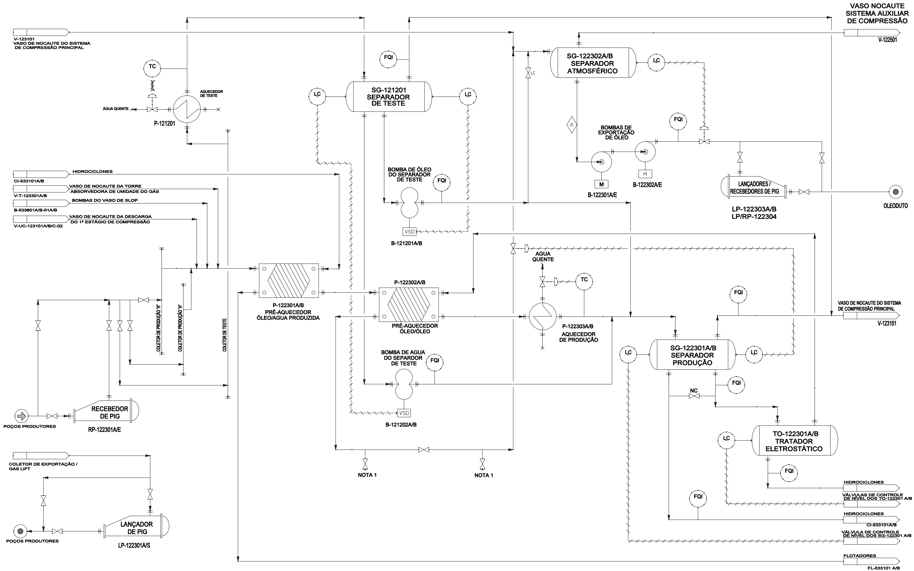
Figura 2.4-3 - Fluxograma Simplificado da Planta de Processamento de Óleo
