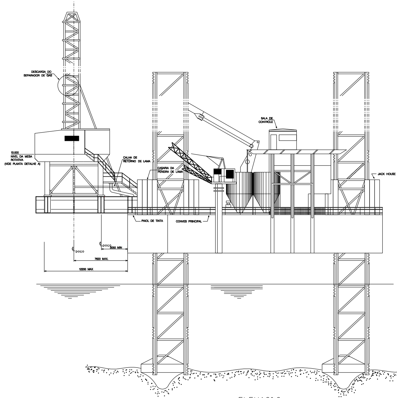
ELEVAÇÃO
