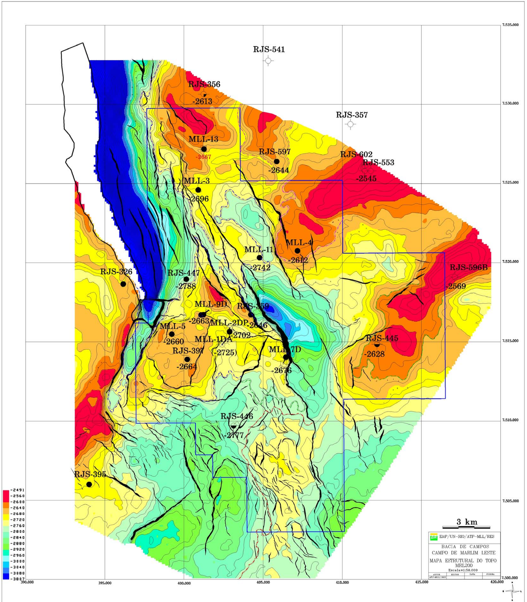
Figura II.5.1.5-8 – Mapa estrutural do topo do reservatório oligomiocênico
