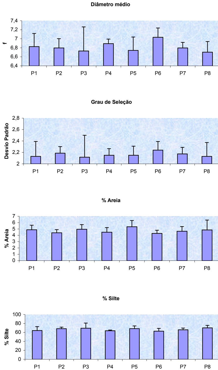
Figura 5.1.5-a. Granulometria do sedimento coletado durante a 1a Campanha do
