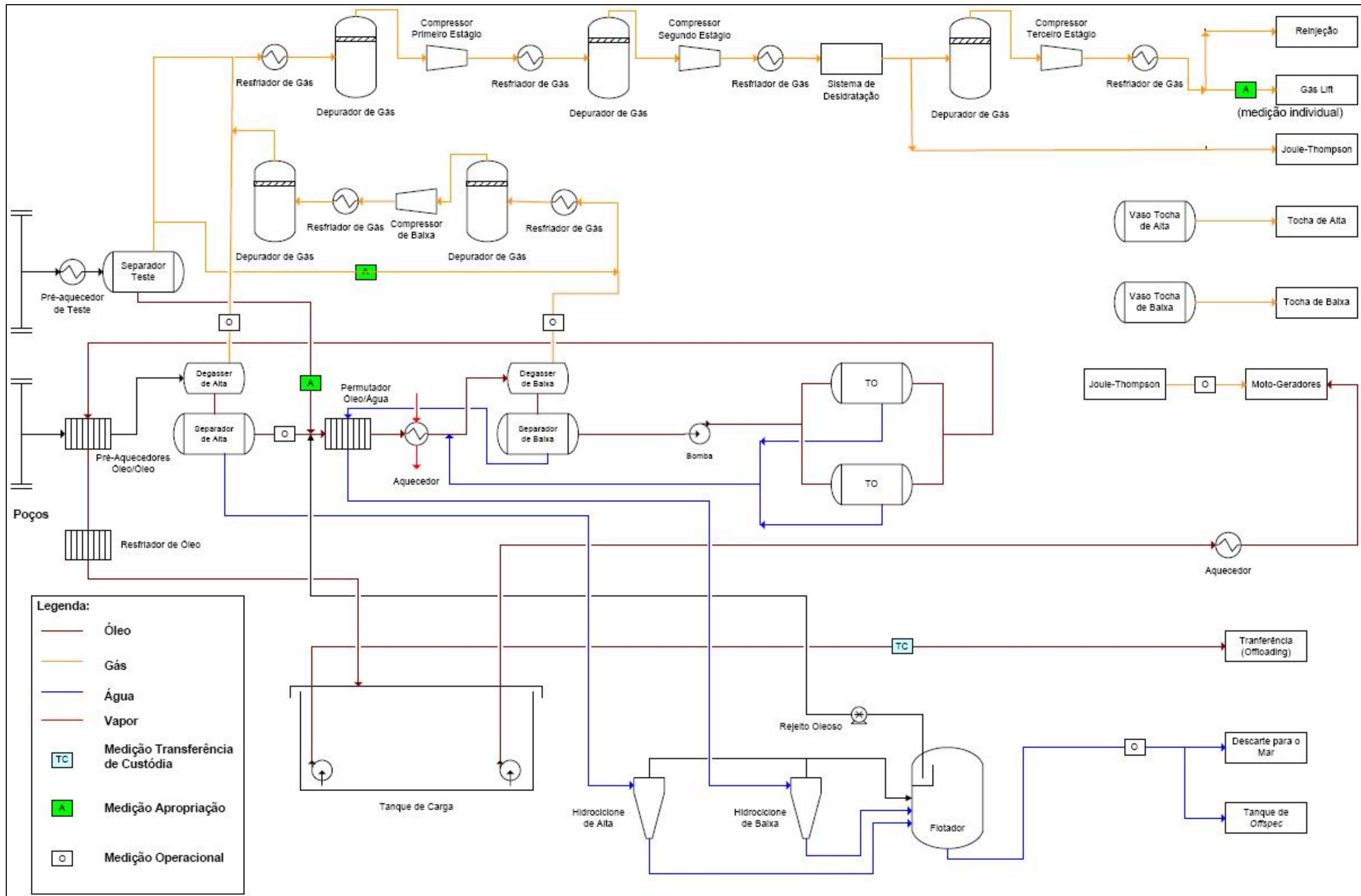
Figura II.2.4-13 - Fluxograma de processo da UEP P-63.
