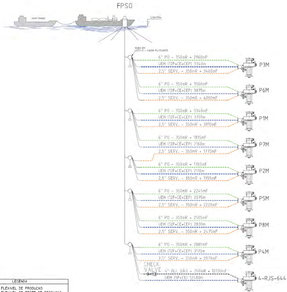
Campo de Maromba – Diagrama Unifilar
