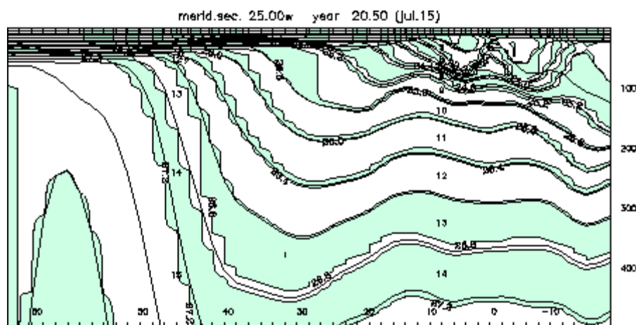
Figura 8: Seção meridional do HYCOM na longitude de 25° W, na porção leste do Atlântico Norte no dia 15 de julho de 2002. Área sombreada: densidade. Linhas finas: interfaces das camadas. Linha grossa: profundidade da camada de mistura. Fonte: http://www.hycom.org/hycom/overview .
