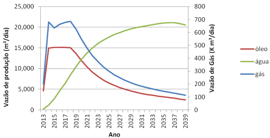
FIGURA II.2.6 – Curva de produção prevista para o Bloco BM-C-41.
