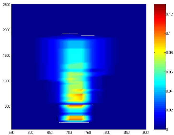
Figura 6.3.8-i: Cenário 3 – Profundidade de 10 metros
