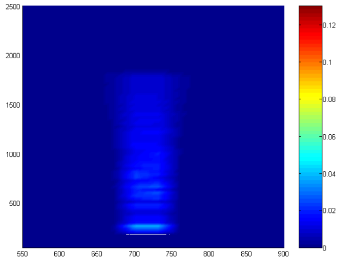
Figura 6.3.8-e: Cenário 1 – Profundidade de 5 metros
