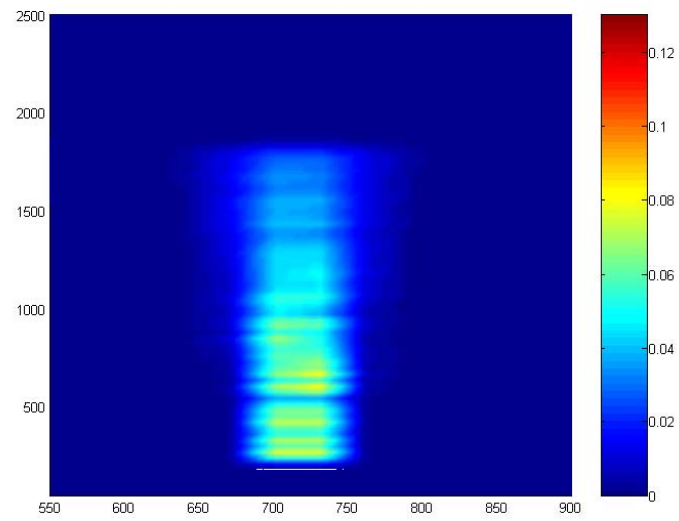
Figura 6.3.8-h: Cenário 2 – Profundidade de 10 metros
