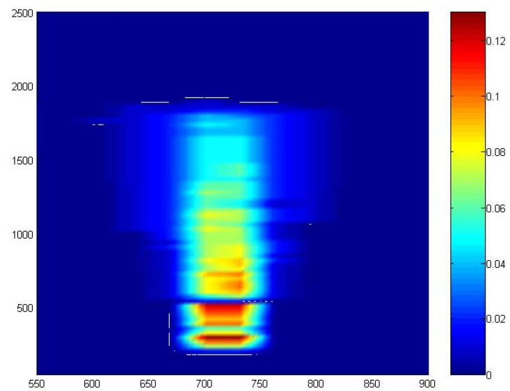
Figura 6.3.8-j: Cenário 3 – Profundidade de 15 metros
