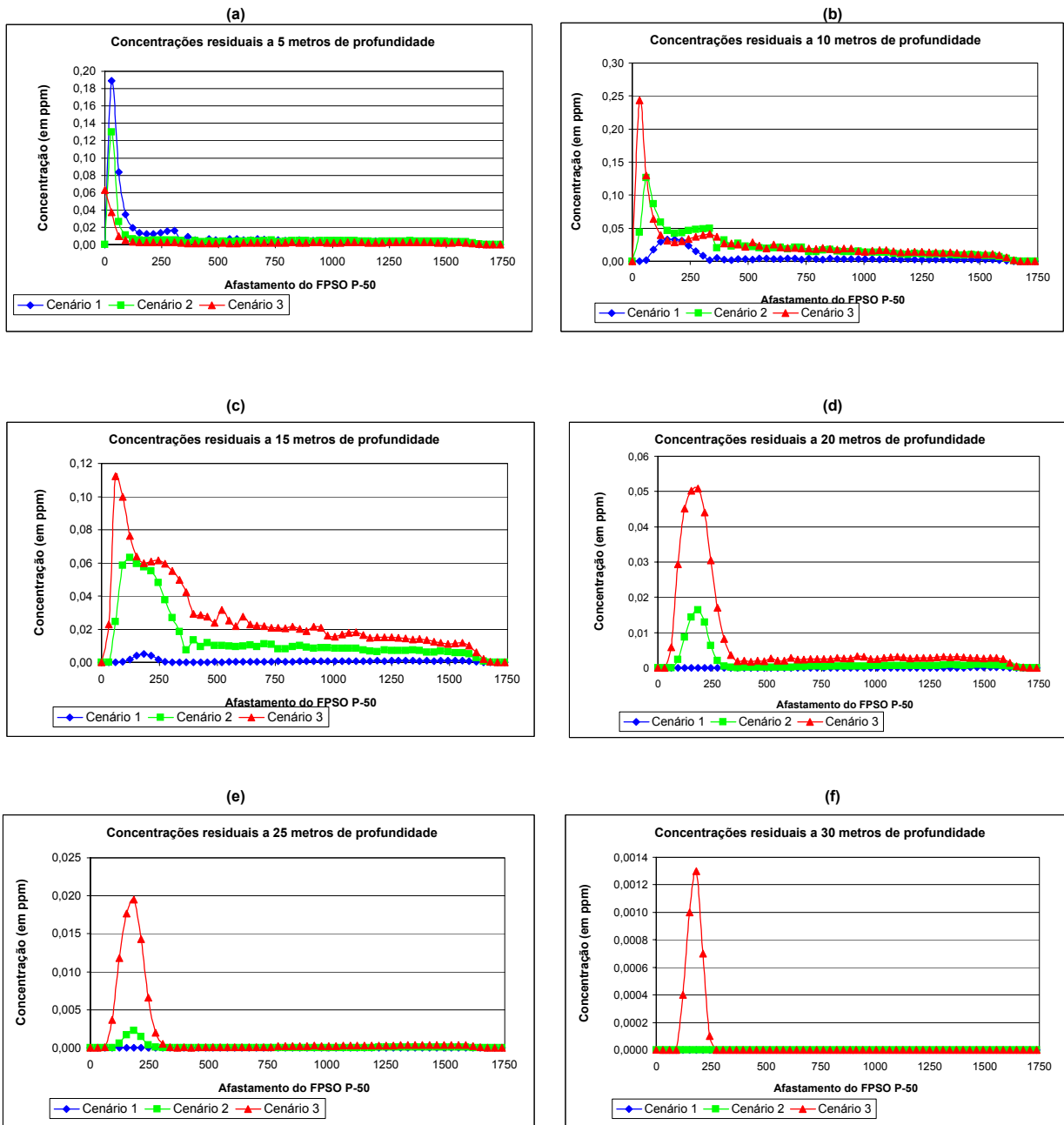
Figura 6.3.8-k. Concentrações residuais de óleo após descarte de água produzida.
