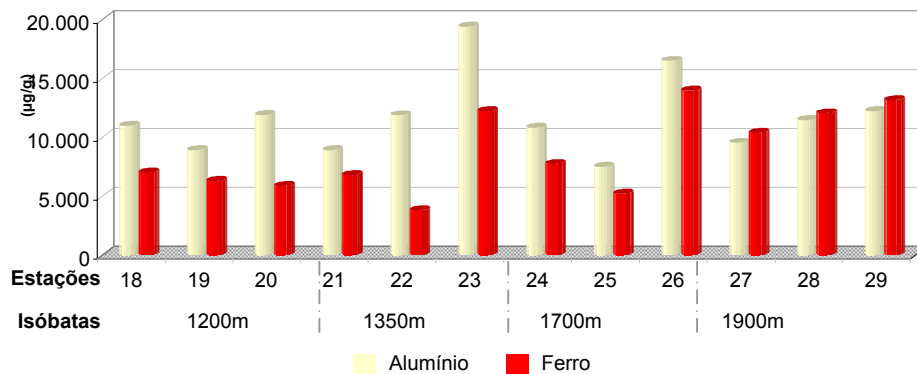
Figura 5.1.5-m. Metais, em µg/g, medidos no sedimento de doze estações no campo de Albacora Leste (Maio/2002).
