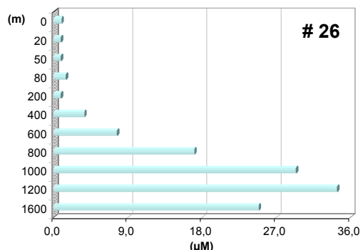
Figura 5.1.4-l. Silicato, em \mu\text{M} , medido em seis estações no campo de Albacora Leste (Maio/2002).
