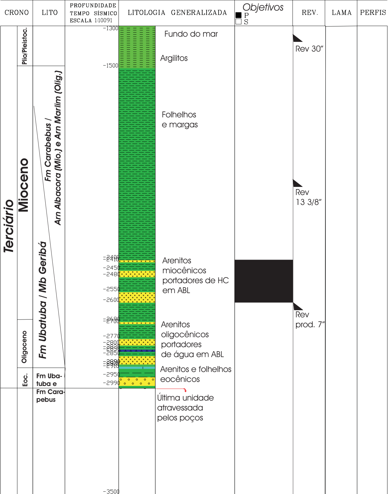
Figura 5.1.2-h - Coluna estratigráfica atravessada por um poço modelo do Campo de Albacora Leste
