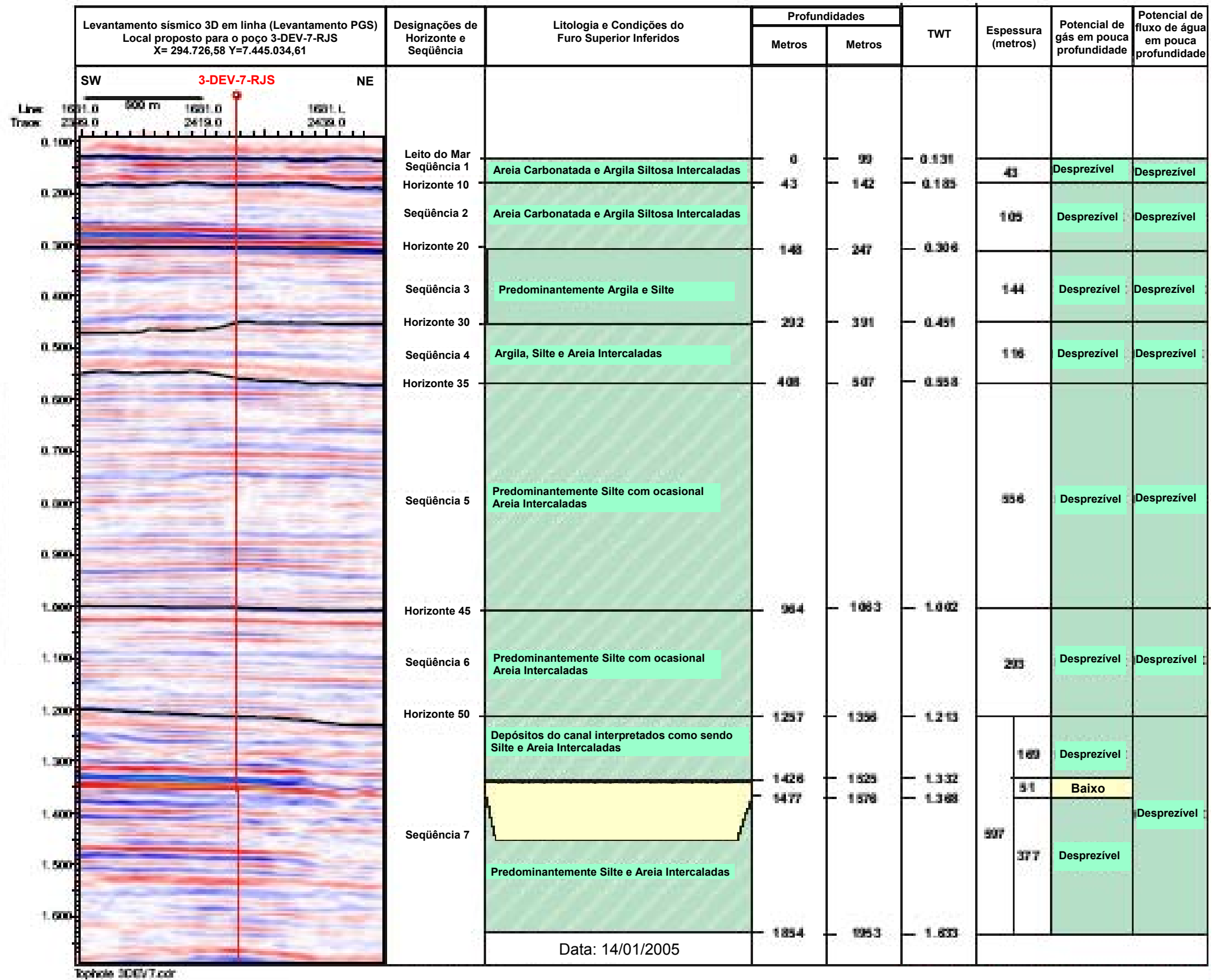
FIGURA II.8.2-1: SEQÜÊNCIA ESTRATIGRÁFICA DO POÇO 3-DEV-7-RJS
