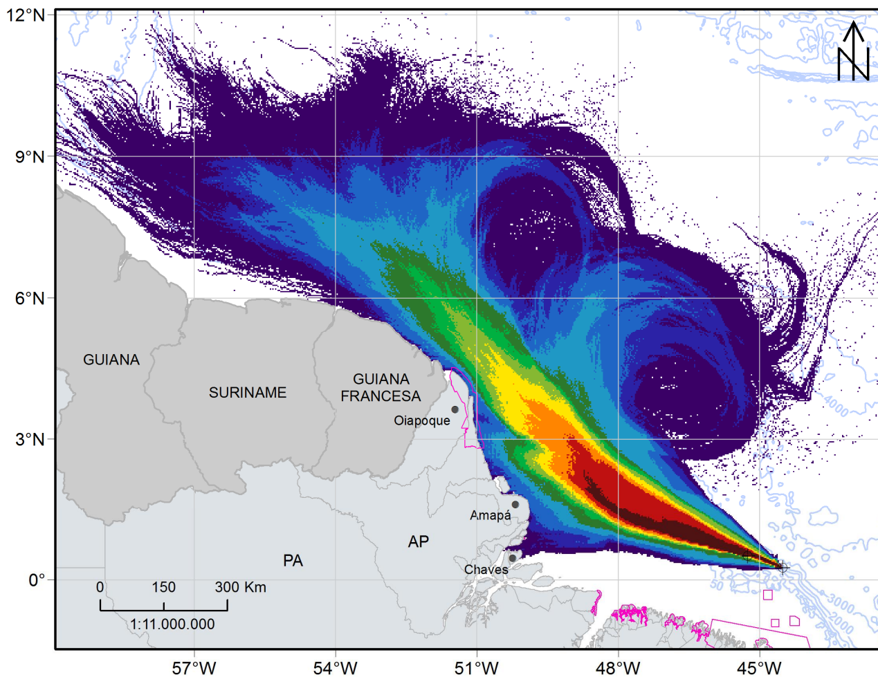
FIGURA II.9.4.1.6 – Probabilidade de presença de óleo em superfície e na coluna d'água para o CENÁRIO 6 (inverno; volume: 20.509 m 3 ; 60 dias de simulação).
