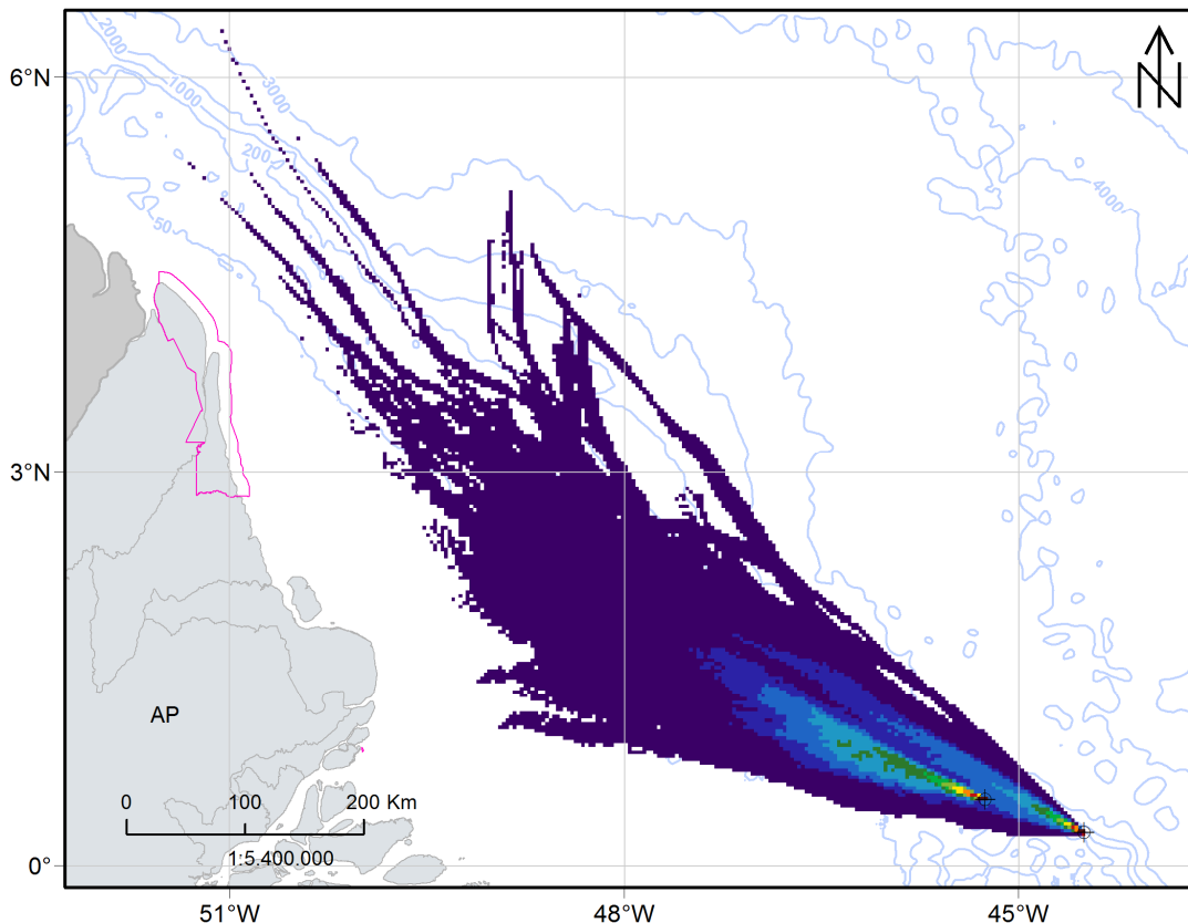
FIGURA II.9.4.1.4 – Probabilidade de presença de óleo em superfície para o CENÁRIO 4 (inverno; volume: 200 m 3 ; 30 dias de simulação).
