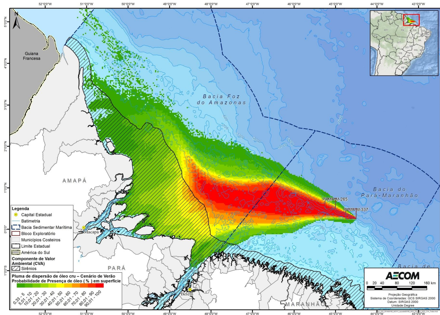
FIGURA II.9.4.2.21 – Cruzamento da área de ocorrência de sirênios com as probabilidades de chegada de óleo, no cenário de verão.
