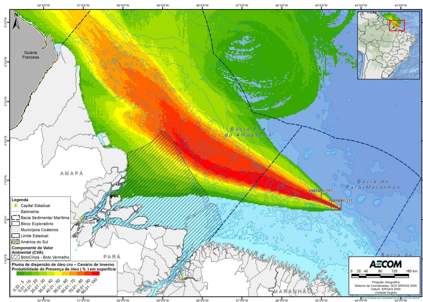
FIGURA II.9.4.2.18 - Área de ocorrência de populações residentes de Sotalia guianensis (boto-cinza) e Inia geoffrensis (boto-vermelho) na área com probabilidades de chegada de óleo, no cenário de inverno, pior caso.
