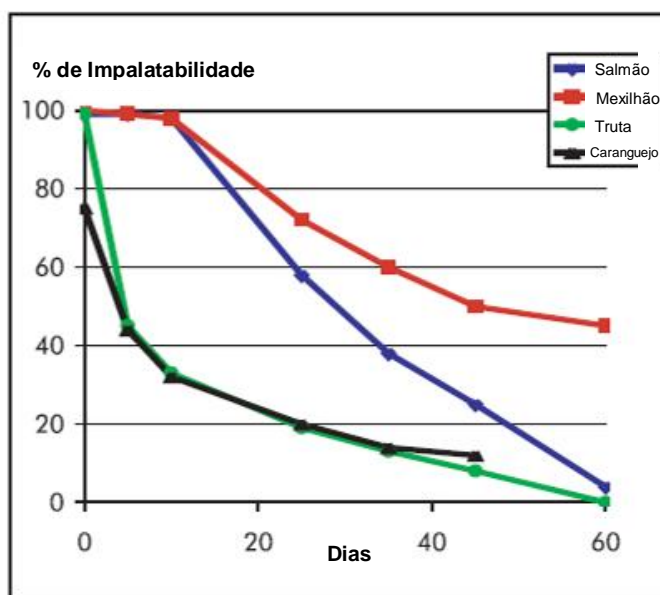
FIGURA II.9.4.2.12 – Taxa de depuração de recursos pesqueiros após contaminação por óleo.
