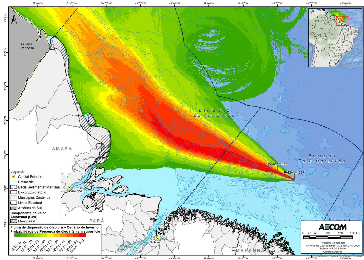
FIGURA II.9.4.2.2 – Localização dos manguezais na área com probabilidades de chegada de óleo, no cenário de inverno, pior caso.
