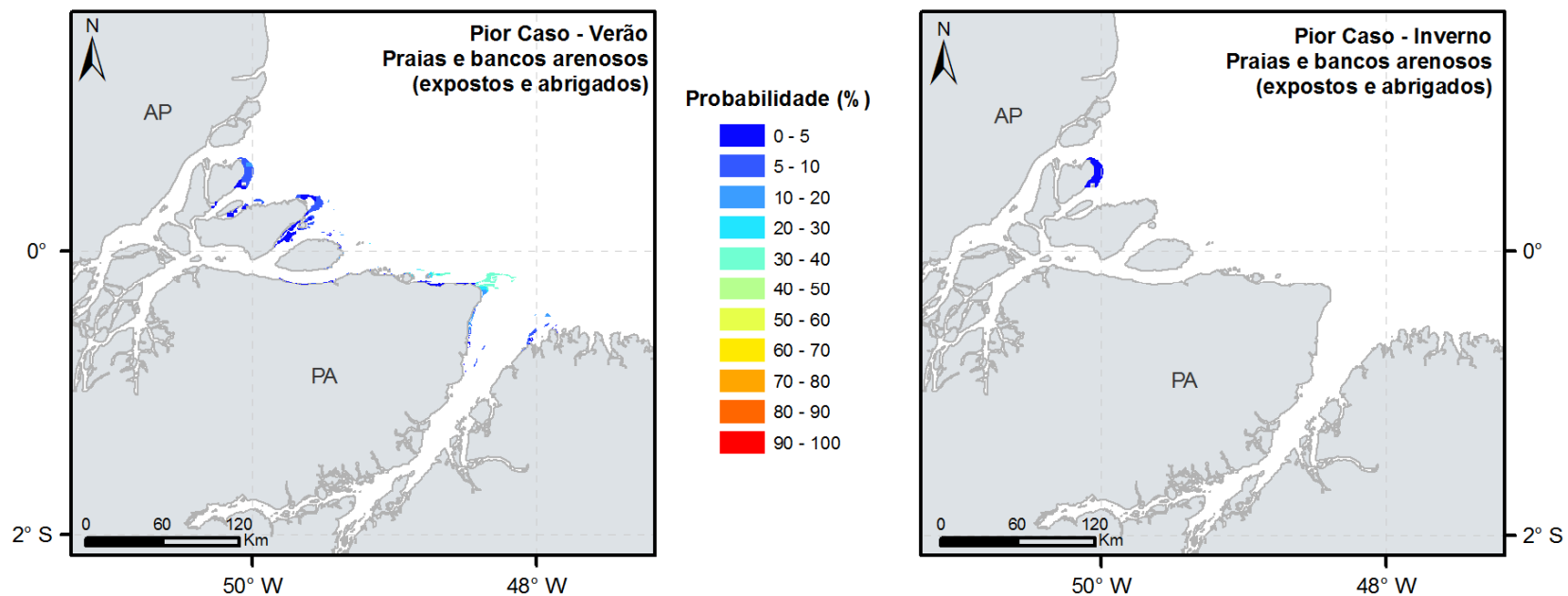
FIGURA II.9.4.3.15 - Probabilidade de presença de óleo no CVA – Praias e Bancos de Areia (Expostos e Abrigados), nos cenários 5 e 6.
