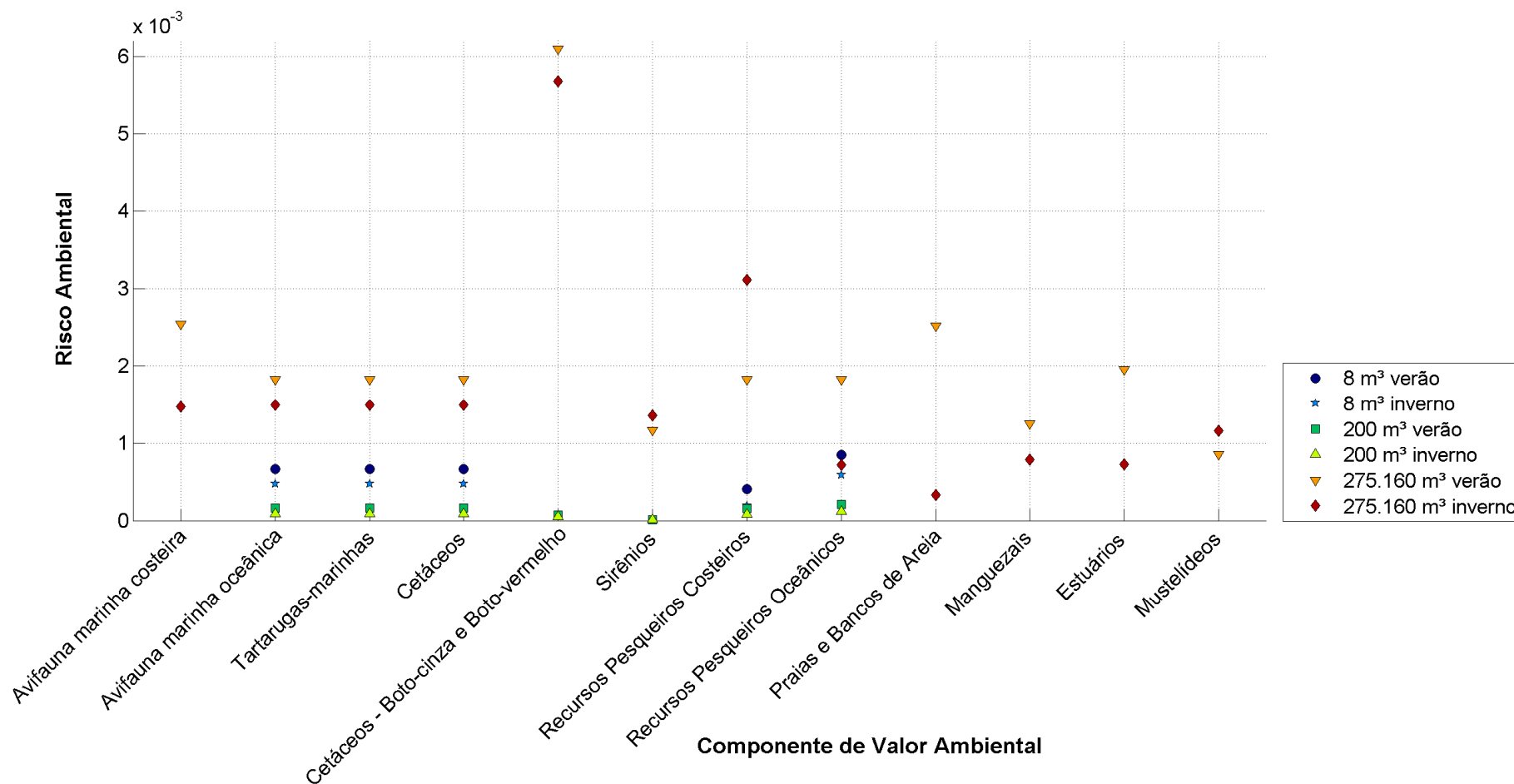
FIGURA II.9.5.1 – Risco Ambiental de todos os Componentes de Valor Ambiental para cada cenário de vazamento.
