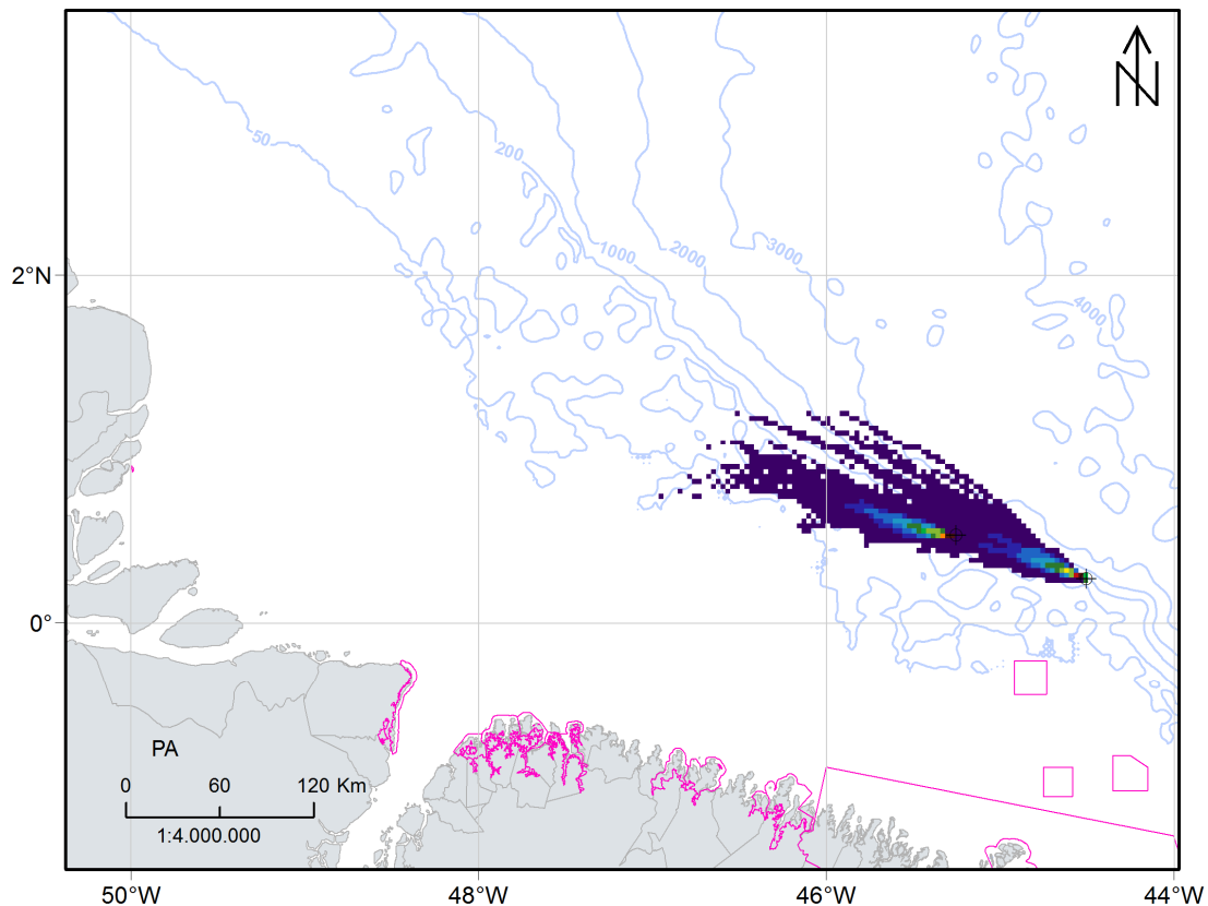
FIGURA II.9.4.1.1 – Probabilidade de presença de óleo em superfície para o CENÁRIO 1 (verão; volume: 8 m 3 ; 30 dias de simulação).
