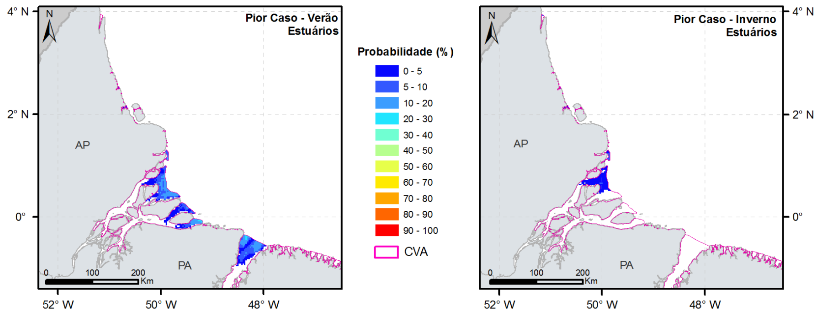
FIGURA II.9.4.3.16 - Probabilidade de presença de óleo no CVA – Estuários, nos cenários 5 e 6.
