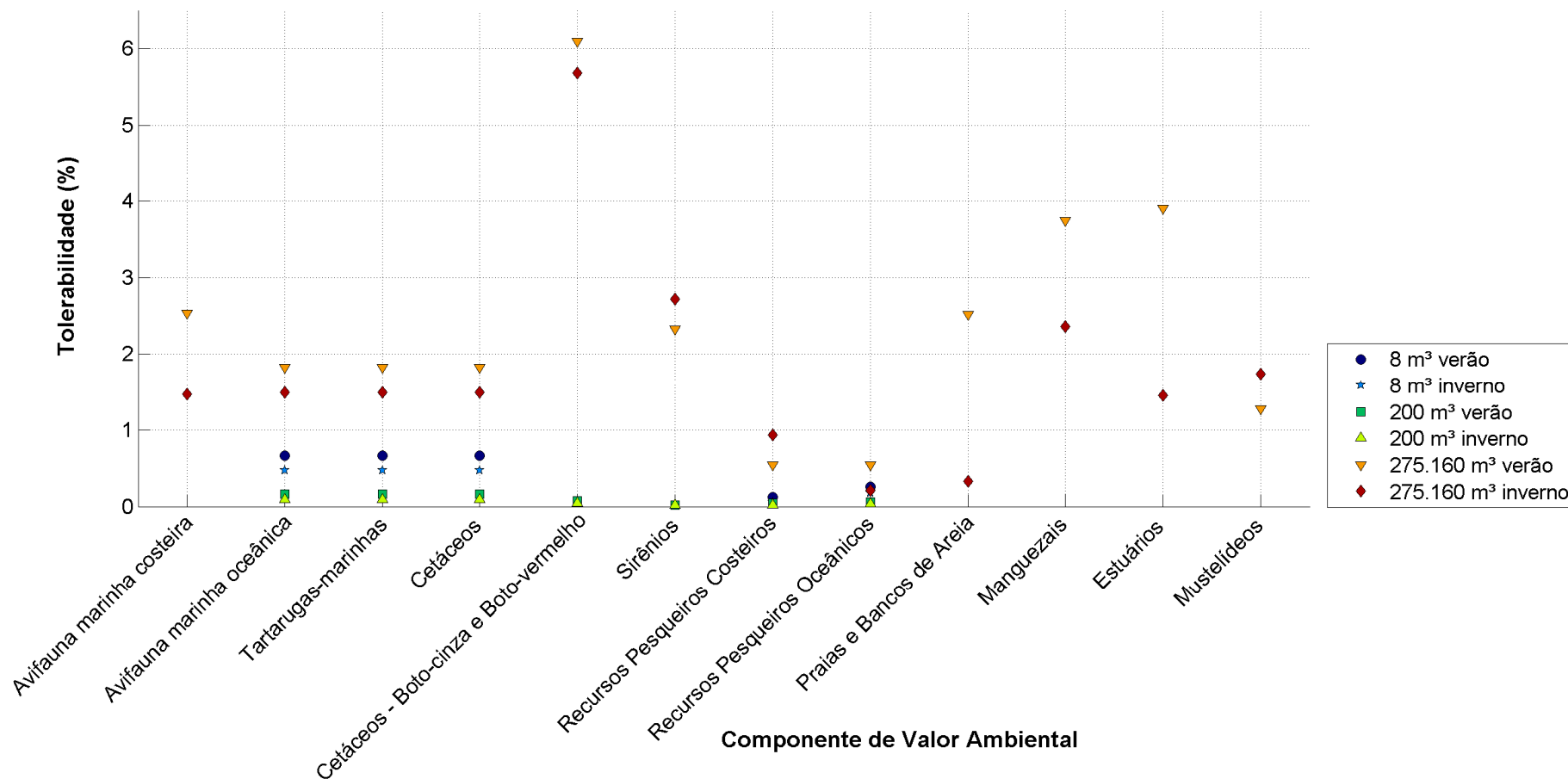
FIGURA II.9.6.1 – Tolerabilidade de cada Componente de Valor Ambiental, para cada cenário de vazamento de óleo.
