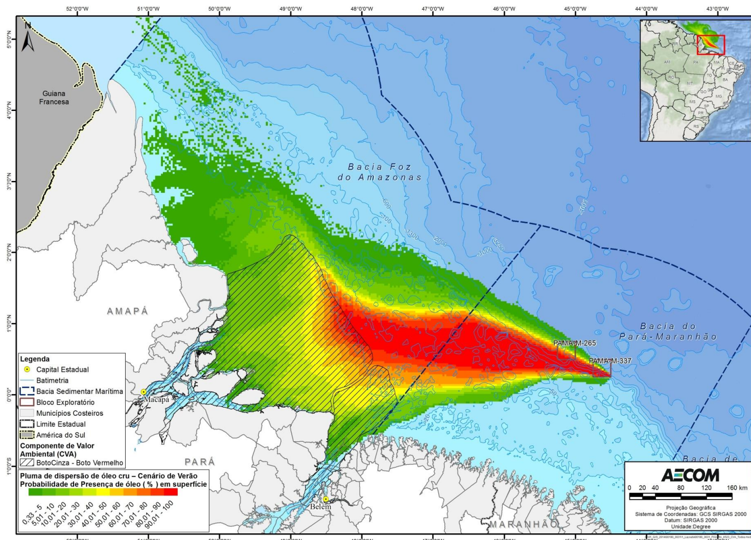
FIGURA II.9.4.2.19 - Área de ocorrência de populações residentes de Sotalia guianensis e Inia geoffrensis na área com probabilidades de chegada de óleo, no cenário de verão, pior caso.
