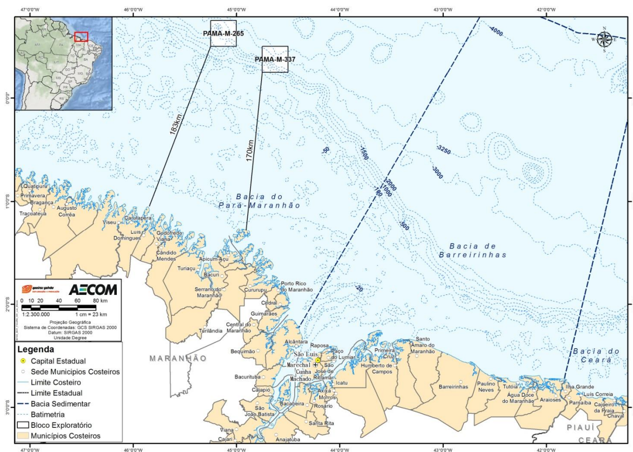
FIGURA II.9.1 – Localização dos Blocos PAMA-M-265 e PAMA-M-337, Bacia do Pará-Maranhão.
