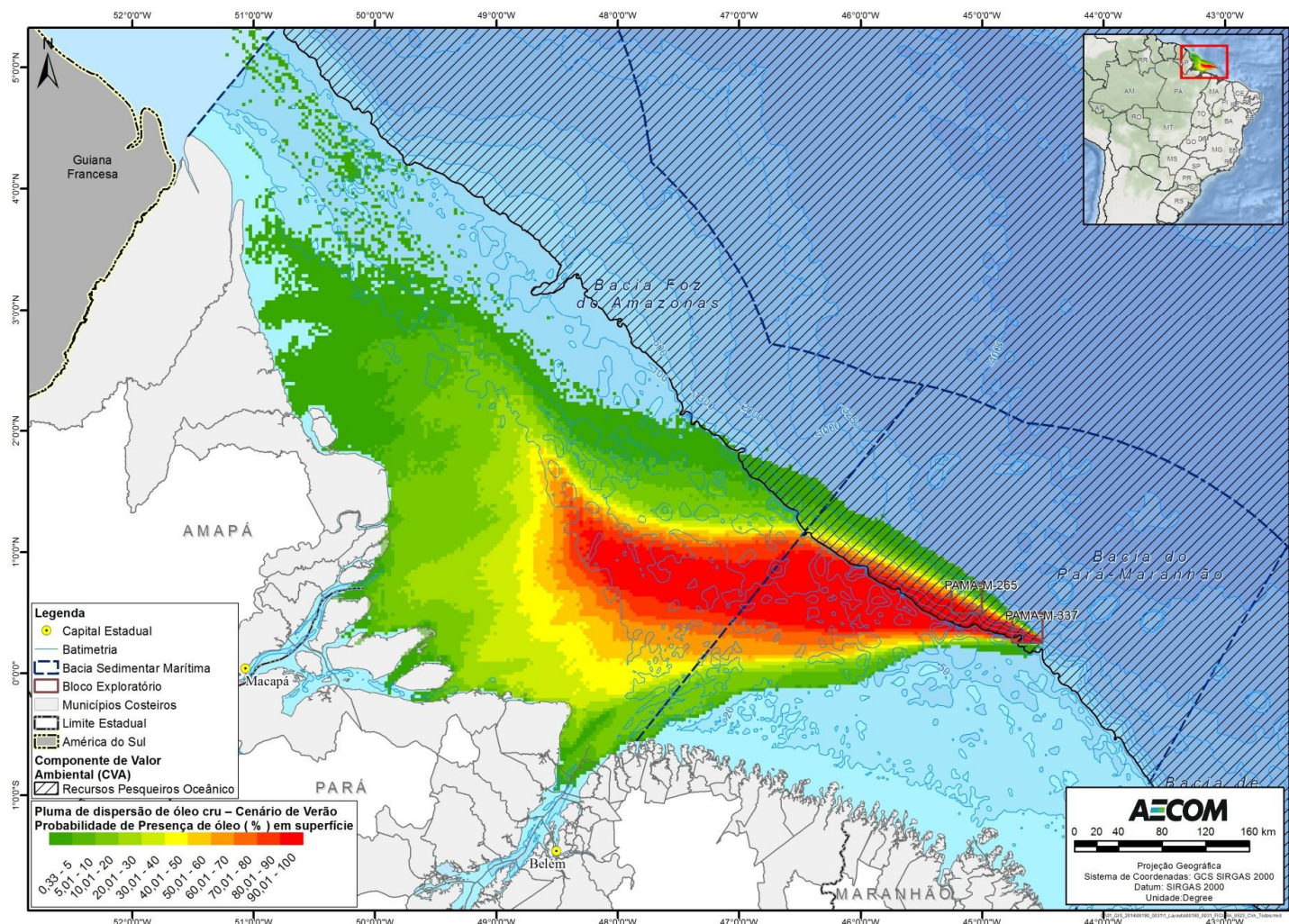
FIGURA II.9.4.2.9 - Área de concentração de recursos pesqueiros oceânicos na área com probabilidades de chegada de óleo, no cenário de verão, pior caso.
