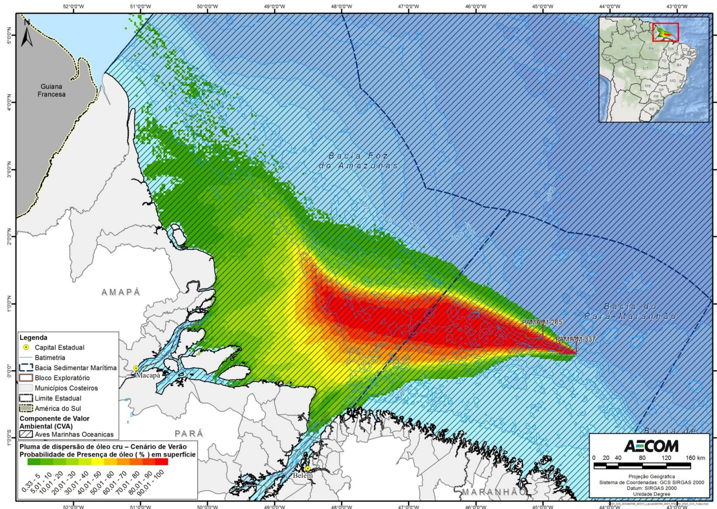
FIGURA II.9.4.2.27 – Áreas de ocorrência de avifauna marinha oceânica na área com probabilidades de chegada de óleo, no cenário de verão, pior caso.
