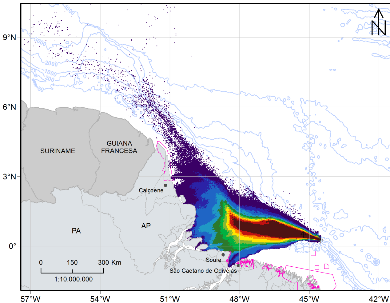
FIGURA II.9.4.1.5 – Probabilidade de presença de óleo em superfície e na coluna d'água para o CENÁRIO 5 (verão; volume: 20.509 m 3 ; 60 dias de simulação).
