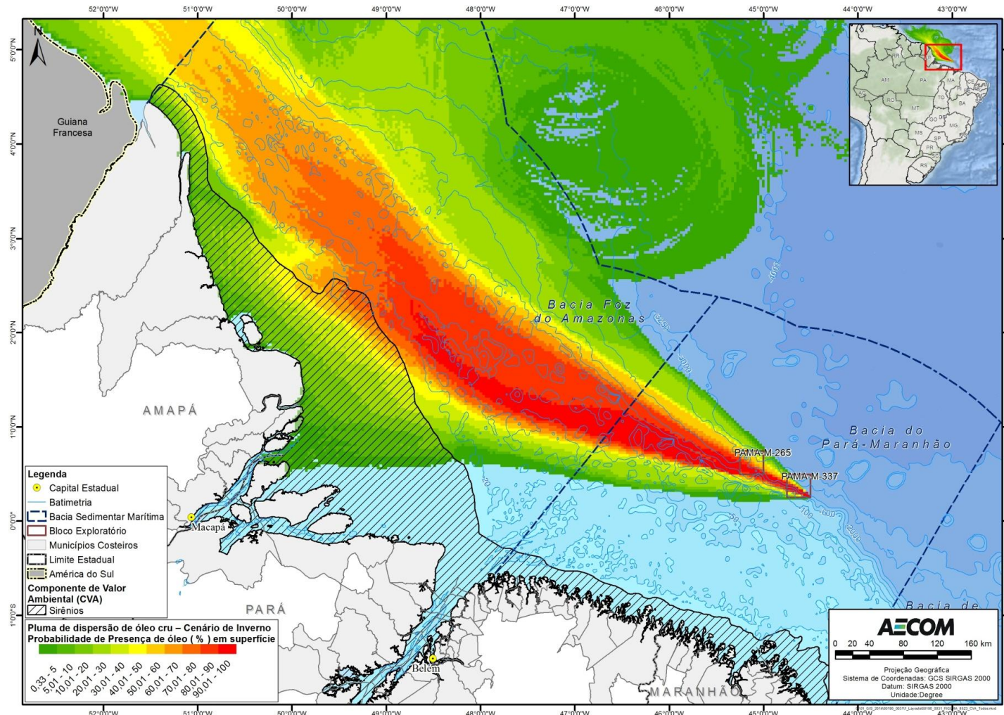
FIGURA II.9.4.2.20 – Cruzamento da área de ocorrência de sirênios com as probabilidades de chegada de óleo, no cenário de inverno.
