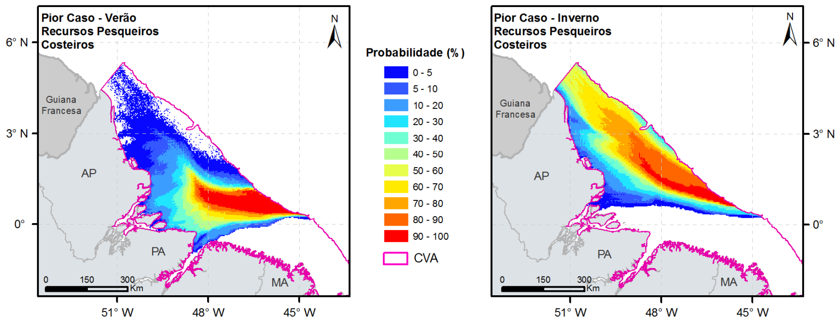
FIGURA II.9.4.3.11 - Probabilidade de presença de óleo no CVA – Recursos Pesqueiros Costeiros, nos cenários 5 e 6.
