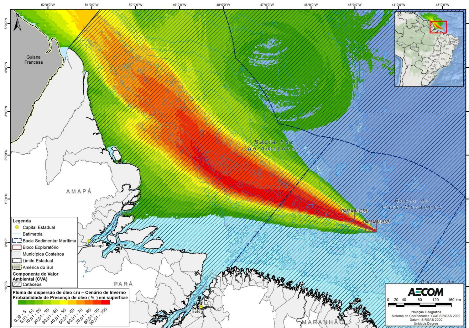
FIGURA II.9.4.2.15 – Área de ocorrência de cetáceos nas áreas com probabilidades de chegada de óleo, no cenário de inverno, pior caso.
