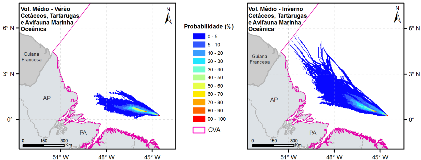
FIGURA II.9.4.3.3 - Probabilidade de presença de óleo nos CVAs Avifauna Marinha Oceânica, Cetáceos; Tartarugas, nos cenários 3 e 4.
