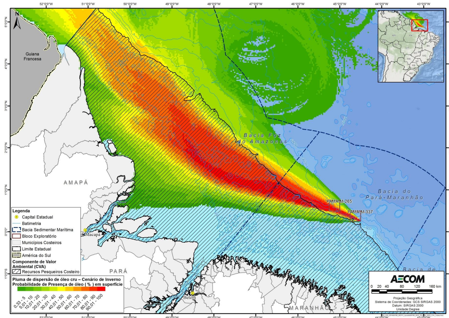
FIGURA II.9.4.2.10 - Área de concentração de recursos pesqueiros costeiros na área com probabilidades de chegada de óleo, no cenário de inverno, pior caso.
