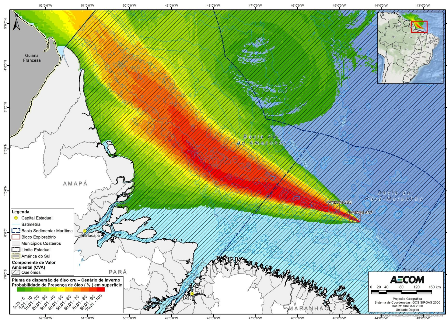
FIGURA II.9.4.2.13 – Área de ocorrência não reprodutiva de tartarugas na área com probabilidades de chegada de óleo, no cenário de inverno, pior caso.
