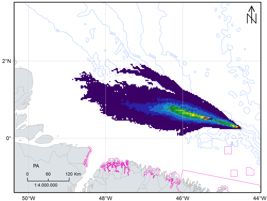
FIGURA II.9.4.1.3 – Probabilidade de presença de óleo em superfície para o CENÁRIO 3 (verão; volume: 200 m 3 ; 30 dias de simulação).
