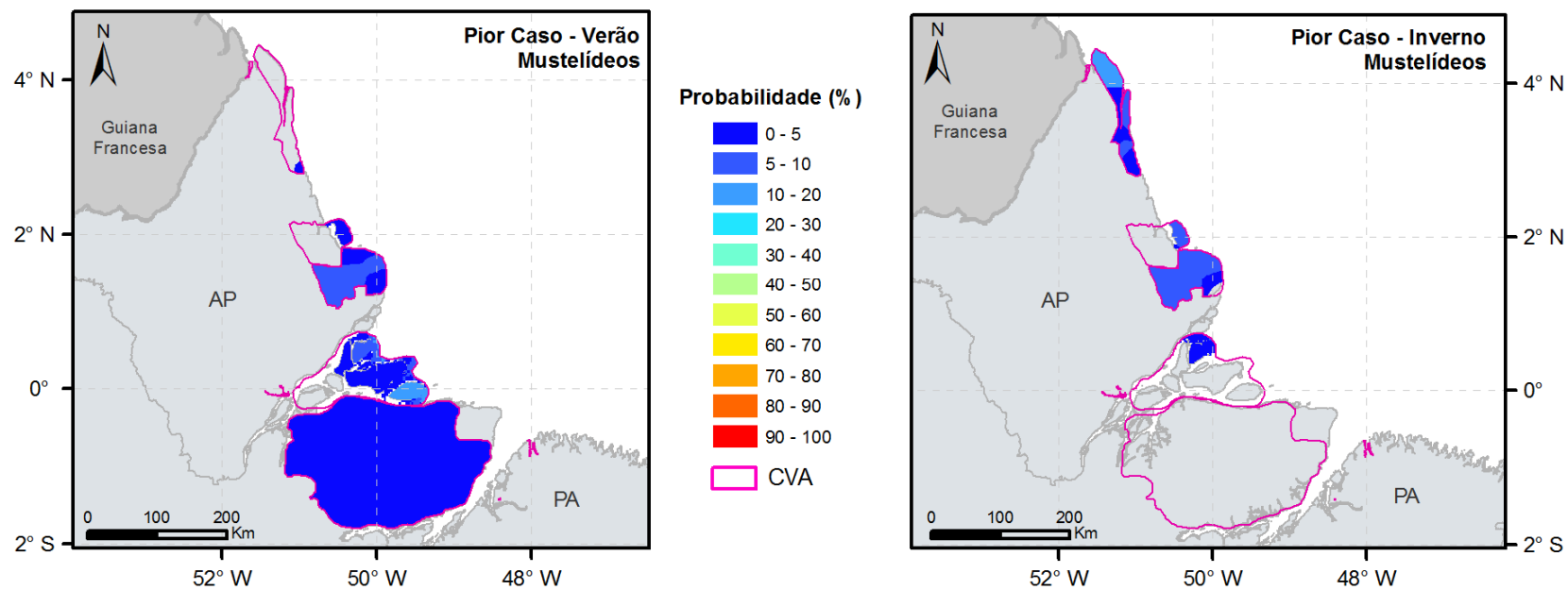
FIGURA II.9.4.3.18 - Probabilidade de presença de óleo no CVA – Recifes de Corais, nos cenários 5 e 6.
