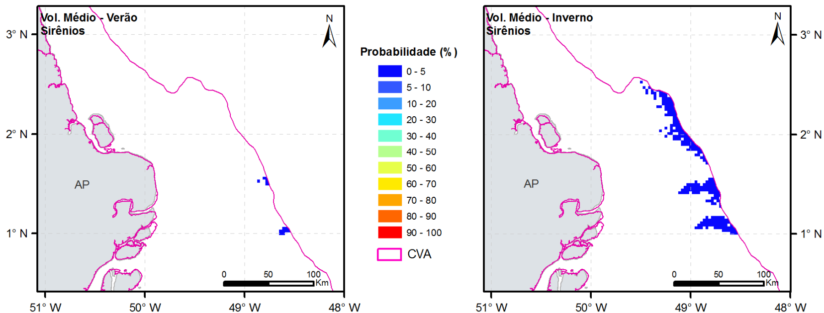
FIGURA II.9.4.3.7 - Probabilidade de presença de óleo no CVA – Sirênios, nos cenários 3 e 4.
