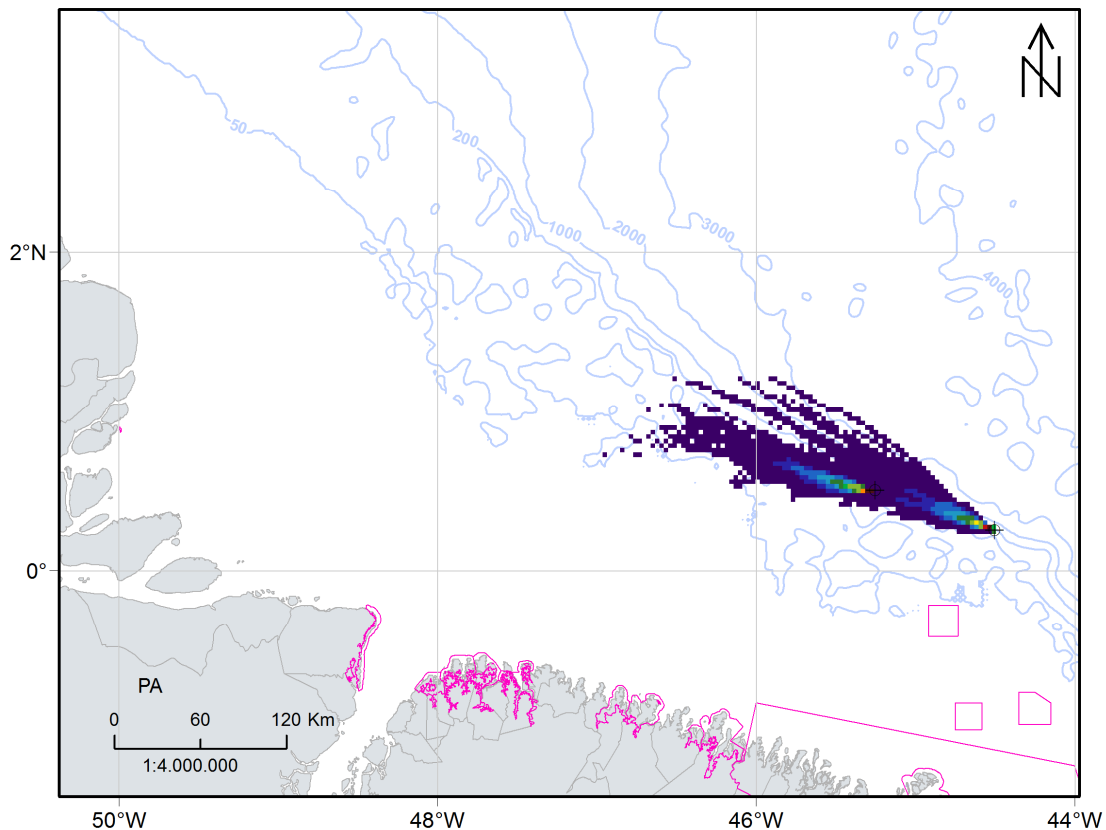
FIGURA II.9.4.1.2 – Probabilidade de presença de óleo em superfície para o CENÁRIO 2 (inverno; volume: 8m 3 ; 30 dias de simulação).
