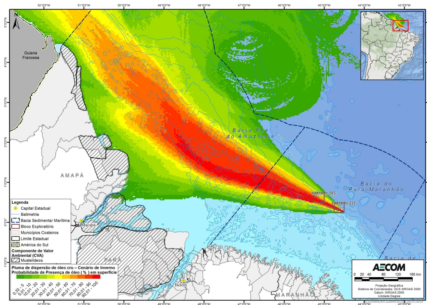
FIGURA II.9.4.2.22 – Cruzamento da área de ocorrência de mustelídeos com as probabilidades de chegada de óleo, no cenário de inverno.
