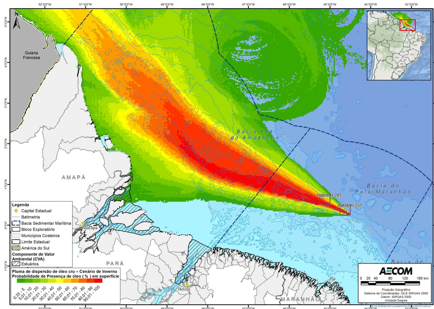
FIGURA II.9.4.2.4 – Localização dos estuários na área com probabilidades de chegada de óleo, no cenário de inverno, pior caso.
