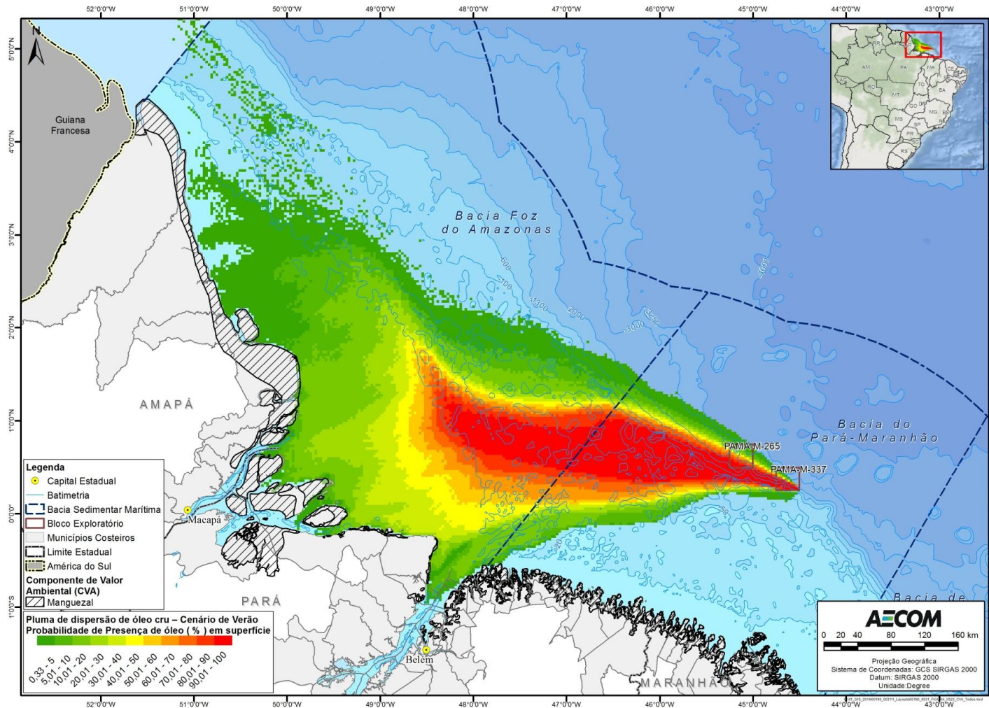
FIGURA II.9.4.2.3 – Localização dos manguezais na área com probabilidades de chegada de óleo, no cenário de verão, pior caso.
