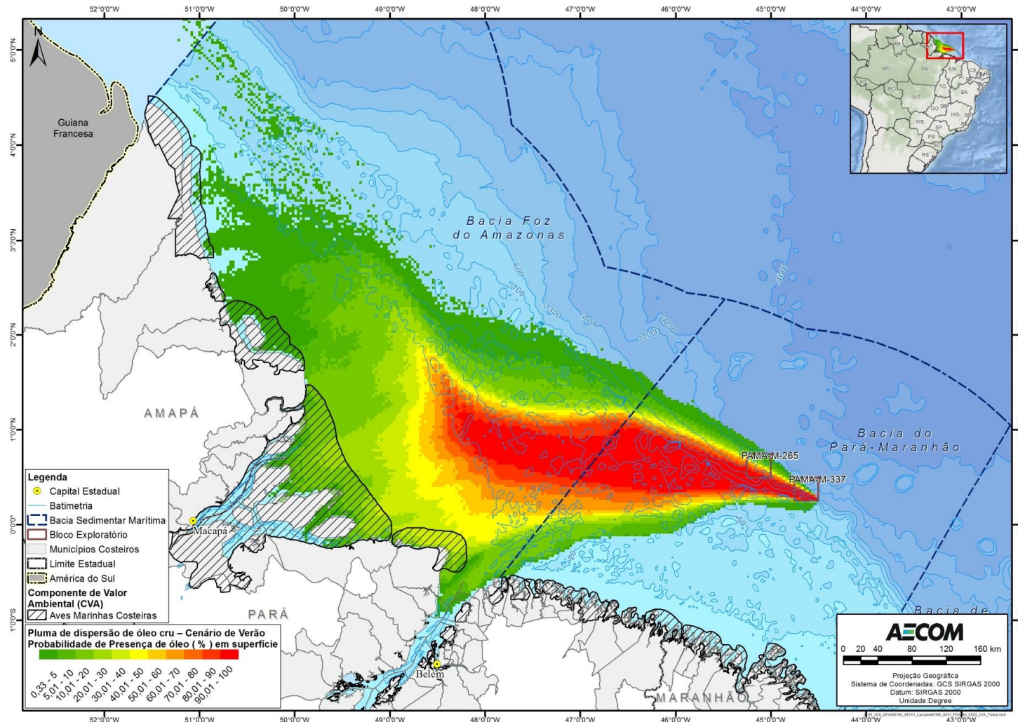
FIGURA II.9.4.2.25 Áreas de concentração de avifauna marinha costeira na área com probabilidades de chegada de óleo, no cenário de verão, pior caso.
