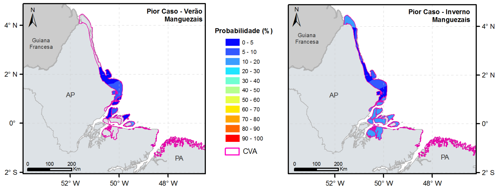
FIGURA II.9.4.3.17 - Probabilidade de presença de óleo no CVA – Manguezais, nos cenários 5 e 6.
