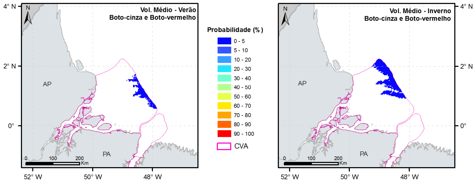
FIGURA II.9.4.3.5 - Probabilidade de presença de óleo no SVA – Cetáceos – Boto-cinza ( Sotalia guianensis ) e Boto-vermelho ( Inia geoffrensis ), nos cenários 3 e 4.
