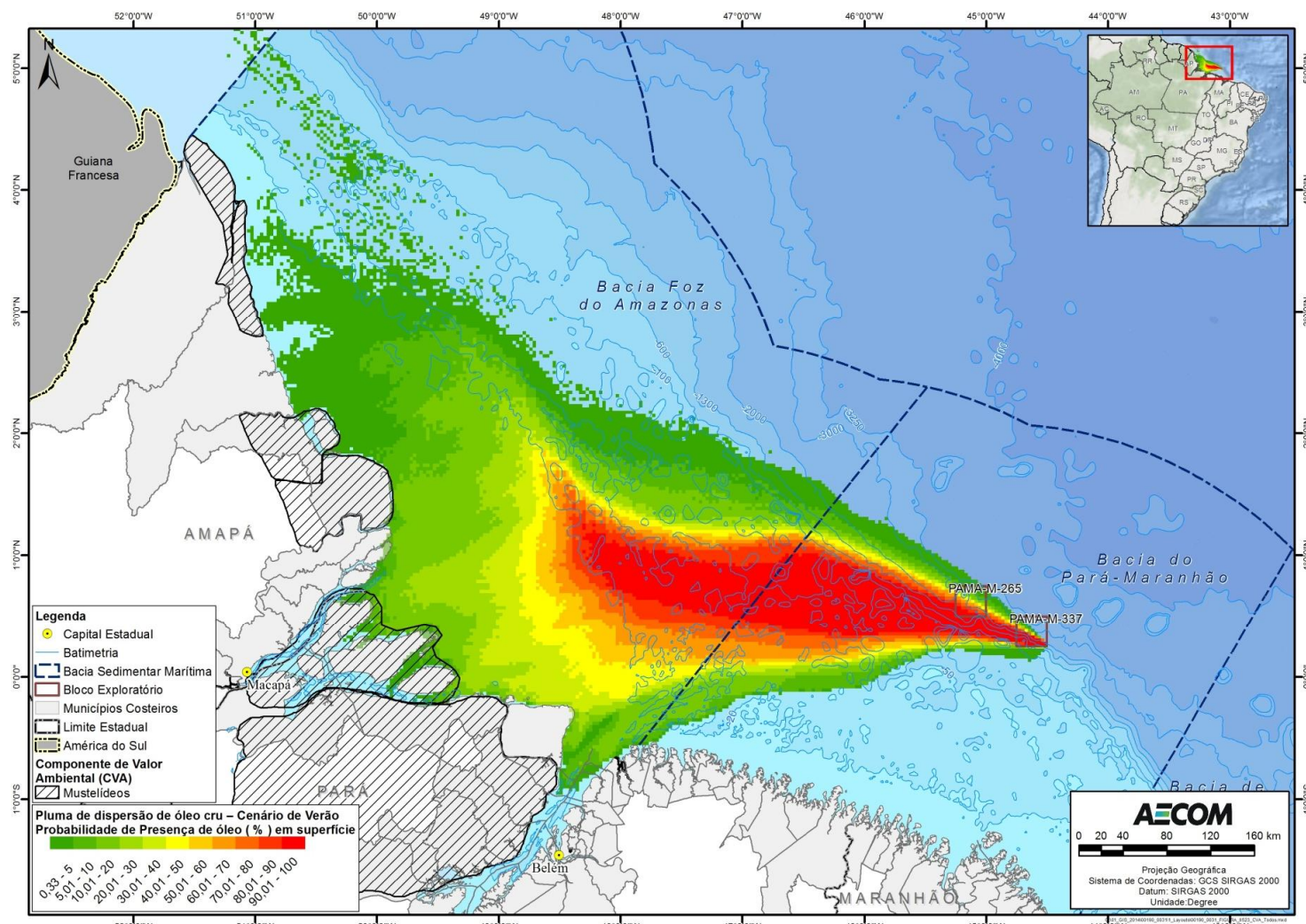
FIGURA II.9.4.2.23 – Cruzamento da área de ocorrência de mustelídeos com as probabilidades de chegada de óleo, no cenário de verão.
