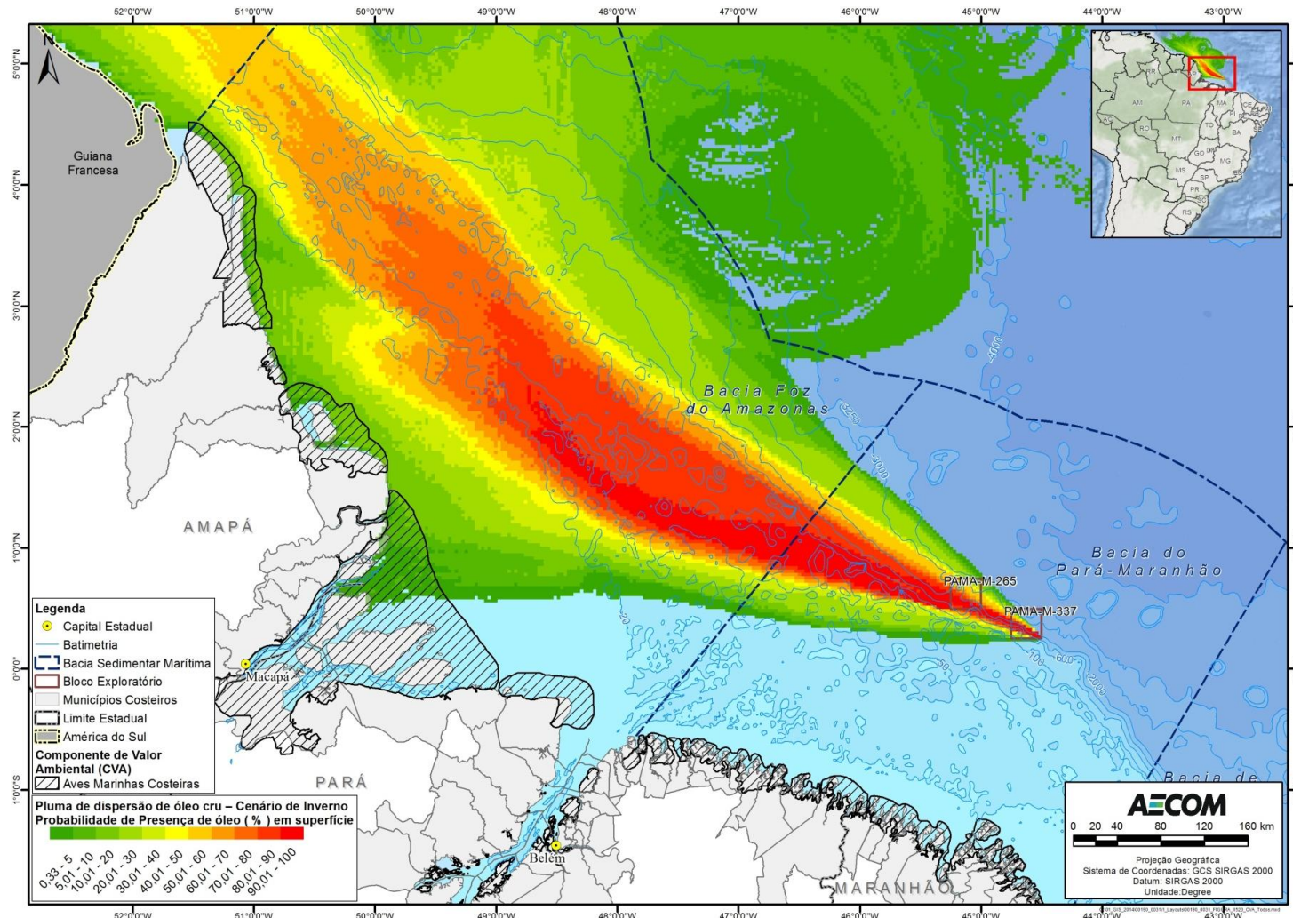
FIGURA II.9.4.2.24 – Áreas de concentração de avifauna marinha costeira na área com probabilidades de chegada de óleo, no cenário de inverno, pior caso.
