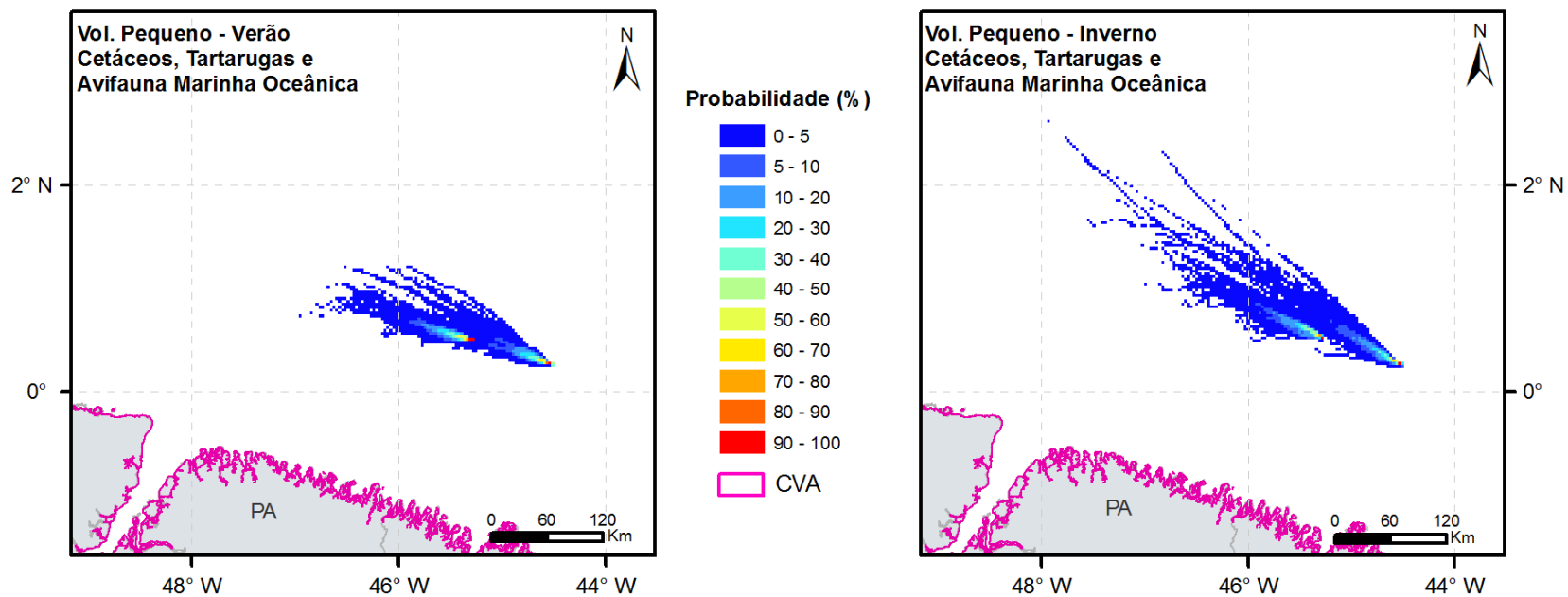
FIGURA II.9.4.3.2 - Probabilidade de presença de óleo nos CVAs Avifauna Marinha Oceânica, Cetáceos; Tartarugas, nos cenários 1 e 2.
