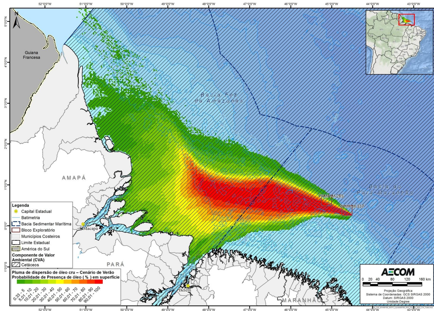
FIGURA II.9.4.2.16 – Área de ocorrência de cetáceos nas áreas com probabilidades de chegada de óleo, no cenário de verão, pior caso.
