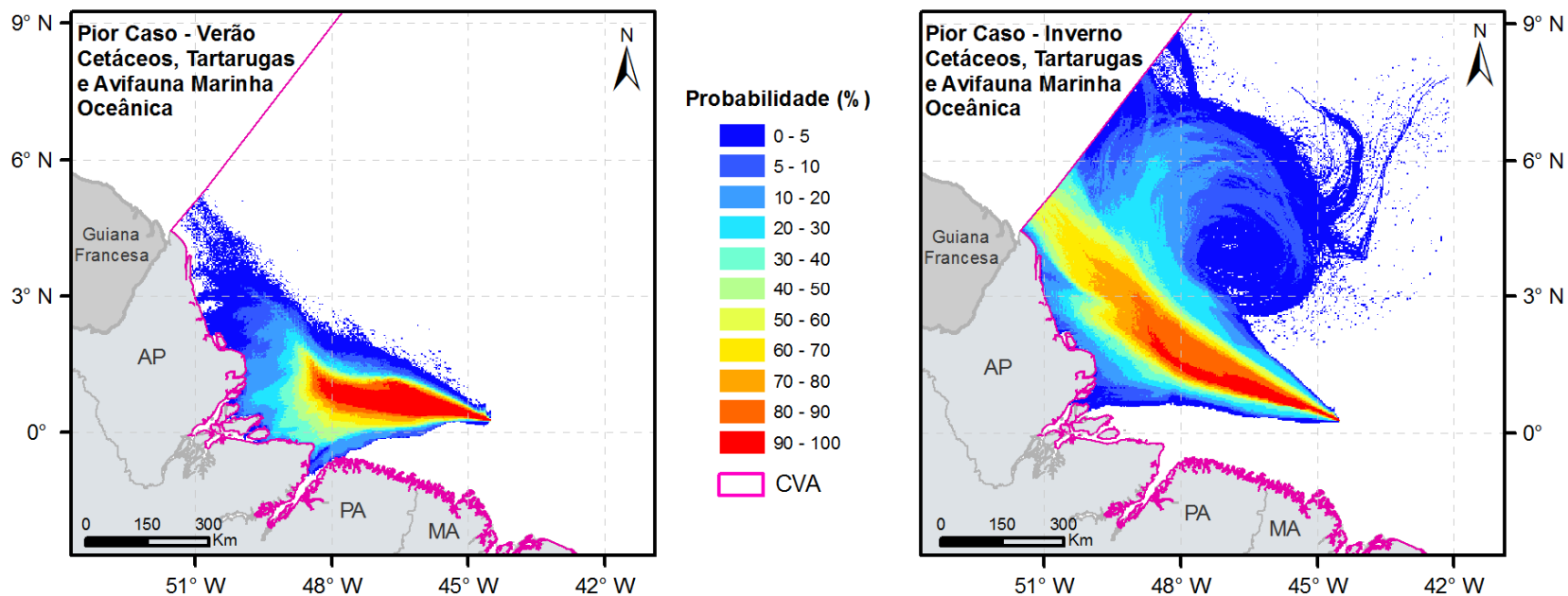
FIGURA II.9.4.3.4 - Probabilidade de presença de óleo nos CVAs Avifauna Marinha Oceânica, Cetáceos; Tartarugas, nos cenários 5 e 6.
