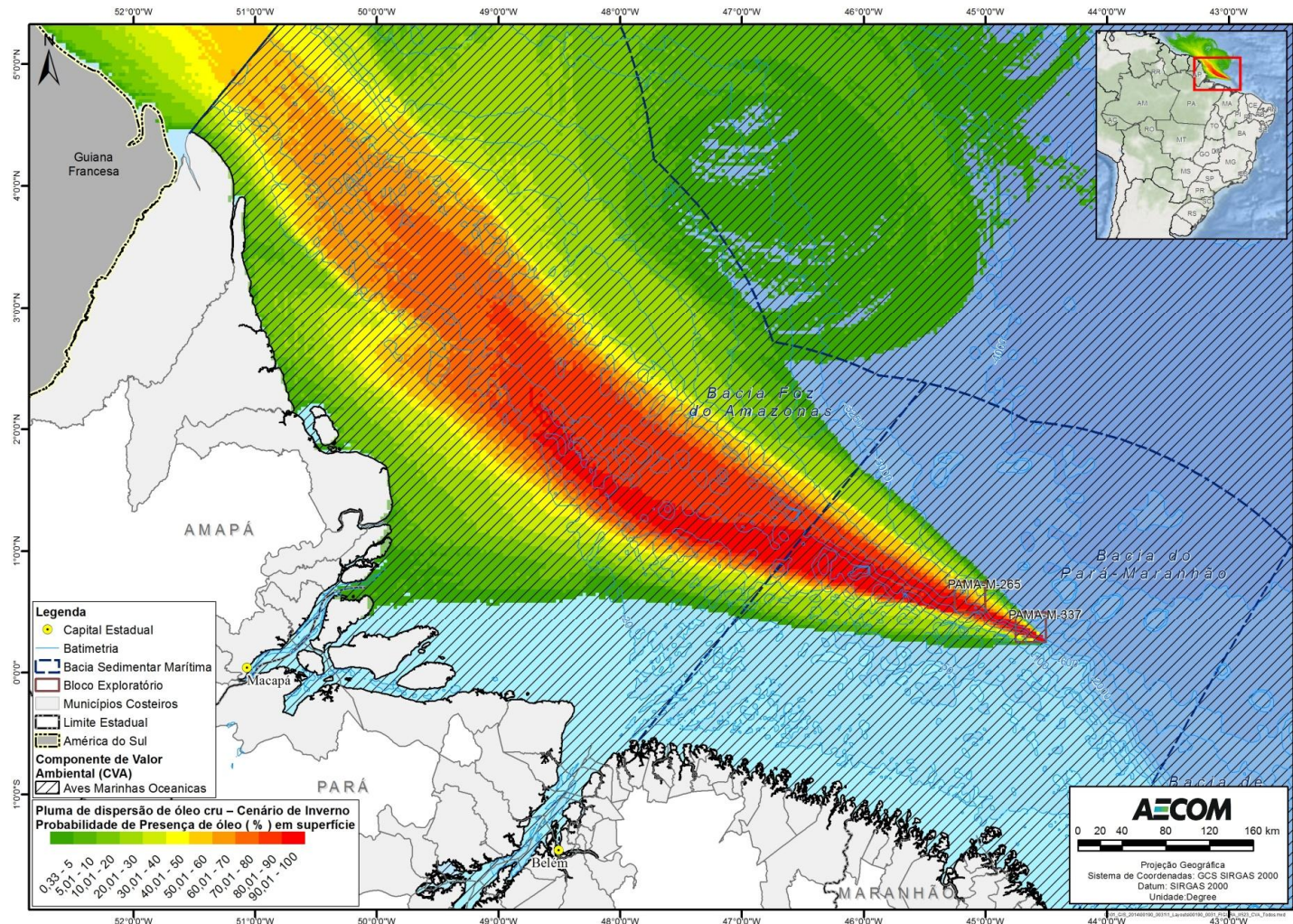
FIGURA II.9.4.2.26 – Áreas de ocorrência de avifauna marinha oceânica na área com probabilidades de chegada de óleo, no cenário de inverno, pior caso.
