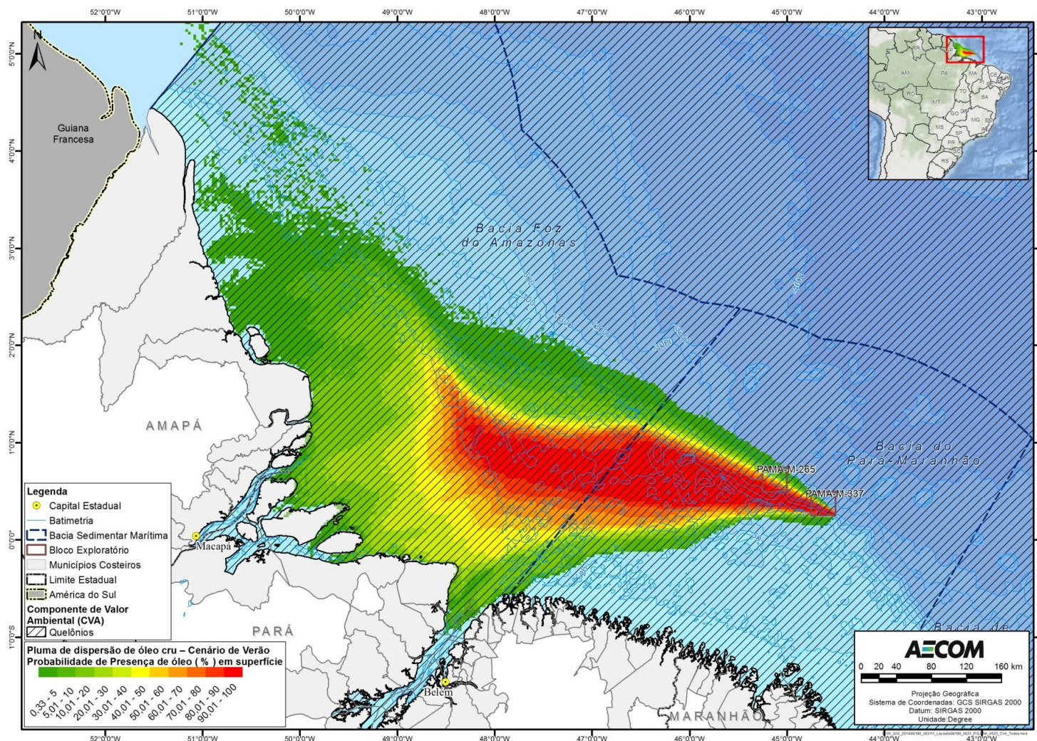
FIGURA II.9.4.2.14 – Área de ocorrência não reprodutiva de tartarugas na área com probabilidades de chegada de óleo, no cenário de verão, pior caso.
