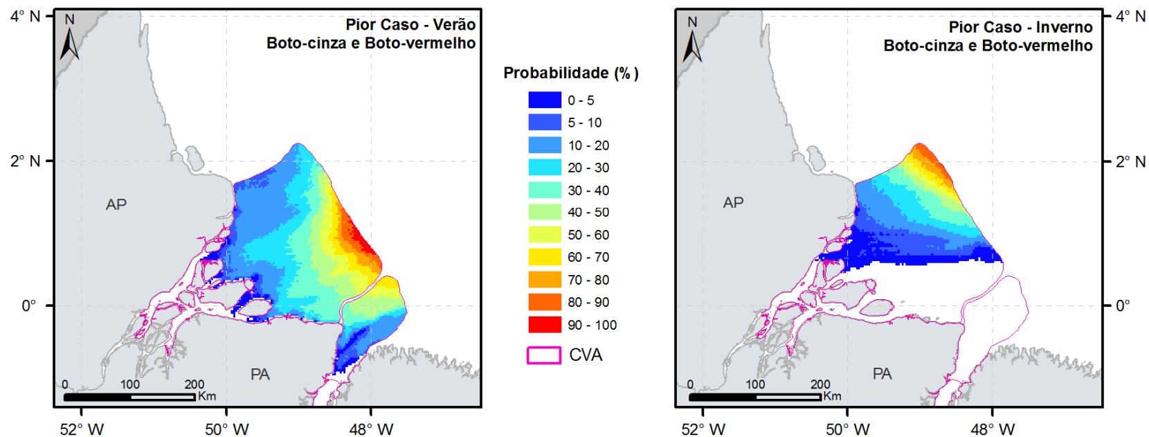
FIGURA II.9.4.3.6 - Probabilidade de presença de óleo no SVA – Cetáceos – Boto-cinza ( Sotalia guianensis ) e Boto-vermelho ( Inia geoffrensis ), nos cenários 5 e 6.
