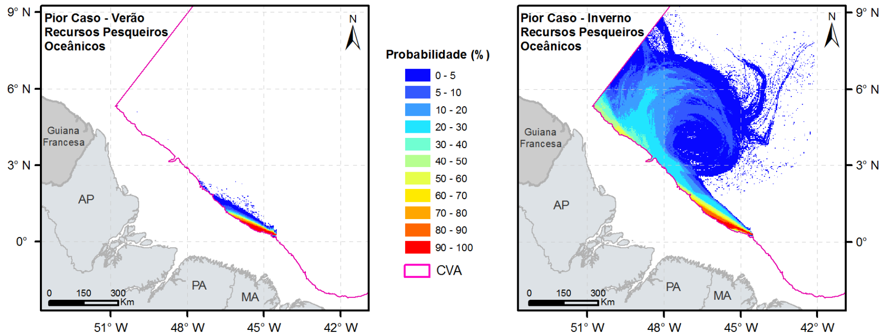
FIGURA II.9.4.3.14 - Probabilidade de presença de óleo no CVA – Recursos Pesqueiros Oceânicos, nos cenários 5 e 6.
