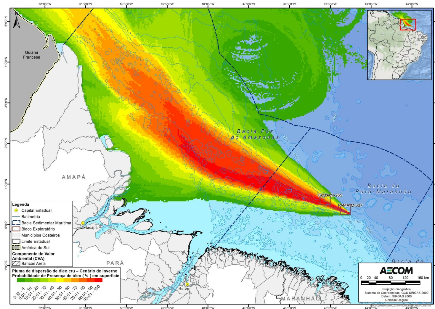
FIGURA II.9.4.2.6 – Localização das praias e bancos arenosos na área com probabilidades de chegada de óleo, no cenário de inverno, pior caso
