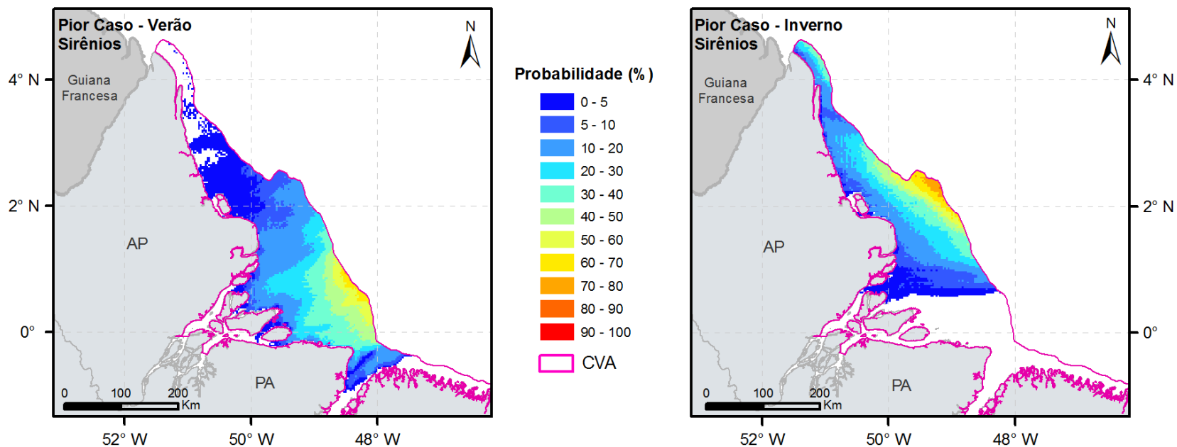
FIGURA II.9.4.3.8 - Probabilidade de presença de óleo no CVA – Sirênios, nos cenários 5 e 6.
