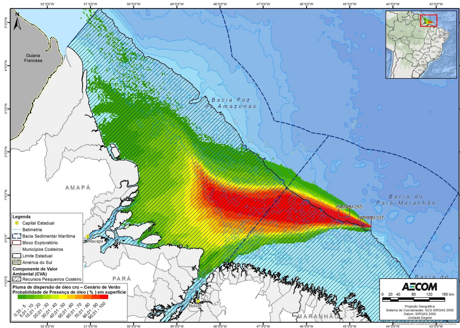
FIGURA II.9.4.2.11 - Área de concentração de recursos pesqueiros costeiros na área com probabilidades de chegada de óleo, no cenário de verão, pior caso.
