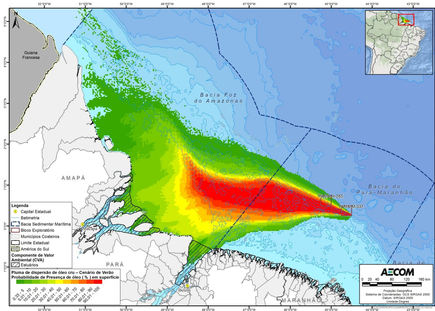
FIGURA II.9.4.2.5 – Localização dos estuários na área com probabilidades de chegada de óleo, no cenário de verão, pior caso.
