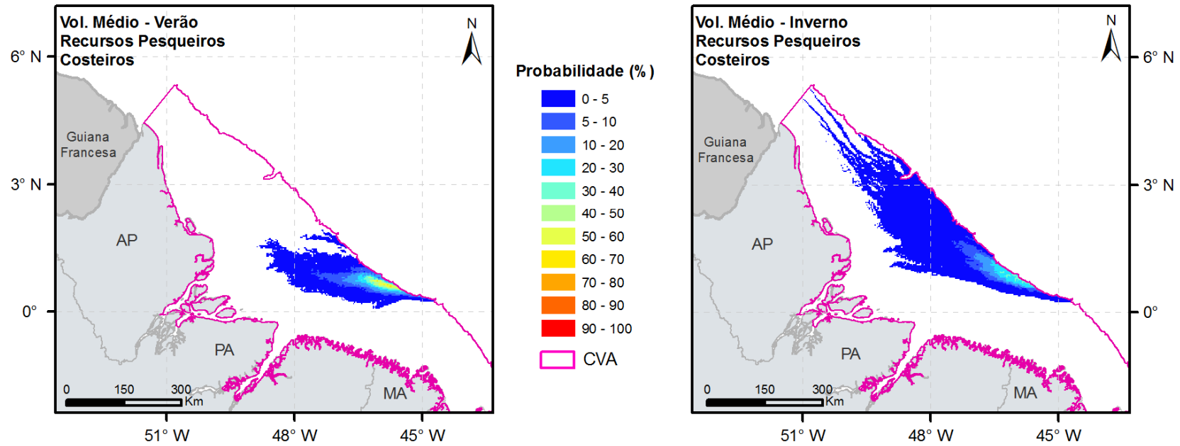
FIGURA II.9.4.3.10 - Probabilidade de presença de óleo no CVA – Recursos Pesqueiros Costeiros, nos cenários 3 e 4.
