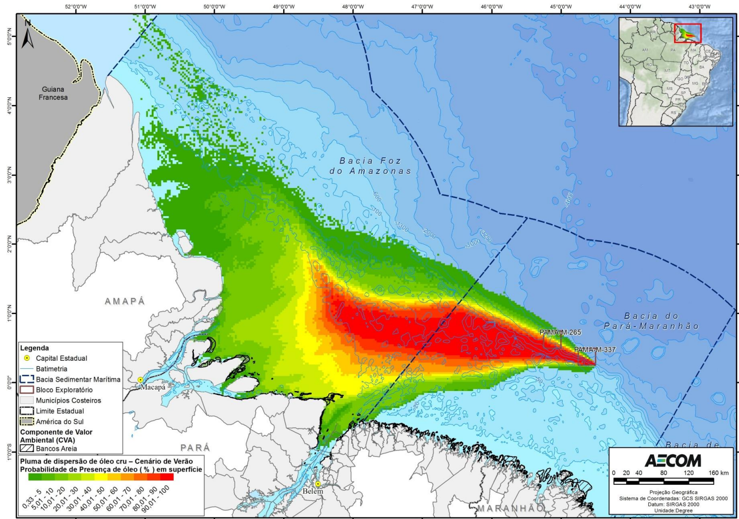
FIGURA II.9.4.2.7 – Localização das praias e bancos arenosos na área com probabilidades de chegada de óleo, no cenário de verão, pior caso
