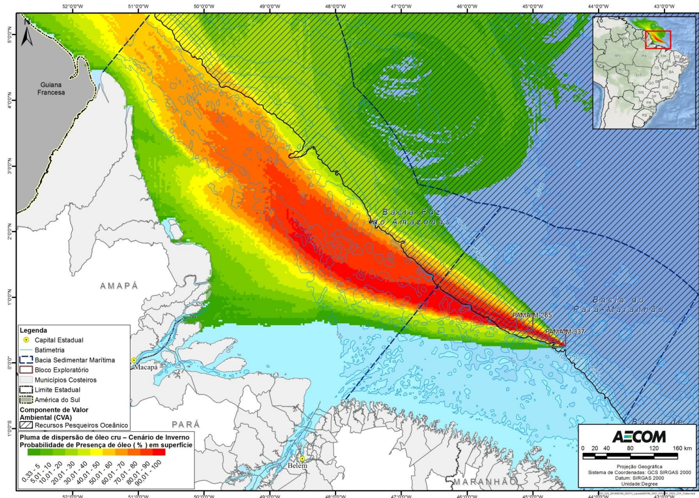
FIGURA II.9.4.2.8 – Área de concentração de recursos pesqueiros oceânicos na área com probabilidades de chegada de óleo, no cenário de inverno, pior caso.
