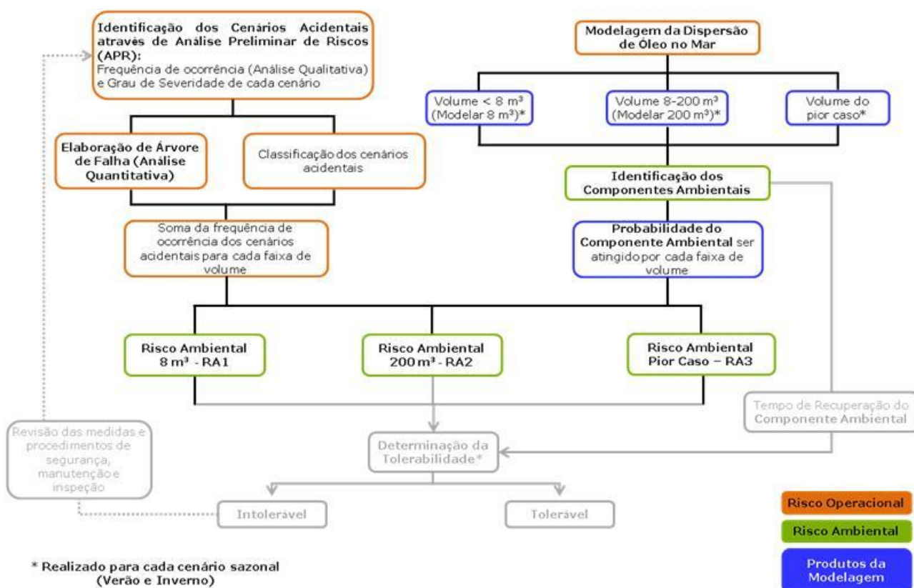
FIGURA II.9.6 – Fluxograma com as etapas para o cálculo do Risco Ambiental.
