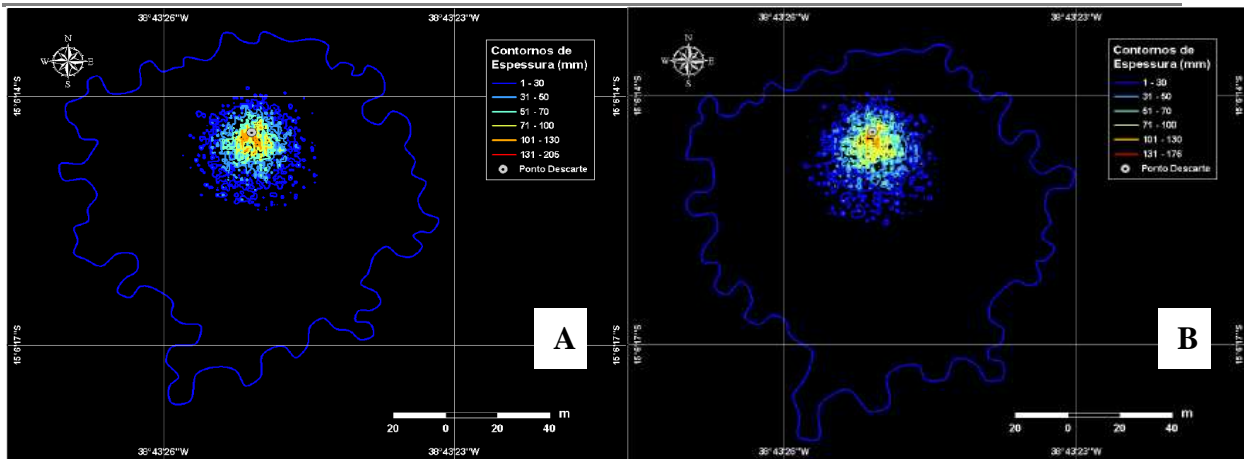
Figura II.6-1 – Resultados da simulação do descarte de cascalhos na Fase I, nos períodos de verão (A) e inverno (B), mostrando áreas de abrangência e espessuras médias da camada de deposição (até o ponto de corte de 1mm), no entorno do Lead F2, Bloco BM-J-1.
