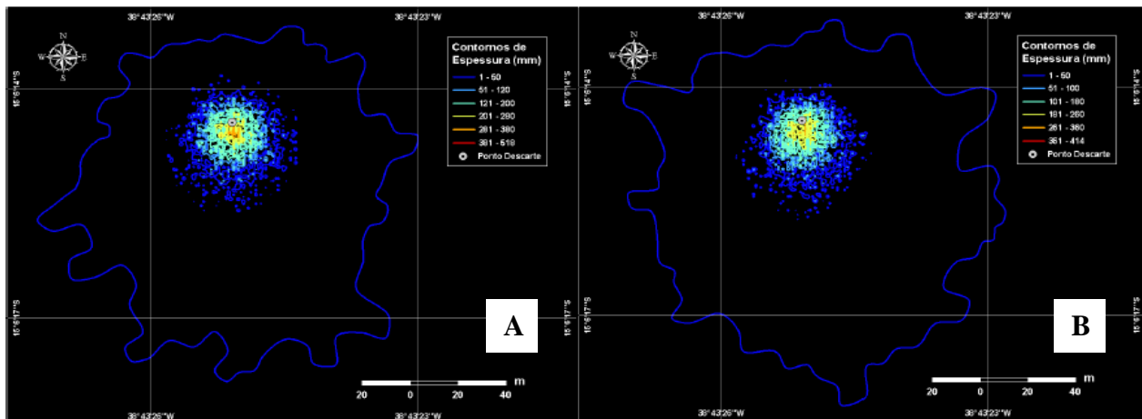
Figura II.6-2 - Resultados da simulação do descarte de cascalhos na Fase II, nos períodos de verão (A) e inverno (B), mostrando áreas de abrangência e espessuras médias da camada de deposição (até o ponto de corte de 1mm), no entorno do Lead F2, Bloco BM-J-1.
