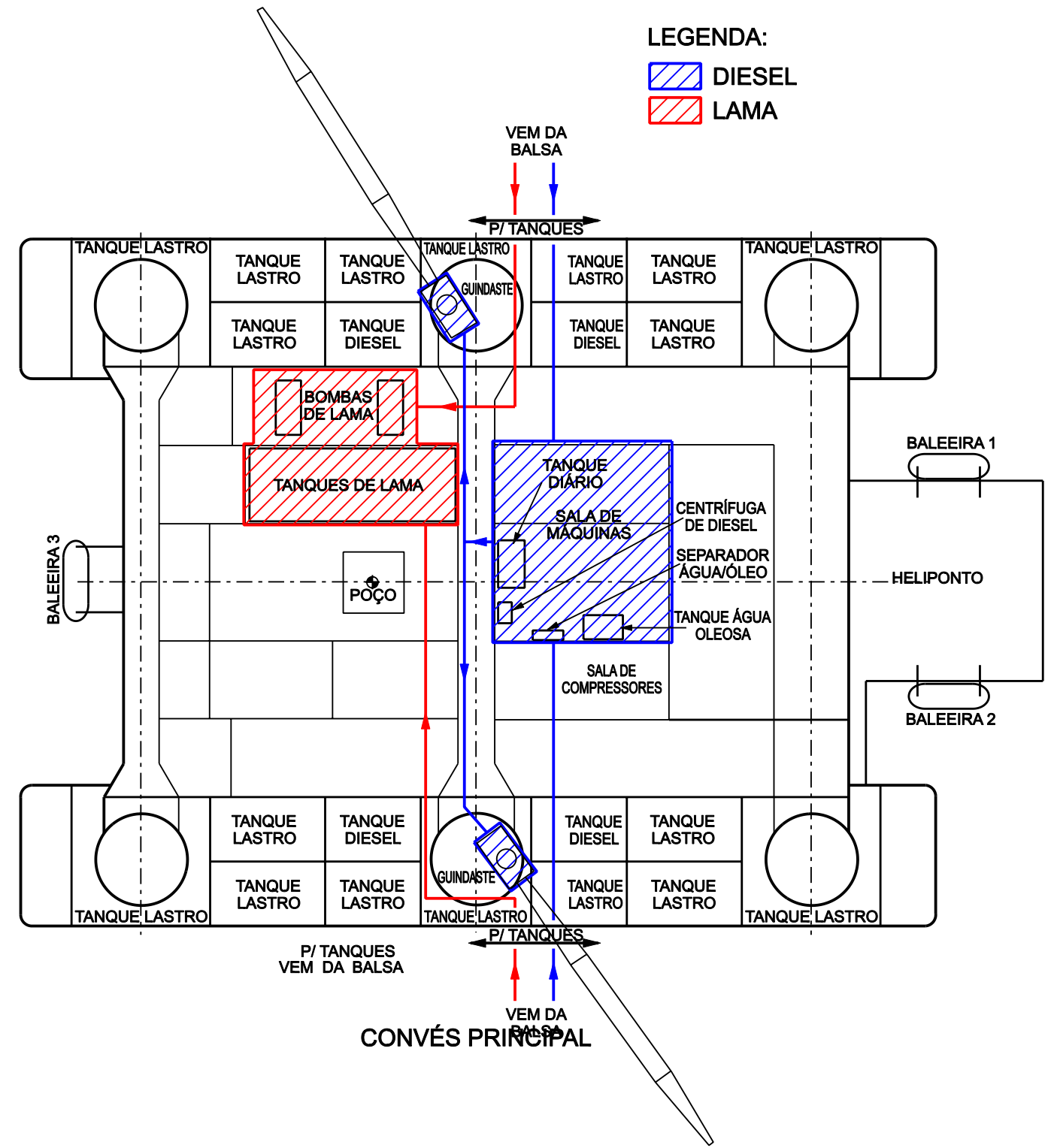
FLUIDO DE PERFURAÇÃO E SISTEMA DE ÓLEO DIESEL
