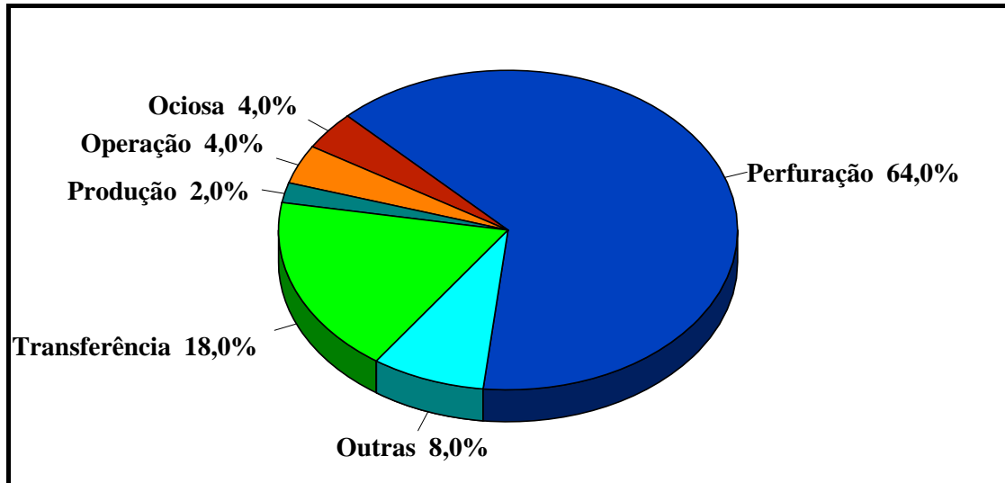
Figura II.1.1.1-1 - Distribuição do número de acidentes/incidentes vs Modo de operação. Somente navios de perfuração.
