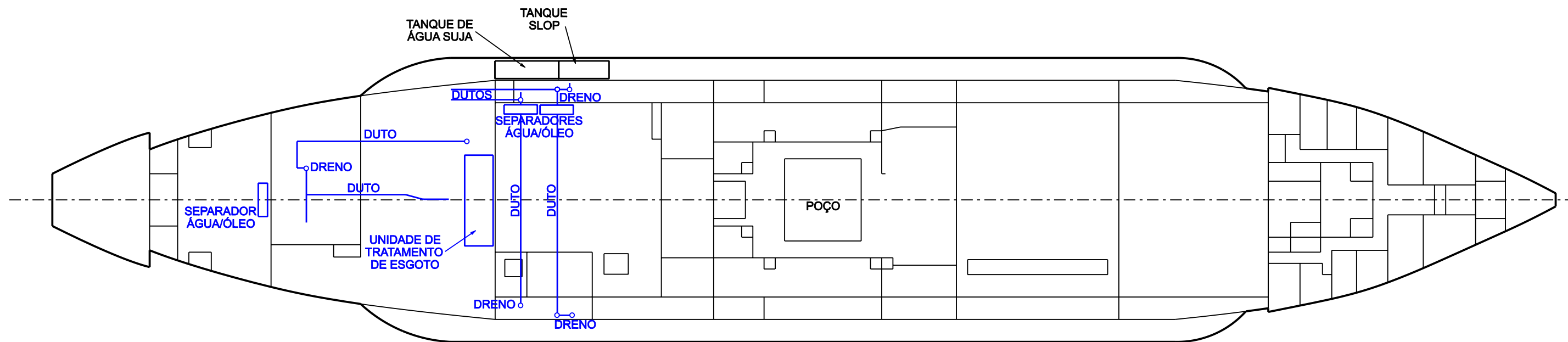
TERCEIRO CONVÉS
