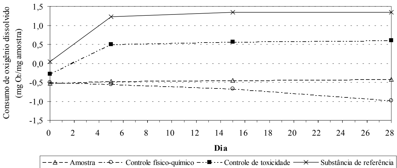
Figura 1 - Consumo líquido de oxigênio dissolvido das soluções preparadas para o Teste de Biodegradabilidade em Água Marinha para o produto FLUIDO DE PERFURAÇÃO BR-MUL - CÓD. 1.10 .
