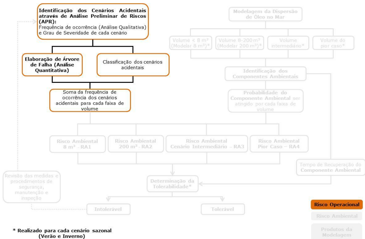
FIGURA II.12.3 – Etapas para o cálculo do Risco Operacional.
