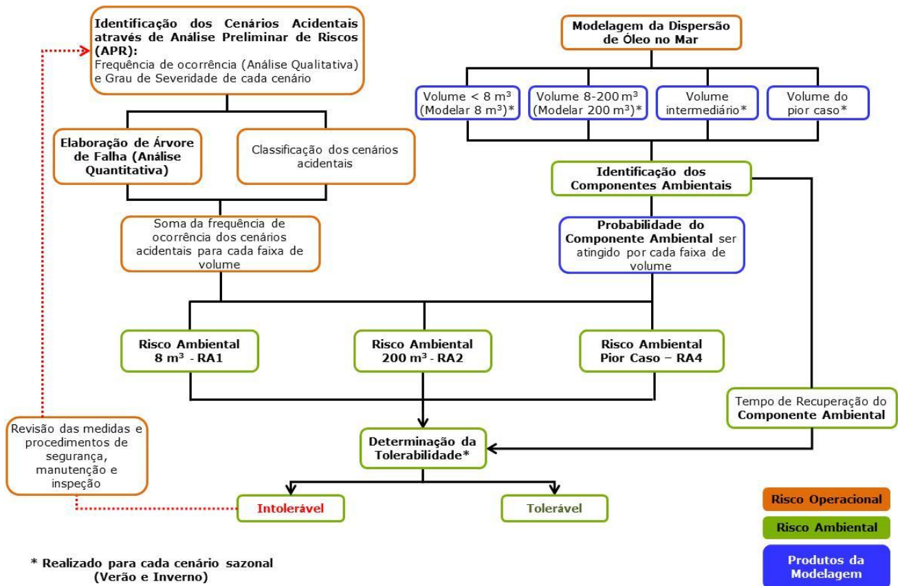
FIGURA II.12.7 – Fluxograma com as etapas para o cálculo do Risco Ambiental e da Relação Tempo de Recuperação/Tempo de Ocorrência.
