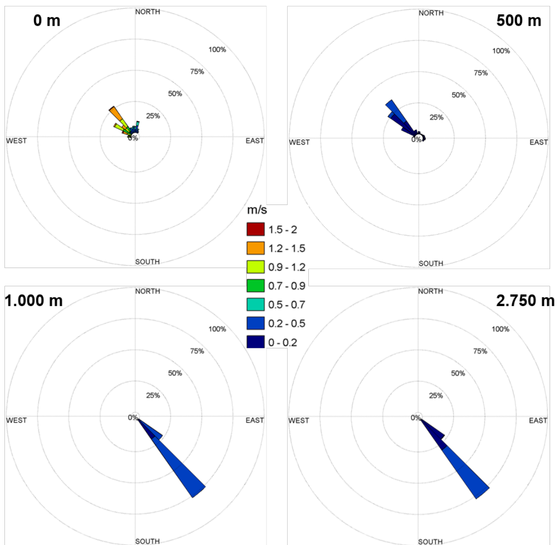
Figura 25: Histogramas direcionais de corrente nas profundidades de 0, 500, 1.000 e 2.750 metros, para o período representativo do cenário determinístico de espessura máxima, do ponto de grade do ROMS mais próximo ao poço.
