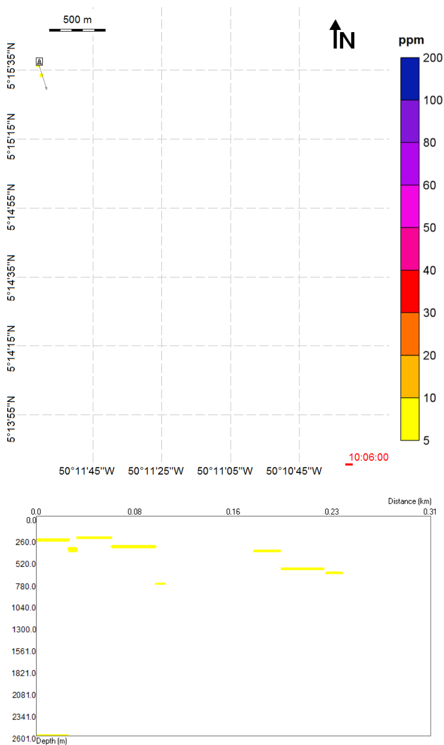
Figura 40: Concentração de sólidos na coluna d'água após 10 dias e 6 h do início do descarte: visão em planta (painel superior) e em perfil de 0,27 km com orientação NW-SE (painel inferior). Caso determinístico – distância máxima. ( Datum SIRGAS 2000).
