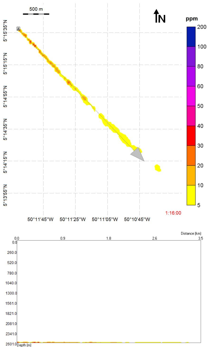
Figura 39: Concentração de sólidos na coluna d'água após 1 dia e 16 h do início do descarte: visão em planta (painel superior) e em perfil de 3,5 km com orientação NW-SE (painel inferior). Caso determinístico – distância máxima. ( Datum SIRGAS 2000).
