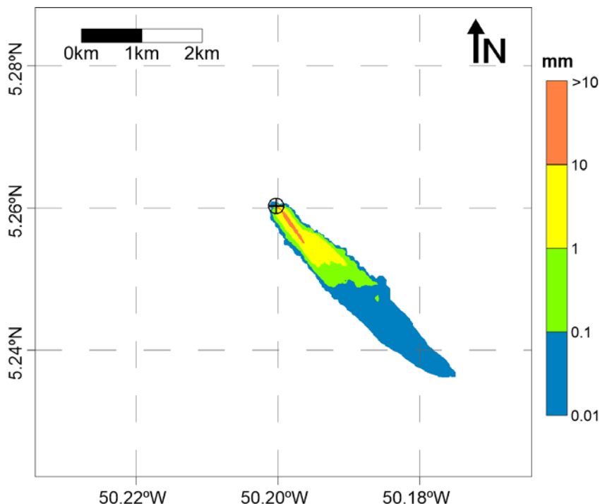
Figura 29: Pilha resultante da integração de todas as seções, considerando o limiar de 0,01 mm. Caso determinístico – espessura máxima. ( Datum SIRGAS 2000).
