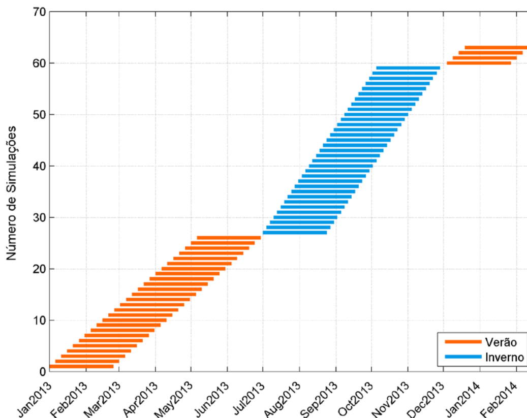
Figura 5: Número de simulações realizadas por período do ano. Cada barra colorida reflete uma simulação distinta com duração de 55 dias (tempo total de simulação). Em laranja, são apresentadas as 30 simulações determinísticas realizadas para o verão e, em azul, as 33 simulações determinísticas realizadas para o inverno.
