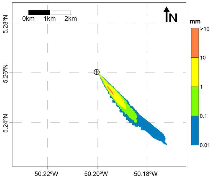
Figura 32: Pilha resultante da integração de todas as seções, considerando o limiar de 0,01 mm. Caso determinístico – distância máxima. ( Datum SIRGAS 2000).
