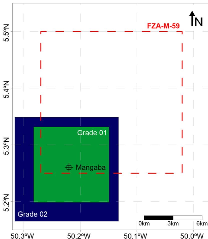
Figura 6: Domínios das grades utilizadas na modelagem para as pilhas de deposição (Grade 01 – em verde); e para as plumas de sólidos em suspensão (Grade 02 – em azul). (Datum SIRGAS 2000).
