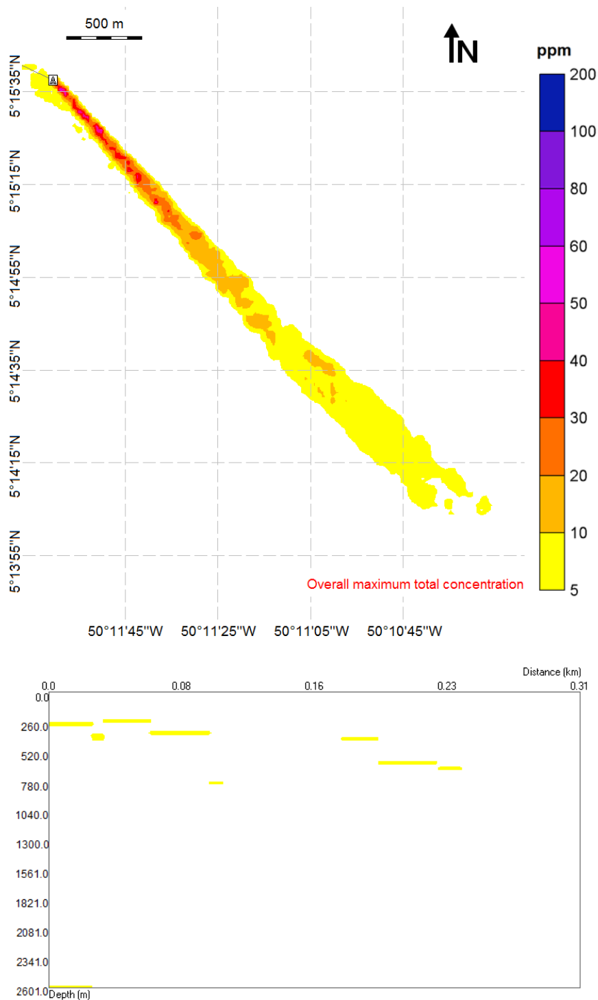
Figura 38: Concentração máxima de sólidos na coluna d'água considerando todo o período de simulação e todos os descartes: visão em planta (painel superior) e em perfil de 0,31 km com orientação SE- NW (painel inferior). Caso determinístico – distância máxima. ( Datum SIRGAS 2000).
