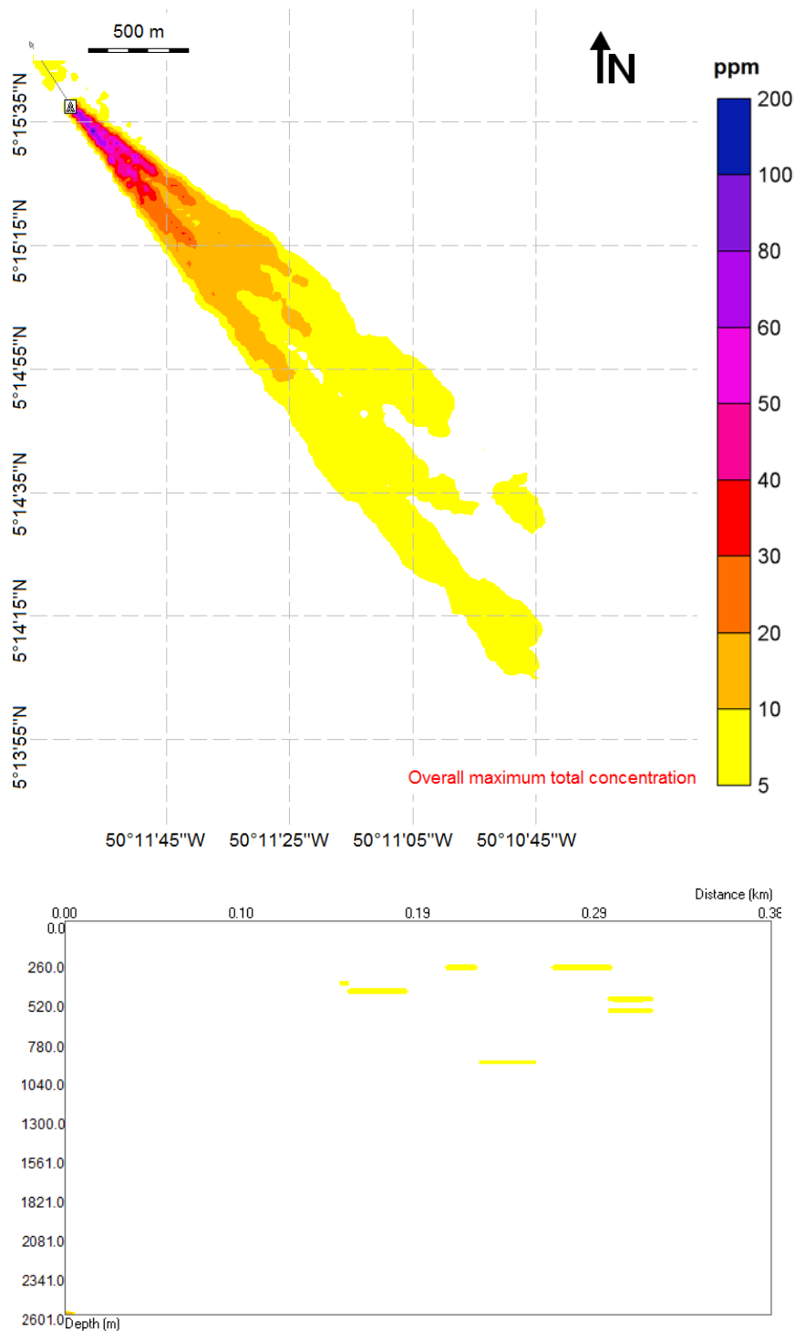
Figura 34: Concentração máxima de sólidos na coluna d'água considerando todo o período de simulação e todos os descartes: visão em planta (painel superior) e em perfil de 0,38 km com orientação SE- NW (painel inferior). Caso determinístico – espessura máxima. (Datum SIRGAS 2000).
