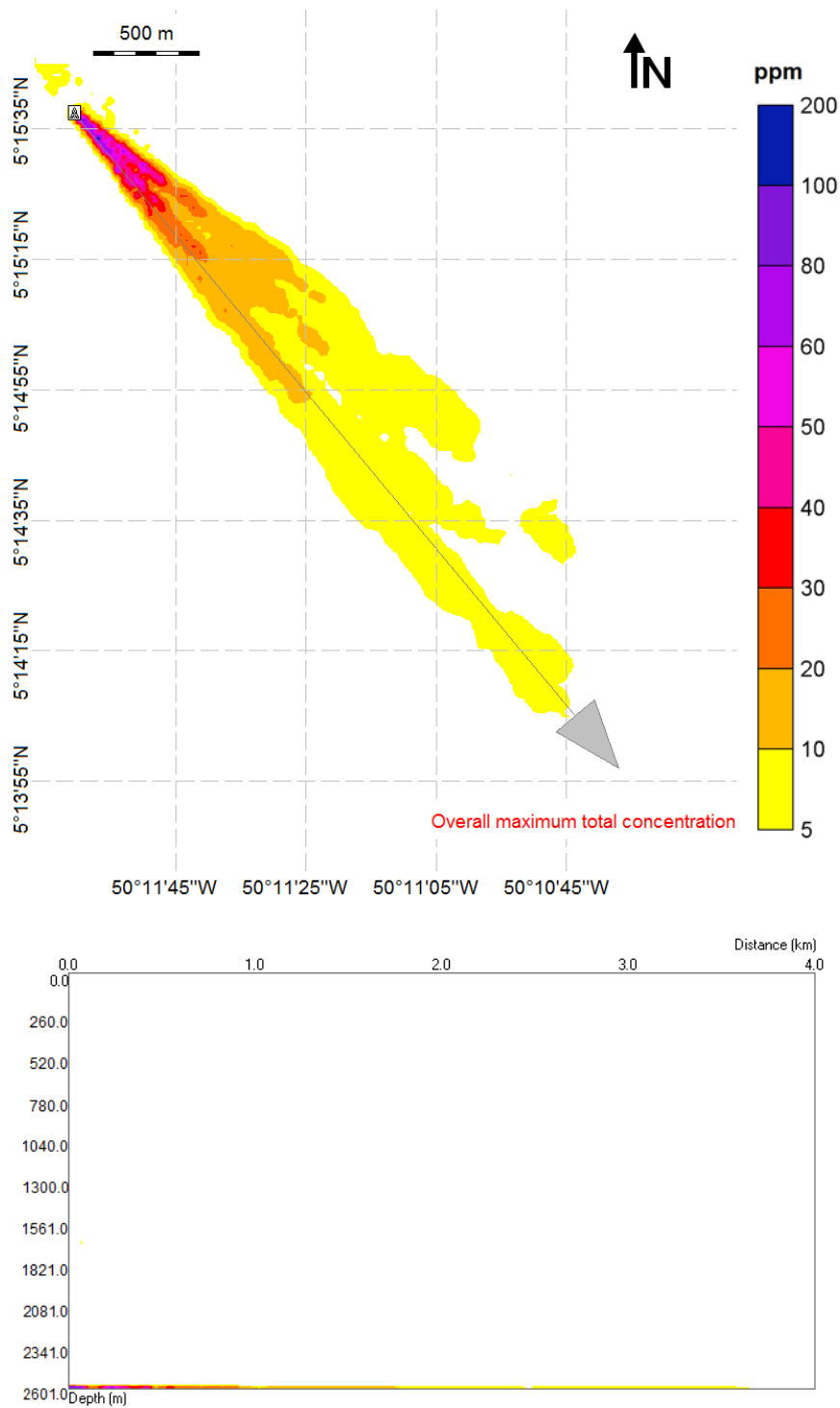
Figura 33: Concentração máxima de sólidos na coluna d'água considerando todo o período de simulação e todos os descartes: visão em planta (painel superior) e em perfil de 4 km com orientação NW-SE (painel inferior). Caso determinístico – espessura máxima. (Datum SIRGAS 2000).
