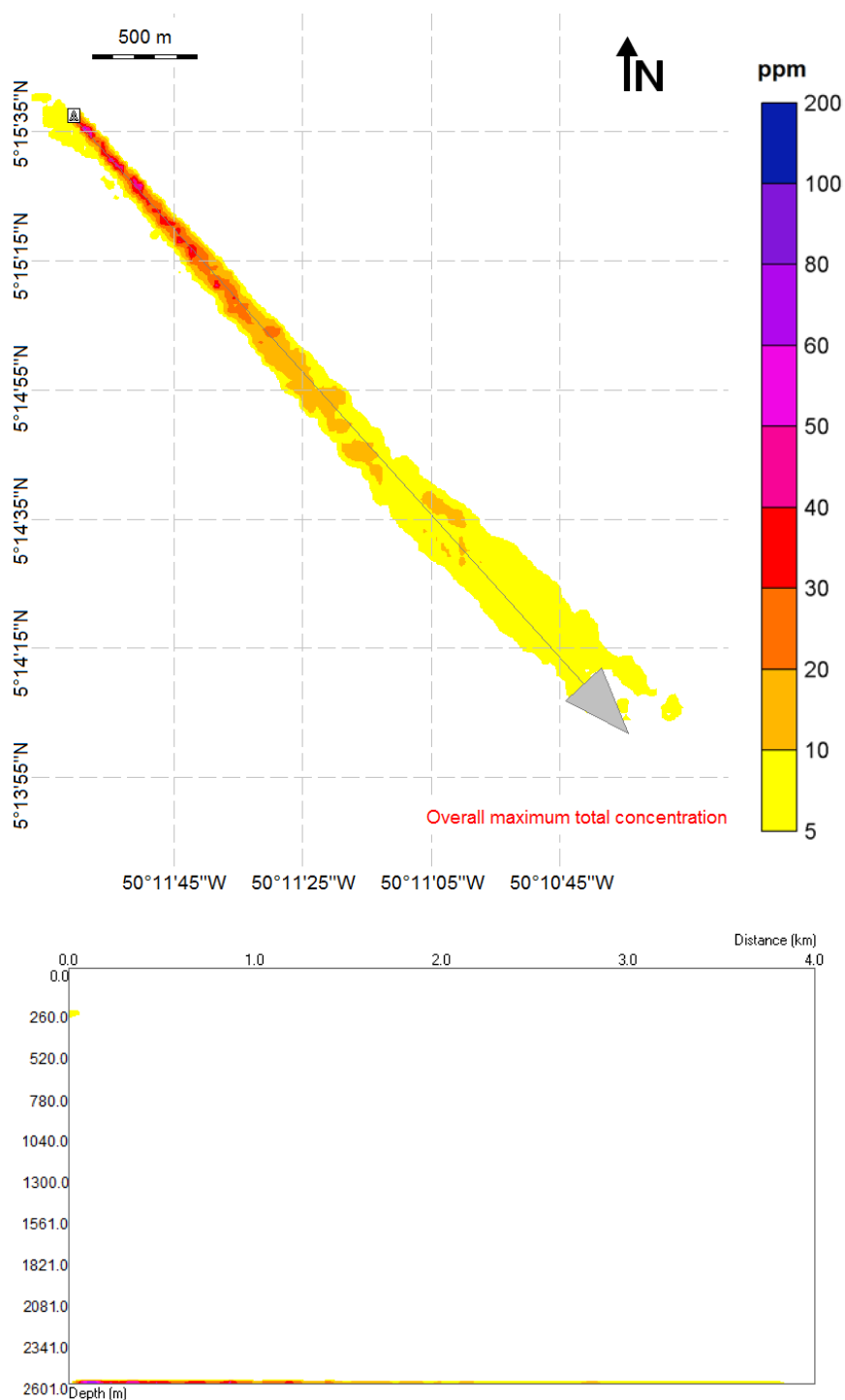
Figura 37: Concentração máxima de sólidos na coluna d'água considerando todo o período de simulação e todos os descartes: visão em planta (painel superior) e em perfil de 4 km com orientação NW-SE (painel inferior). Caso determinístico – distância máxima. ( Datum SIRGAS 2000).
