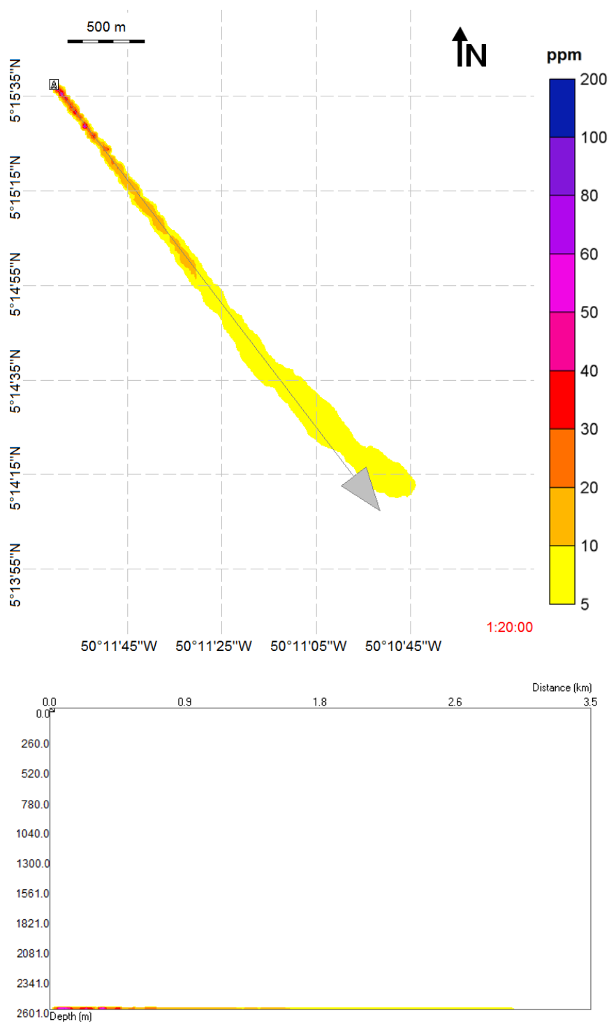
Figura 35: Concentração de sólidos na coluna d'água após 1 dia e 20 h do início do descarte: visão em planta (painel superior) e em perfil de 3,5 km com orientação NW-SE (painel inferior). Caso determinístico – espessura máxima. (Datum SIRGAS 2000).
