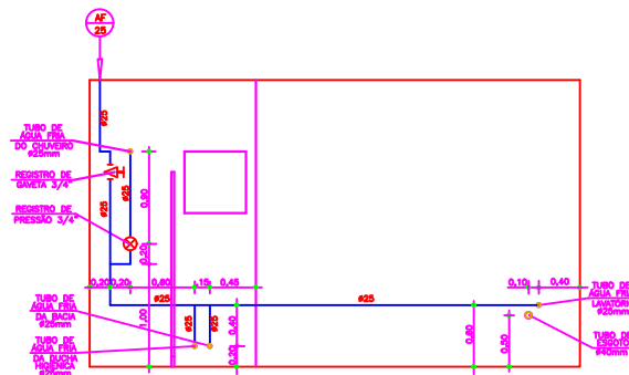
DETALHE DE ÁGUA FRIA DO VESTIÁRIO MASCULINO ESCALA 1:25
