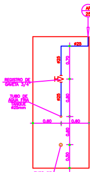
DETALHE DE ÁGUA FRIA DO DML ESCALA 1:25
