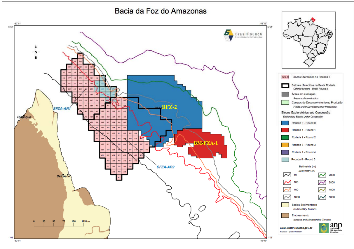
FIGURA II.6.2.11-10 – Localização dos Blocos BFZ-2 e BM-FZA-1, destacados em azul e vermelho respectivamente, na Bacia da Foz do Amazonas.
