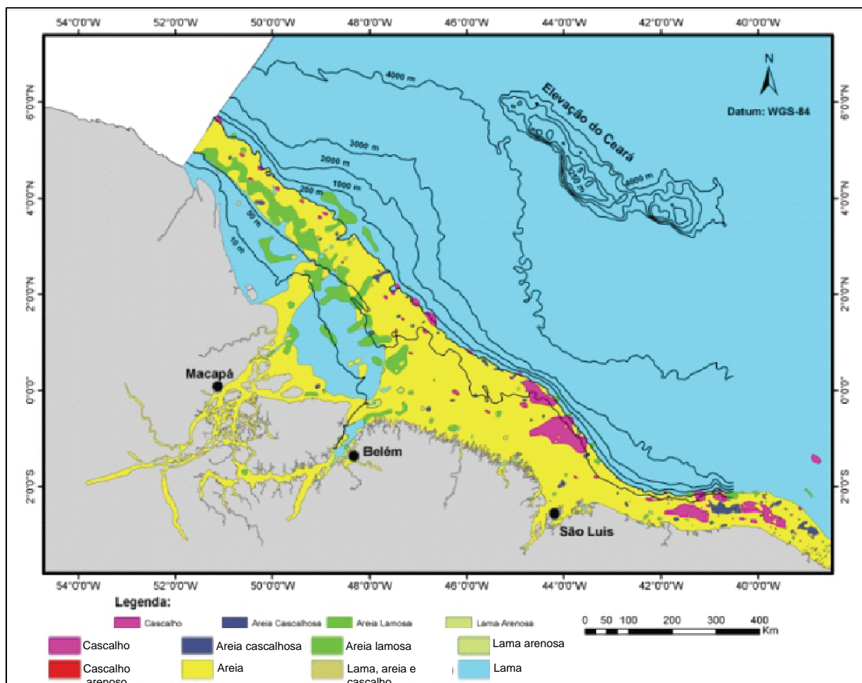
FIGURA II.6.2.11-1 – Mapa da distribuição sedimentar na costa norte do Brasil, segundo a classificação de Shepard.
