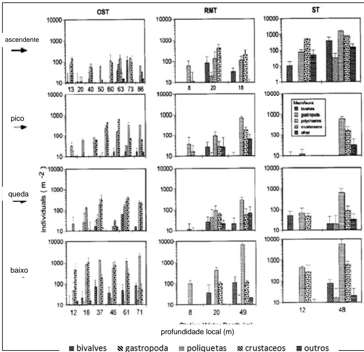
FIGURA II.6.2.11-8 – Densidade dos grupos taxonômicos da macrofauna nos períodos de enchente, cheia, vazante e mínima descarga do rio Amazonas, nos transects (OST, RMT e ST), registrados durante o cruzeiro AmasSeds.
