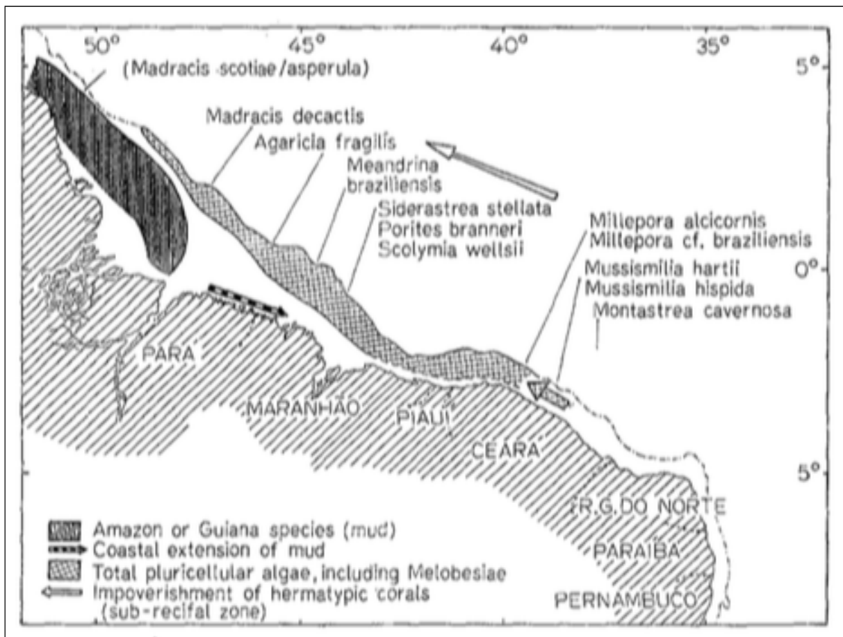
FIGURA II.6.2.11-4 – Algumas populações encontradas na margem equatorial brasileira.
