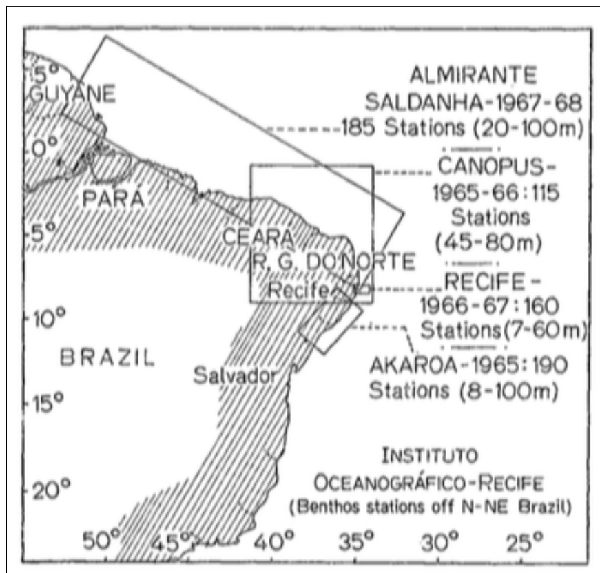
FIGURA II.6.2.11-3 – Malha Amostral das campanhas realizadas na margem equatorial pelo Instituto Oceanográfico de Recife, cujos dados foram analisados por KEMPF (1970).
