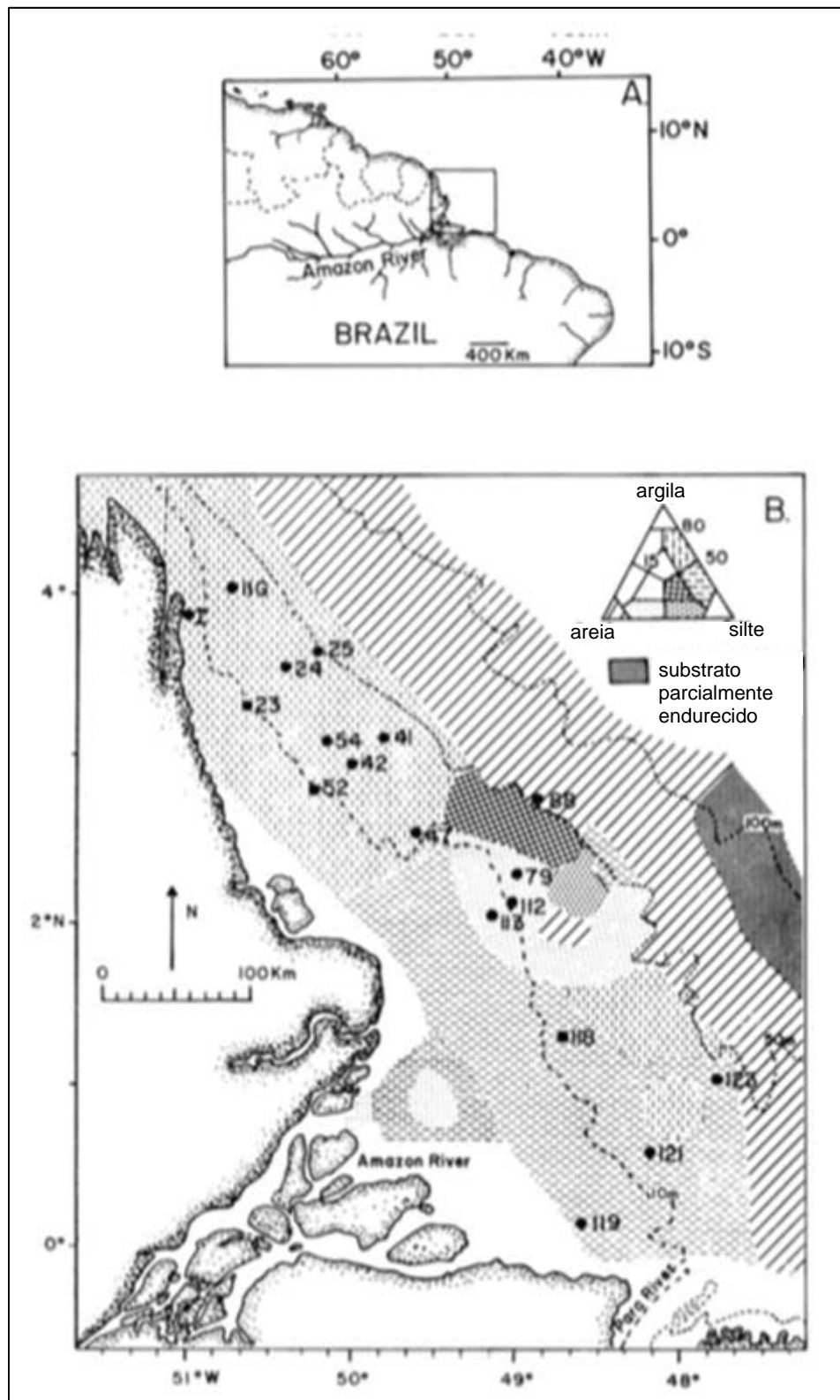
FIGURA II.6.2.11-5 – Malha Amostral realizada por Aller & Aller na margem equatorial pelo navio R.V. Ivelin em 1983, dentro do Projeto AmasSeds. Os tipos de sedimento encontrados na área estão destacados na figura.
