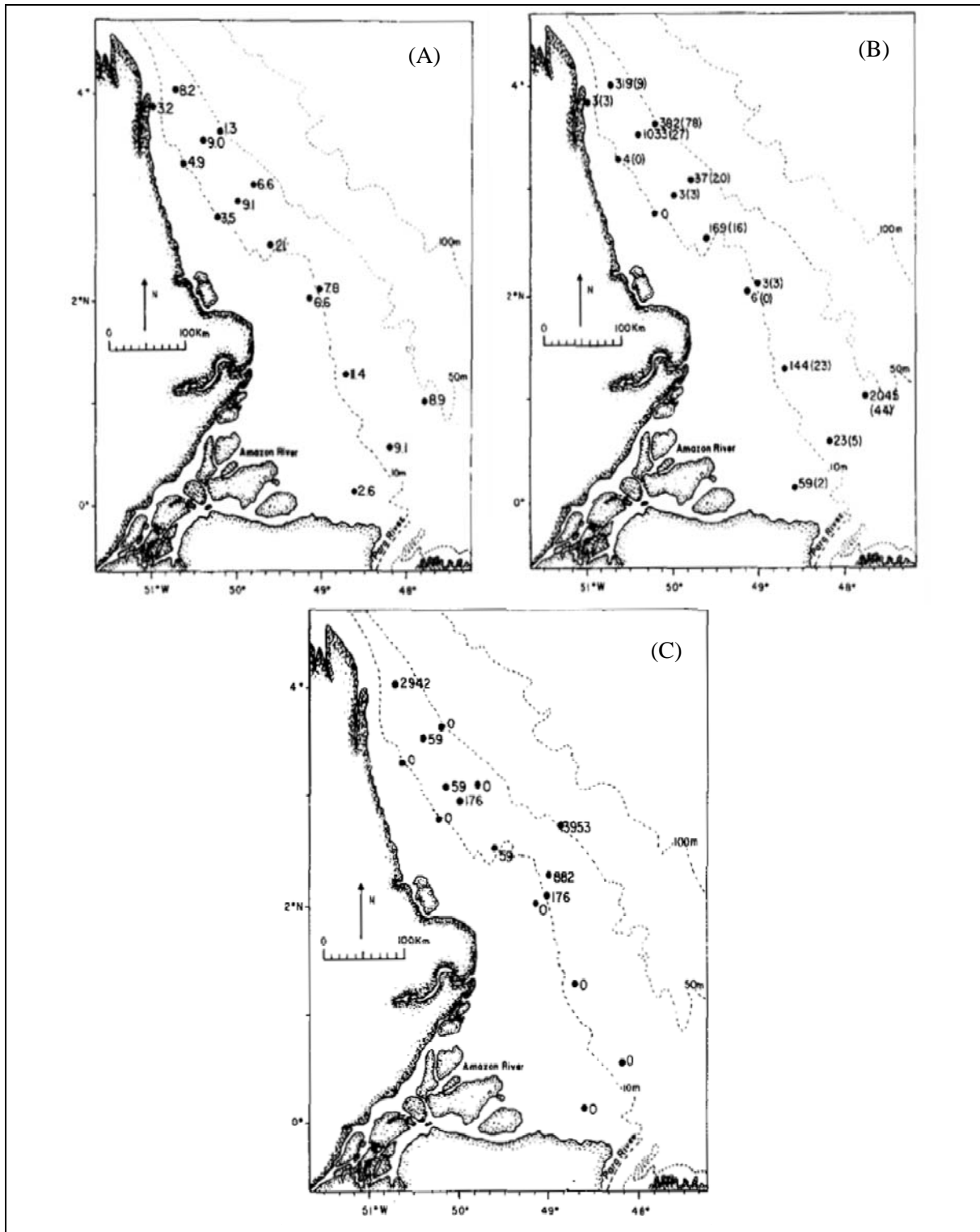
FIGURA II.6.2.11-6 – Distribuição da densidade bacteriana ( \times 10^9 \cdot g^{-1} ) nos primeiros 10cm do sedimento (A), meiofauna ( 10cm^2 ) nos 10 cm superficiais do sedimento (a não ser na estação 47 com 25cm de profundidade) (B) e macrofauna ( m^2 ) nos primeiros 20cm (C), nas estações.
