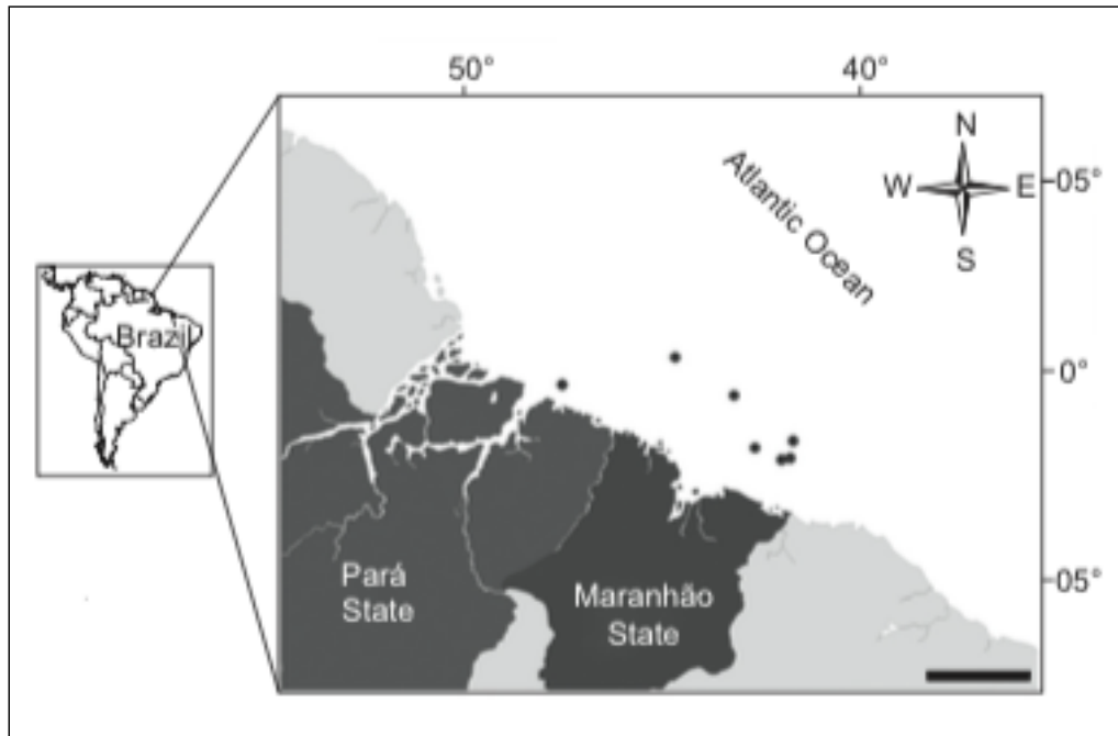
FIGURA II.6.2.11-9 – Malha Amostrada realizada pelo Programa REVIZEE, operações NORTE II, III e IV.
