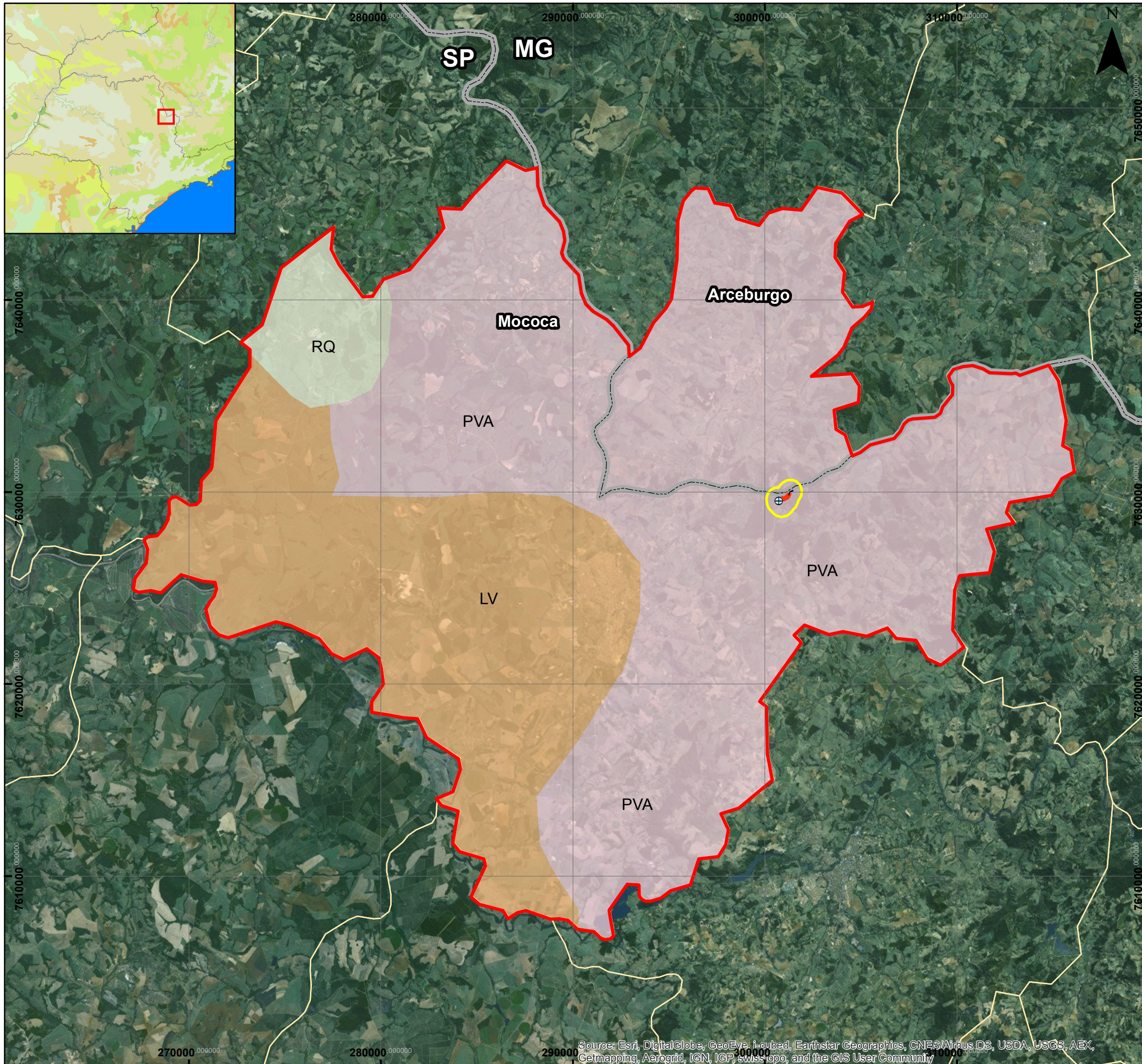
Figura 4.1.4.a Mapa Pedológico
