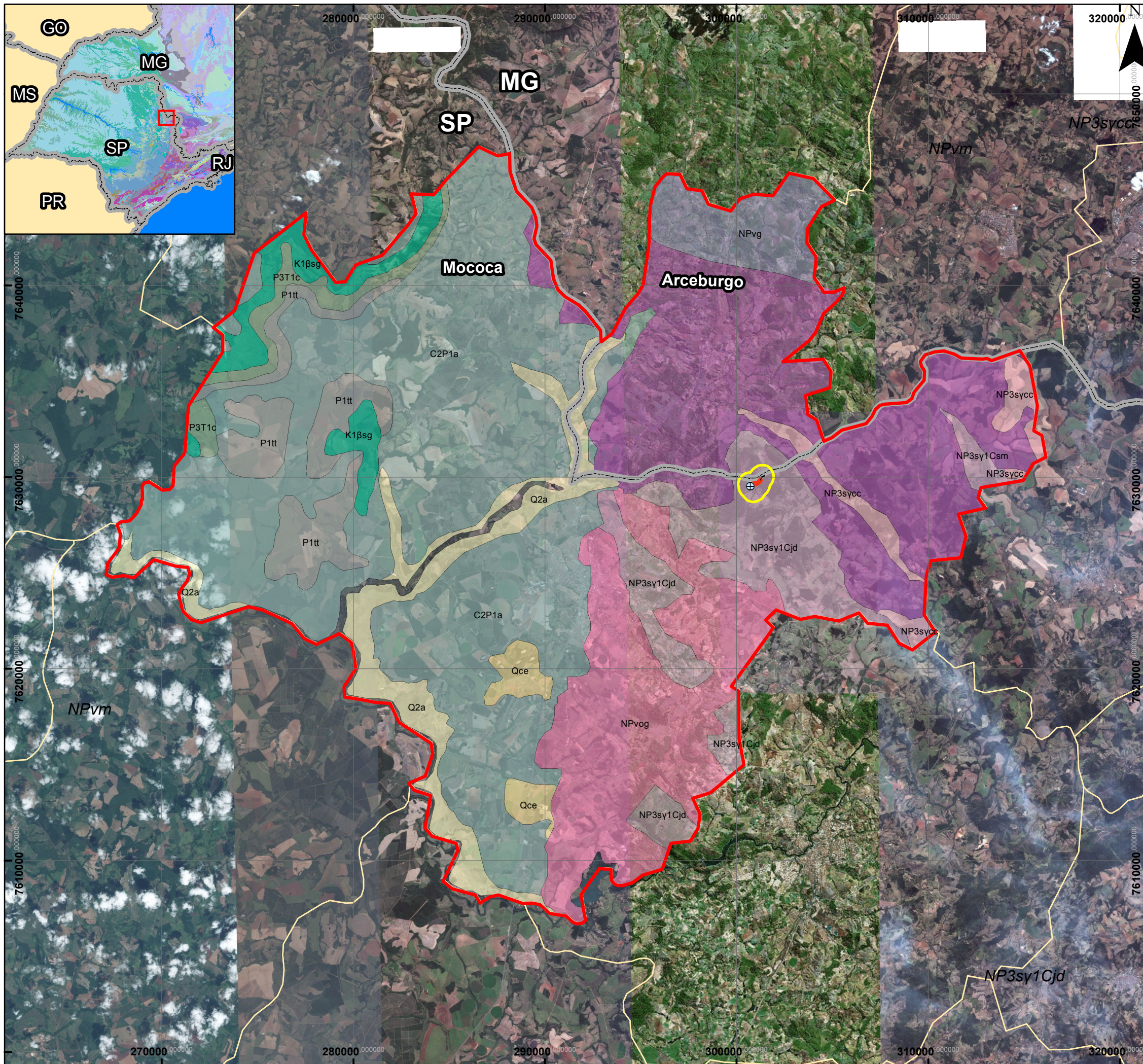
Figura 4.1.2.a Mapa Geológico
