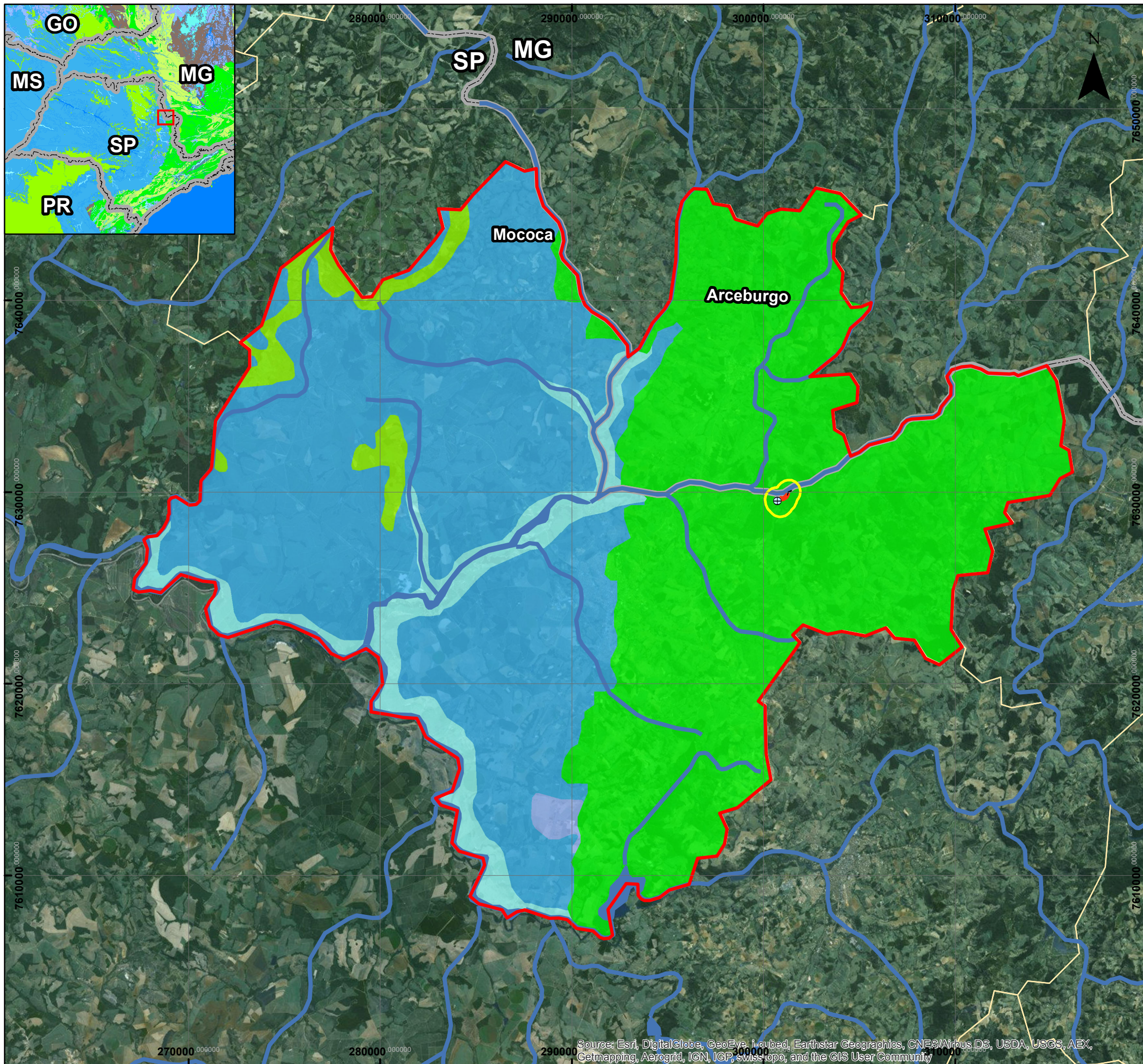
Figura 4.1.2.1.a Mapa Hidrogeológico
