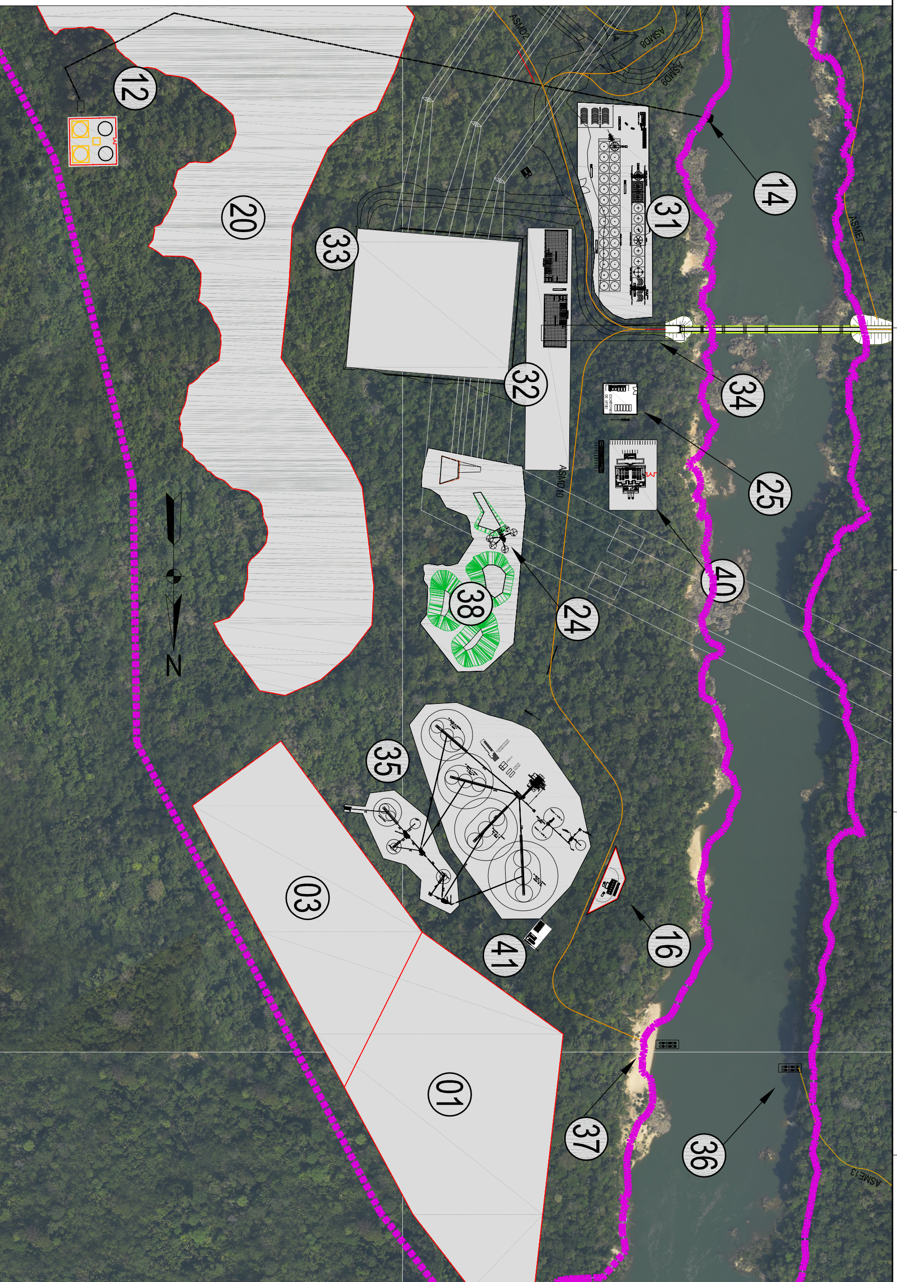
PLANTA (S/ ESCALA)
