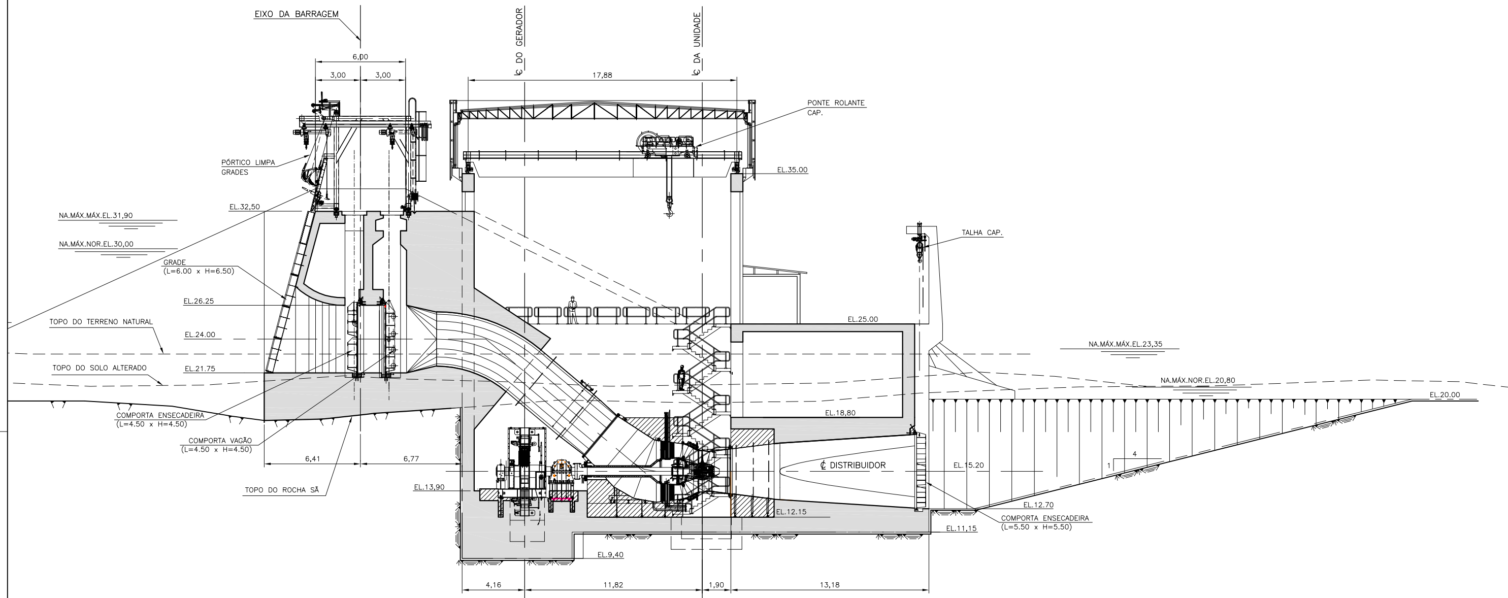
SEÇÃO TRANSVERSAL
