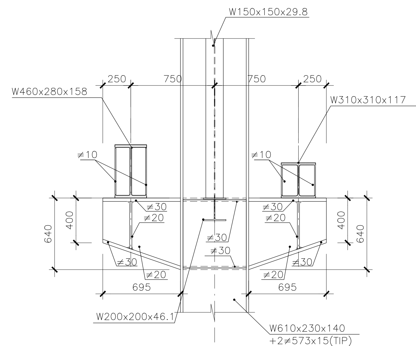
DETALHE 2 ESCALA 1:20
