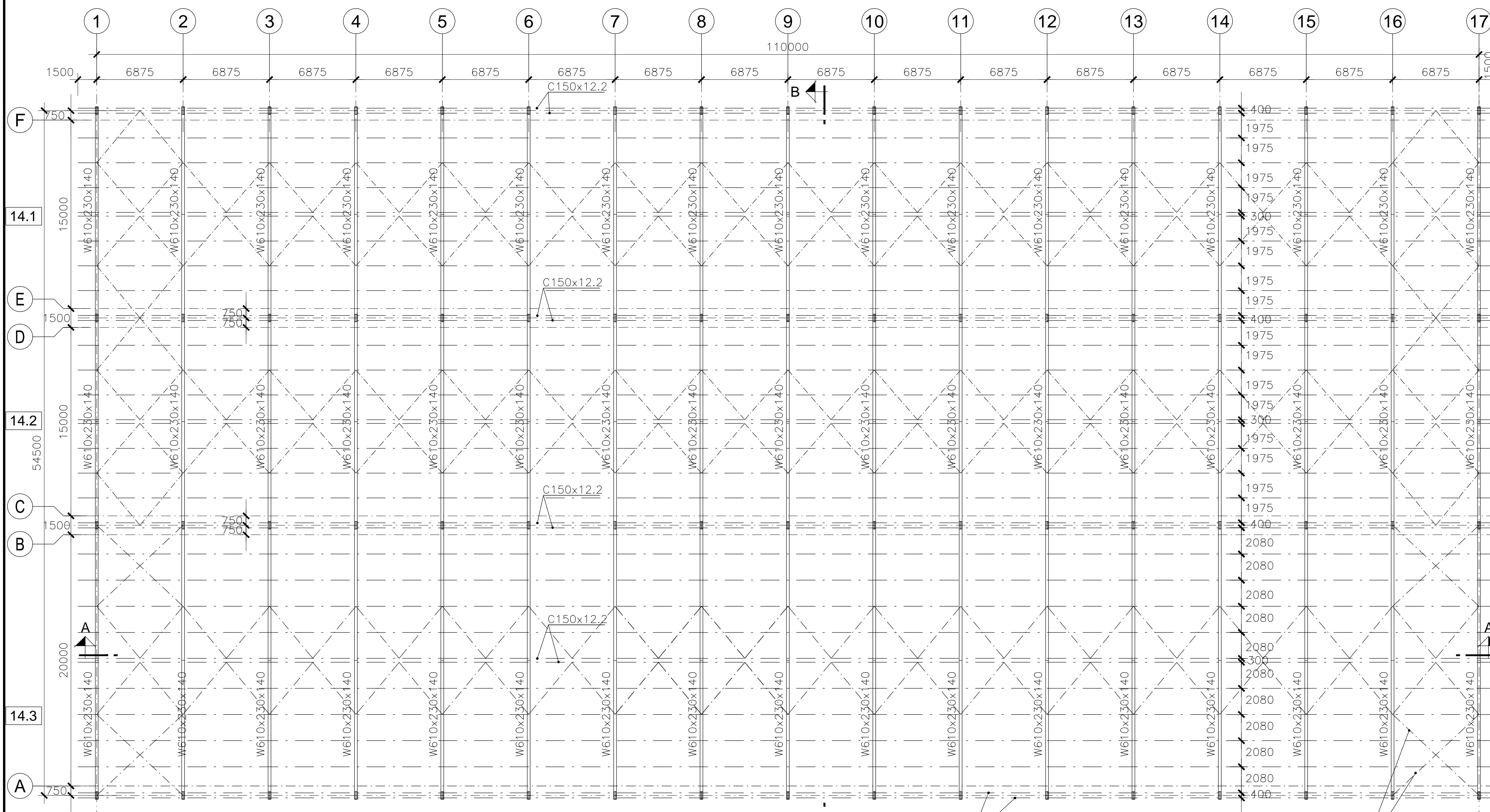
PLANTA DE COBERTURA ESCALA 1:200
