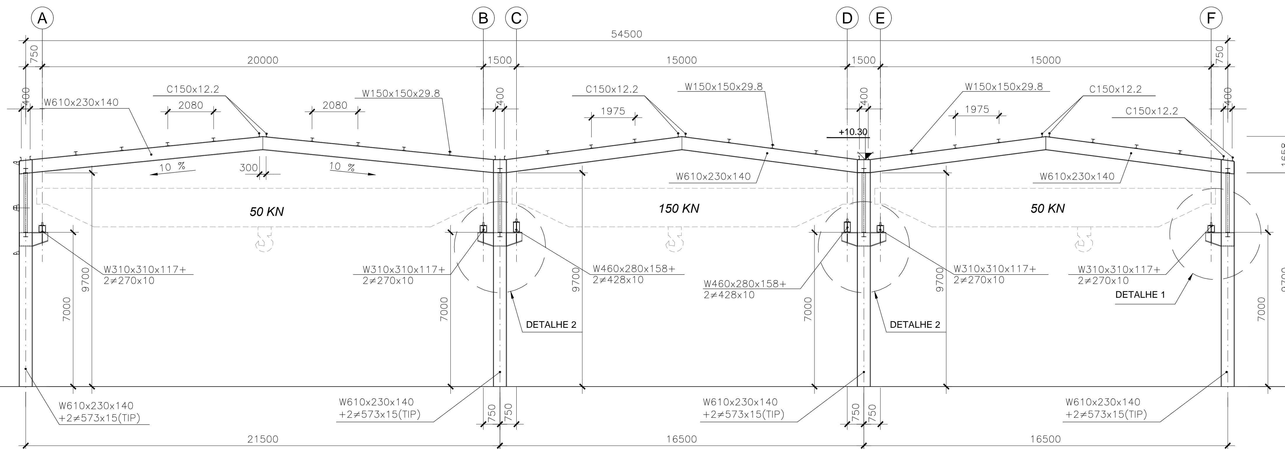
SEÇÃO B-B ESCALA 1:100
