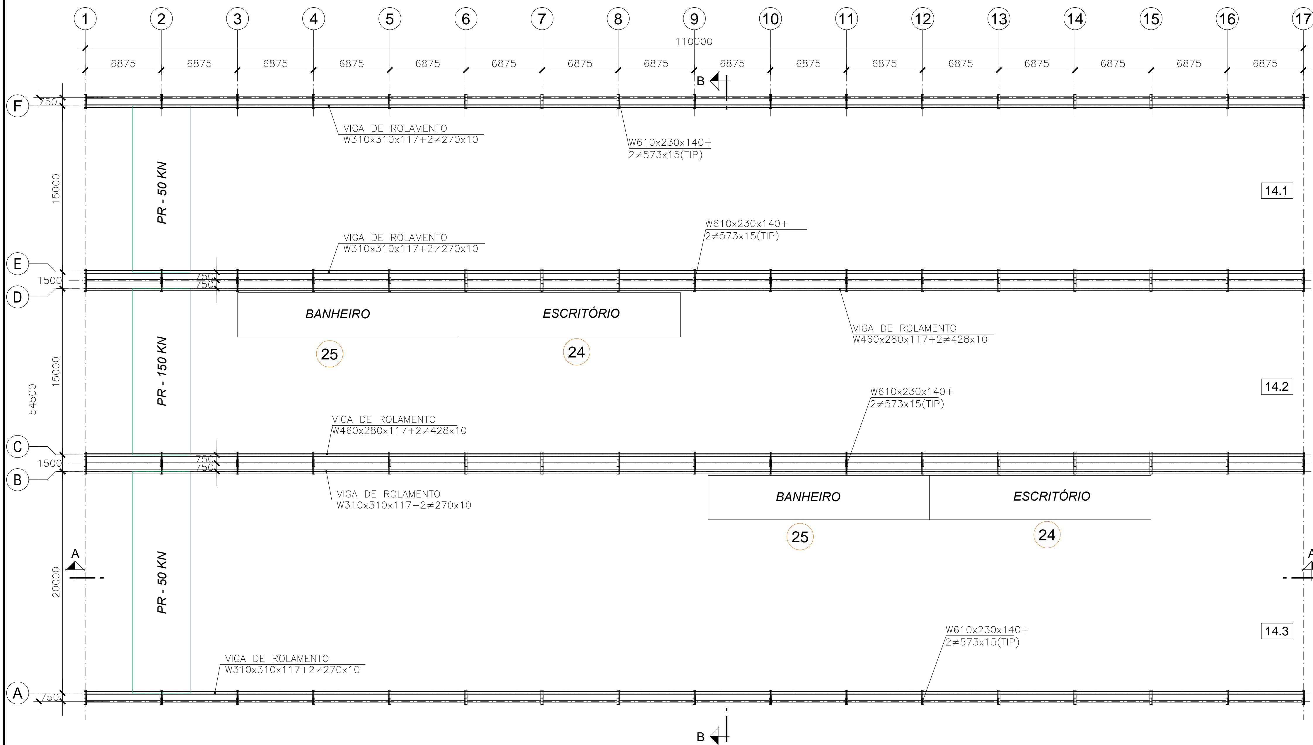
PLANTA VIGAS DE ROLAMENTO ESCALA 1:200
