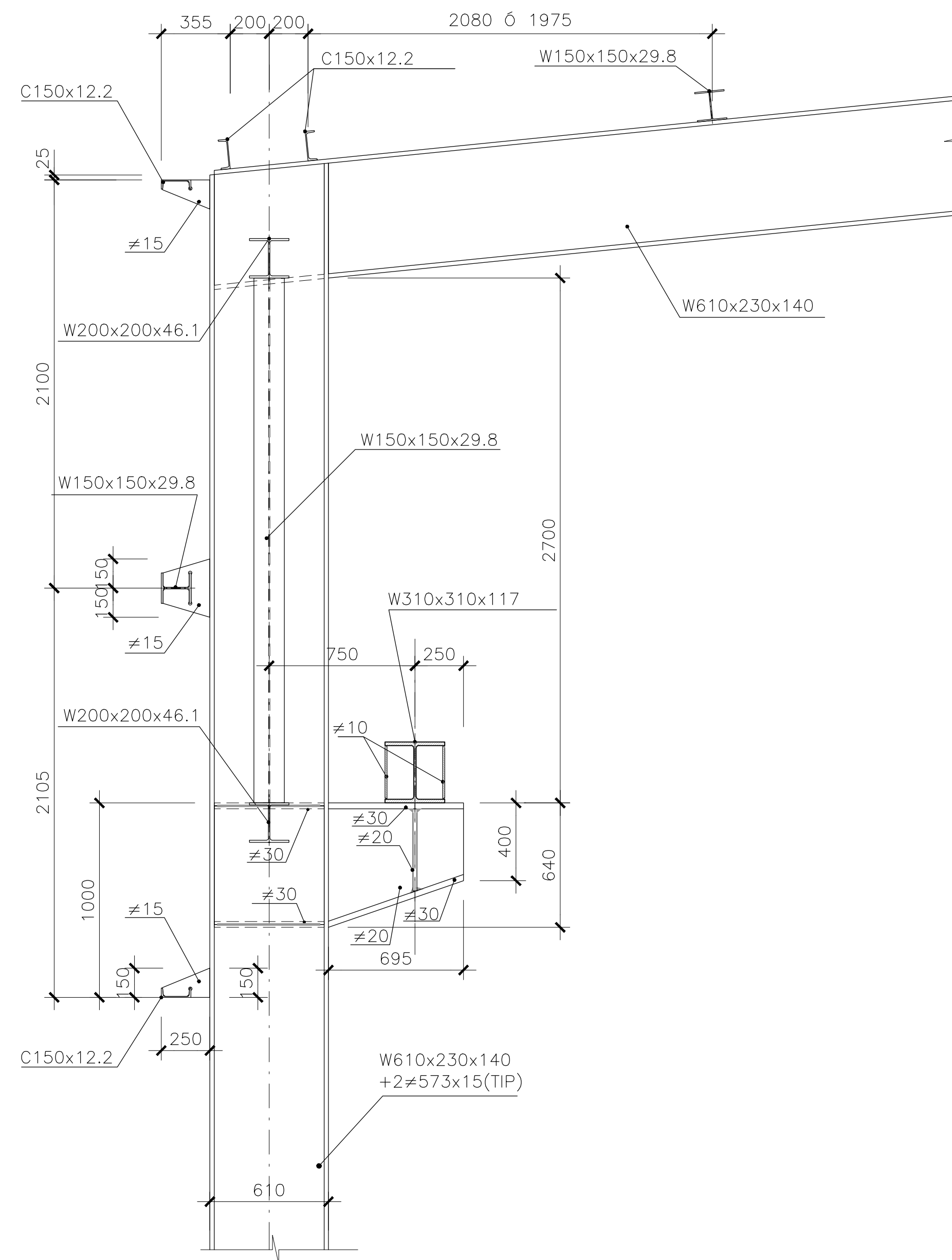
DETALHE 1 ESCALA 1:20
