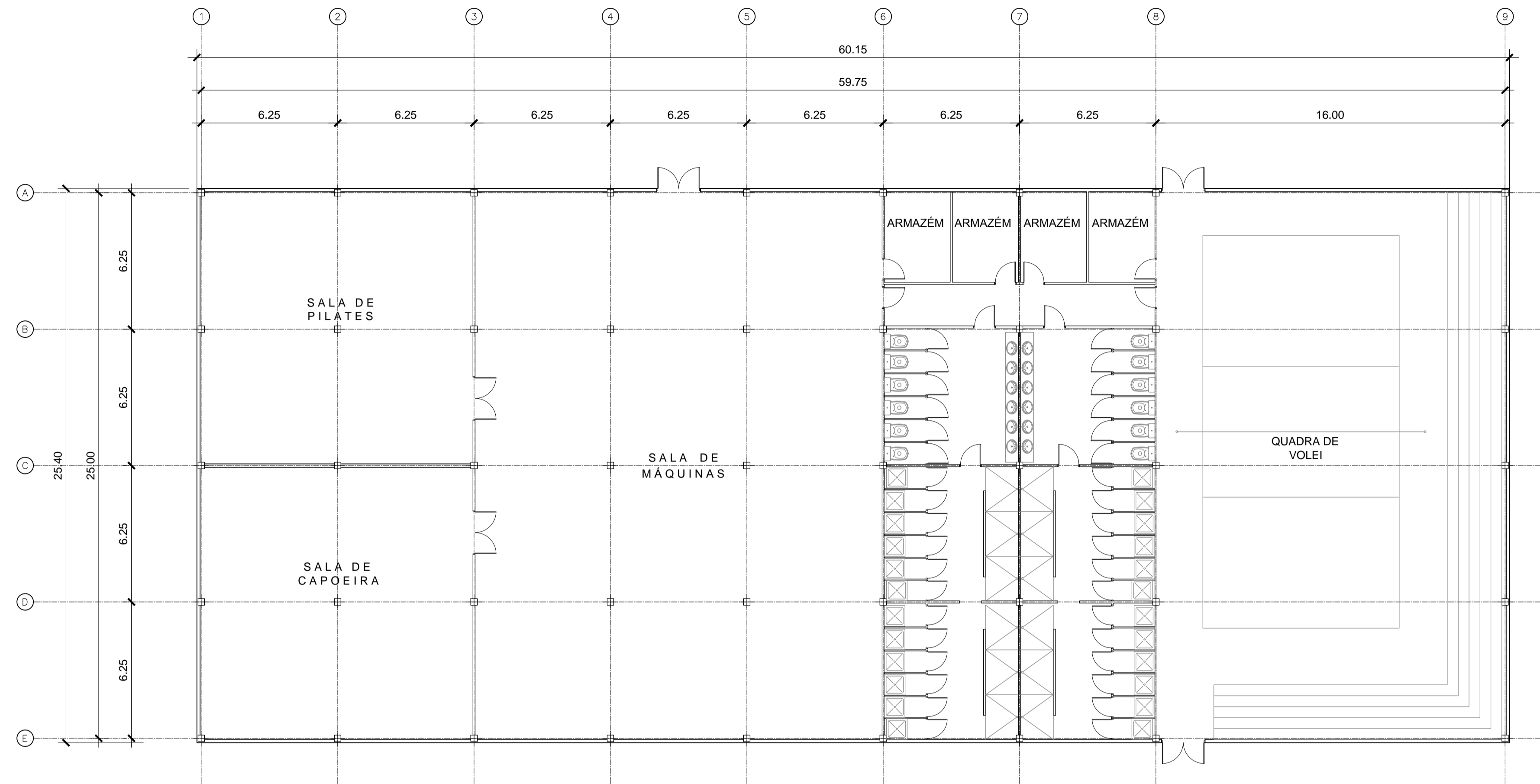
PLANTA ESCALA 1:150
