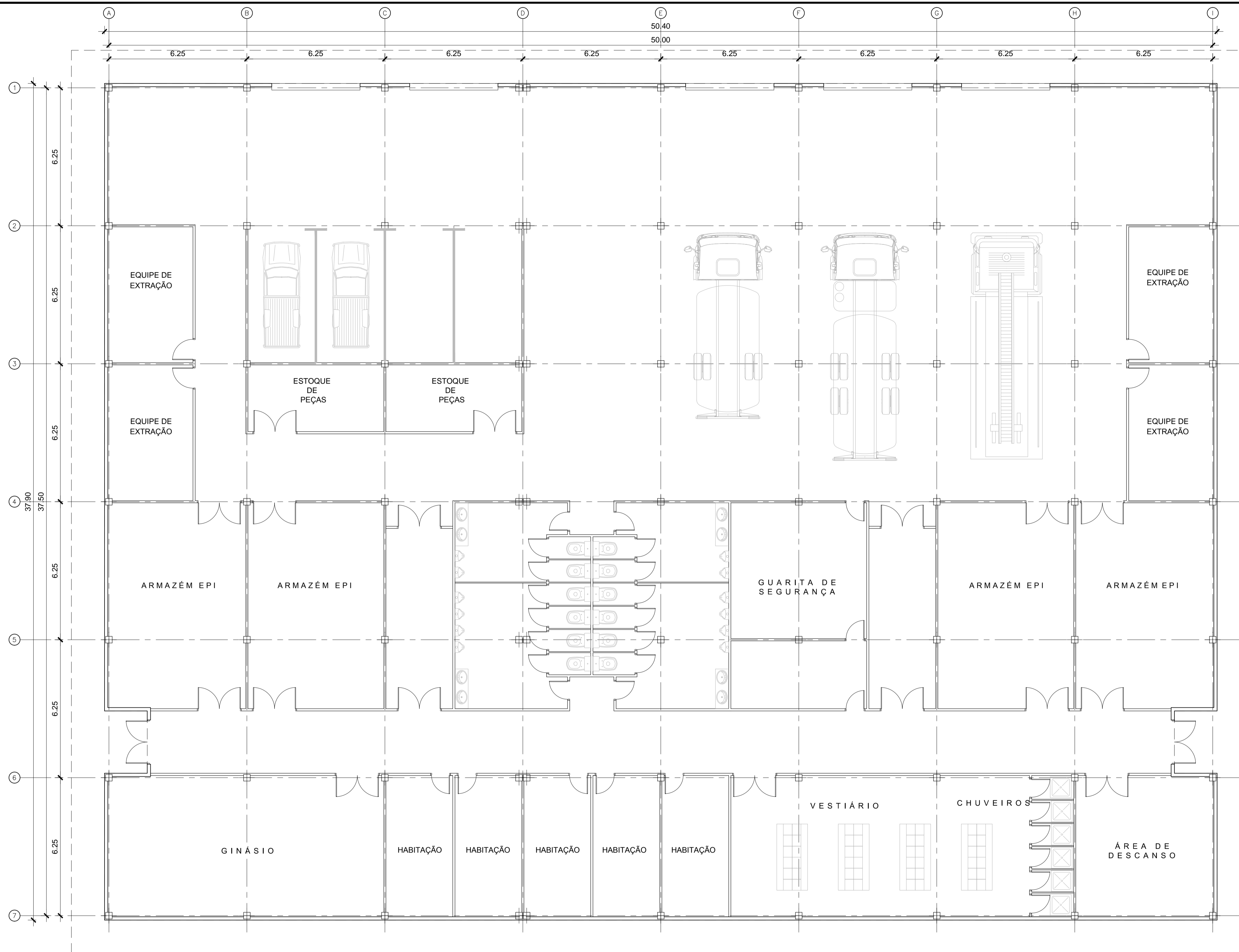
PISO TÉRREO ESCALA 1:200
