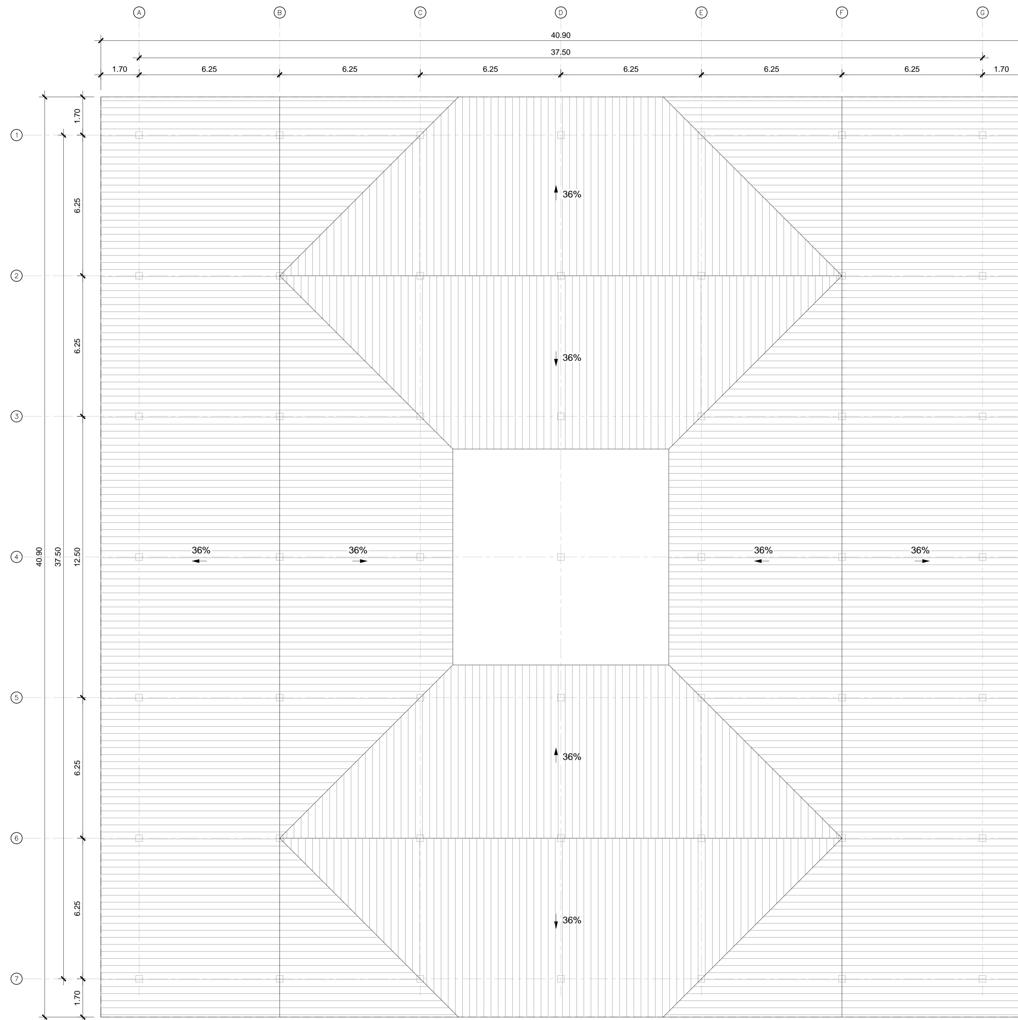
PLANTA DE COBERTURA-LAJE ESCALA 1:100
