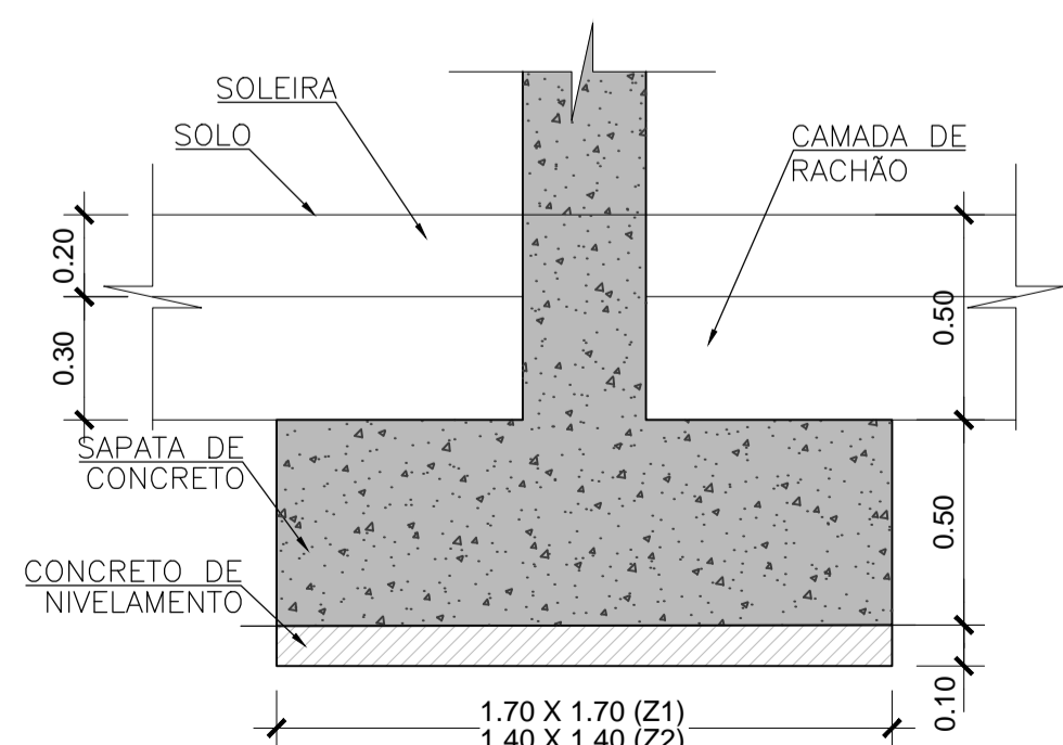
DETALHE FUNDAÇÃO ESCALA 1:20
