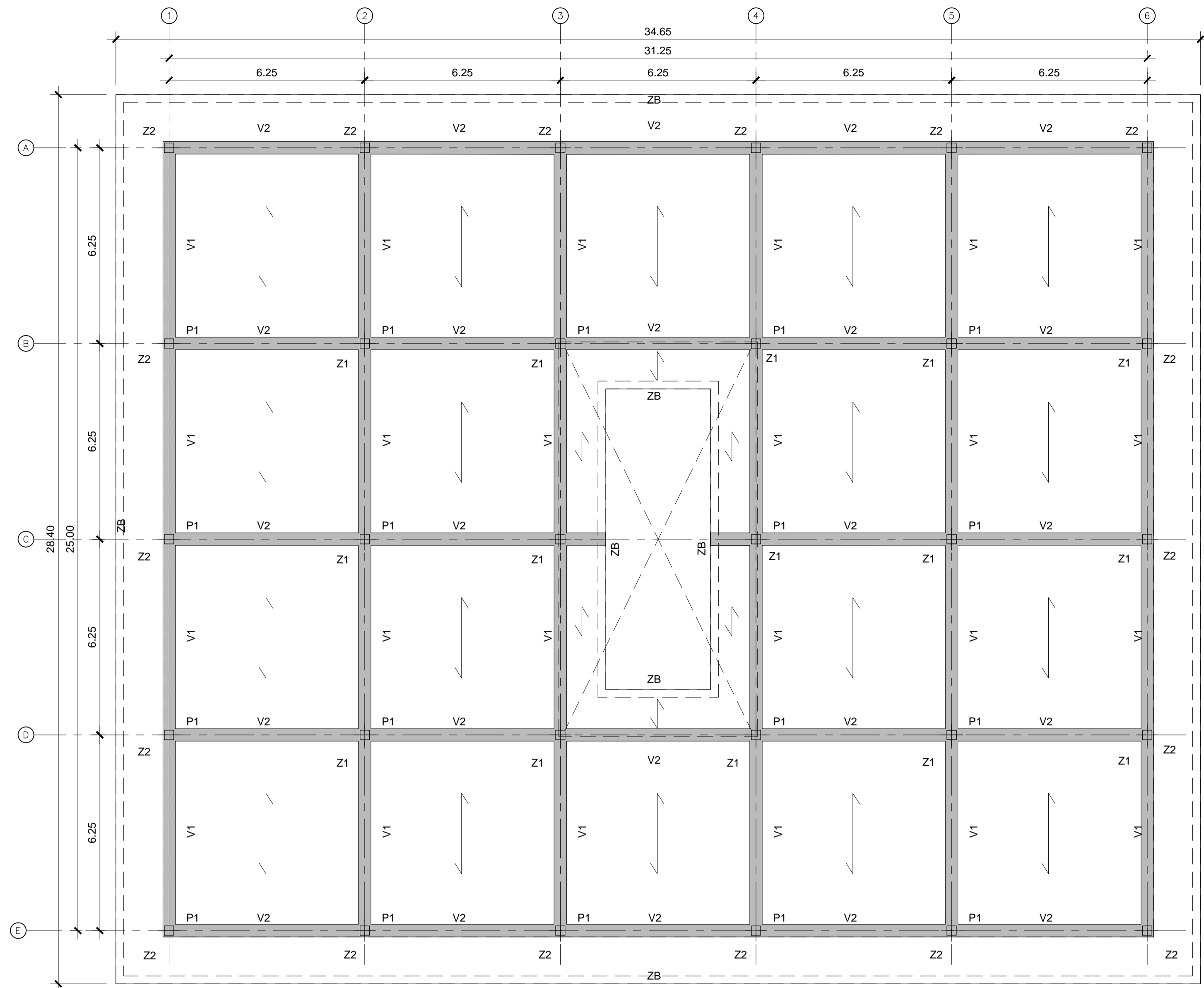
PLANTA DE COBERTURA-LAJE ESCALA 1:100
