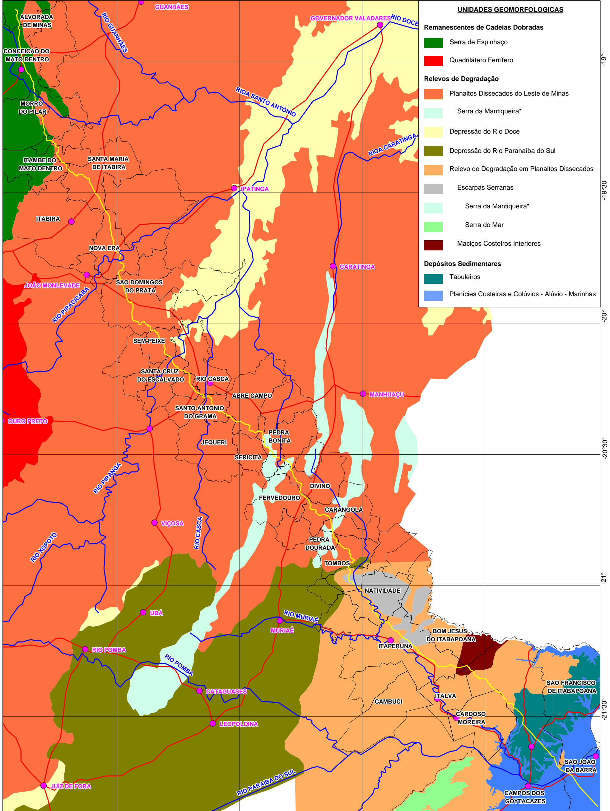
FIGURA 4.25 - Mapa de compartimentação geomorfológica mostrando as principais unidades da área de estudo do mineroduto Minas - Rio.
