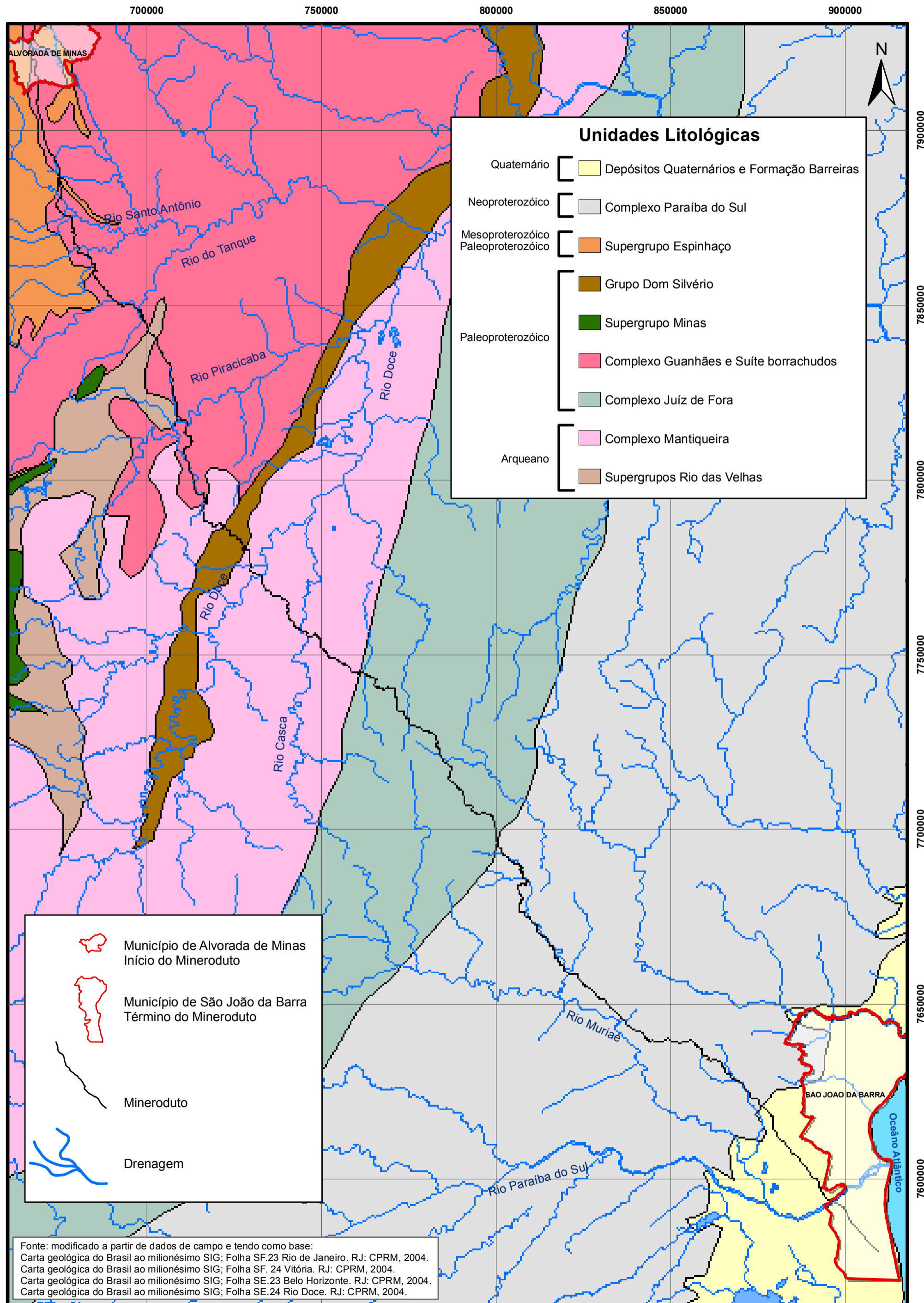
FIGURA 4.23 - Mapa geológico da porção sudeste do Brasil com o mineroduto em destaque.
