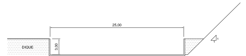
SEÇÃO VERTEDOURO ESC. 1:200
